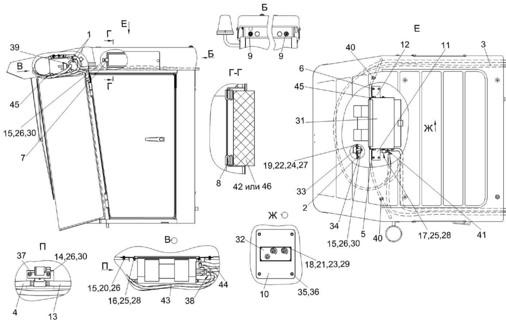
Рисунок 155 – Установка испарителя КЗК-12-0113040-02
