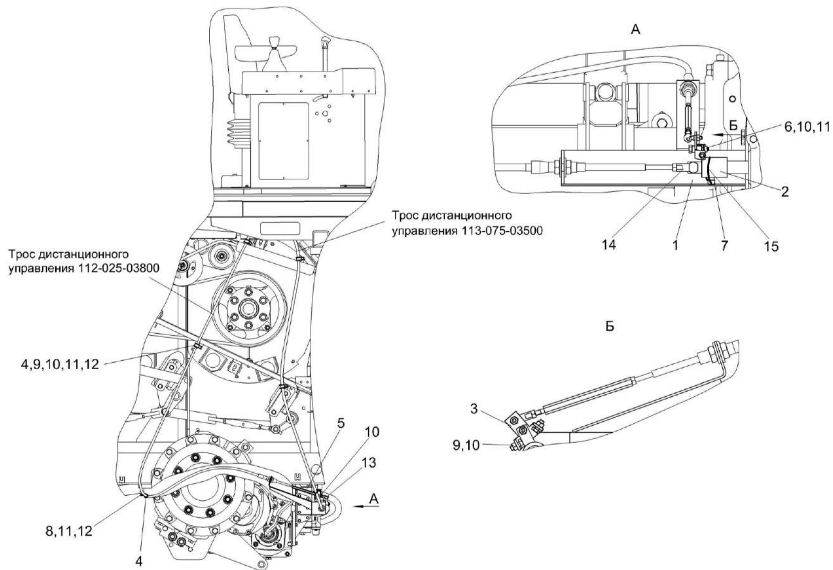
Рисунок 179 – Установка механизма КПП КЗК-12-0122500
