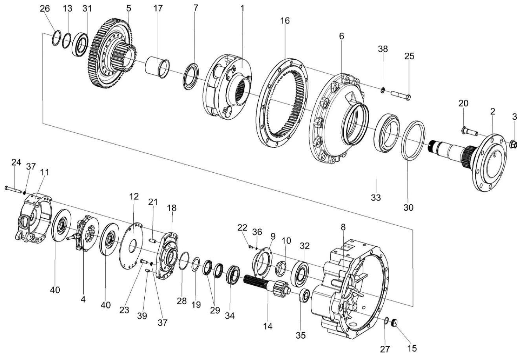
Рисунок 80 – Редуктор бортовой КЗК-10-0107200-04 (лист 2)
