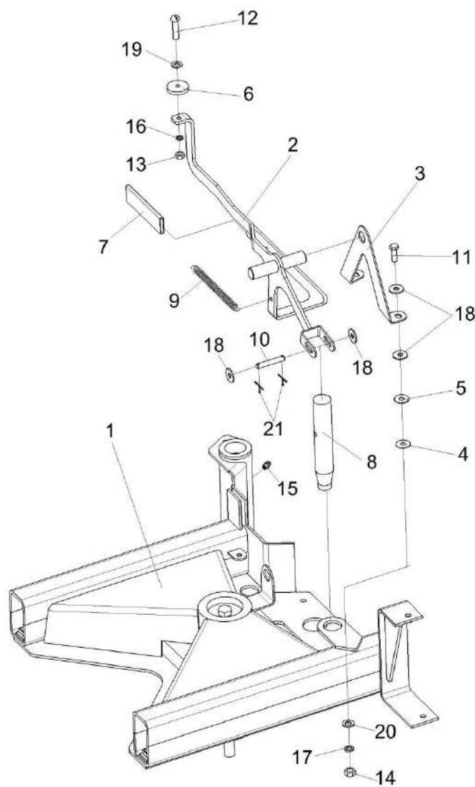
Рисунок 185 – Рама КЗК-12-0117010Б
