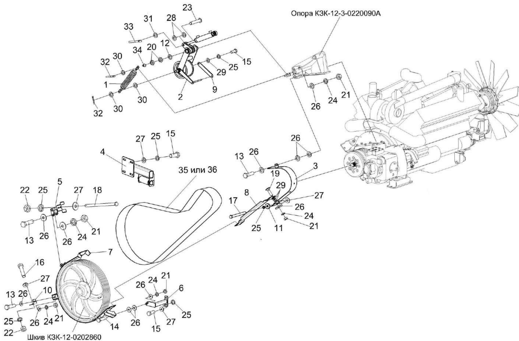
Рисунок 238 – Привод главного контрпривода КЗК-12-3-0220000
