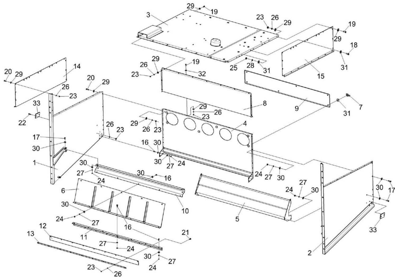
Рисунок 229 – Капот КЗК-2-12-0228300
