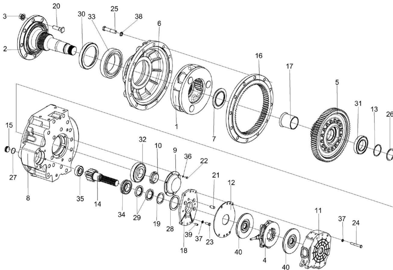
Рисунок 78 – Редуктор бортовой КЗК-10-0107200 (лист 2)
