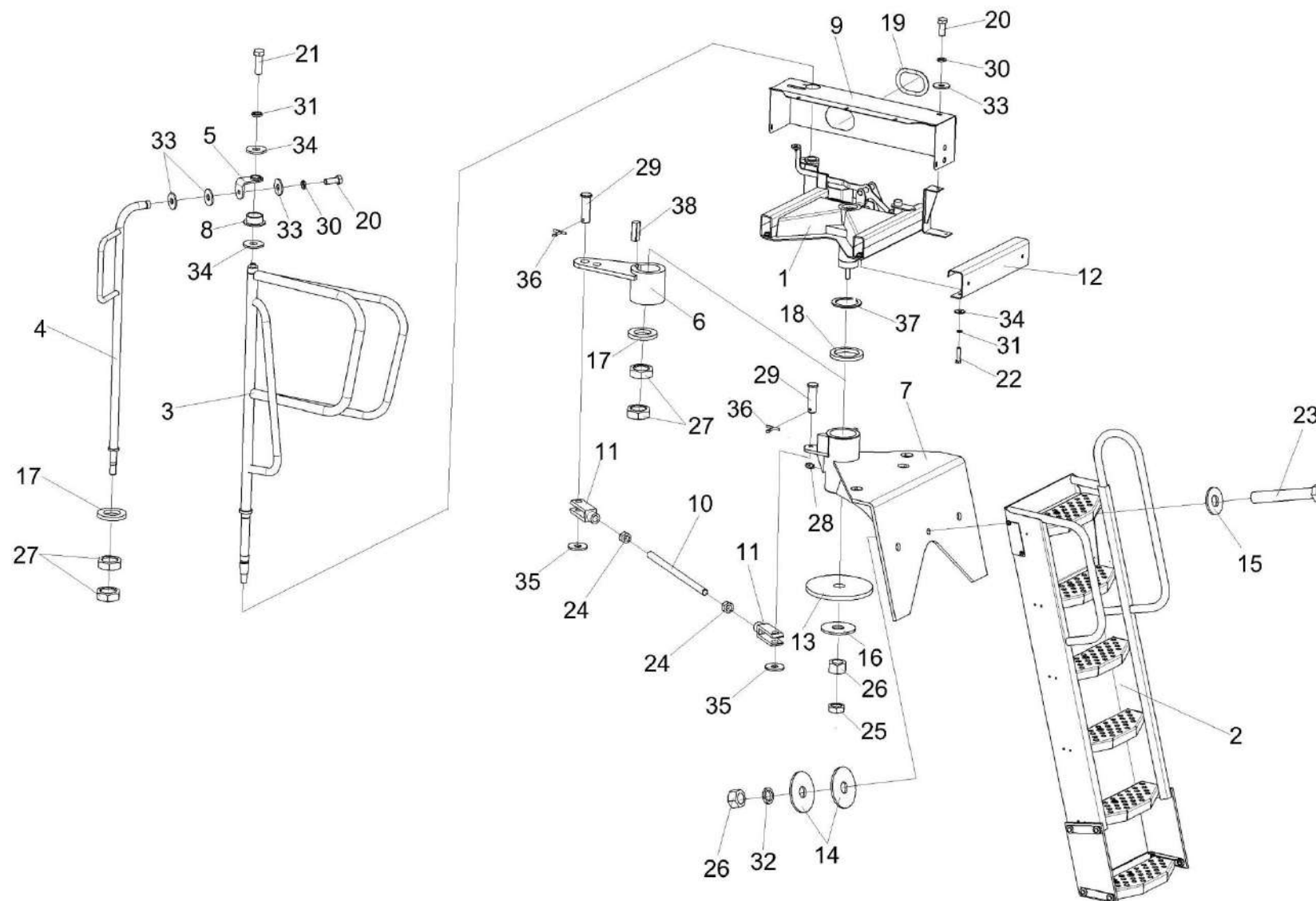
Рисунок 184 – Установка трапа КЗК-12-0117000А
