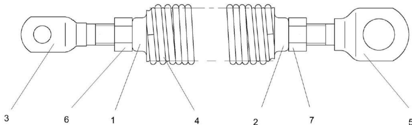
Рисунок 247 – Пружина КЗК-10-0100720А
