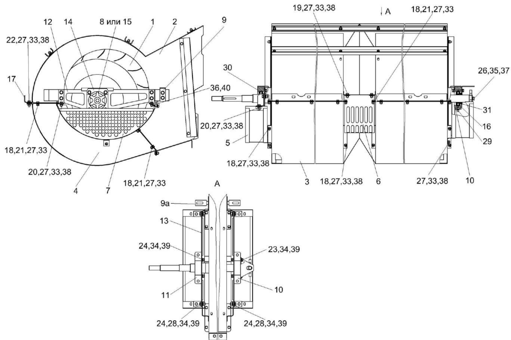
Рисунок 95 – Вентилятор КЗК-10-0217000
