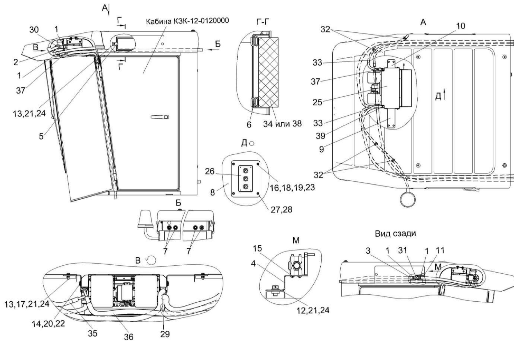
Рисунок 154 – Установка испарителя КЗК-12-0113040-01
