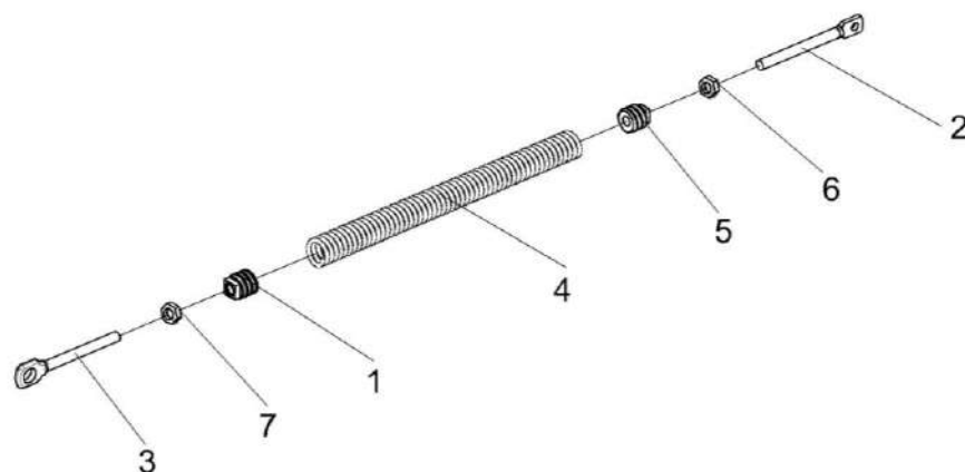
Рисунок 242 – Пружина КЗК 0202840А-03
