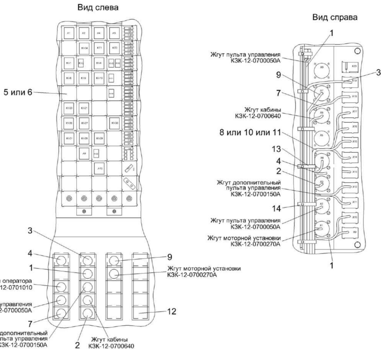
Рисунок 10 – Электрооборудование шкафа электрического КЗК-12-0116000А
