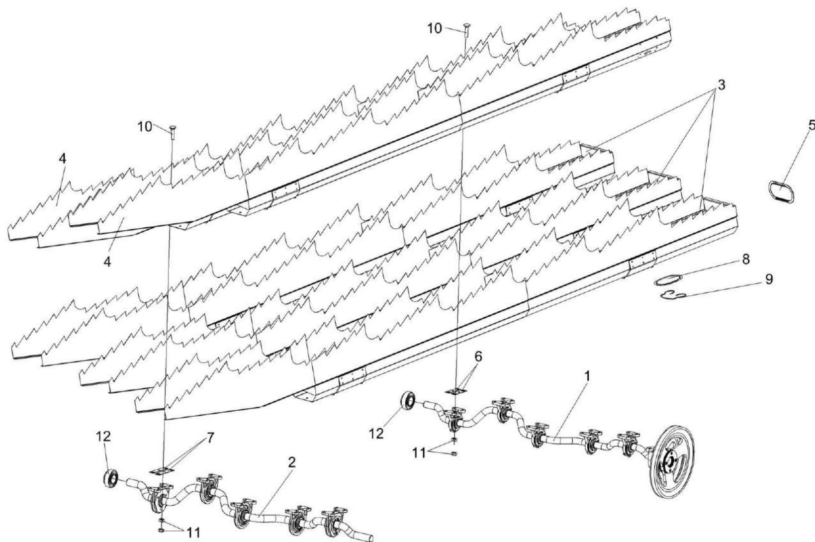
Рисунок 68 – Соломотряс КЗК-12-0212040
