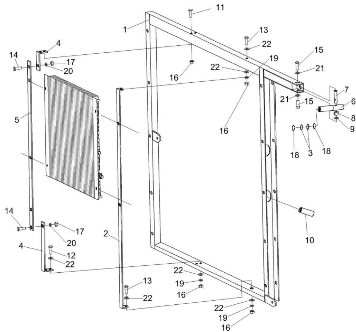
Рисунок 218 – Рама КЗК-12-3-0112080
