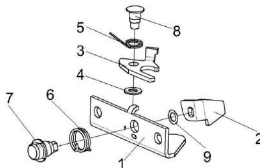
Рисунок 192 – Замок КВС-1-0160240
