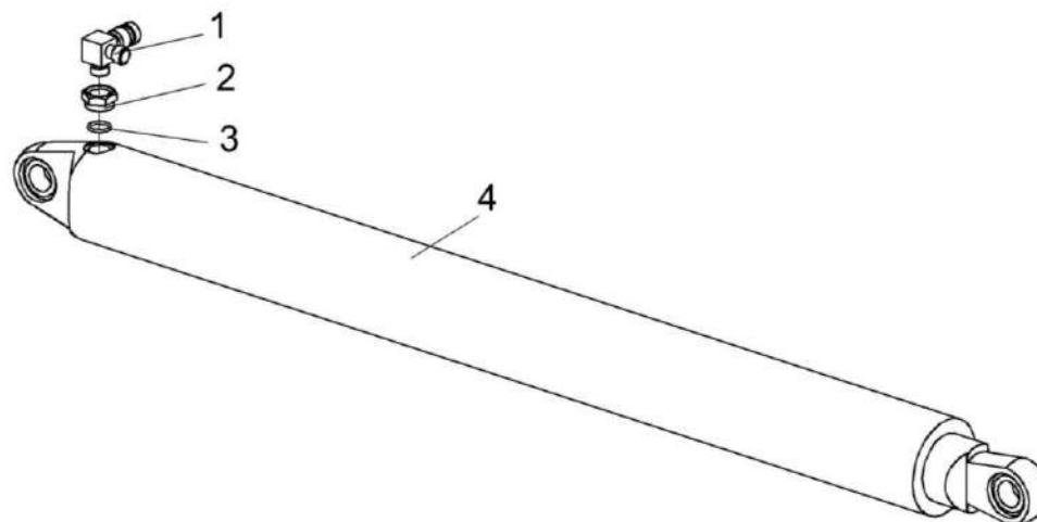
Рисунок 268 – Гидроцилиндр КЗК-12-0602740-01
