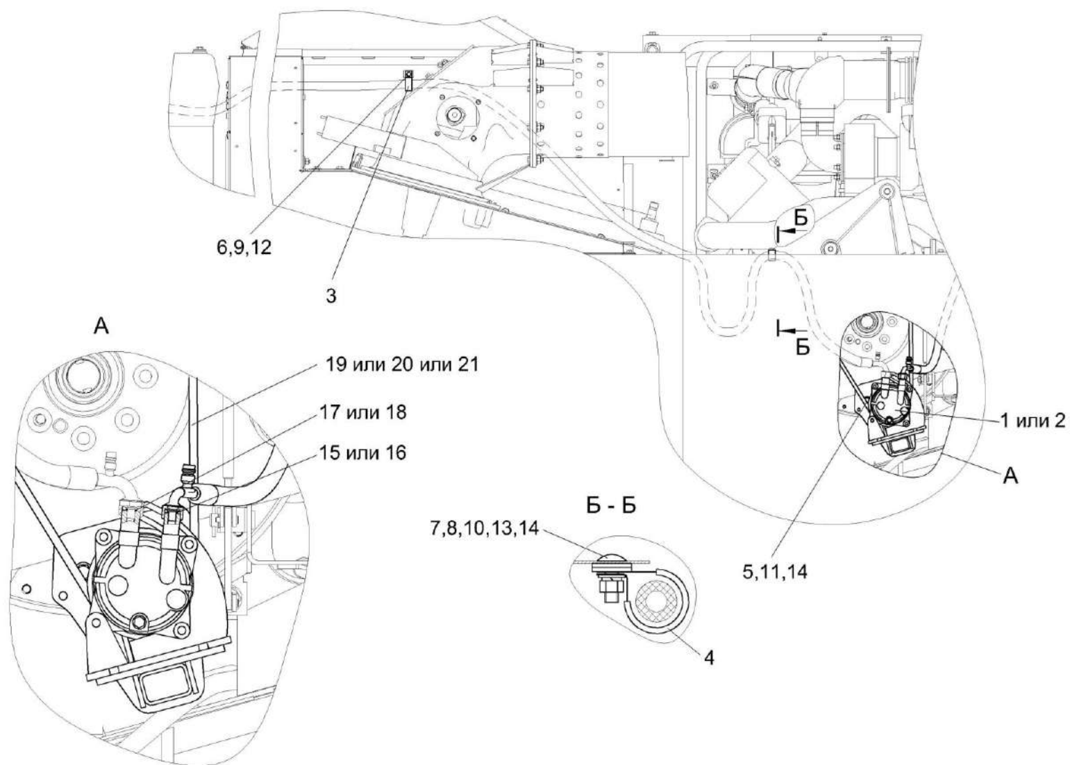
Рисунок 151 – Установки компрессора КЗК-12-0113030-01, КЗК-12-0113030-02 (лист 2)
