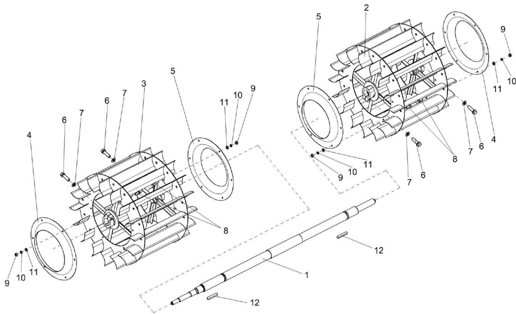
Рисунок 96 – Крылач КЗК-10-0217020
