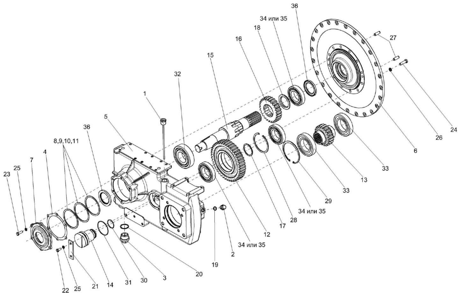
Рисунок 211 – Мультипликатор КЗК-12-0114000-01
