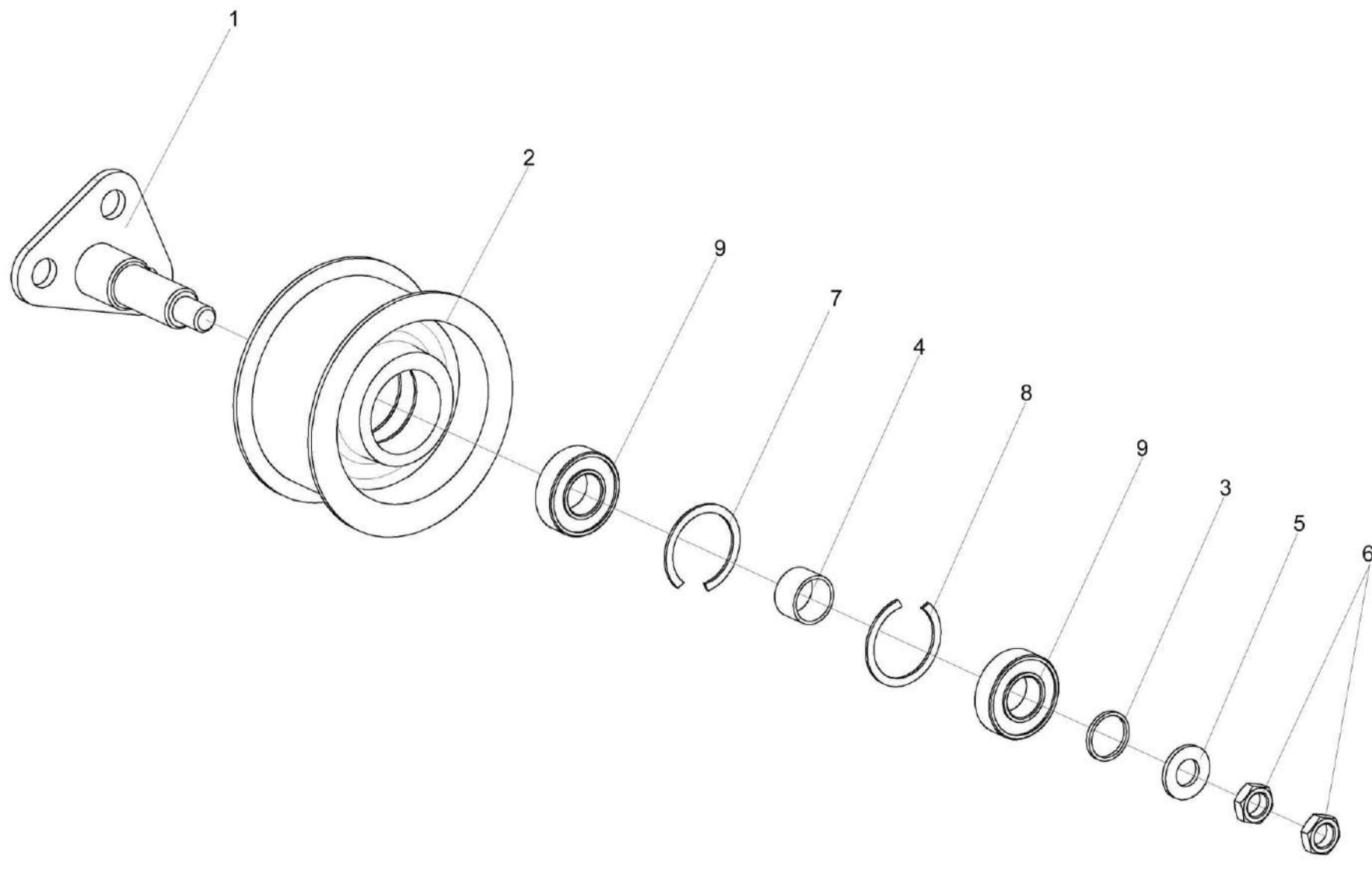
Рисунок 31 – Ролик натяжной КЗК-12-0125090
