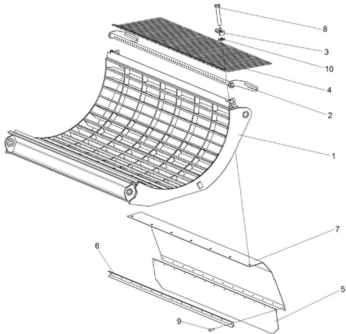
Рисунок 62 – Подбарабанье КЗК-12-0103000
