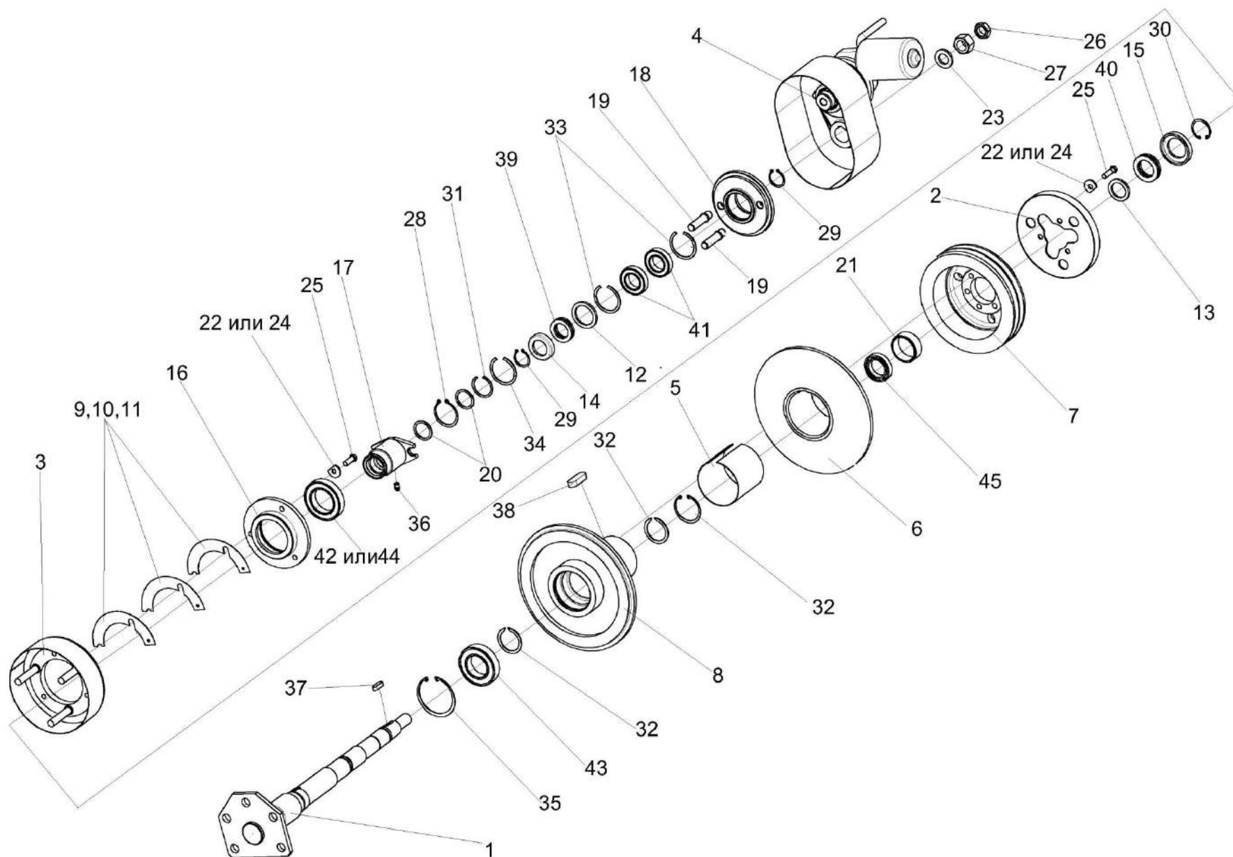
Рисунок 48 – Контрпривод вариатора K3K-12-0202500A
