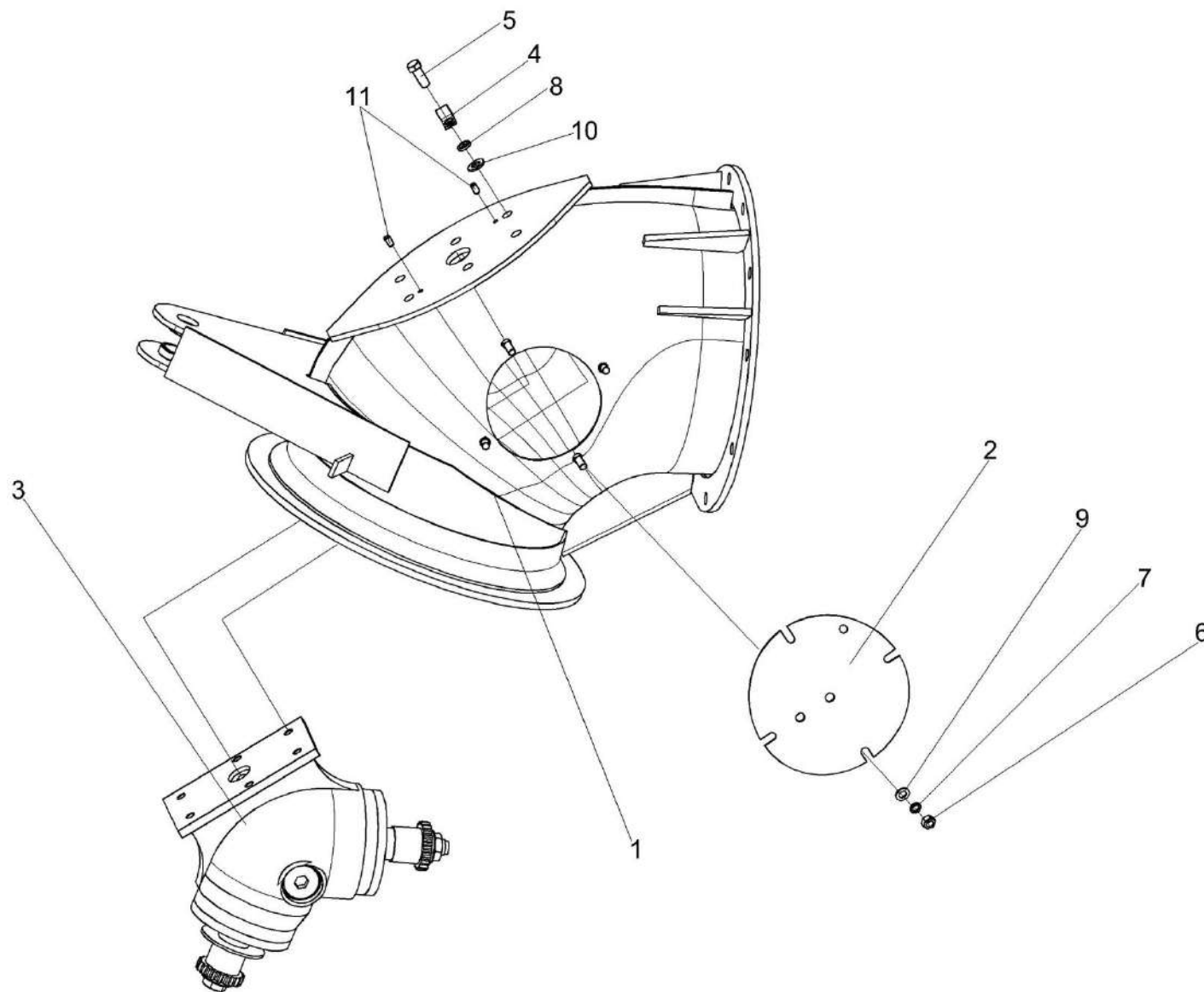
Рисунок 108 – Отвод с редуктором K3K-12-0206090A
