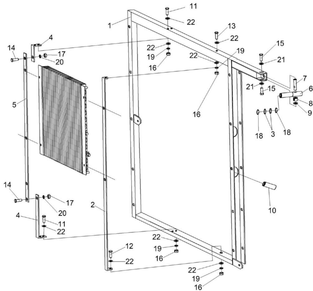
Рисунок 194 – Рама K3K-12-3-0112080
