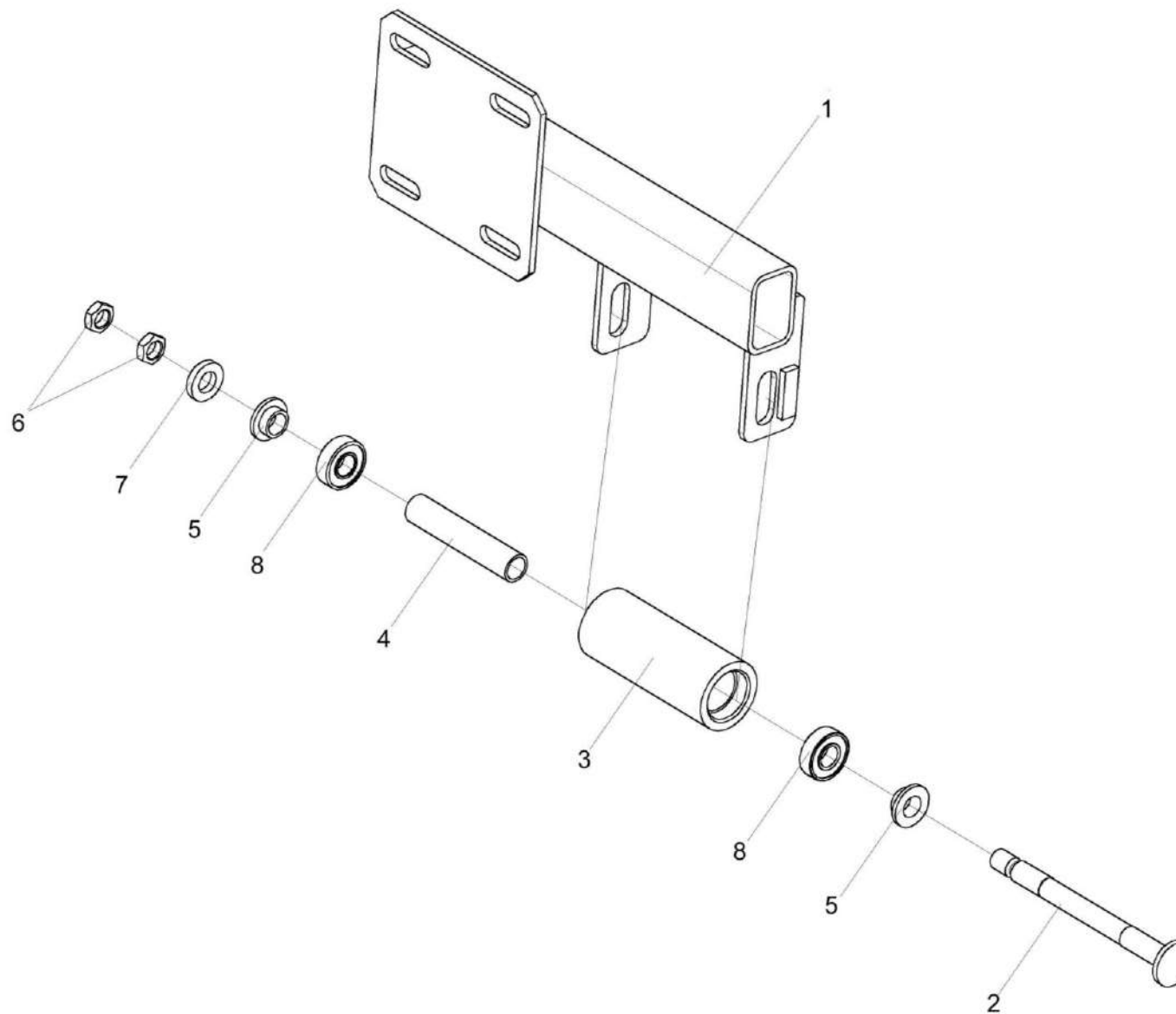
Рисунок 210 – Ограничитель K3K-12-3-0220260
