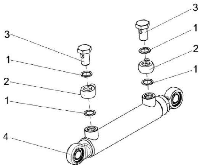
Рисунок 232 – Гидроцилиндр КЗК-12-0602730
