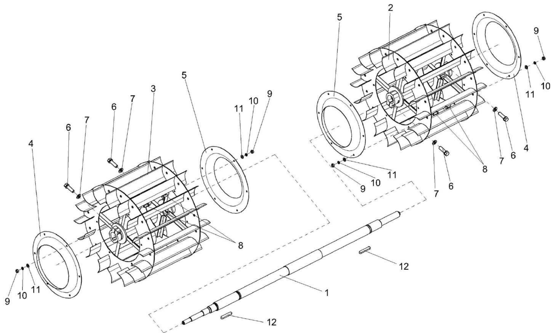
Рисунок 86 – Крылач КЗК-10-0217010
