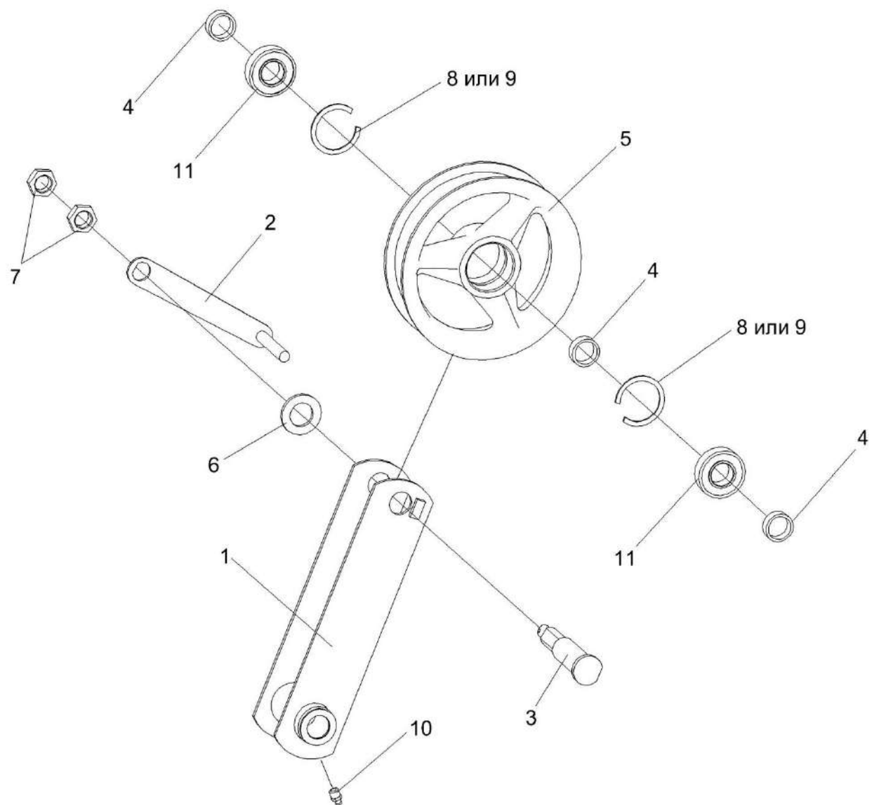
Рисунок 119 – Рычаг КЗК-12-0221110
