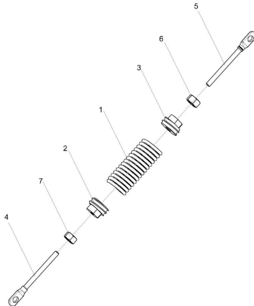
Рисунок 208 – Пружина КЗК-12-3-0220050
