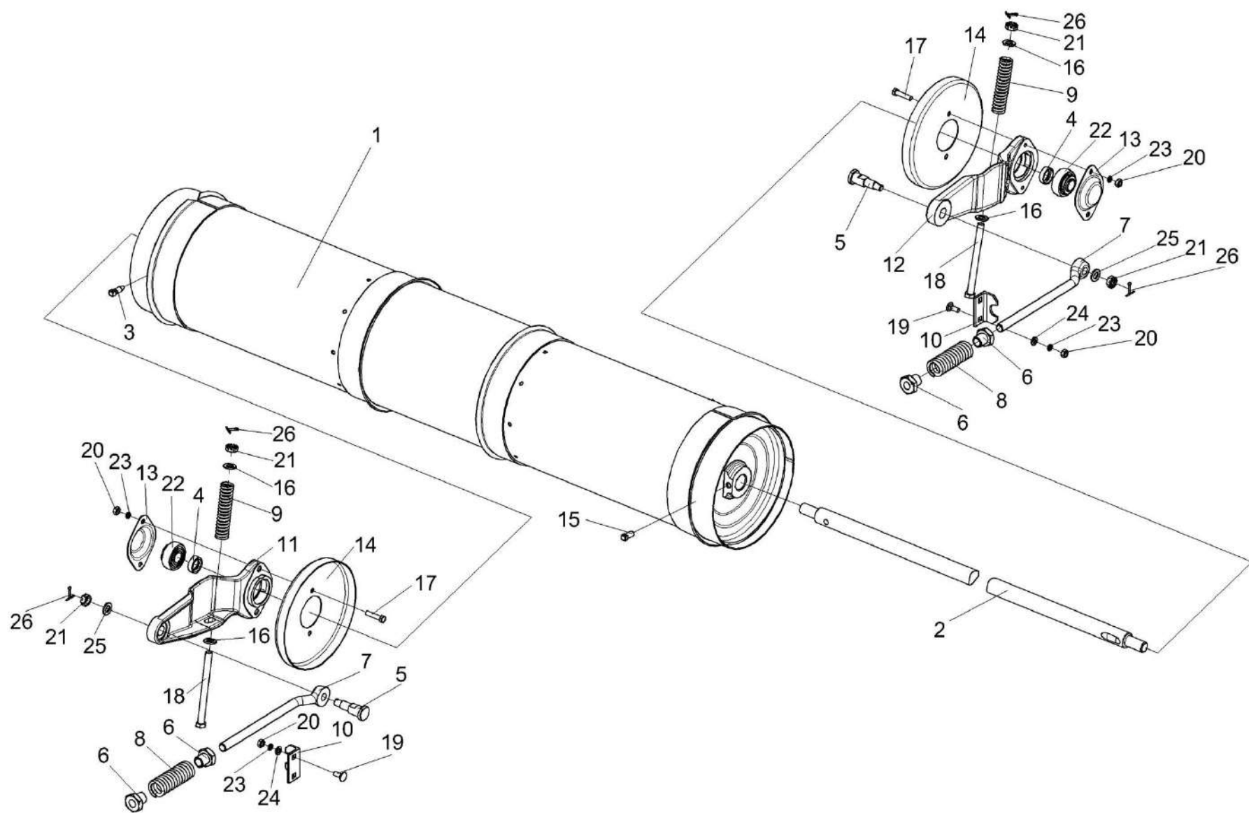
Рисунок 23 – Установка вала нижнего K3K-12-1806000A
