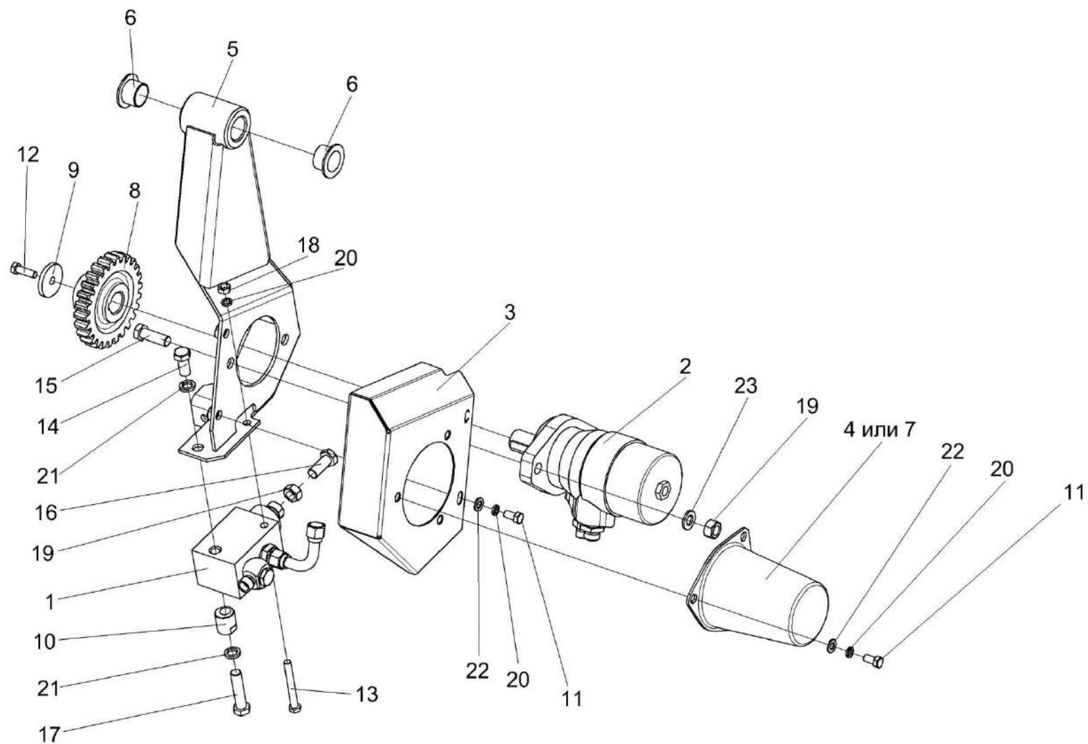
Рисунок 19 – Гидрореверс КЗК-12-1804100
