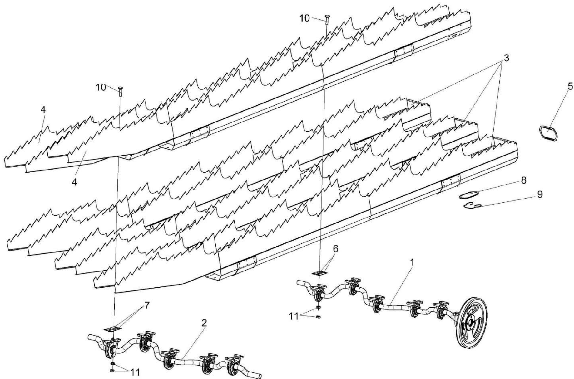
Рисунок 92 – Соломотряс КЗК-12-0212040
