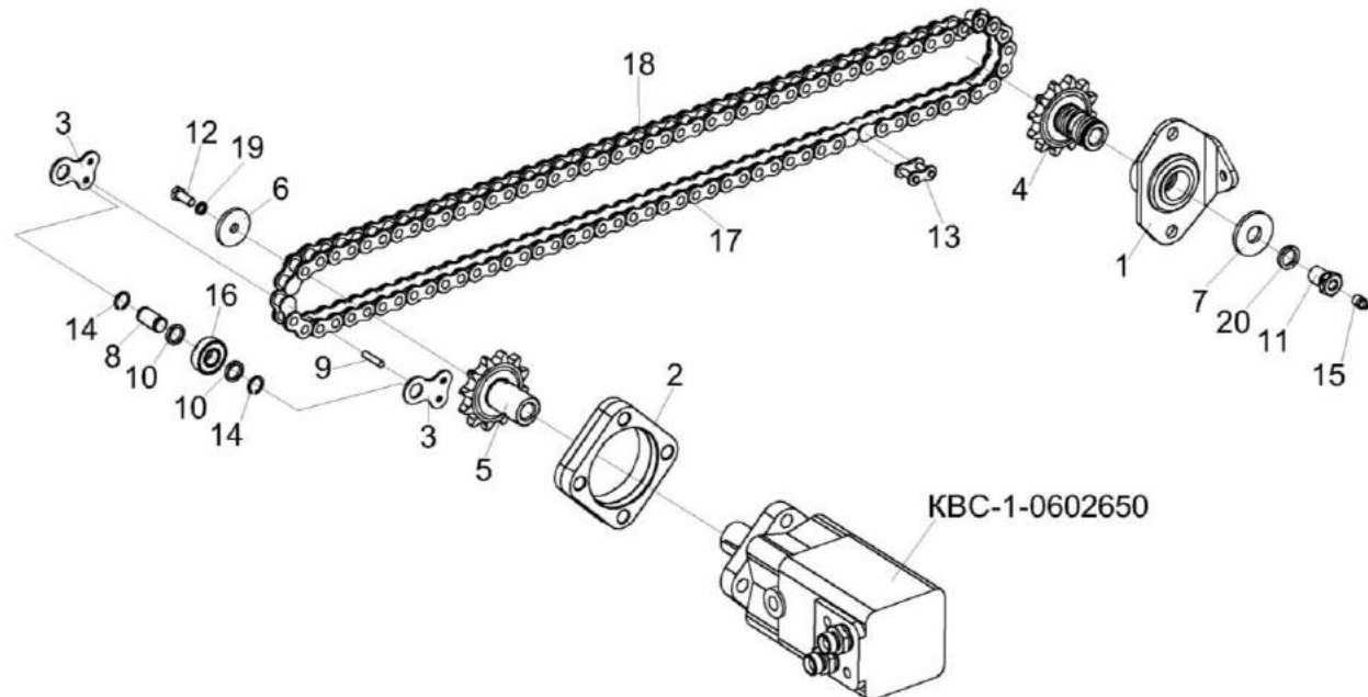
Рисунок 31 – Привод каретки KBC-2-0116510
