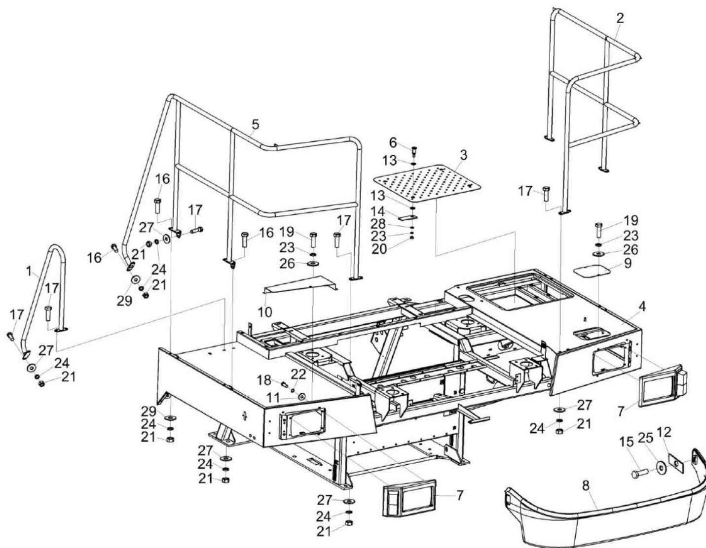
Рисунок 144 – Установка площадки входа КВС-2-0124000 (лист 1)
