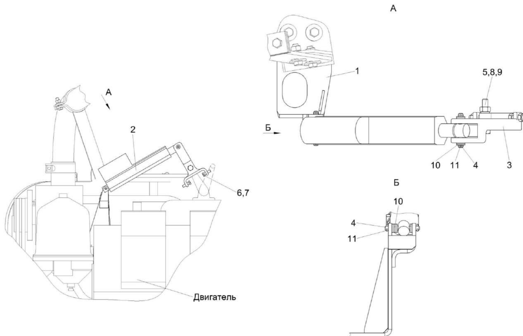
Рисунок 136 – Механизм управления топливным насосом КВС-5-0129300А
