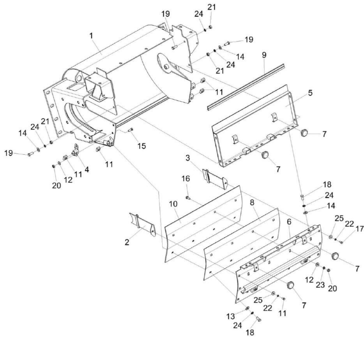
Рисунок 53 – Ускоритель выброса КВС-1-0142000 (лист 1)
