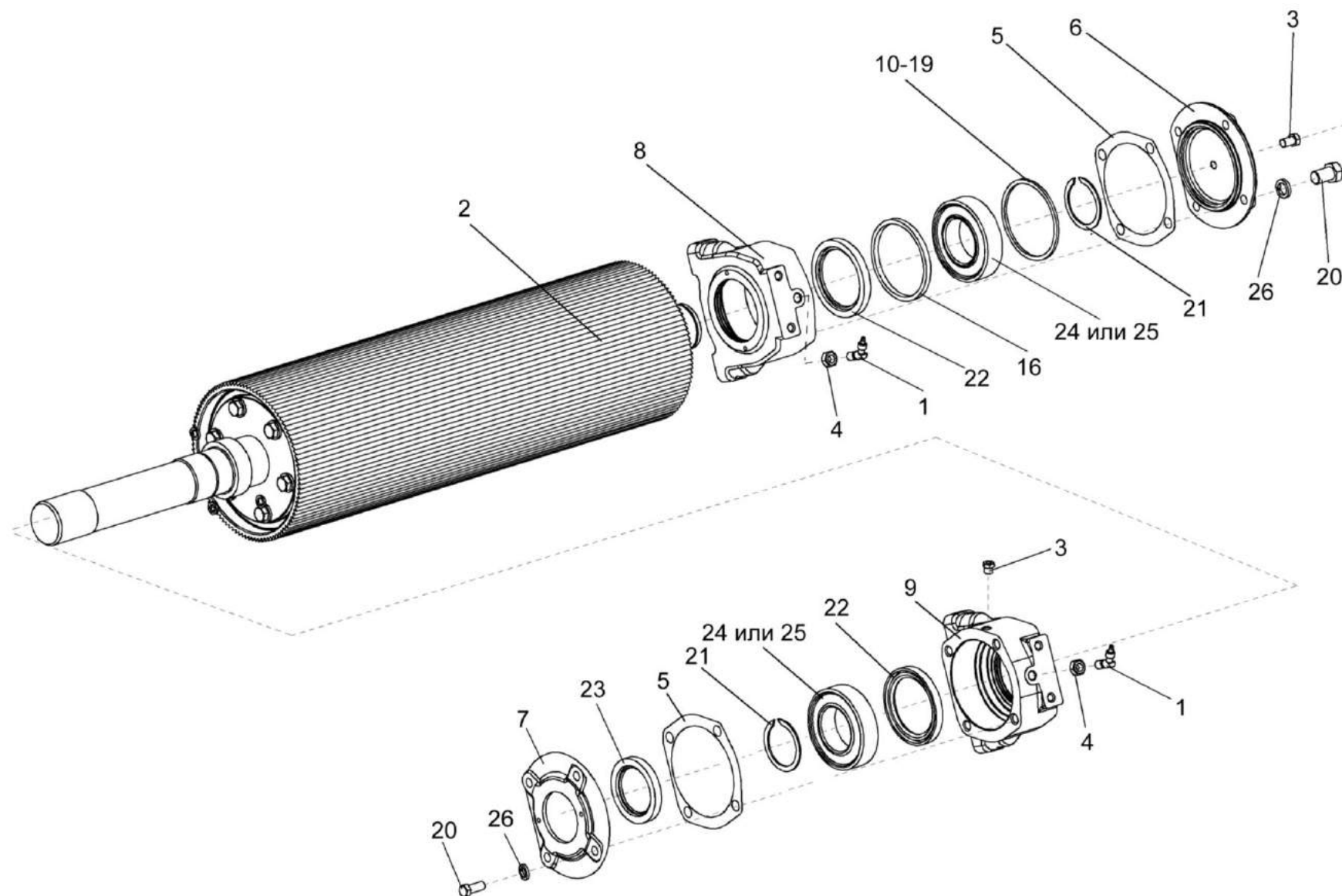
Рисунок 44 – Валец верхний КВС-1-0148600
