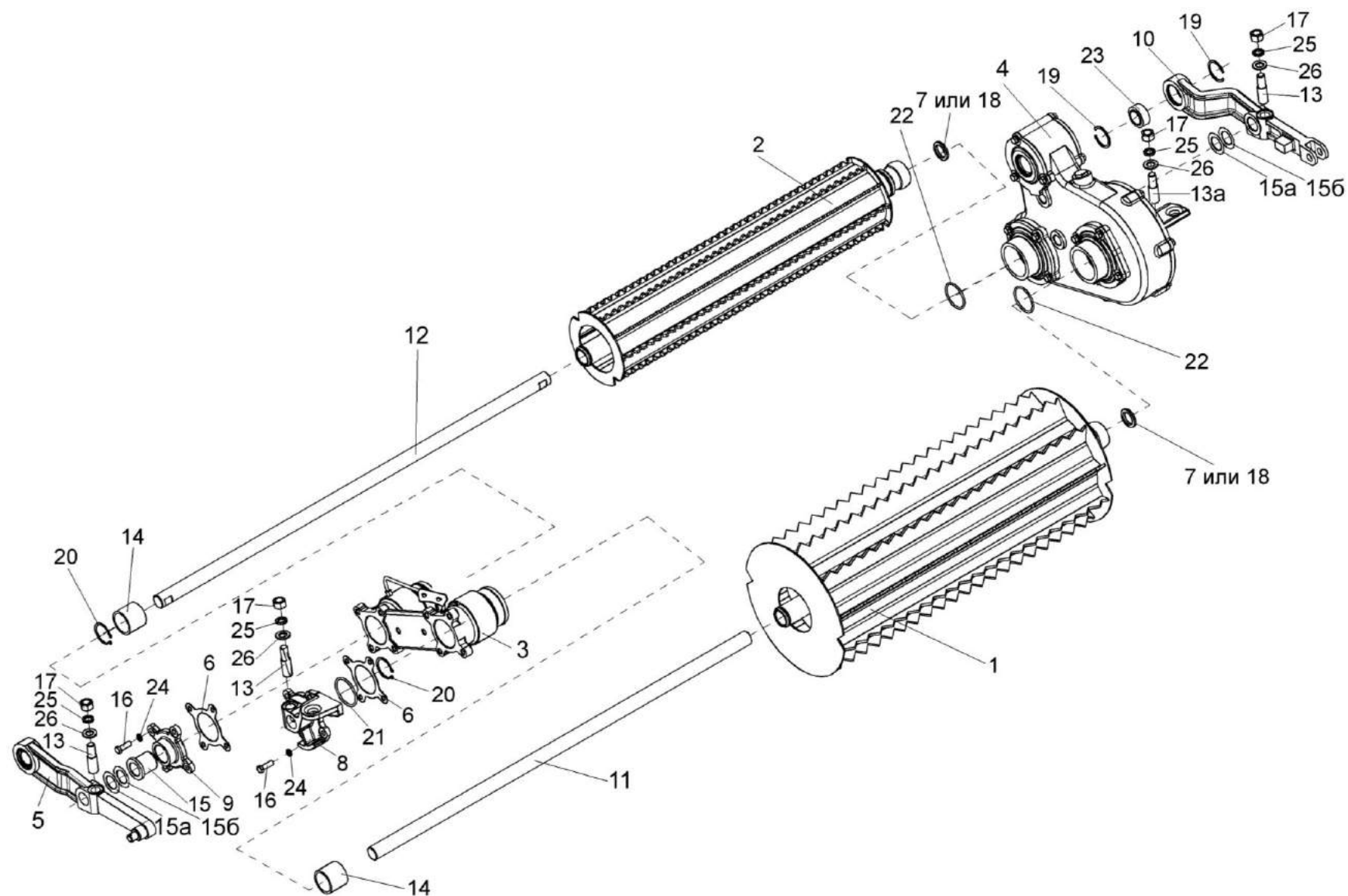
Рисунок 10 – Вальцы верхние КВС-2-0111100
