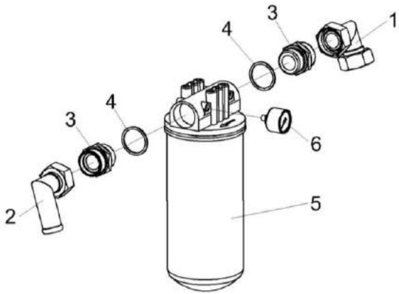
Рисунок 186 – Фильтр всасывающий КВС-2-0601090Б
