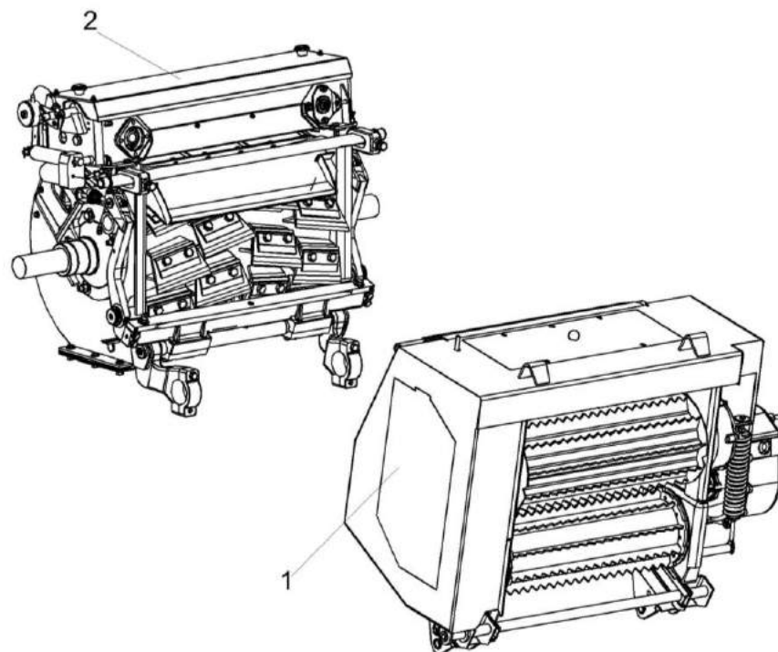
Рисунок 3 – Аппарат питающе-измельчающий КВС-2-0110000А-02
