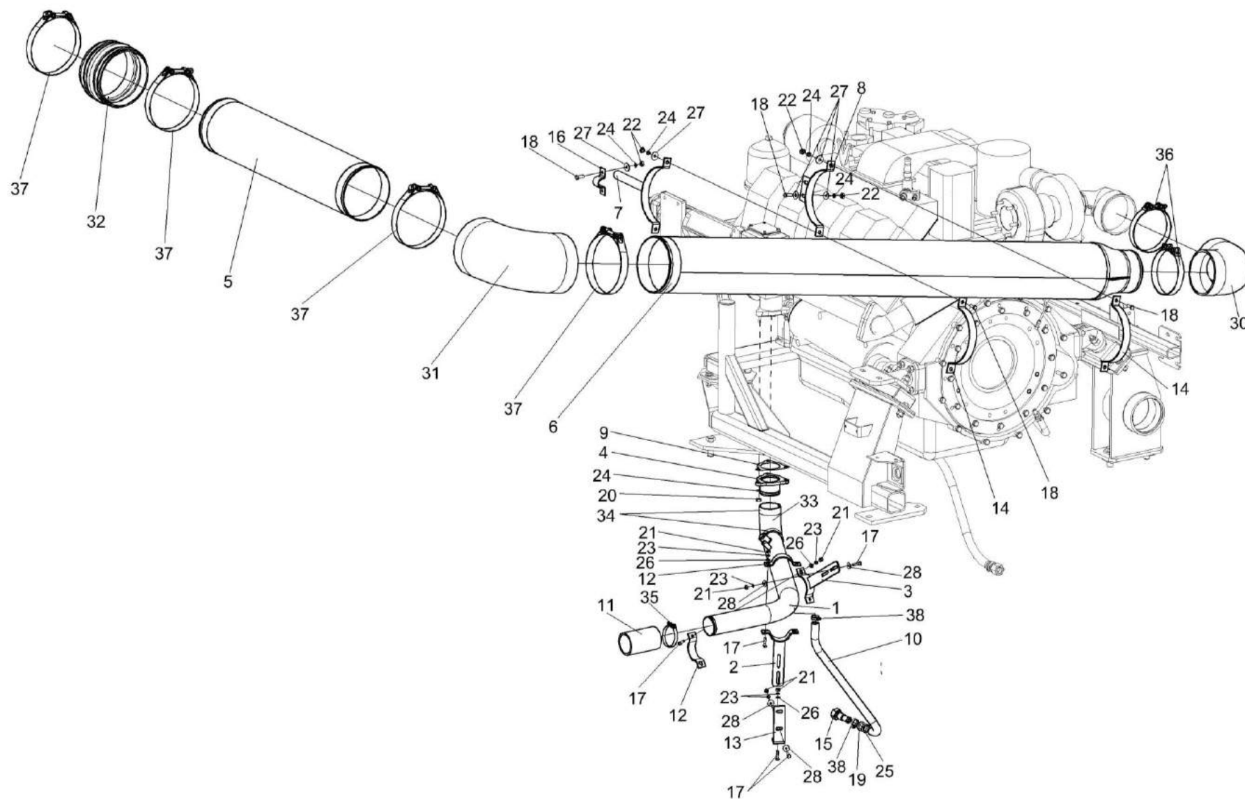
Рисунок 64 – Установка дизеля Д-280.1S2 KBC-5-0150000A (установка трубопроводов)
