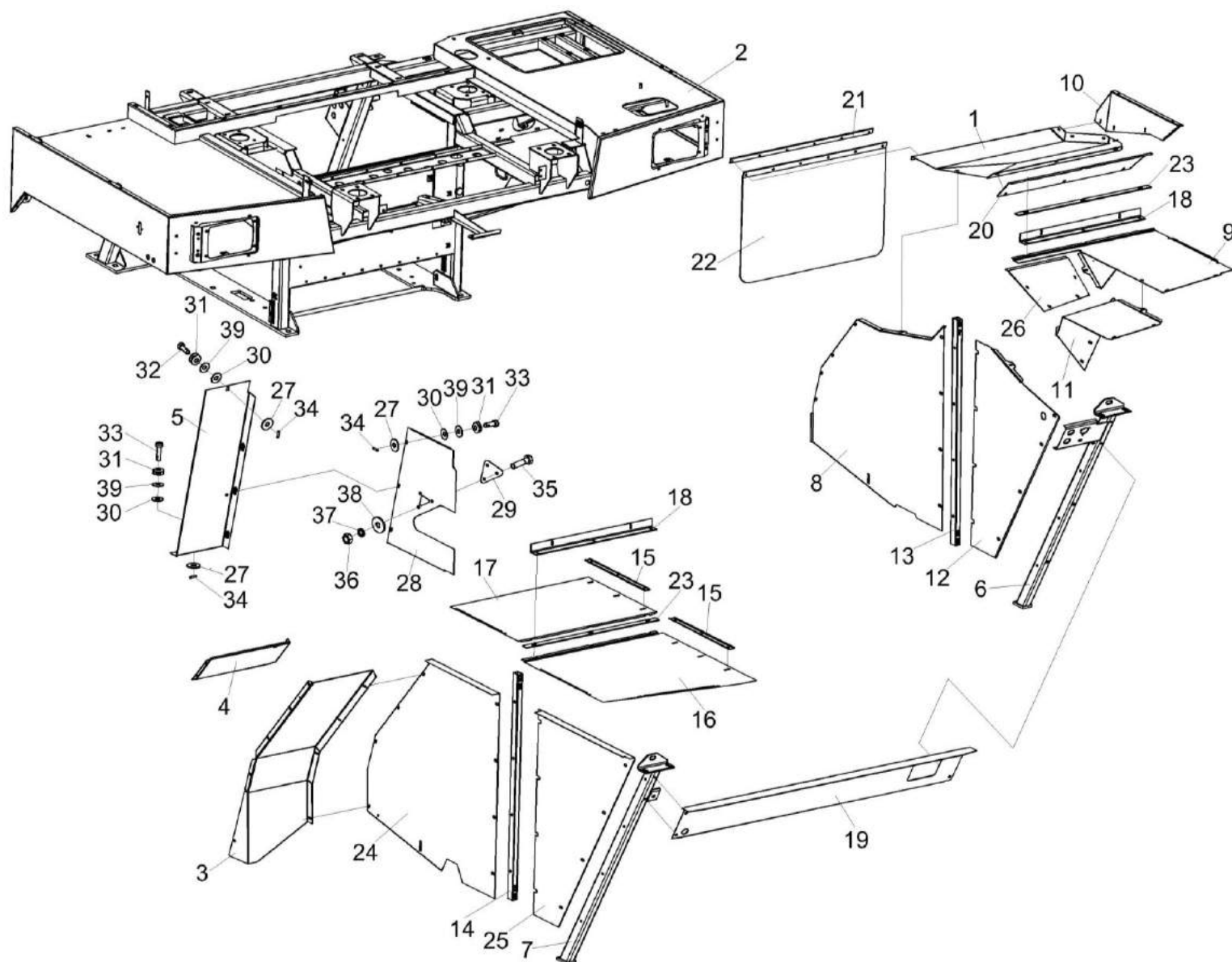
Рисунок 145 – Установка площадки входа КВС-2-0124000 (лист 2)
