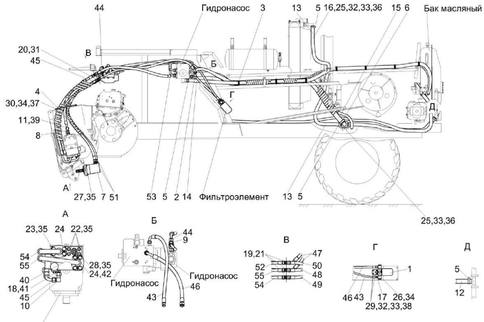
Гидромотор привода питающего аппарата Рисунок 172 – Гидросистема привода питающего аппарата и адаптеров комбайна КВК-800-36 КВК-5-0624000 (лист 1)
