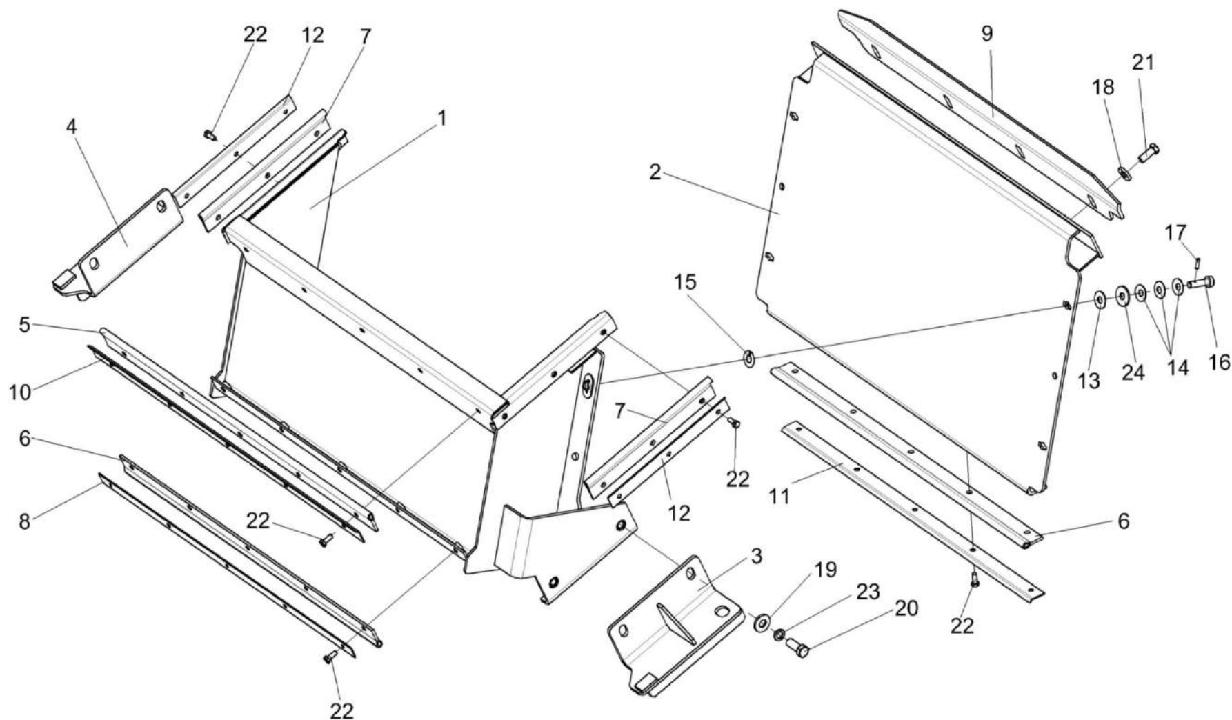
Рисунок 59 – Проставка КВС-1-0147500
