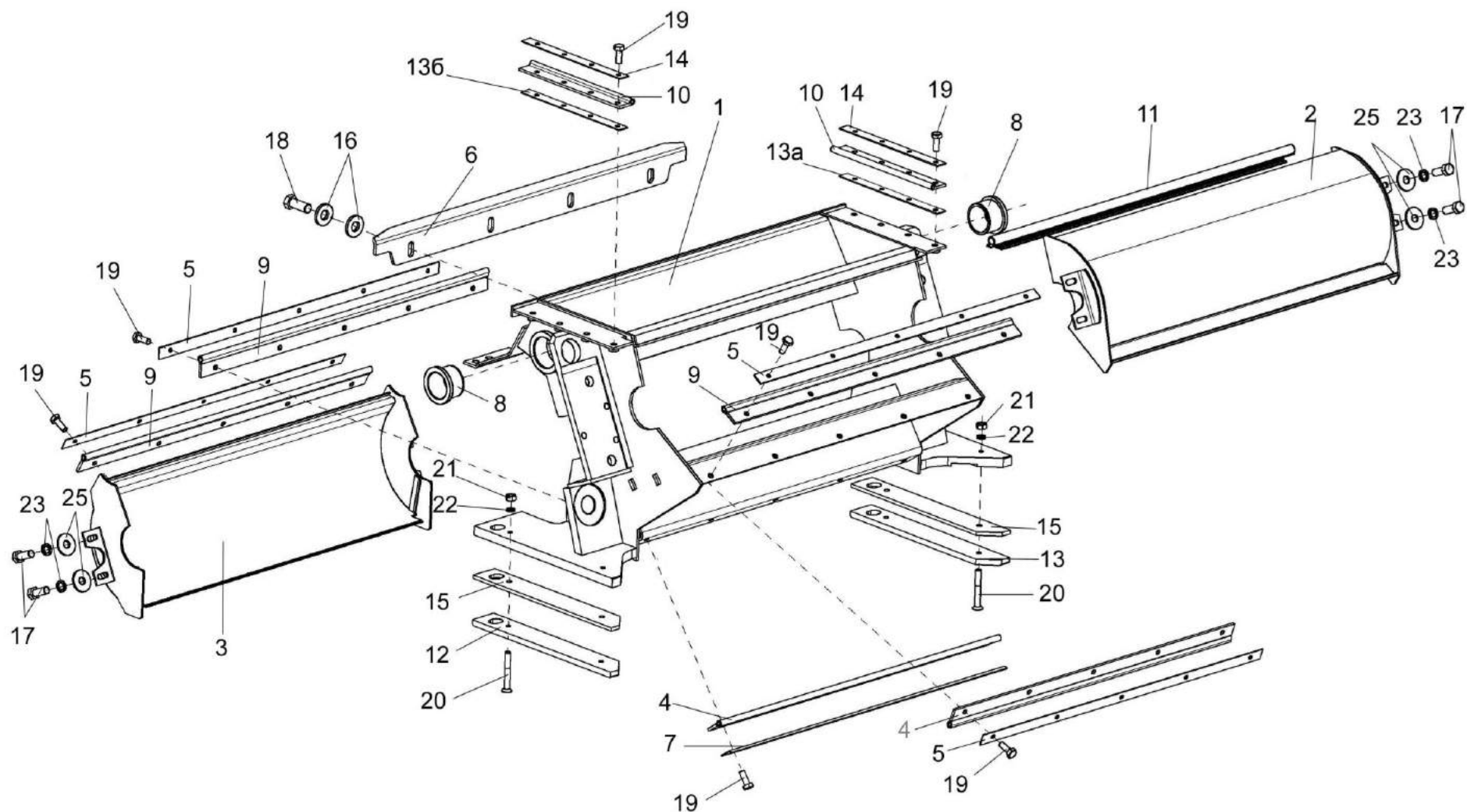
Рисунок 41 – Устройство доизмельчающее КВС-1-0148310 (установка кожухов)
