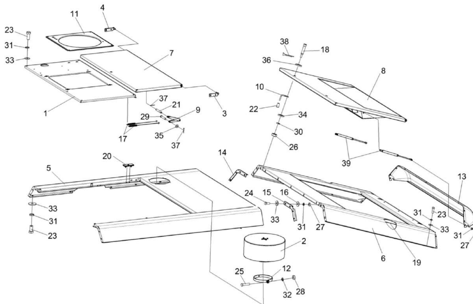
Рисунок 159 – Капот верхний КВС-2-0162000-02 (лист 1)
