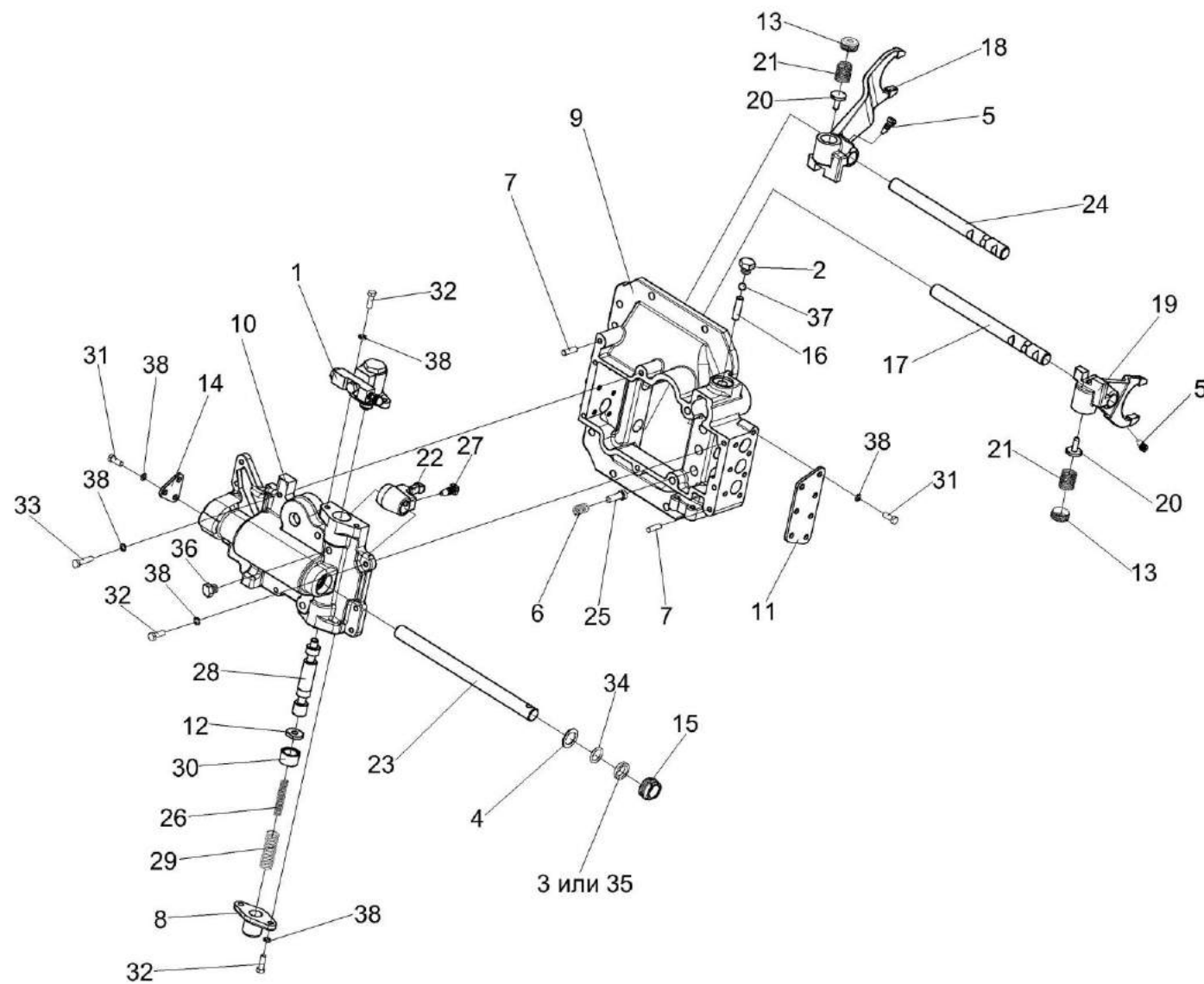
Рисунок 105 – Механизм переключения диапазонов 3518020-46160
