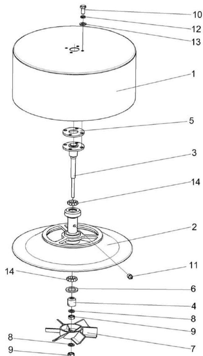
Рисунок 162 – Воздухозаборник вращающийся КВС-1-0153000А
