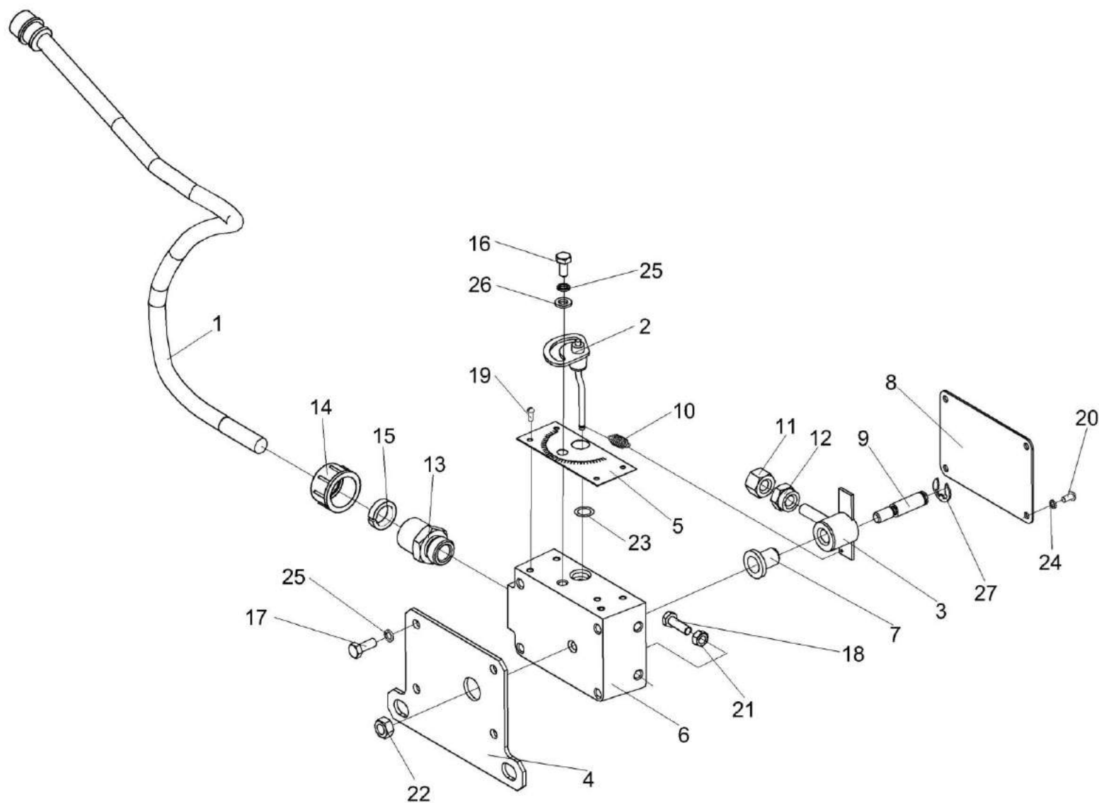
Рисунок 8 – Датчик камнедетектора КВС-1-0111070-01
