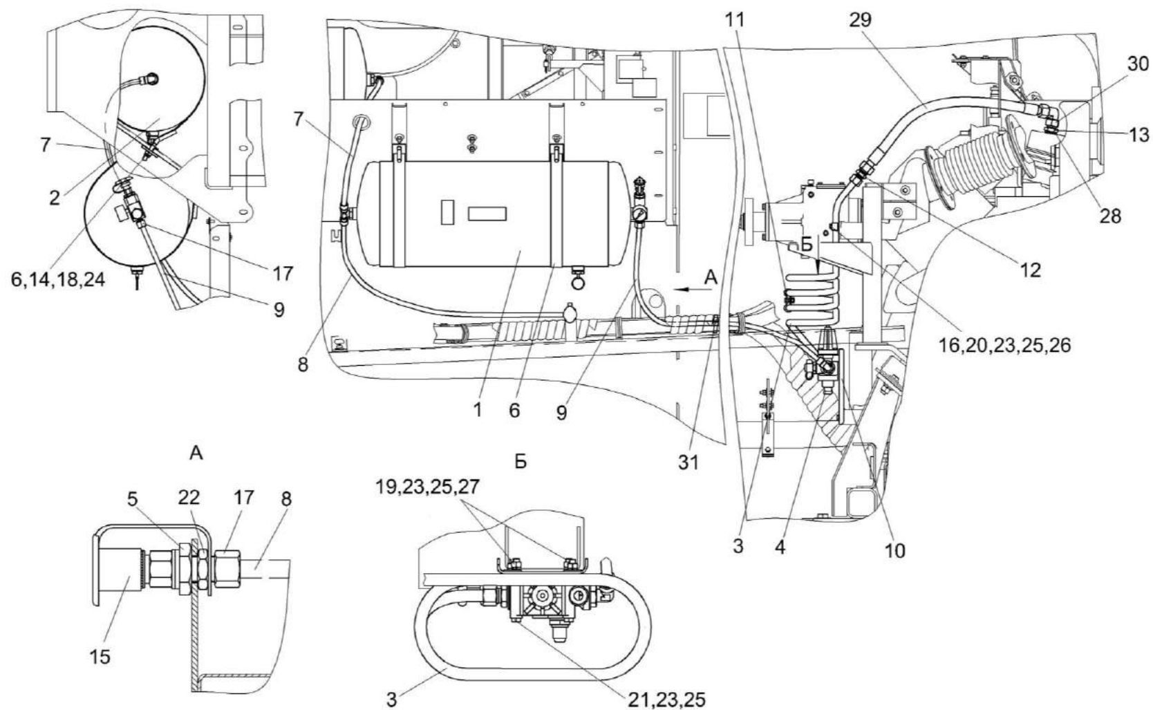
Рисунок 204 – Пневмосистема КВС-5-0800000
