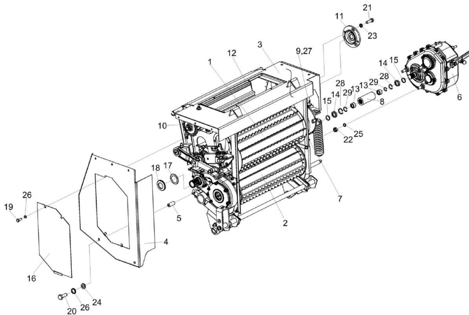
Рисунок 4 – Аппарат питающий КВС-2-0111000В-01
