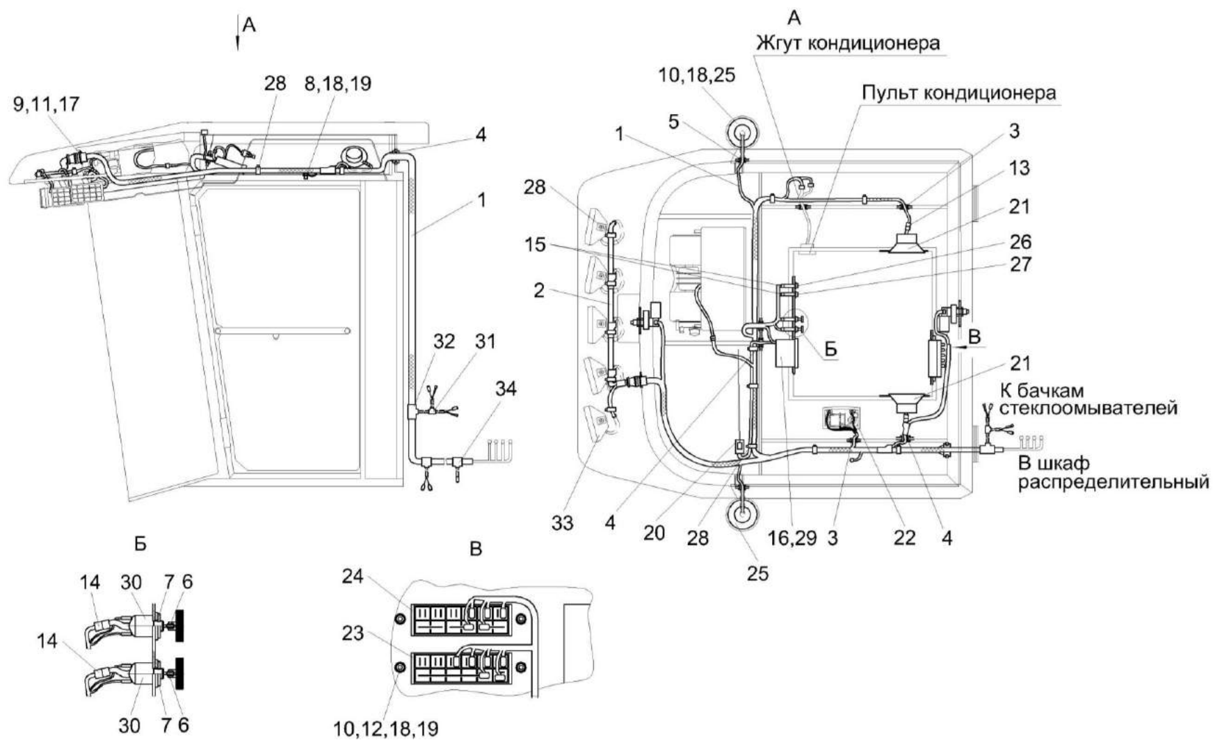
Рисунок 152 – Электрооборудование кабины КВС-2-0122000
