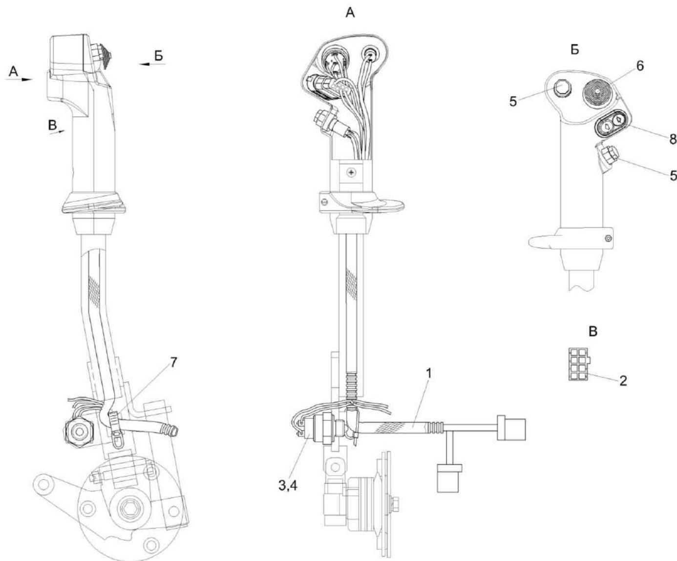
Рисунок 120 – Установка электрооборудования привода КВС-5-0724000
