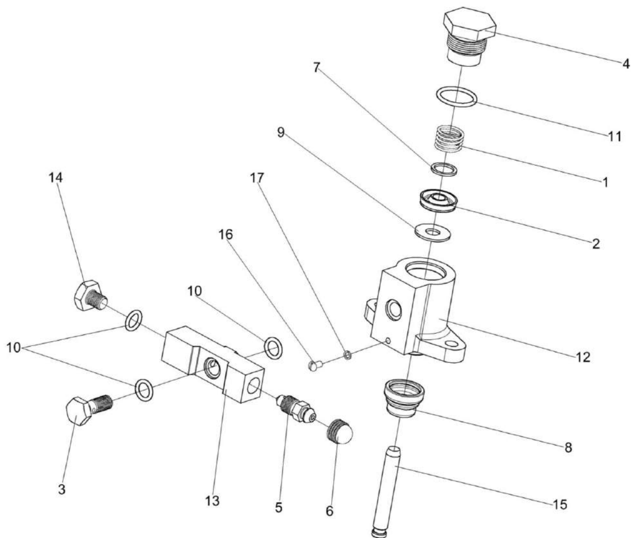
Рисунок 106 – Гидроцилиндр блокировки диапазонов 3518020-46330
