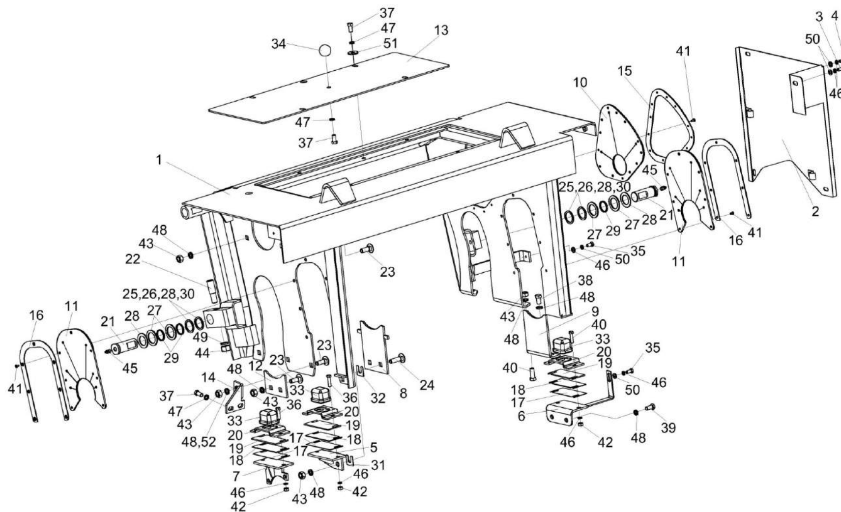
Рисунок 5 – Установка рамы верхней КВС-2-0111300Б
