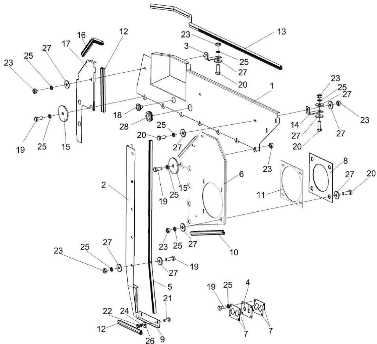
Рисунок 77 – Установка щитов КВС-5-0156000А
