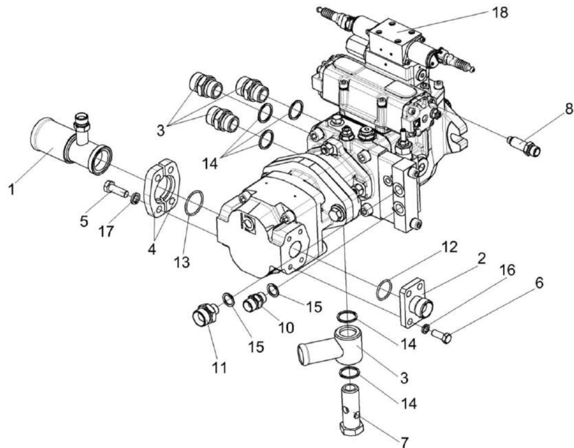
Рисунок 179 – Гидронасос двухсекционный KBC-5-0604330
