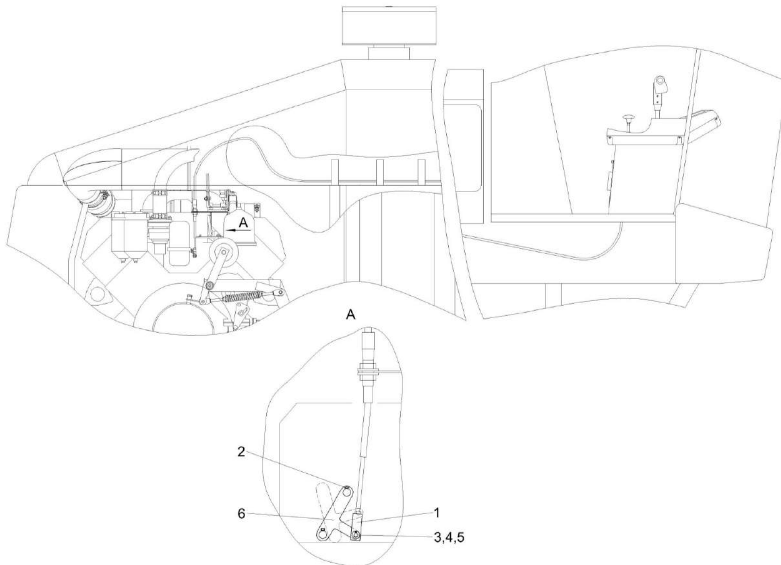
Рисунок 137 – Установка тросов управления двигателем КВС-5-0129600А
