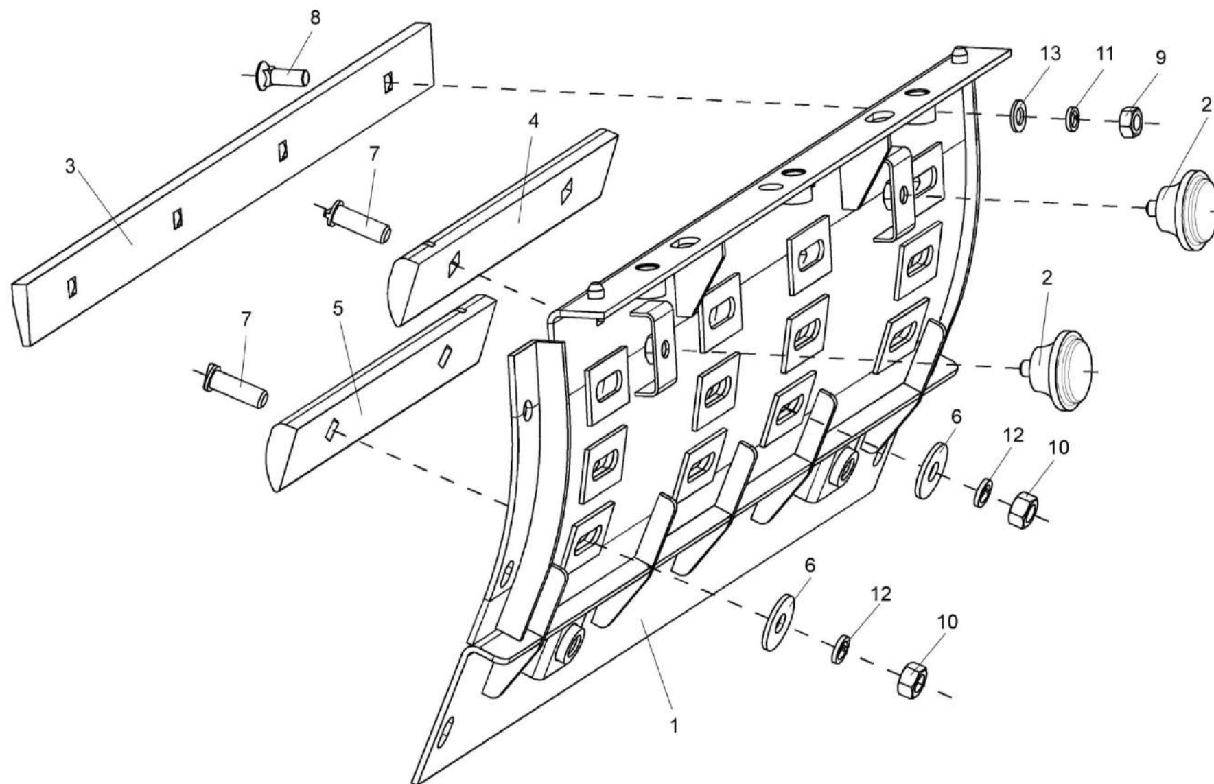
Рисунок 57 – Поддон бичевой КВС-1-0142320 (сменный)
