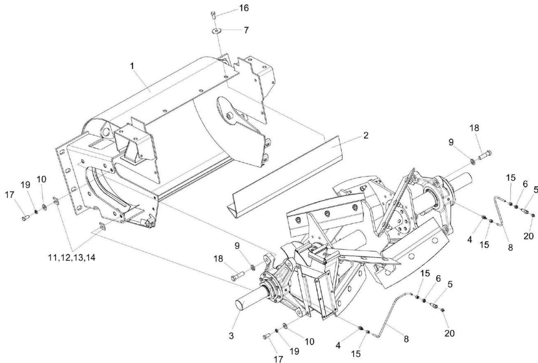
Рисунок 54 – Ускоритель выброса КВС-1-0142000 (лист 2)
