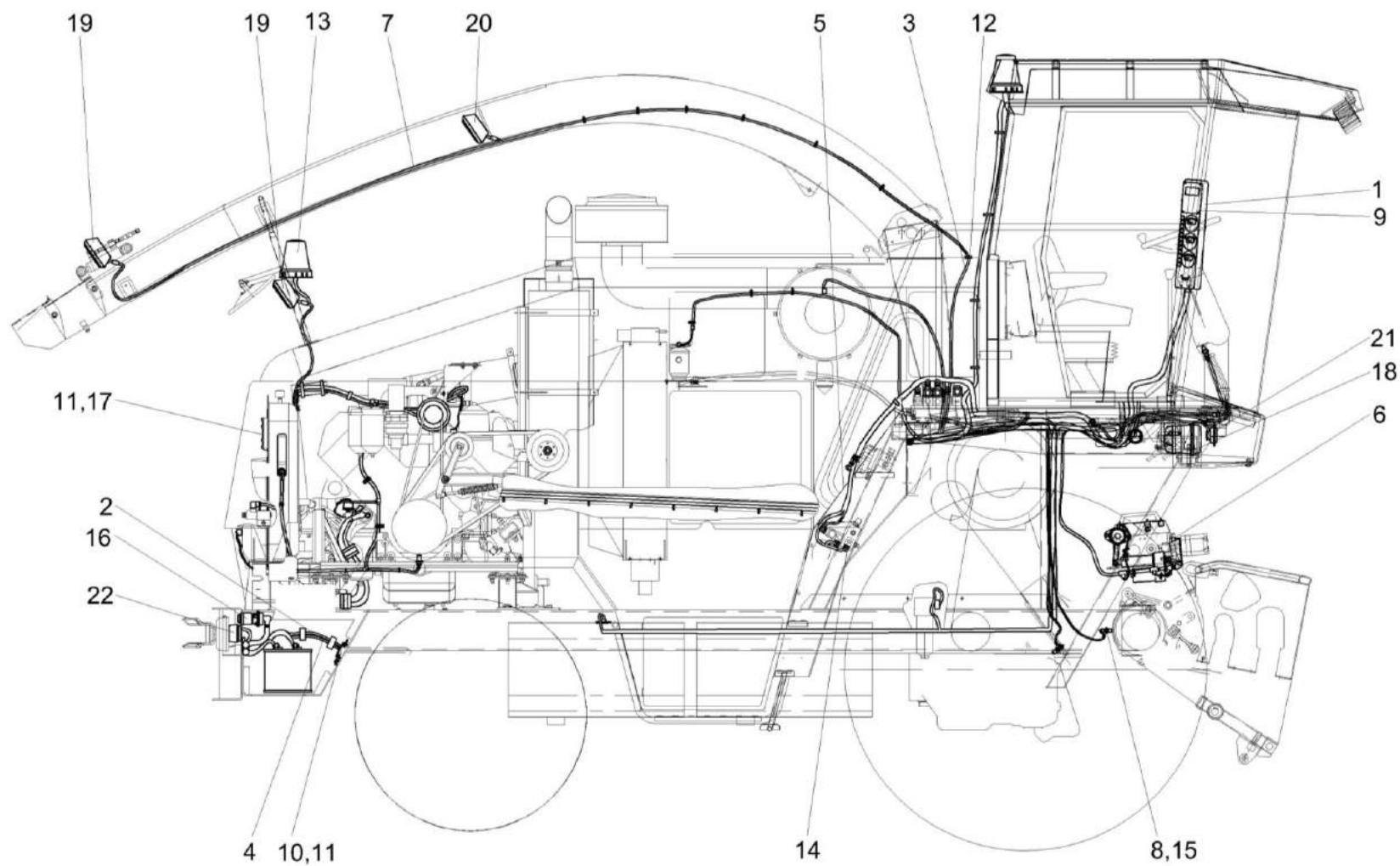
Рисунок 208 – Электрооборудование измельчителя самоходного КВС-5-0100000 (лист 2)
