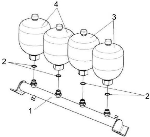
Рисунок 195 – Блок пневмогидроаккумуляторов КВС-1-0602540
