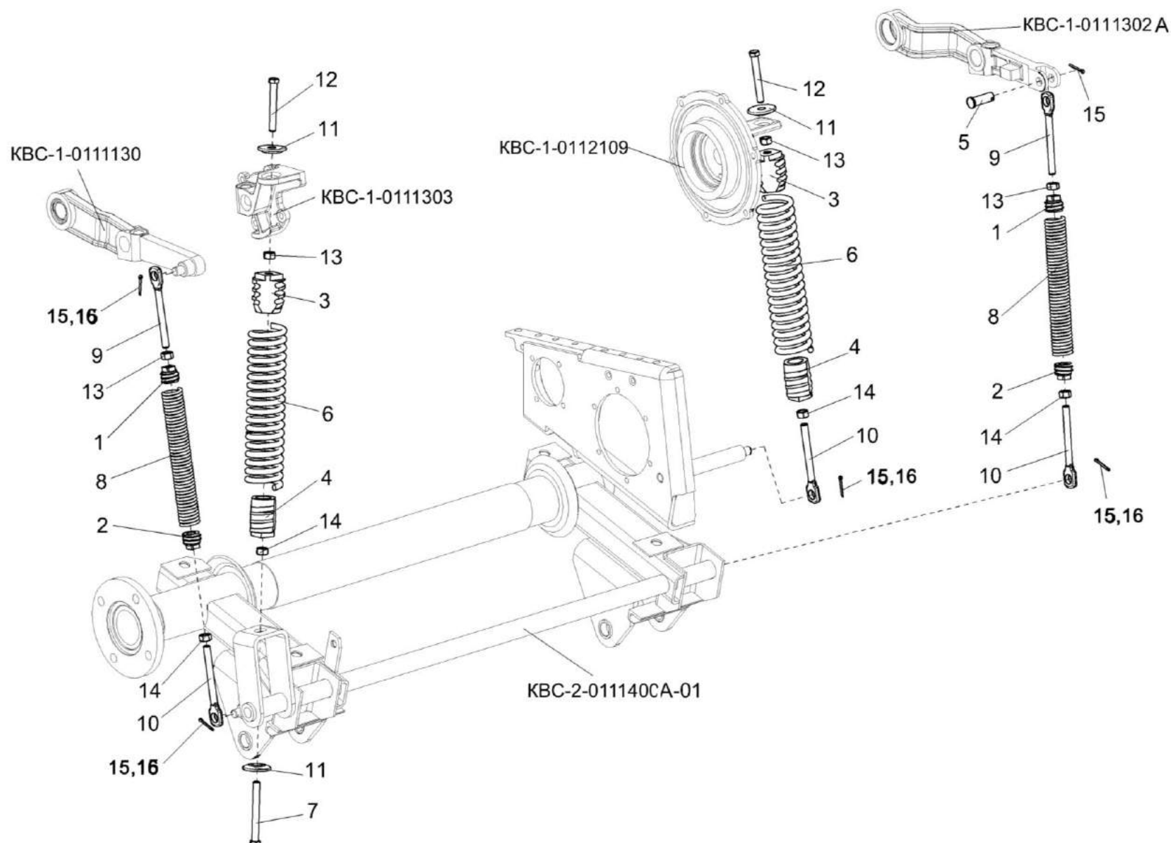
Рисунок 7 – Пружины аппарата питающего
