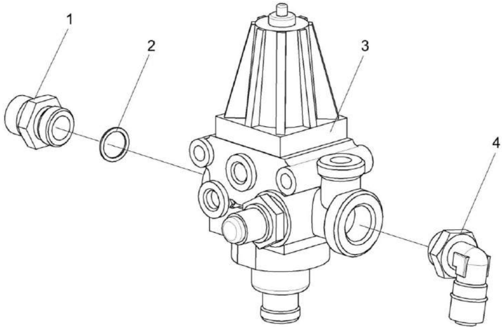
Рисунок 206 – Регулятор давления КВС-5-0800190
