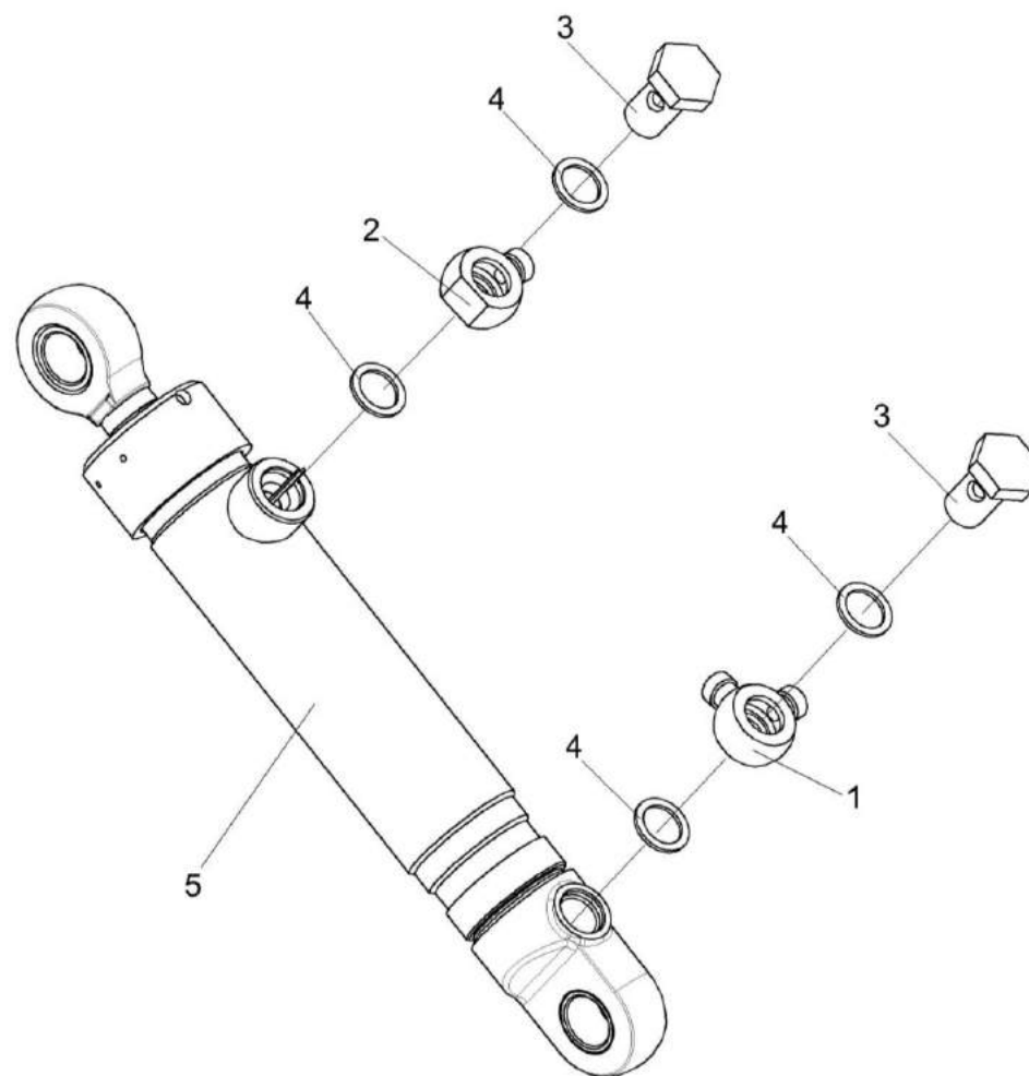
Рисунок 61 – Гидроцилиндр КВС-2-0602500
