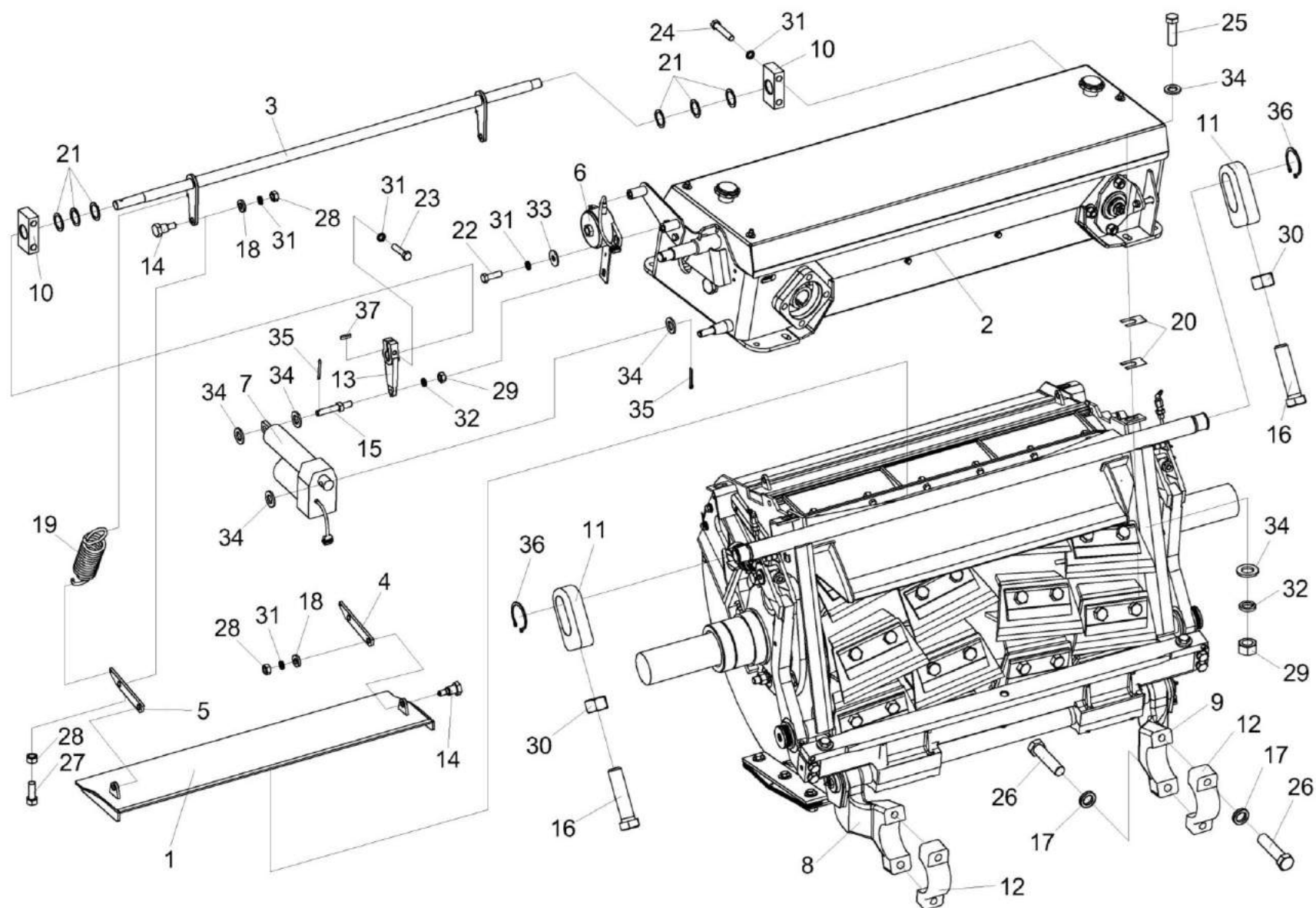
Рисунок 22 – Аппарат измельчающий КВС-2-0115000Б
