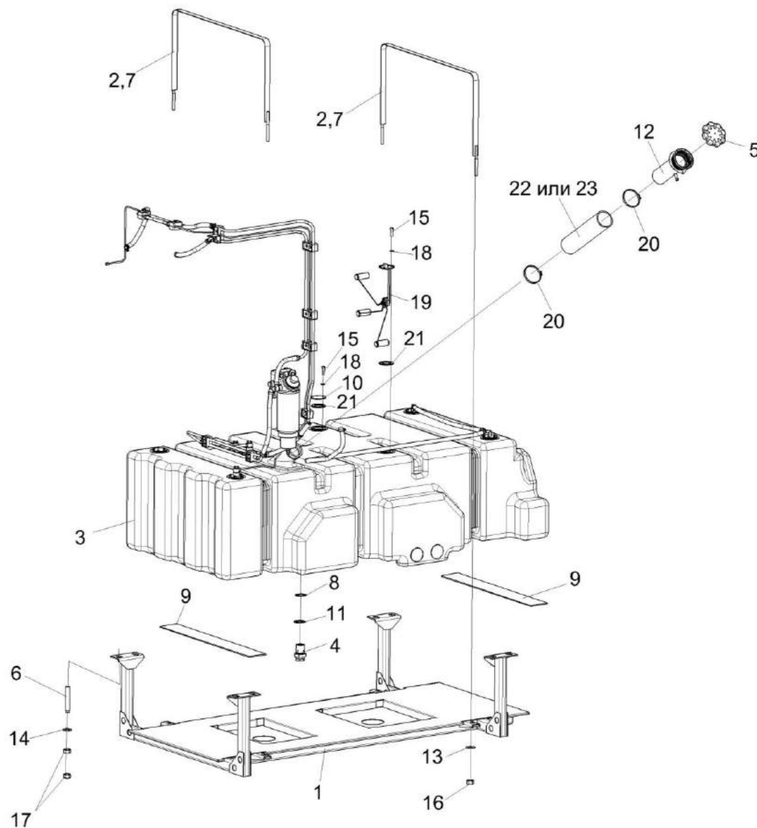
Рисунок 87 – Установка топливного оборудования КВС-5-0103700А (лист 1)
