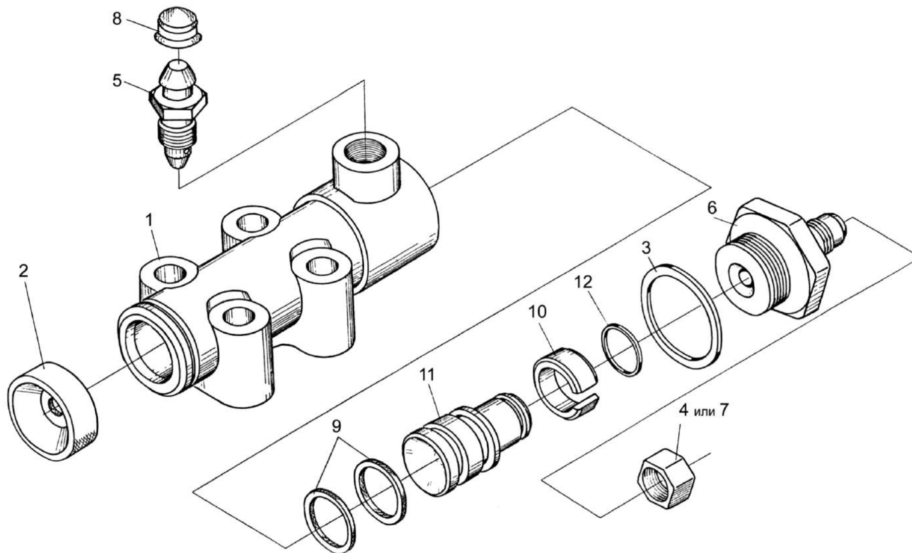
Рисунок 101 – Гидроцилиндр тормоза МК-23М.03.220А
