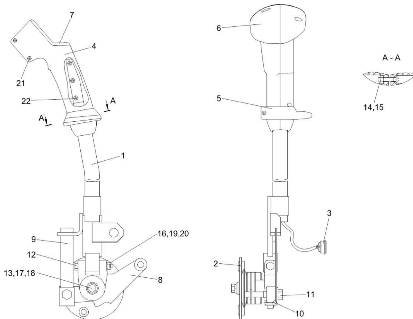
Рисунок 118 – Привод КВС-5-0129550
