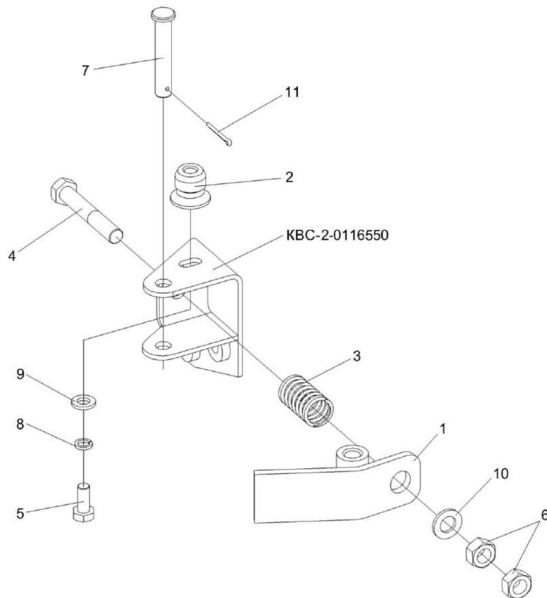
Рисунок 32 – Установка опоры KBC-2-0116550
