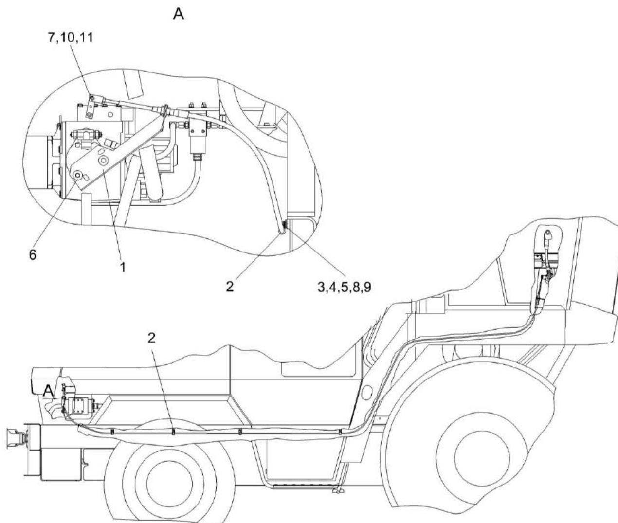
Рисунок 143 – Привод управления КВС-1-0129530А
