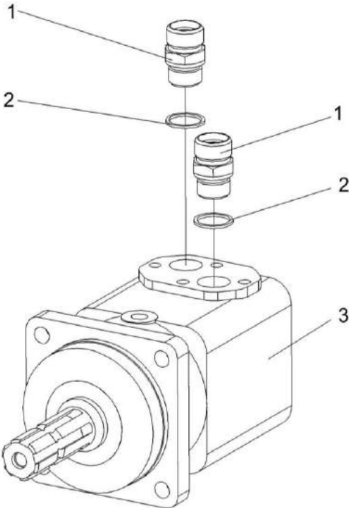
Рисунок 176 – Гидромотор привода адаптеров КГС 0115380
