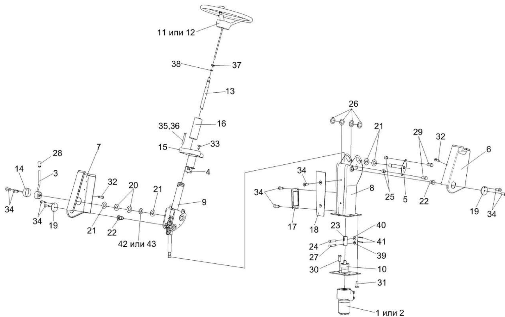
Рисунок 125 – Рулевая колонка КВС-1-0129230 и КВС-1-0129230-03
