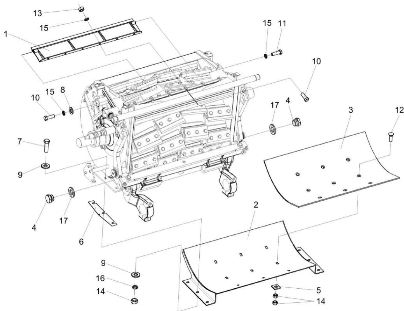
Рисунок 23 – Установка поддона КВС-2-0115050
