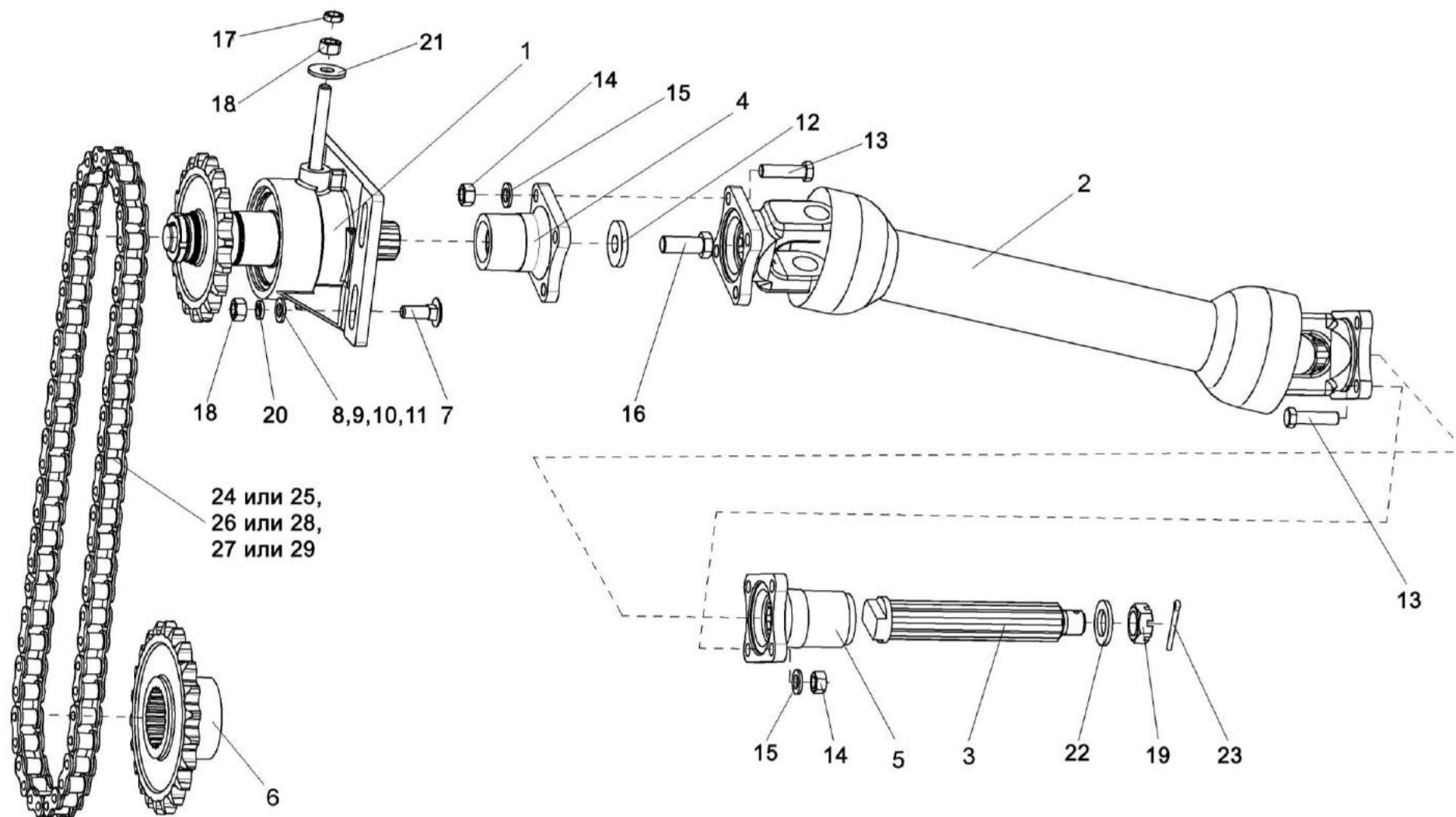
Рисунок 6 – Установка карданного вала KBC-1-0119000-01
