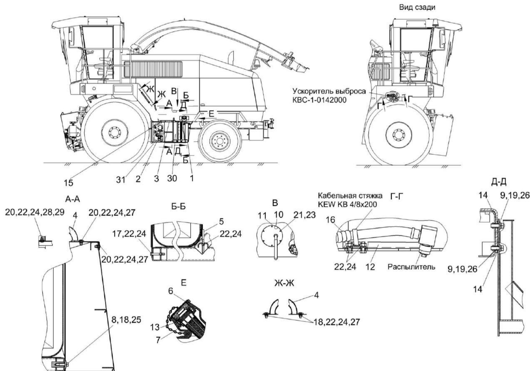
Рисунок 212 – Установка ОВК КВС-2-0900000А
