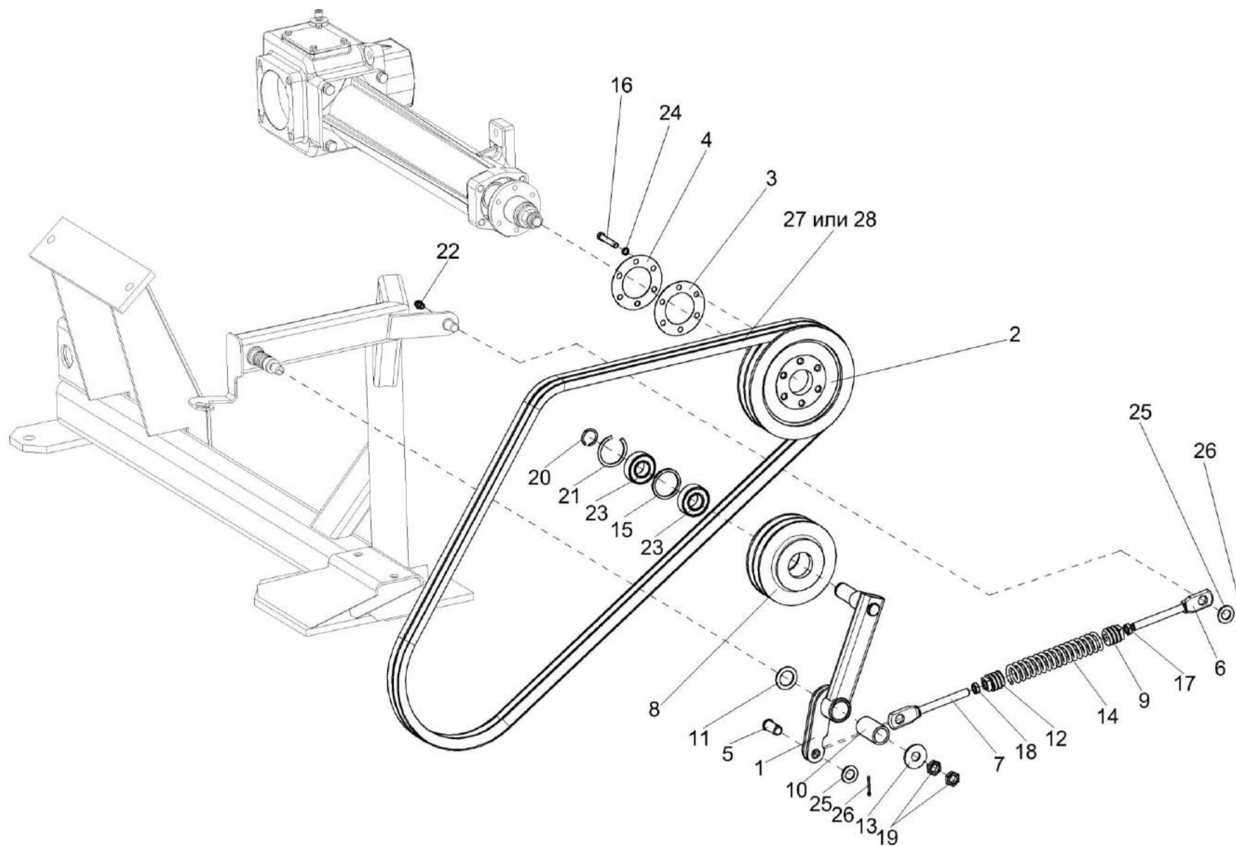
Рисунок 75 – Привод вентилятора КВС-5-0150260
