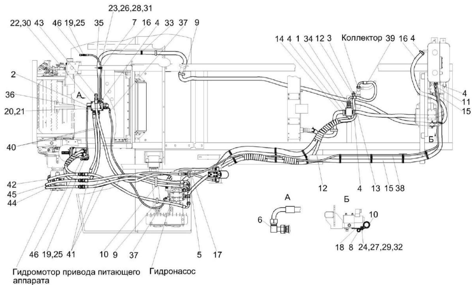
Рисунок 169 – Гидросистема привода питающего аппарата и адаптеров комбайна КВК-800-36 КВС-5-0604000 (лист 2)
