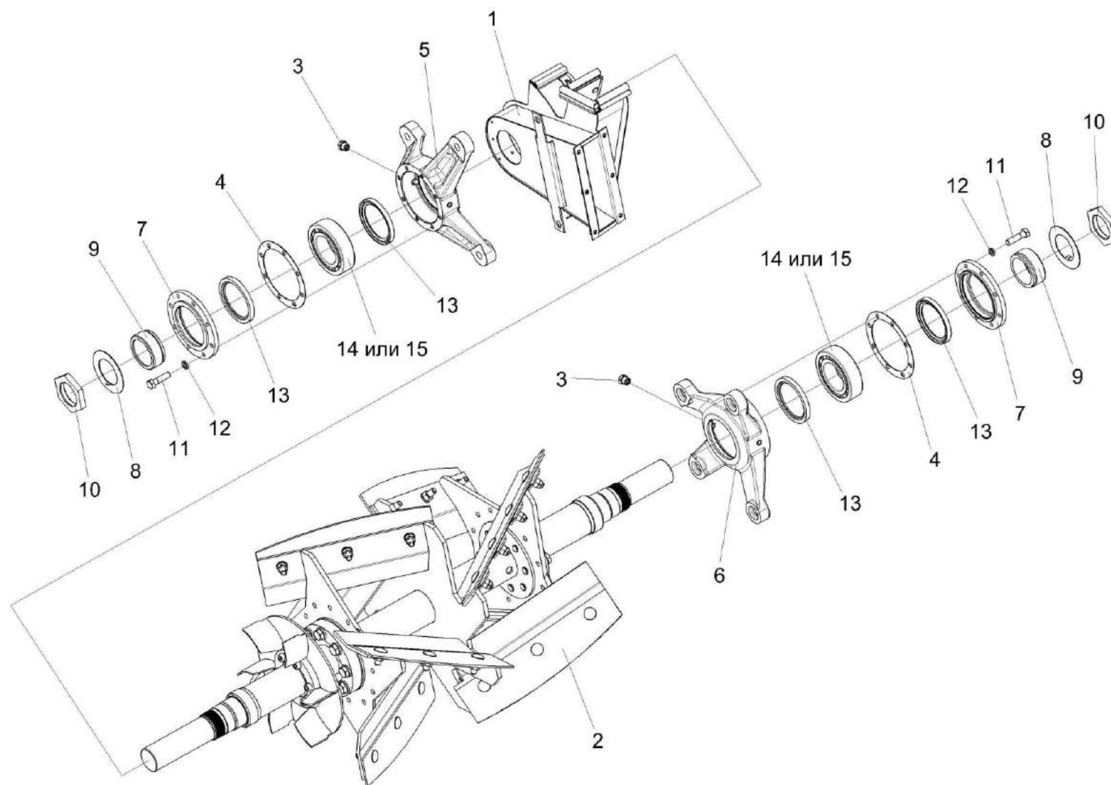
Рисунок 55 – Вал ускорителя выброса КВС-1-0142900
