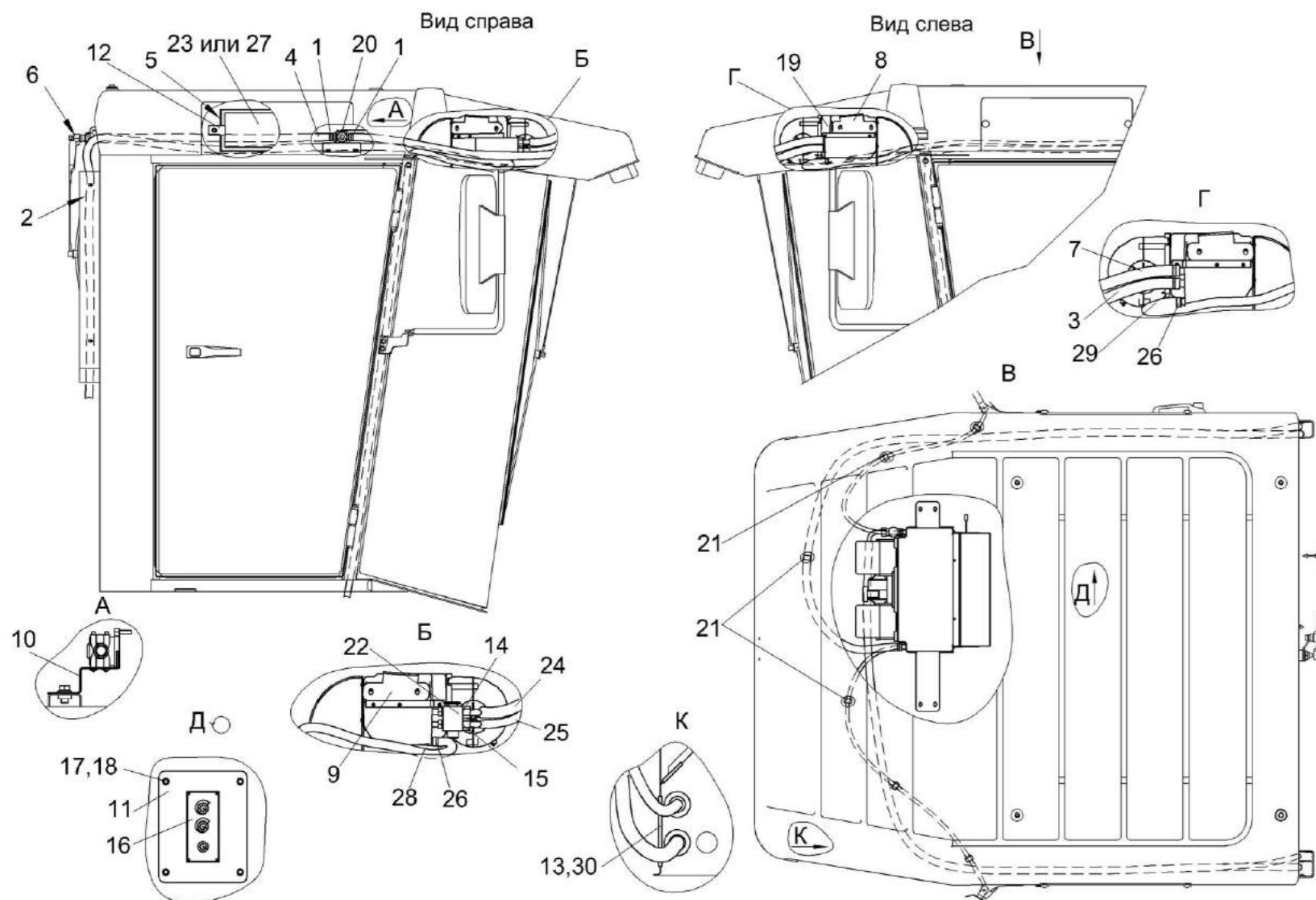
Рисунок 155 – Установка испарителя КВС-2-0121050
