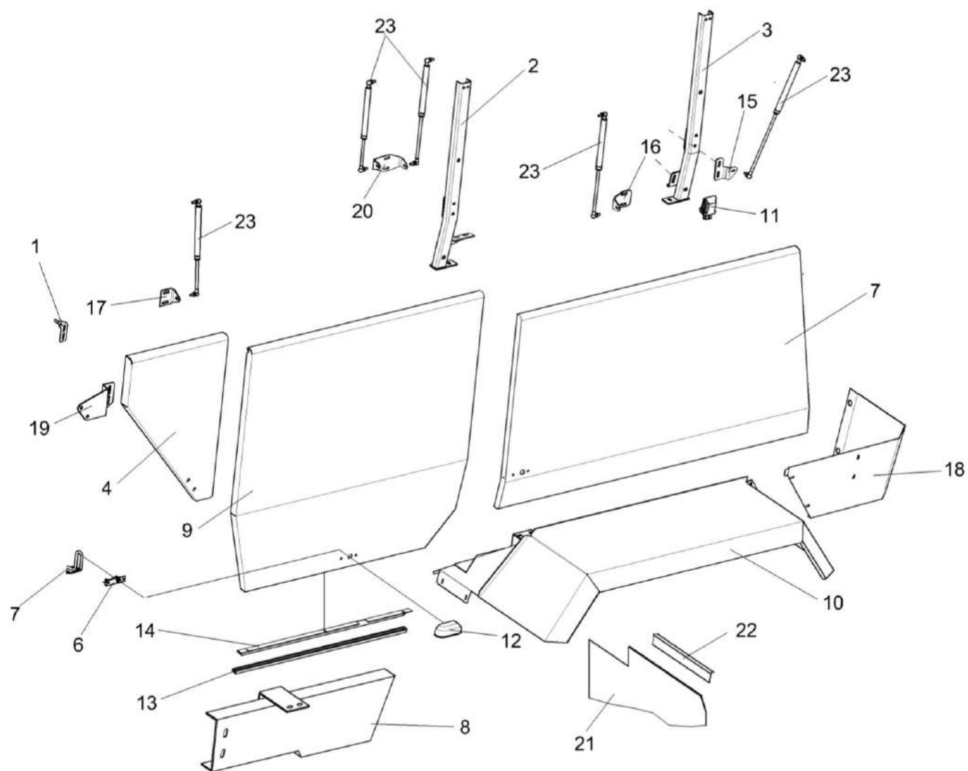
Рисунок 156 – Установка капотов КВС-2-0160000-03 (лист 1)
