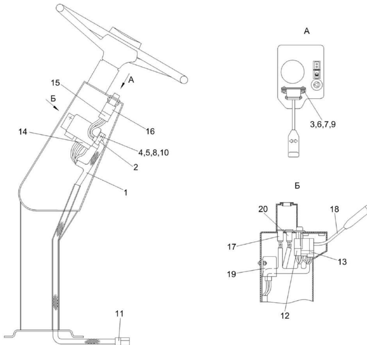
Рисунок 133 – Электрооборудование рулевой колонки КВС-1-0129230 и КВС-1-0129230-03
