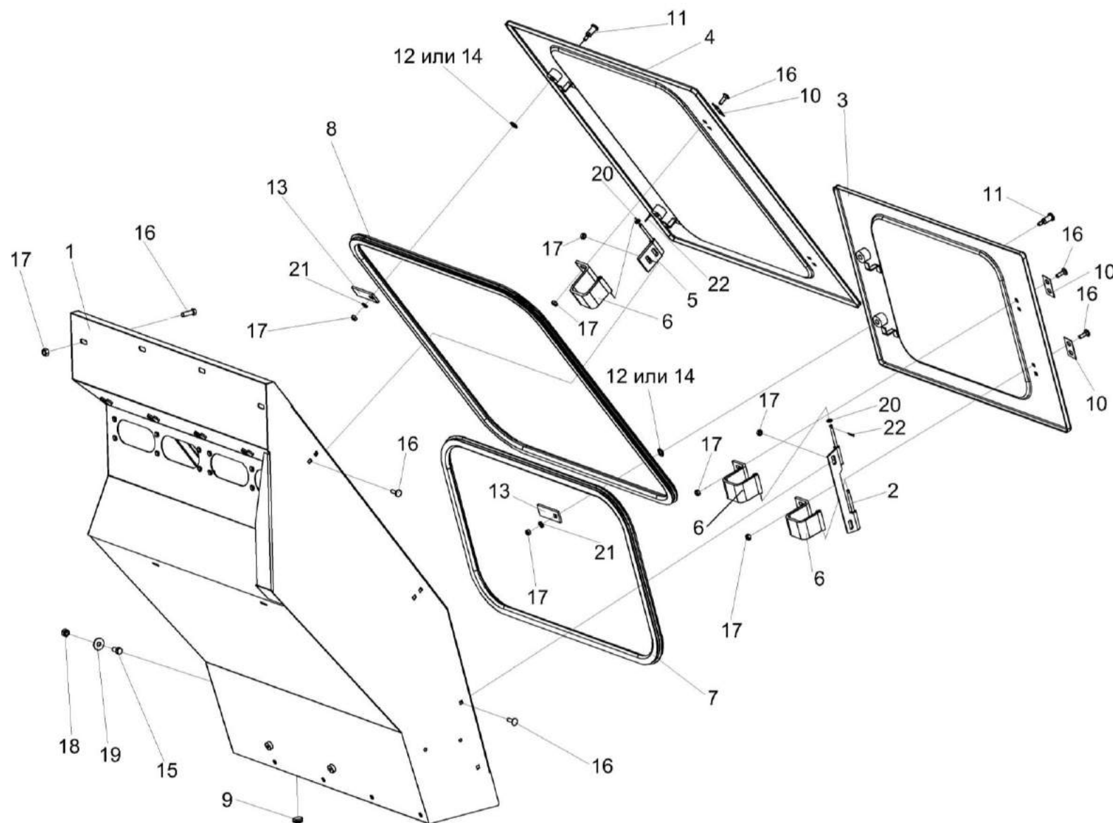
Рисунок 211 – Электрощкаф КВС-2-0702010А-01
