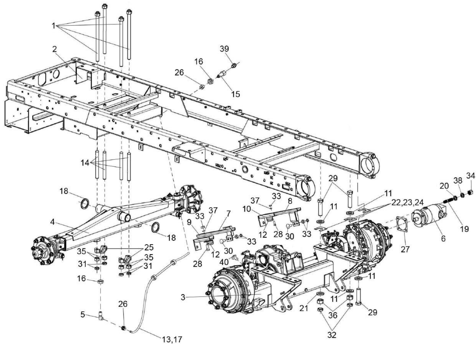
Рисунок 90 – Шасси КВС-2-0101500 (лист 2)
