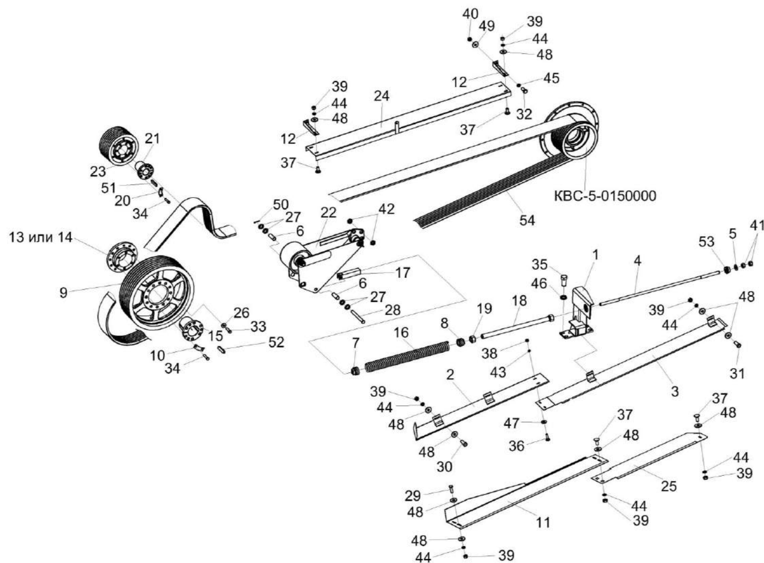
Рисунок 34 – Привод измельчающего барабана КВС-5-0130000-01
