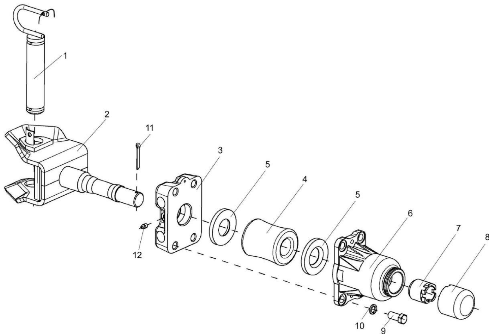
Рисунок 110 – Устройство тягово-сцепное УЭС 0003150
