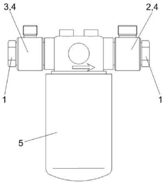
Рисунок 174 – Фильтр напорный КВС-5-0604300
