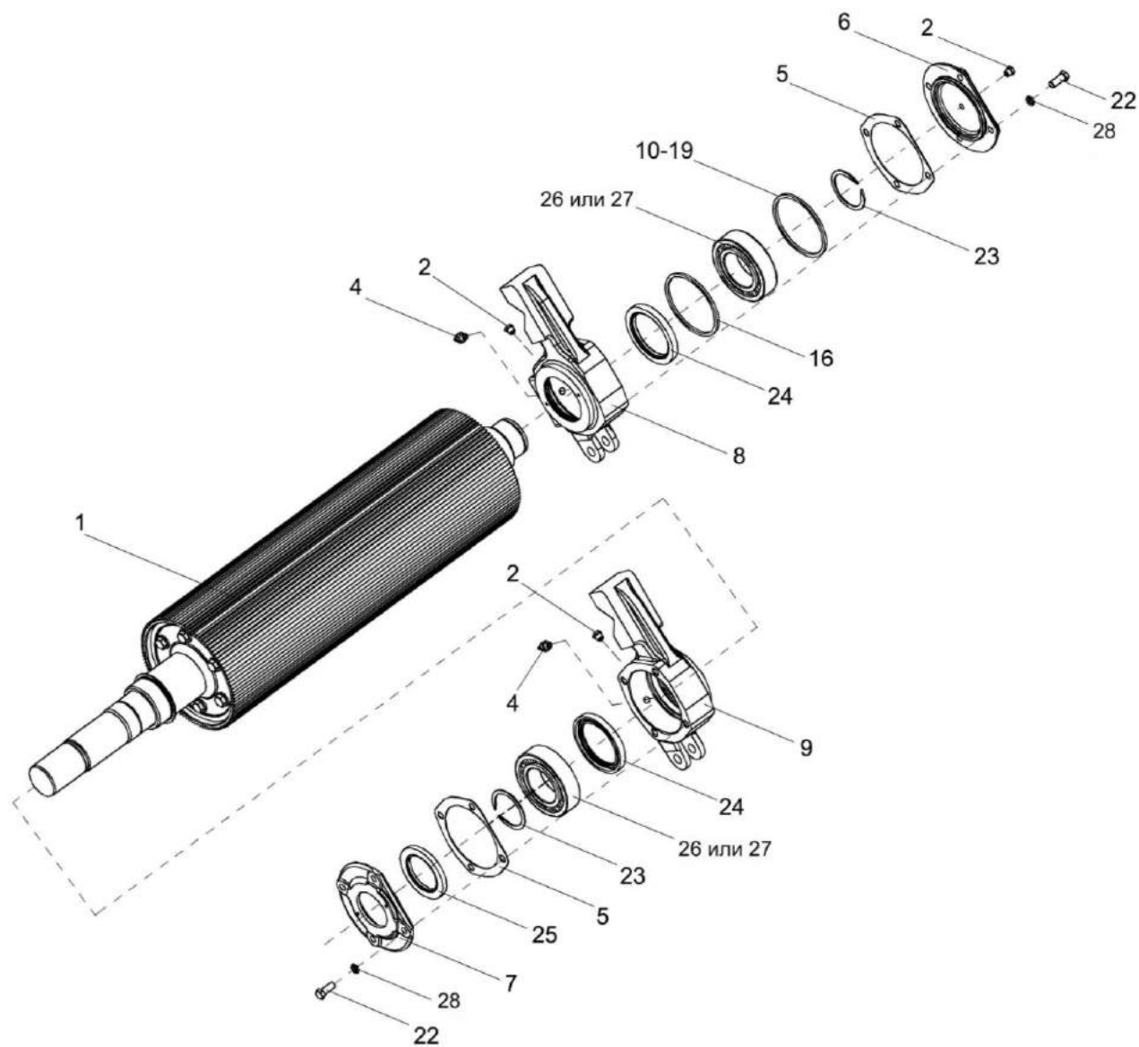
Рисунок 45 – Валец нижний КВС-1-0148610
