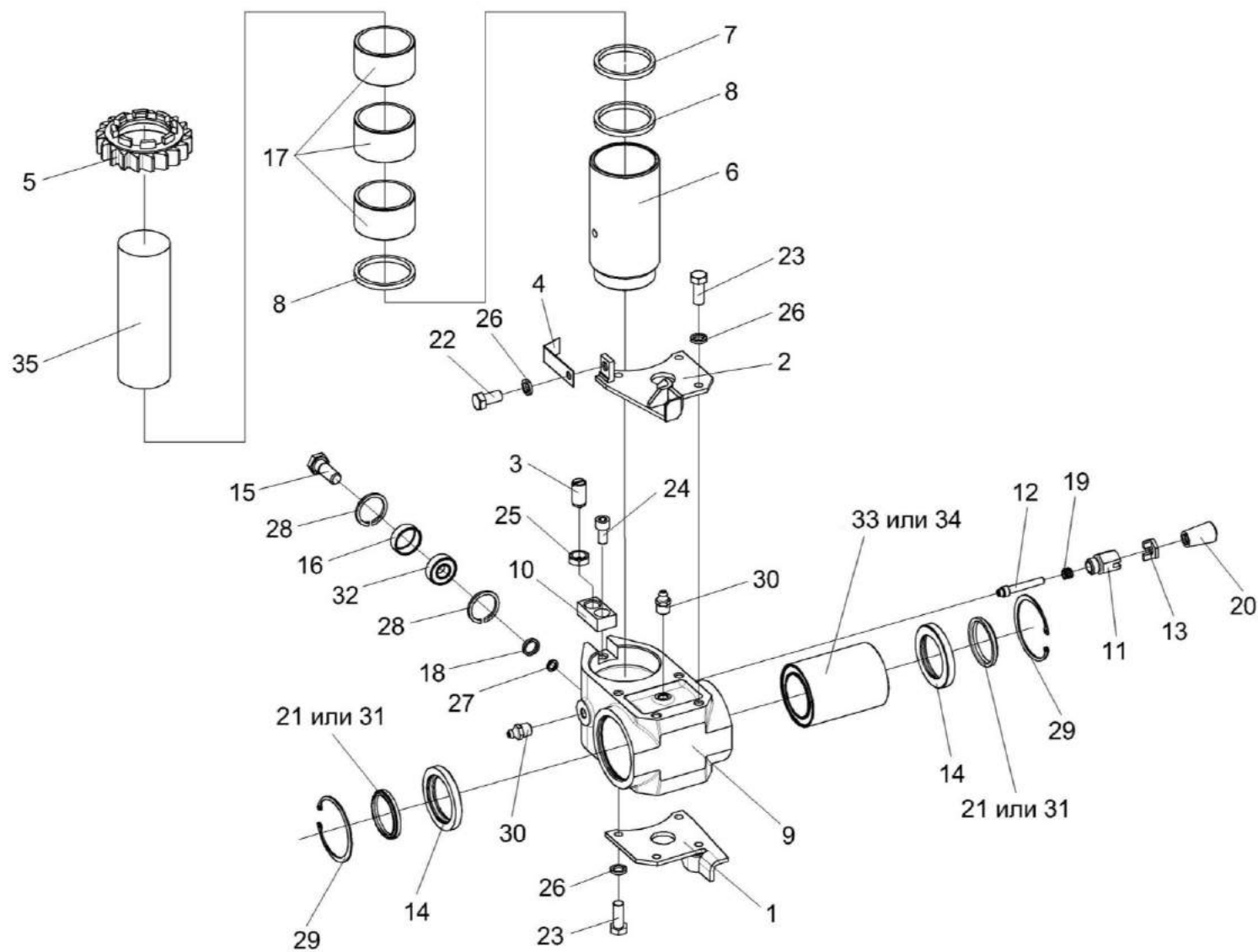
Рисунок 30 – Установка каретки КВС-2-0116510
