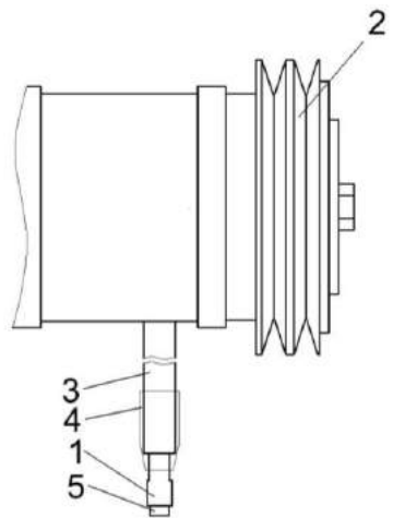
Рисунок 81 – Компрессор КВС-1-0150630-01
