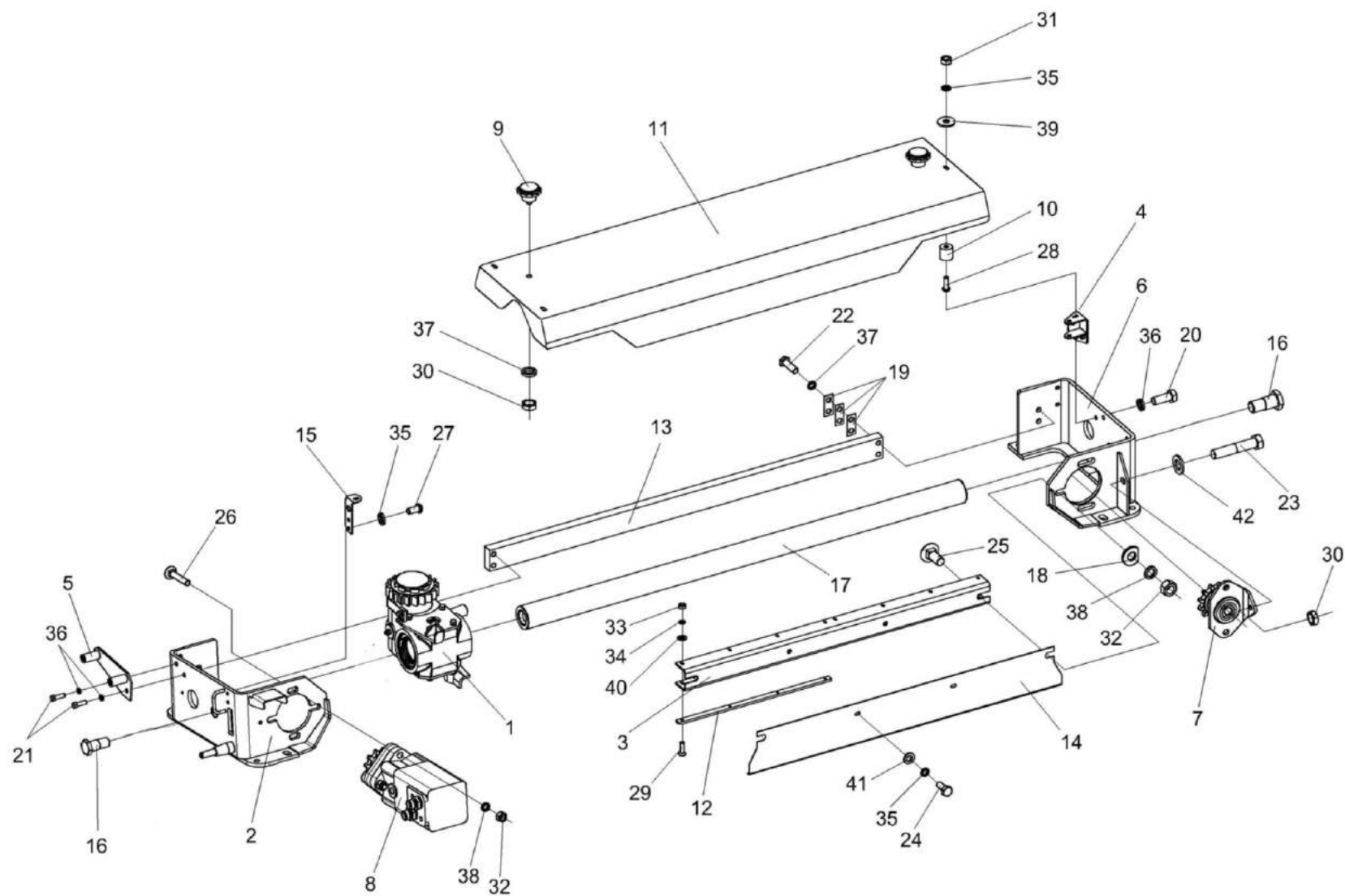
Рисунок 29 – Устройство заточное КВС-2-0116500
