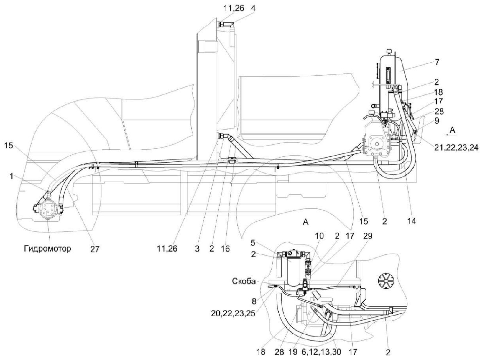
Рисунок 184 – Гидросистема привода ходовой части KBC-5-0601000 (лист 2)
