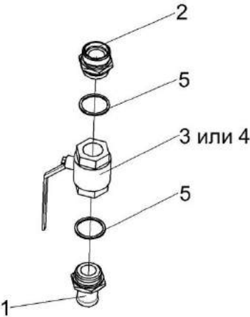
Рисунок 203 – Кран КЗК-10-0602380
