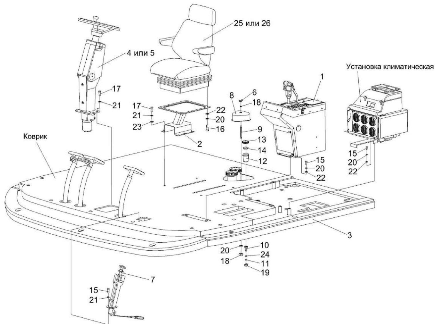
Рисунок 114 – Площадка управления КВС-5-0129000-04 (лист 1)
