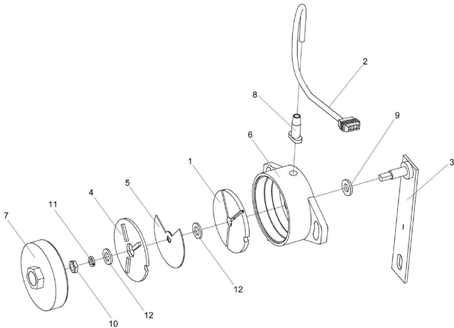
Рисунок 28 – Датчик положения КВС-1-0701500-01
