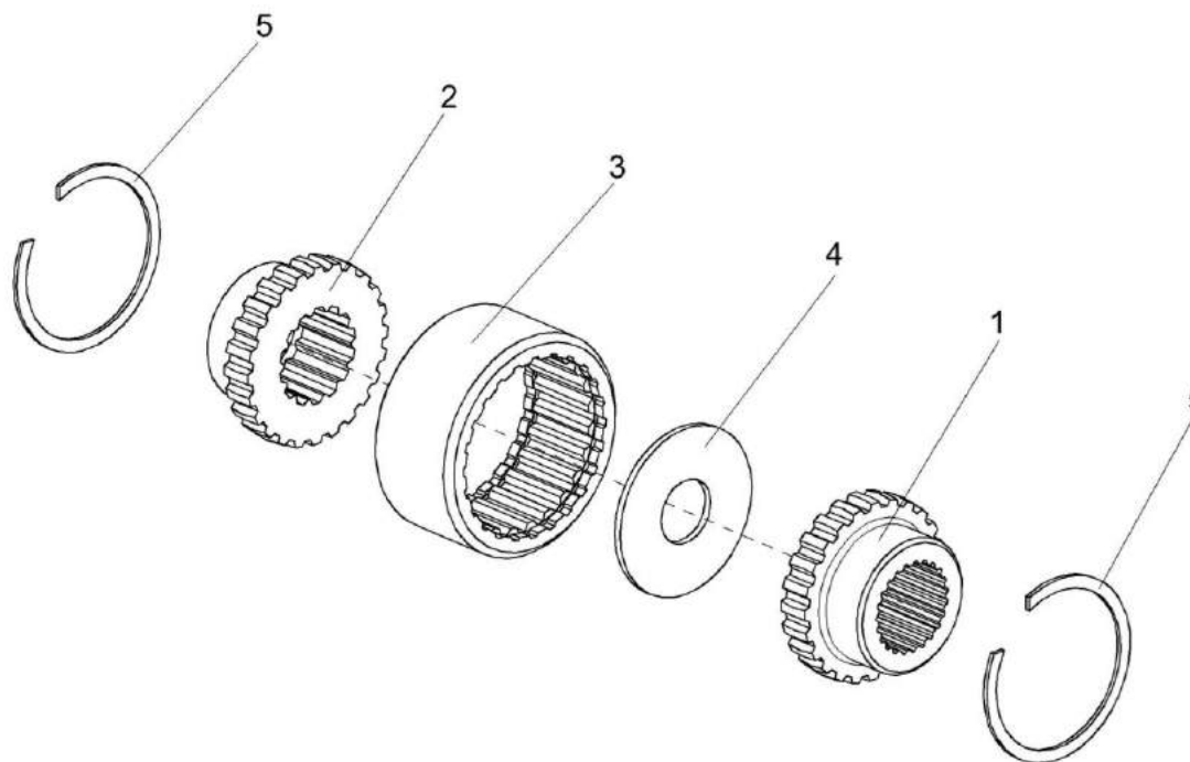
Рисунок 21 – Муфта КГС 0100120
