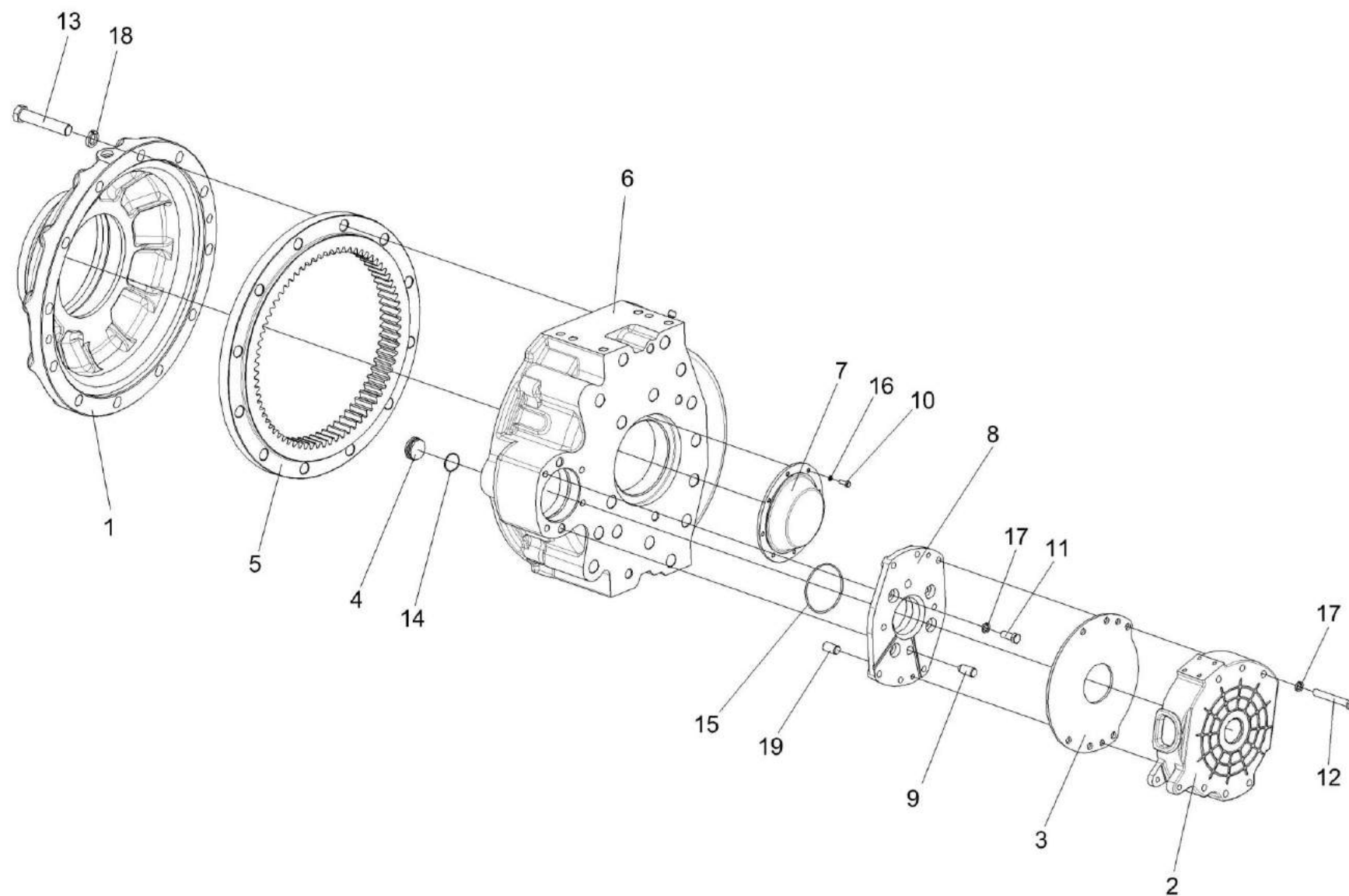
Рисунок 95 – Редуктор бортовой КЗК-10-0107200-02 (Корпуса и крышки)
