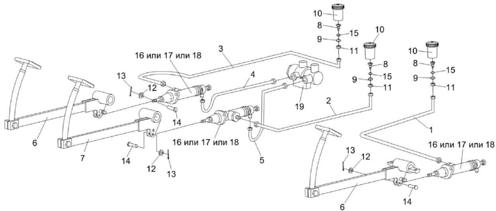
Рисунок 116 – Рычаги и трубопроводы площадки управления
