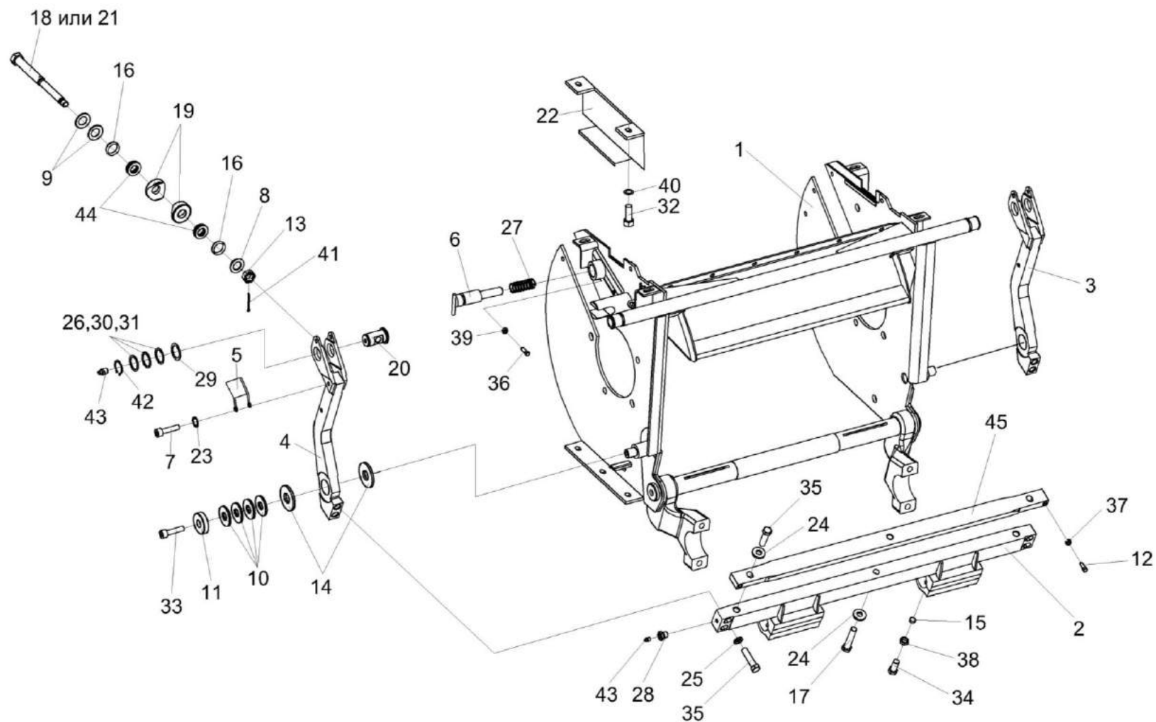
Рисунок 25 – Установка рычагов КВС-2-0117020 и КВС-2-0117020-01
