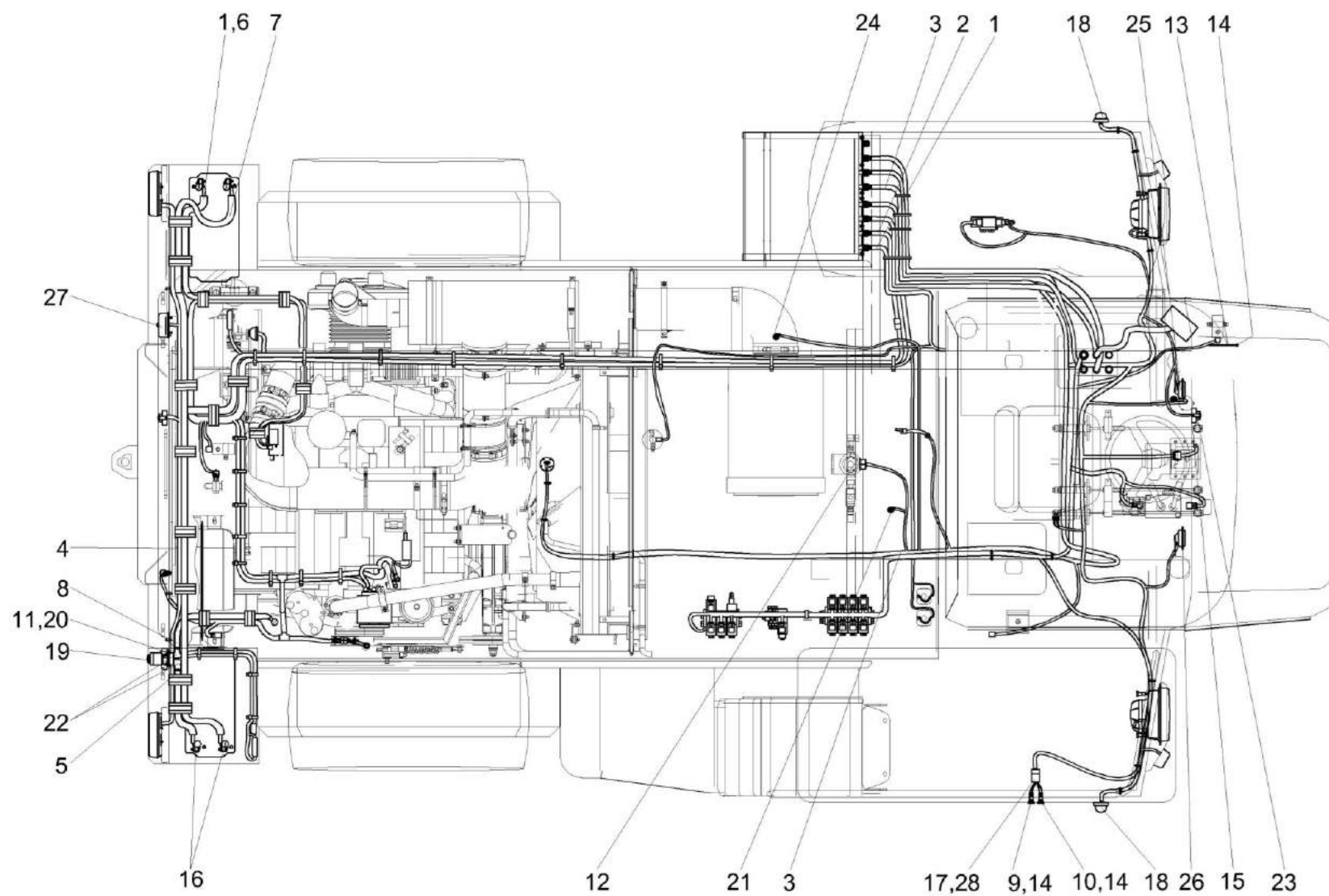
Рисунок 207 – Электрооборудование измельчителя самоходного КВС-5-0100000 (лист 1)
