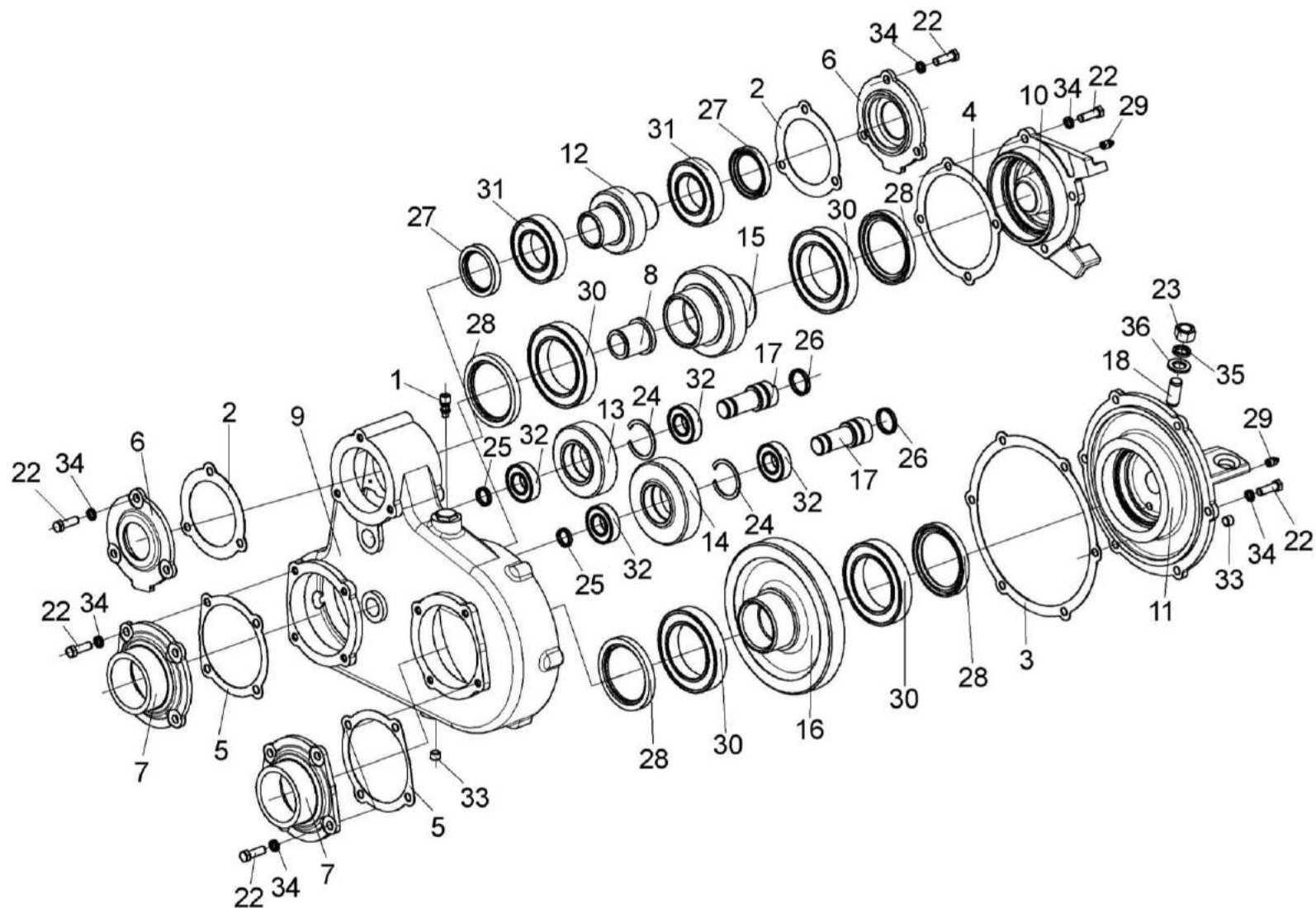
Рисунок 12 – Редуктор верхних вальцев КВС-2-0112000
