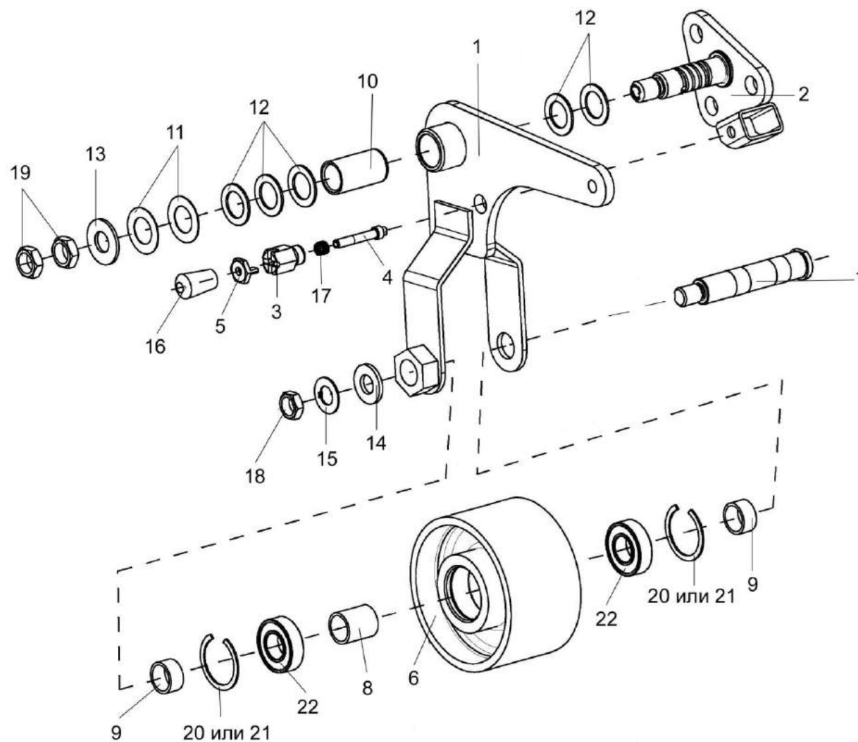
Рисунок 38 – Рычаг КВС-1-0132010
