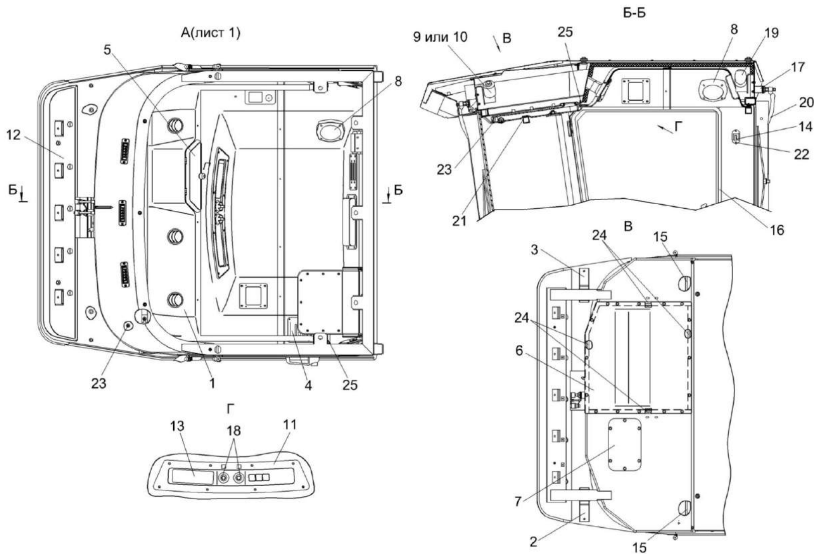
Рисунок 147 – Кабина КВС-2-0122000 (лист 2)
