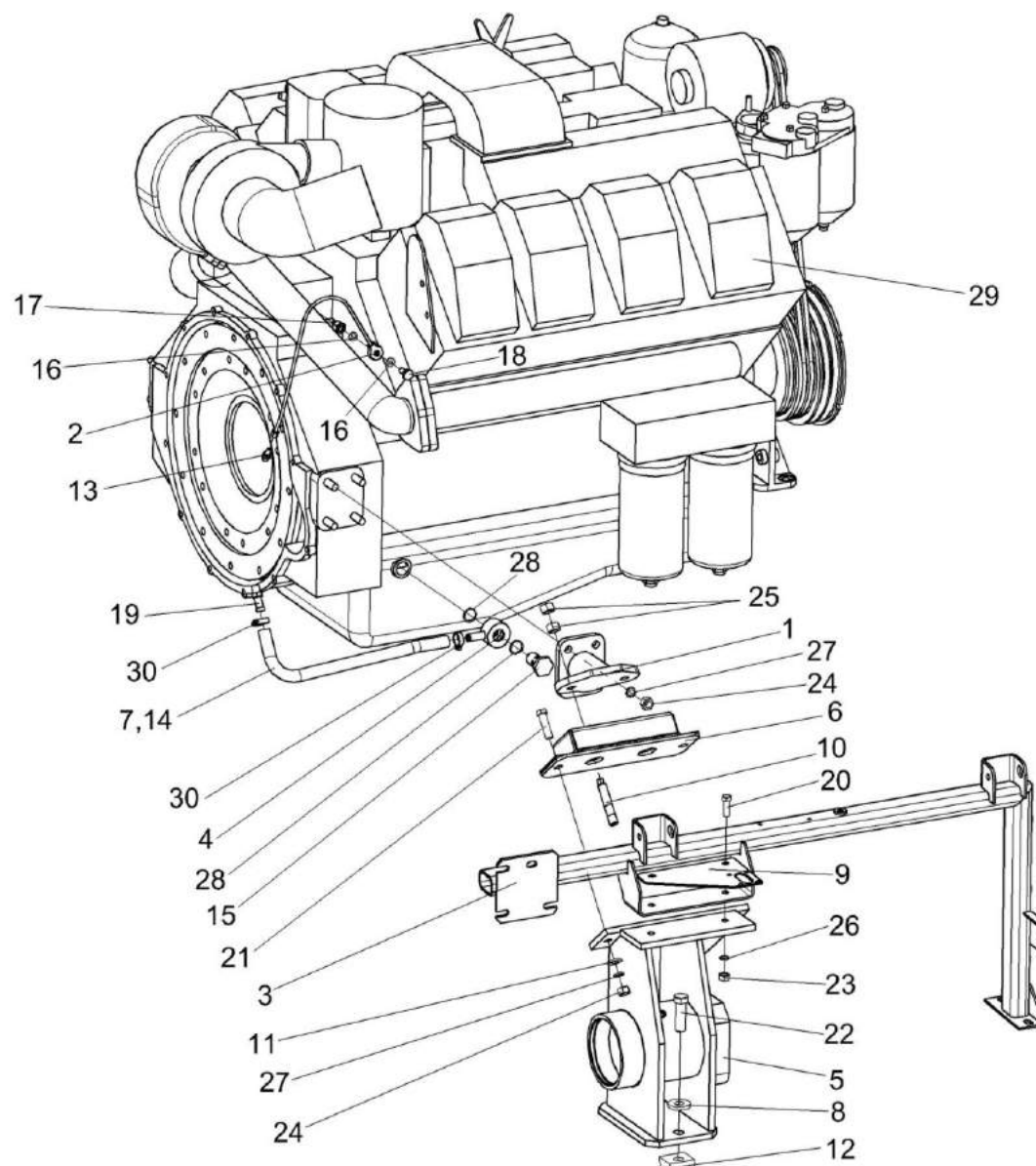
Рисунок 66 – Установка дизеля Д-280.1S2 КВС-5-0150000А (установка дизеля) (лист 2)
