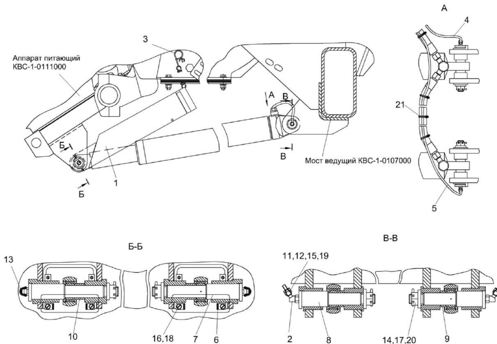
Рисунок 111 – Механизм вывешивания KBC-1-0105000A-01
