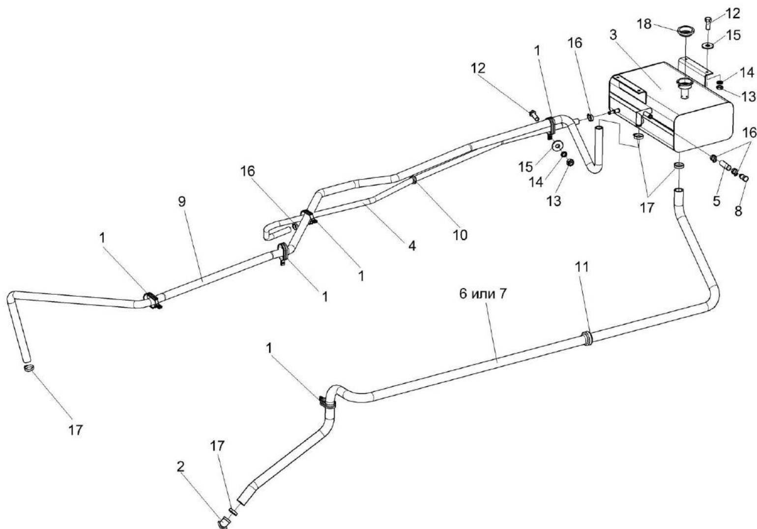
Рисунок 76 – Установка бачка расширительного КВС-5-0154000Б
