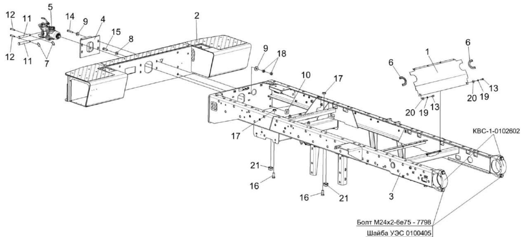
Рисунок 89 – Шасси КВС-2-0101500 (лист 1)
