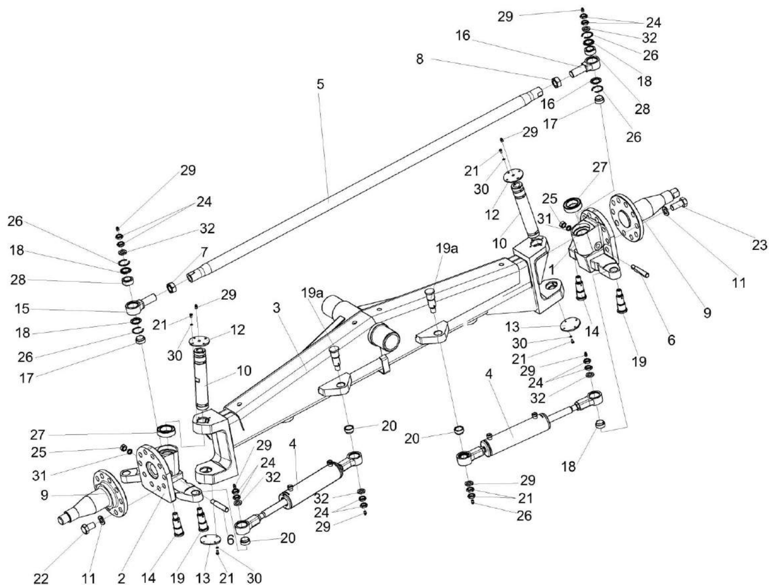
Рисунок 107 – Мост управляемых колес КВС-2-0109000
