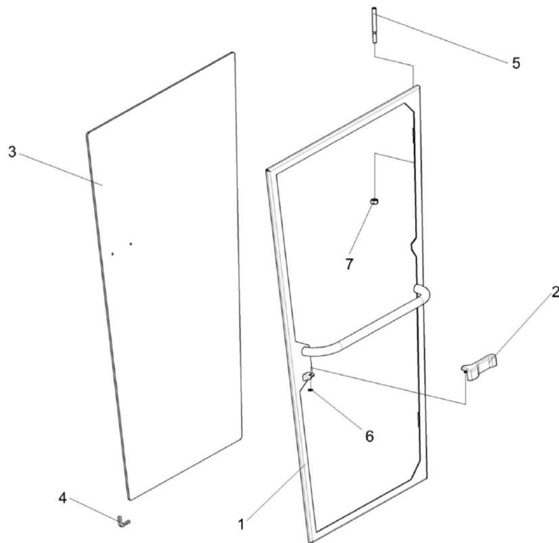
Рисунок 149 – Дверь КЗК-10-0200120
