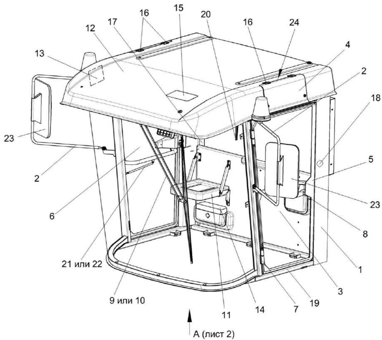
Рисунок 146 – Кабина КВС-2-0122000 (лист 1)
