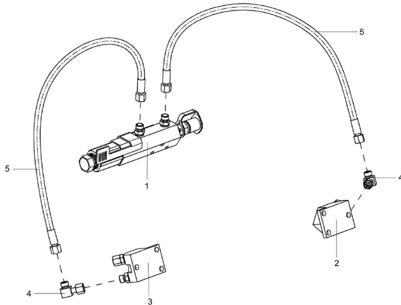
Рисунок 47 – Гидросистема регулировки зазора КВС-1-0603000
