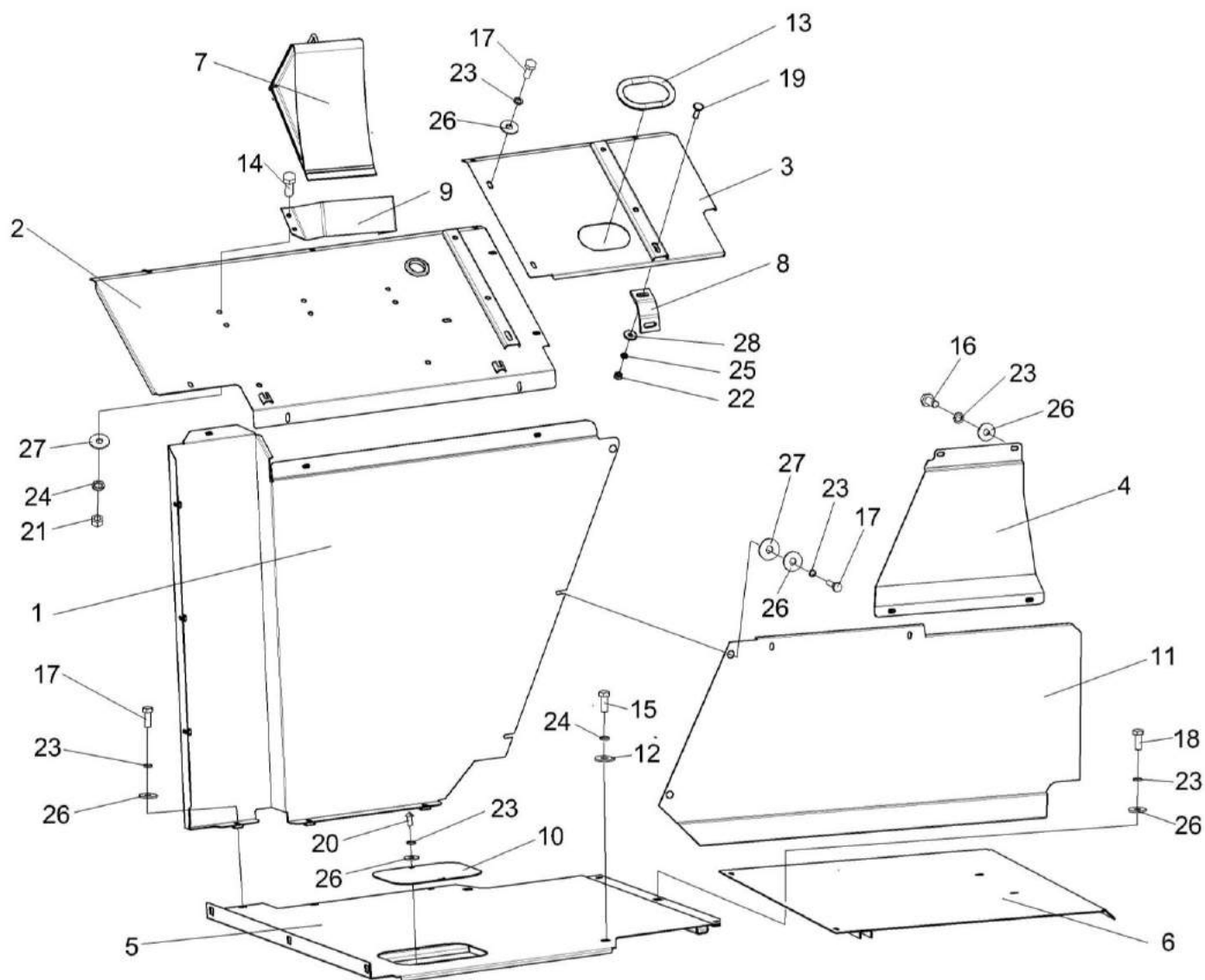
Рисунок 163 – Установка настилов и ограждений КВС-2-0169000-02
