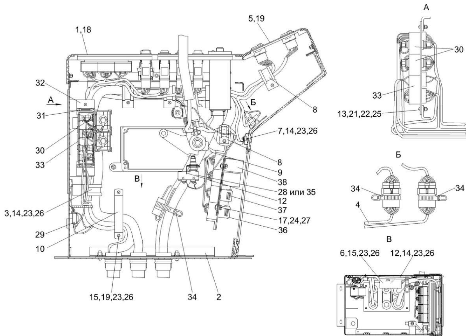
Рисунок 121 – Электрооборудование пульта управления КВС-5-0129050А-02
