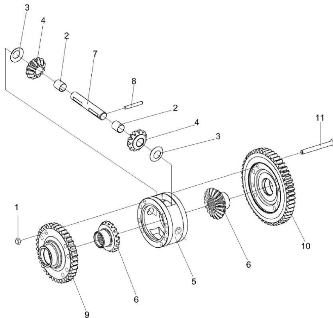
Рисунок 104 – Дифференциал 3518020-43190
