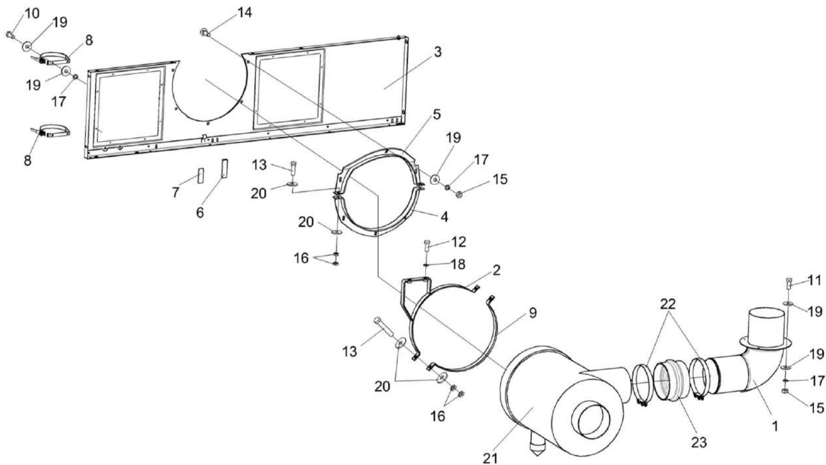
Рисунок 161 – Капот верхний КВС-2-0162000-02 (лист 3)
