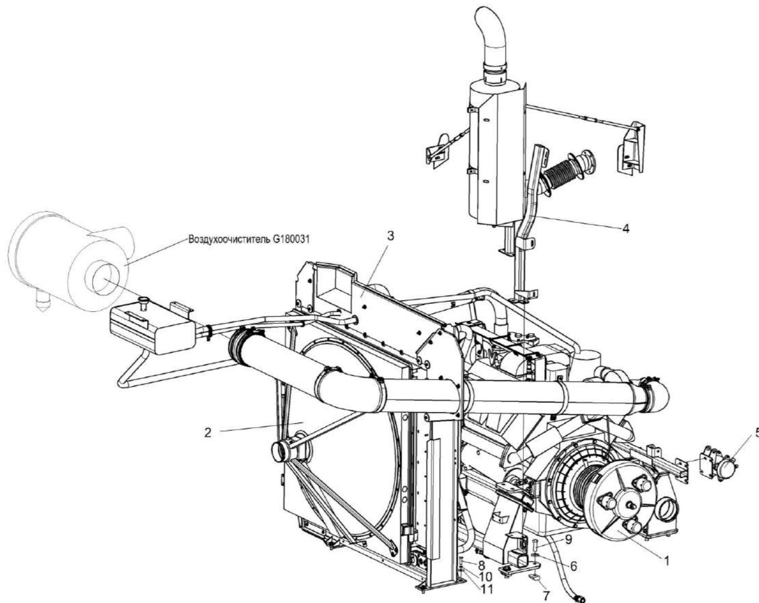
Рисунок 62 – Установка дизеля Д-280.1S2 KBC-5-0150000A (вид справа)
