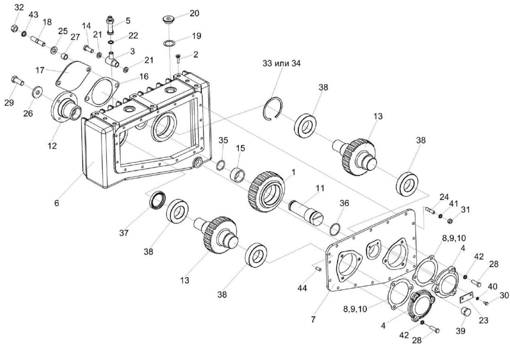
Рисунок 166 – Редуктор КВС-2-0104100
