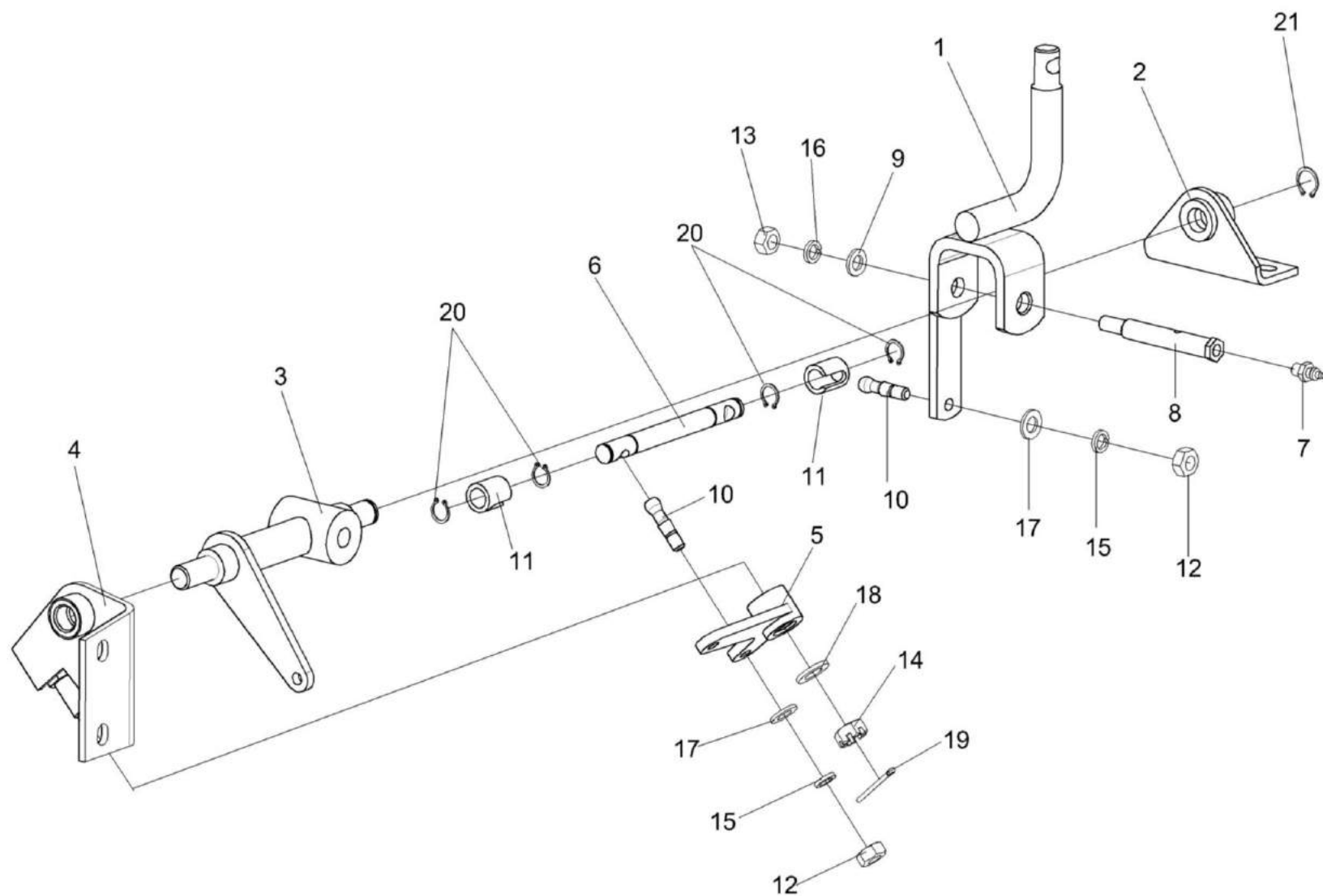
Рисунок 139 – Блок переключения КВС-2-0129070
