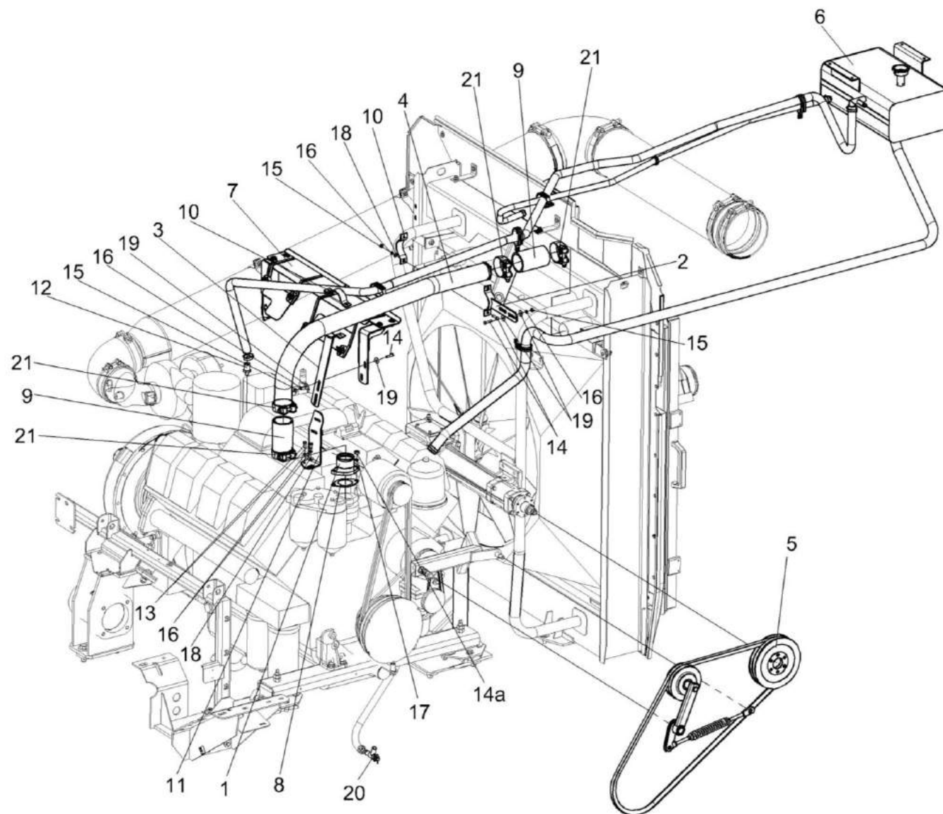
Рисунок 63 – Установка дизеля Д-280.1S2 КВС-5-0150000А (вид слева)
