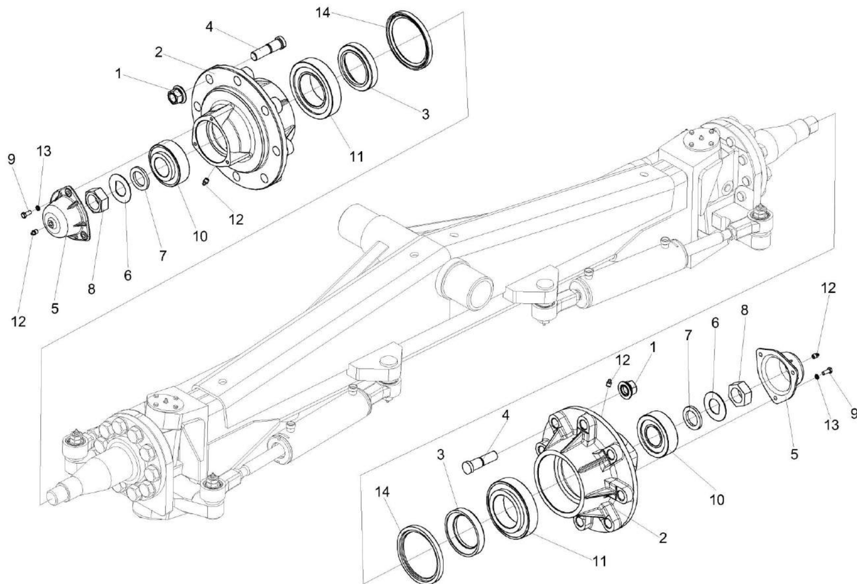
Рисунок 108 – Мост управляемых колес КВС-2-0109000 (установка ступиц)
