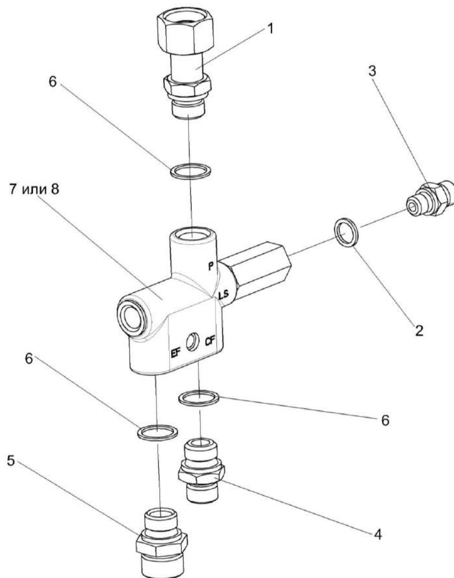
Рисунок 201 – Клапан приоритетный KBC-5-602340
