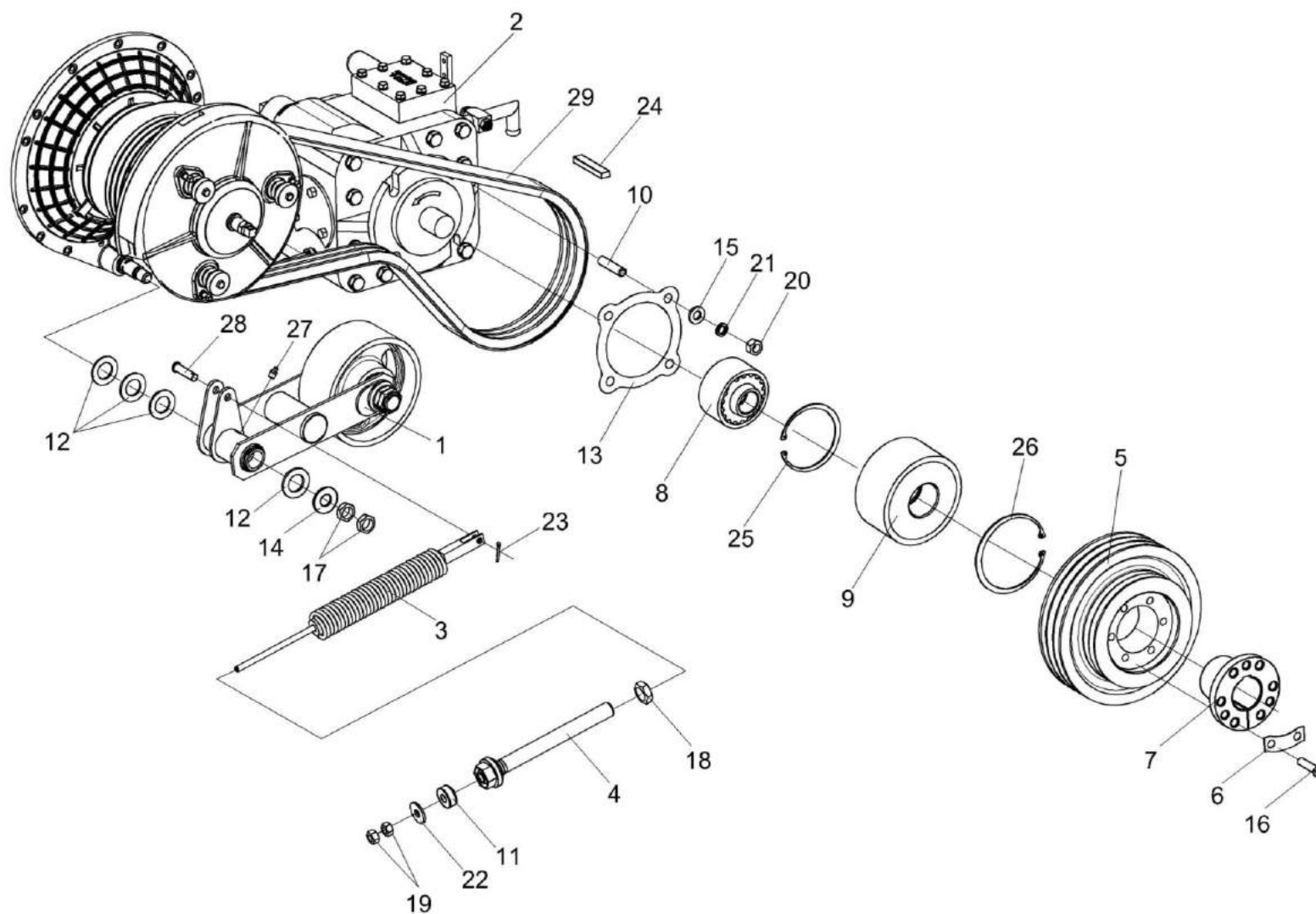
Рисунок 82 – Привод гидростата КВС-5-0133000А
