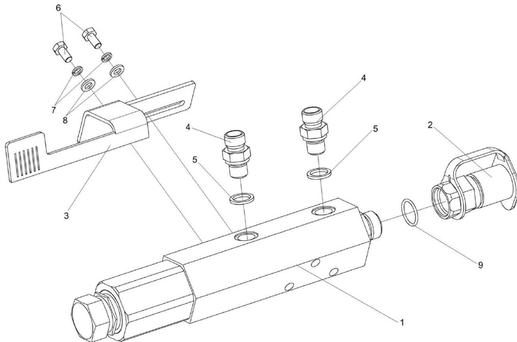
Рисунок 48 – Цилиндр КВС-1-0603110
