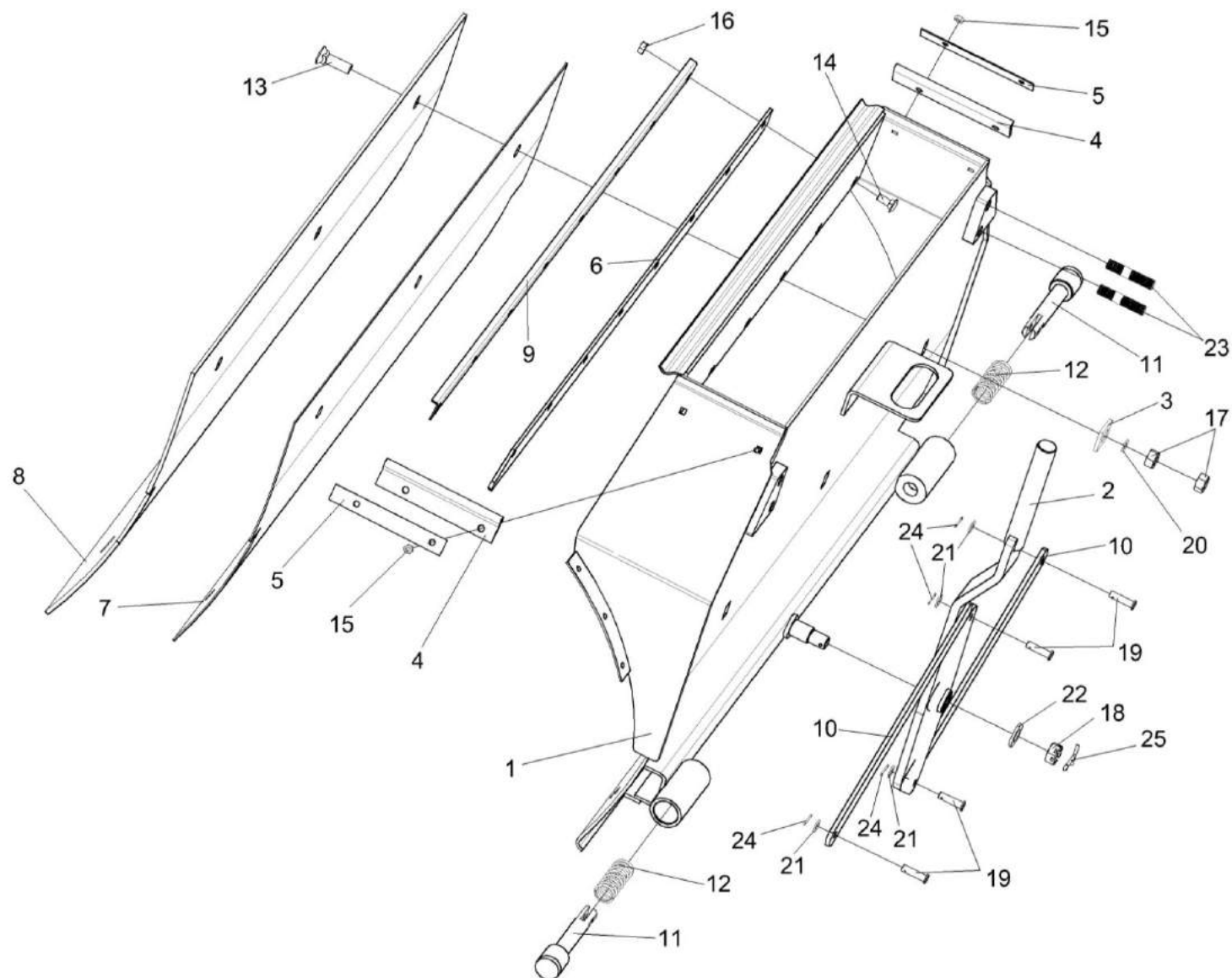
Рисунок 52 – Камера приемная КВС-1-0147000
