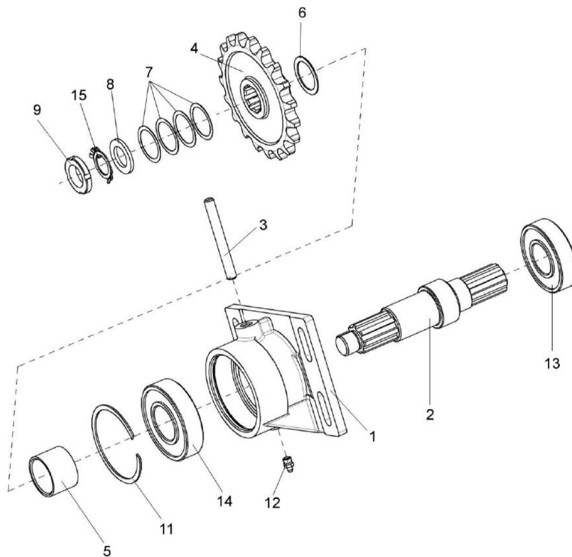
Рисунок 9 – Контрпривод КВС-1-0111170
