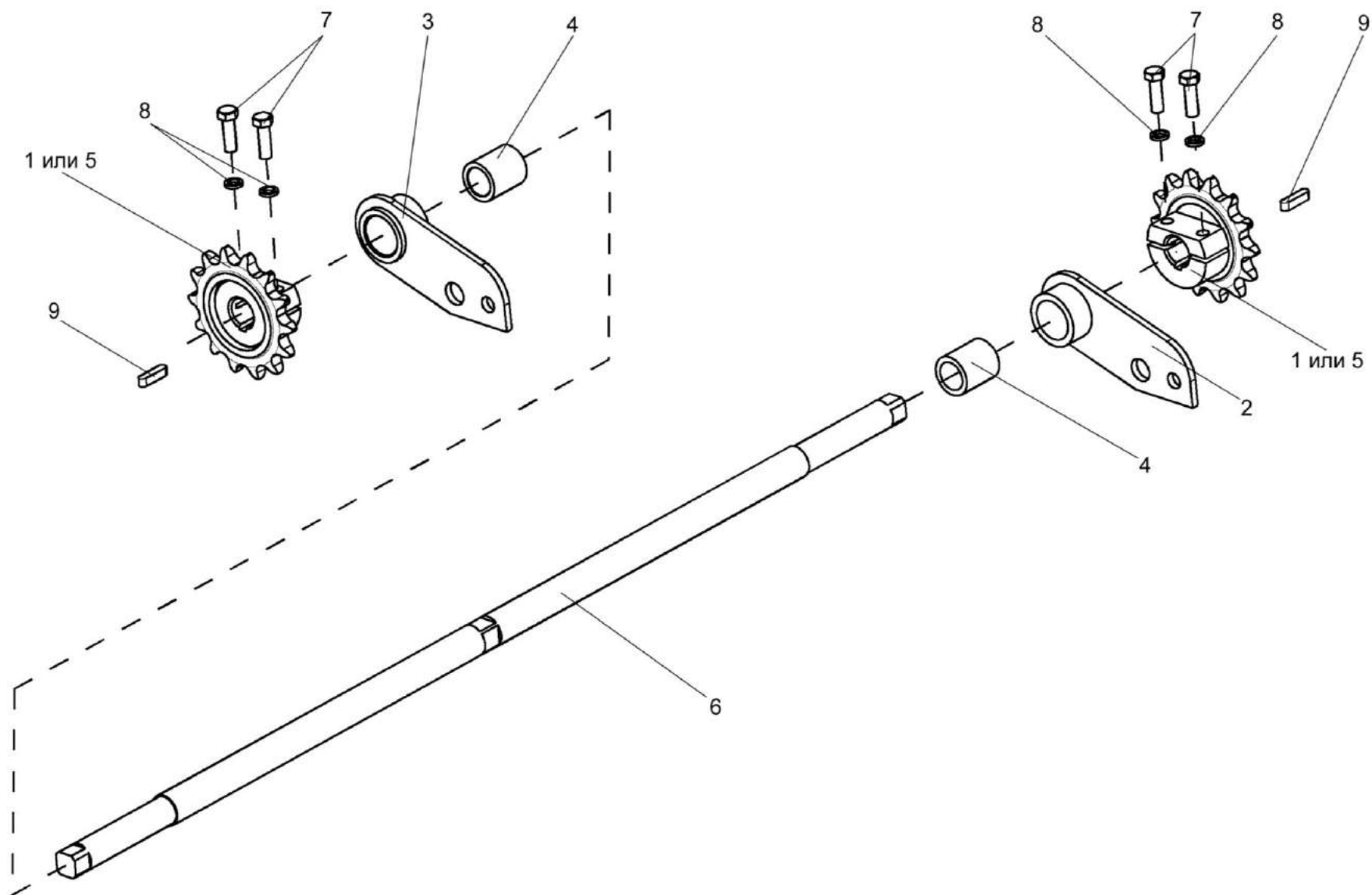
Рисунок 50 – Механизм перемещения КВС-1-0148170
