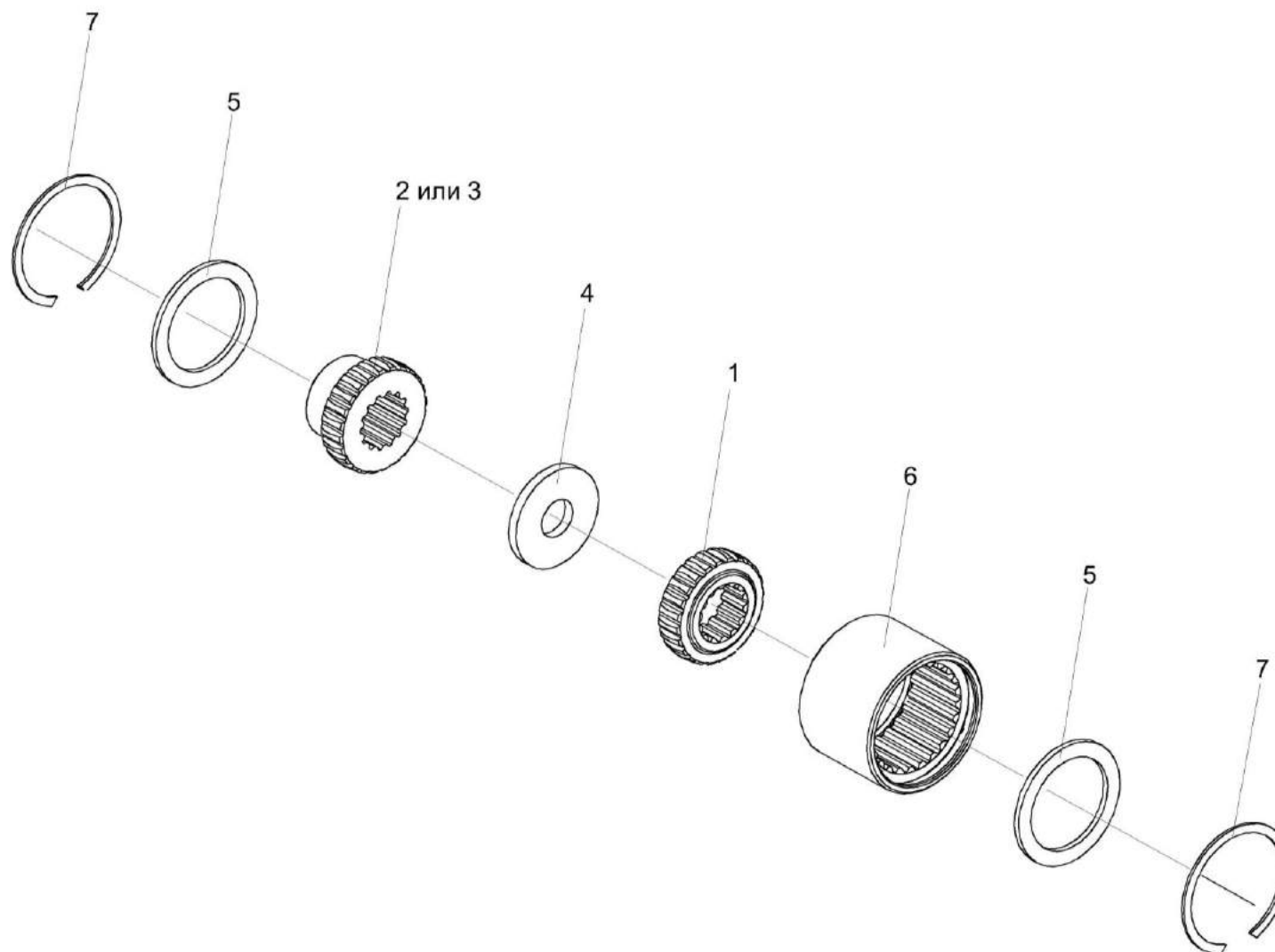
Рисунок 182 – Муфта КГС 0100110 и КГС 0100140
