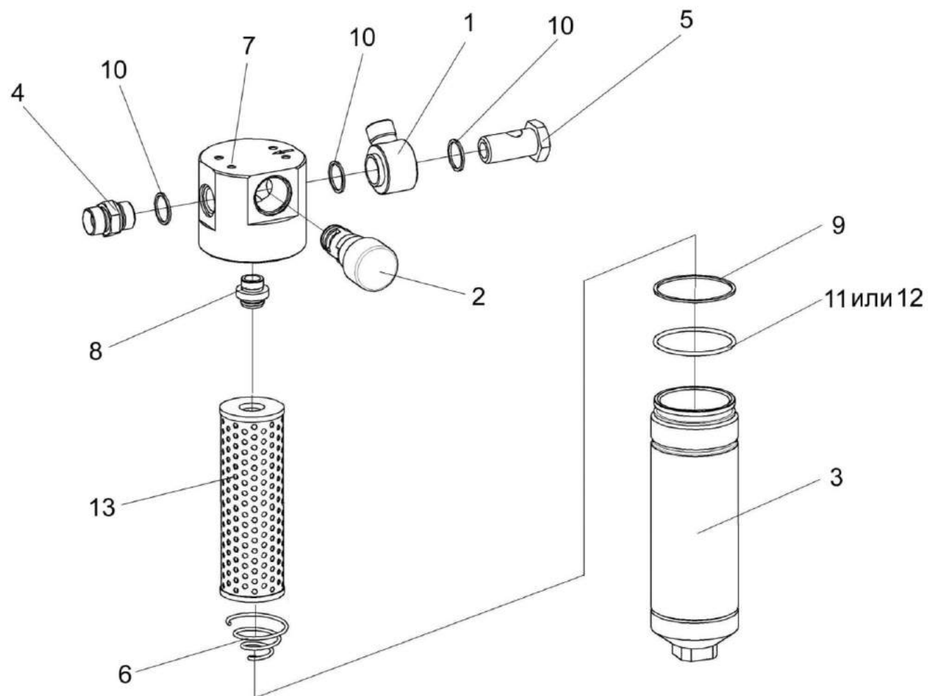
Рисунок 191 – Фильтр напорный КВС-5-0602370
