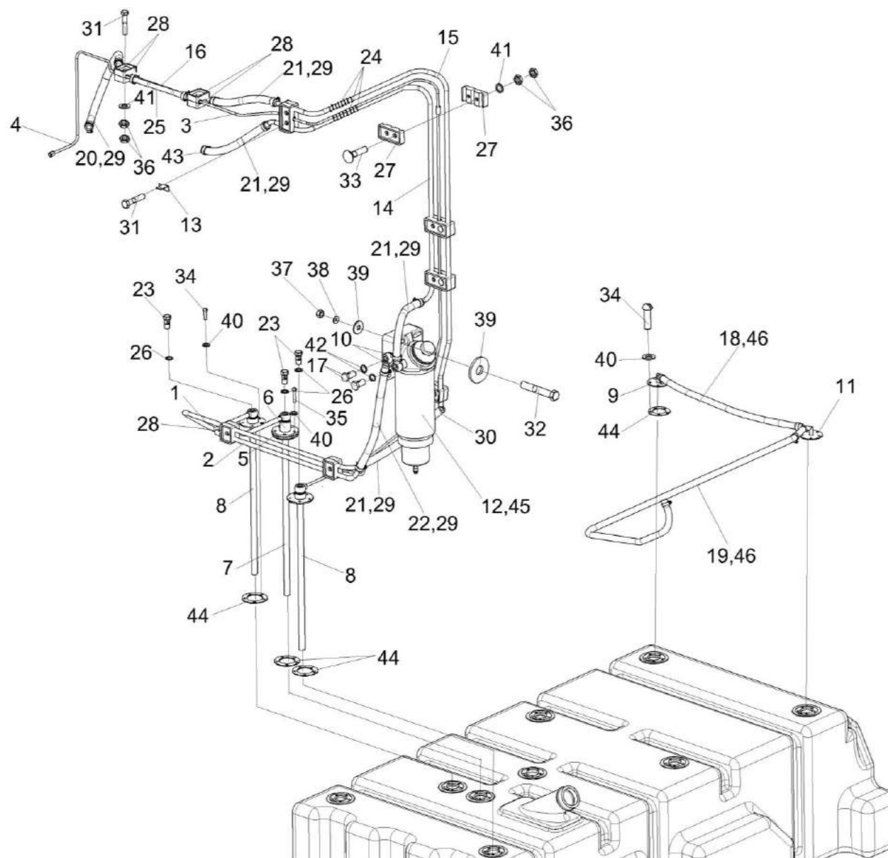
Рисунок 88 – Установка топливного оборудования КВС-5-0103700А (лист 2)
