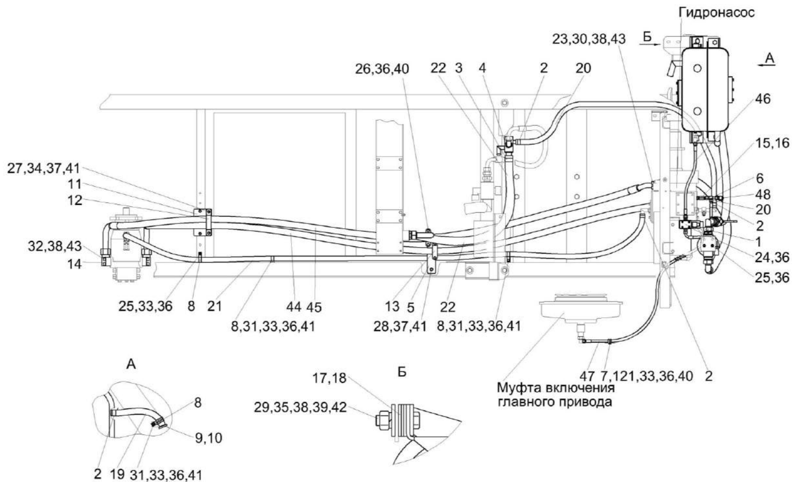
Рисунок 183 – Гидросистема привода ходовой части КВС-5-0601000 (лист 1)
