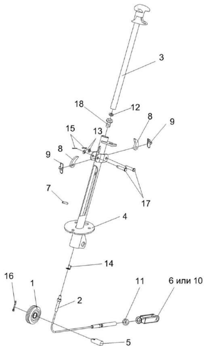
Рисунок 135 – Колонка привода УЭС 0300710
