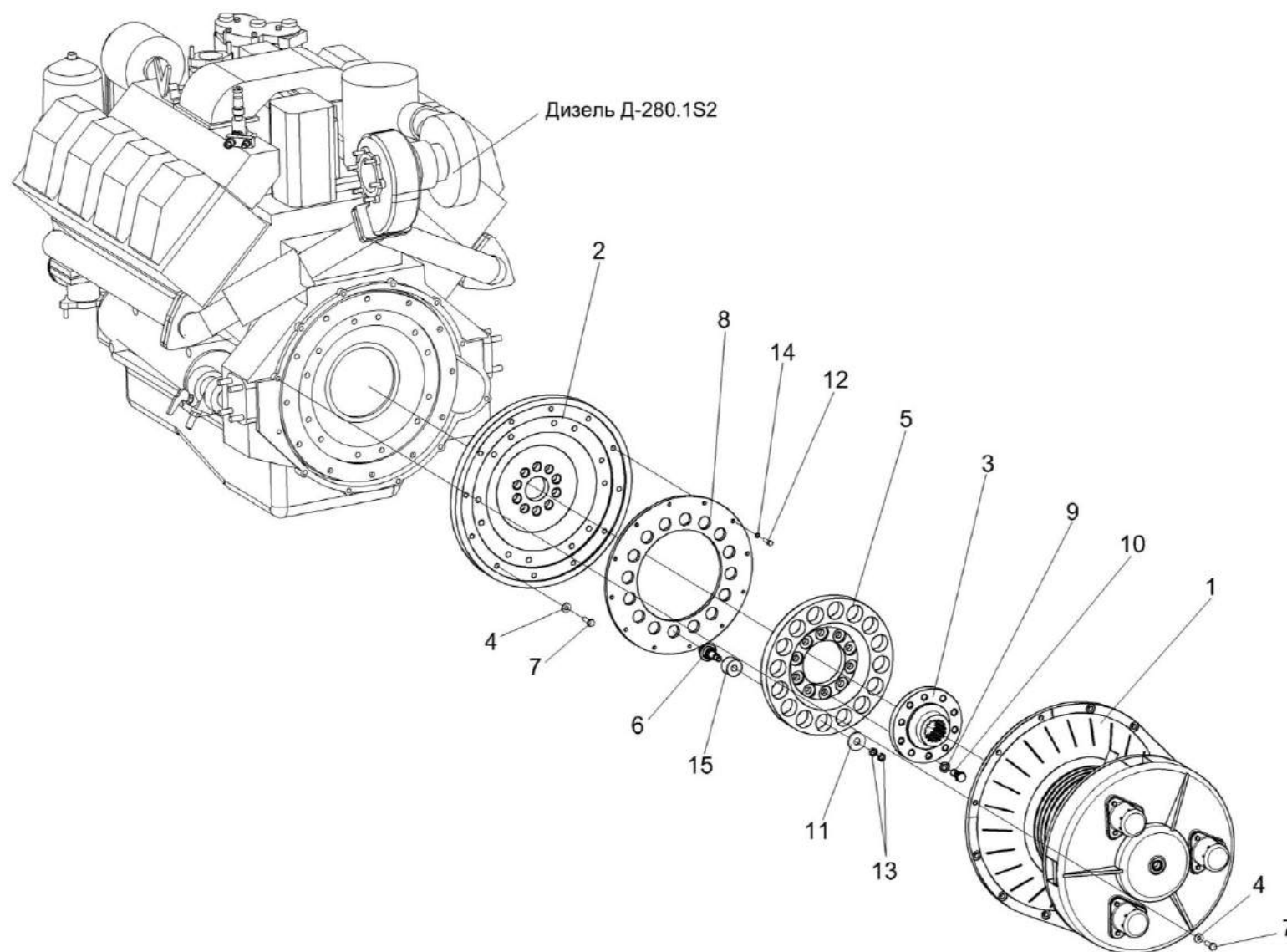
Рисунок 67 – Установка главного привода КВС-5-0151000В
