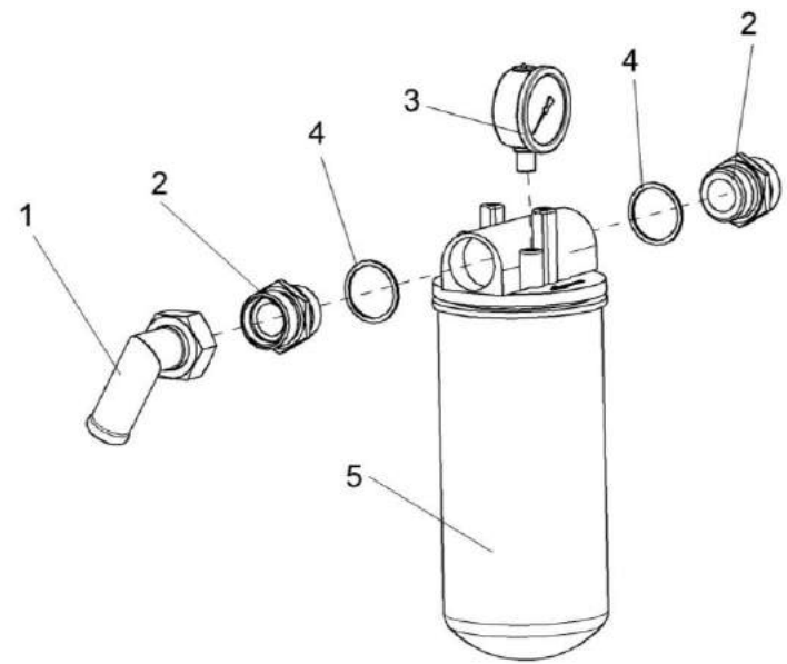
Рисунок 197 – Фильтр сливной КВС-2-0602020-01
