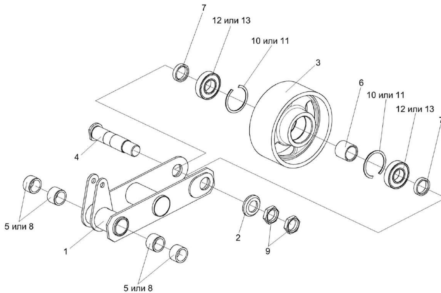
Рисунок 83 – Рычаг КВС-5-0133020
