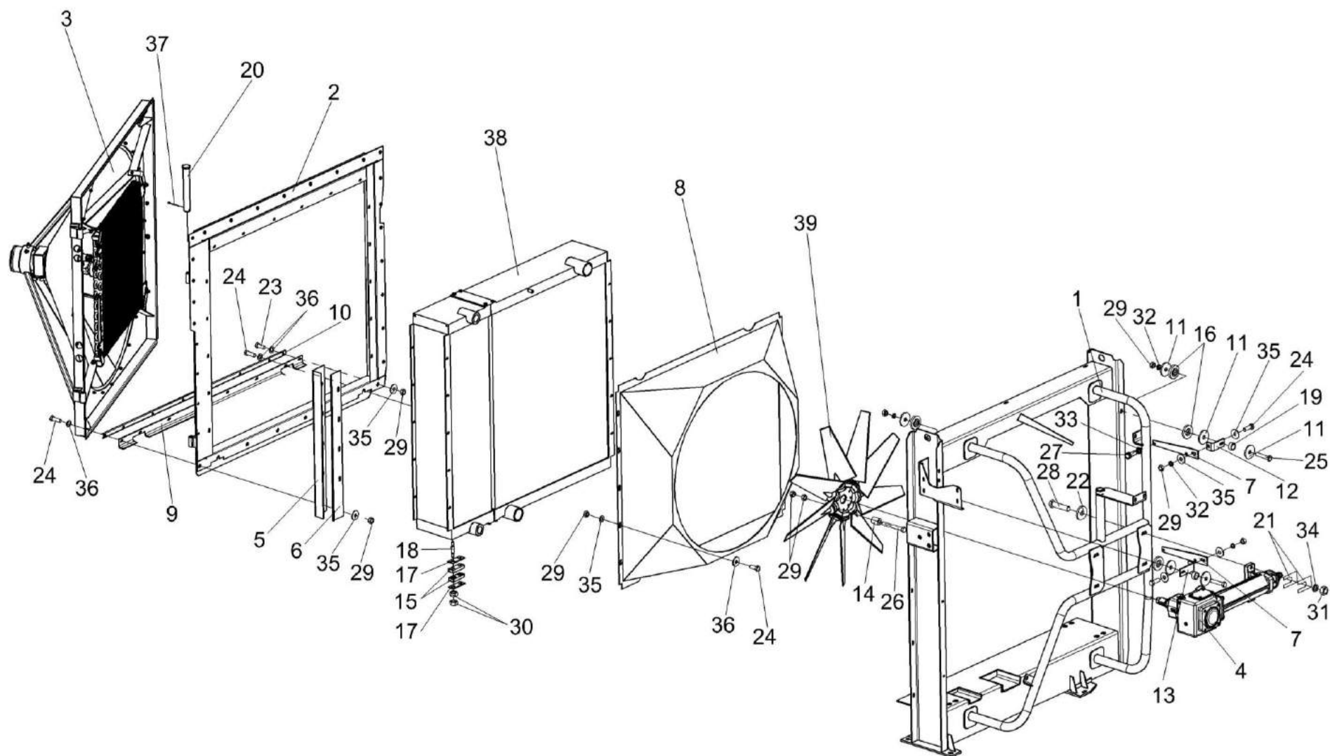
Рисунок 69 – Установка блока радиаторов КВС-5-0152000
