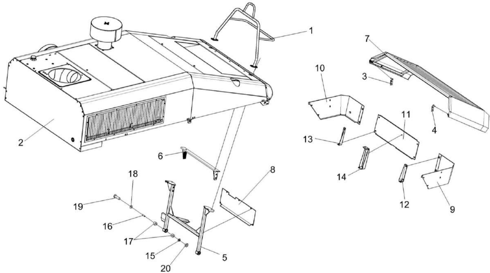
Рисунок 158 – Установка капотов КВС-2-0160000-03 (лист 3)
