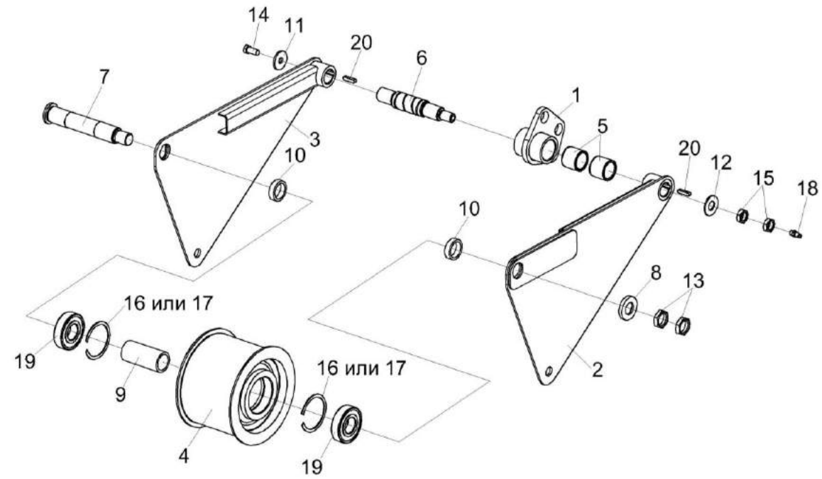
Рисунок 35 – Рычаг КВС-2-0130050
