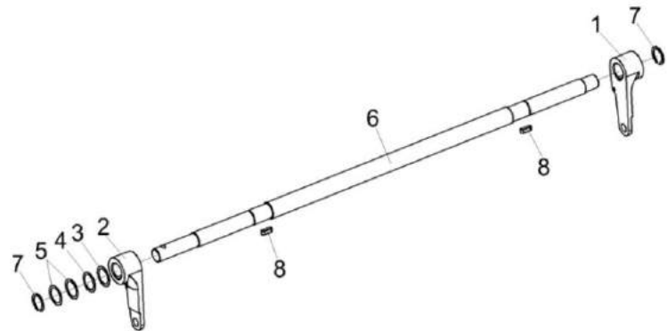
Рисунок 26 – Привод КВС-1-0115140Б
