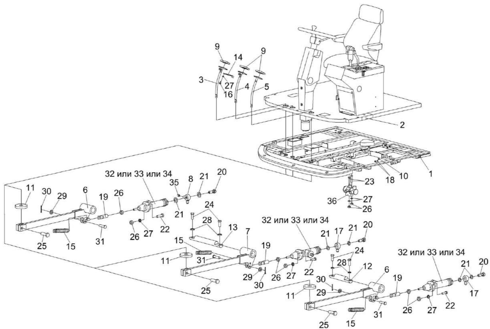
Рисунок 115 – Площадка управления КВС-5-0129000-04 (лист 2)
