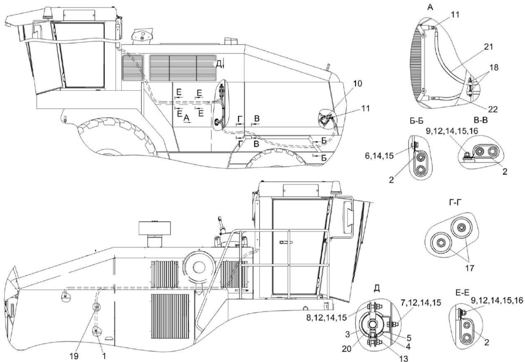
Рисунок 154 – Установка климатическая КВС-5-0121000А
