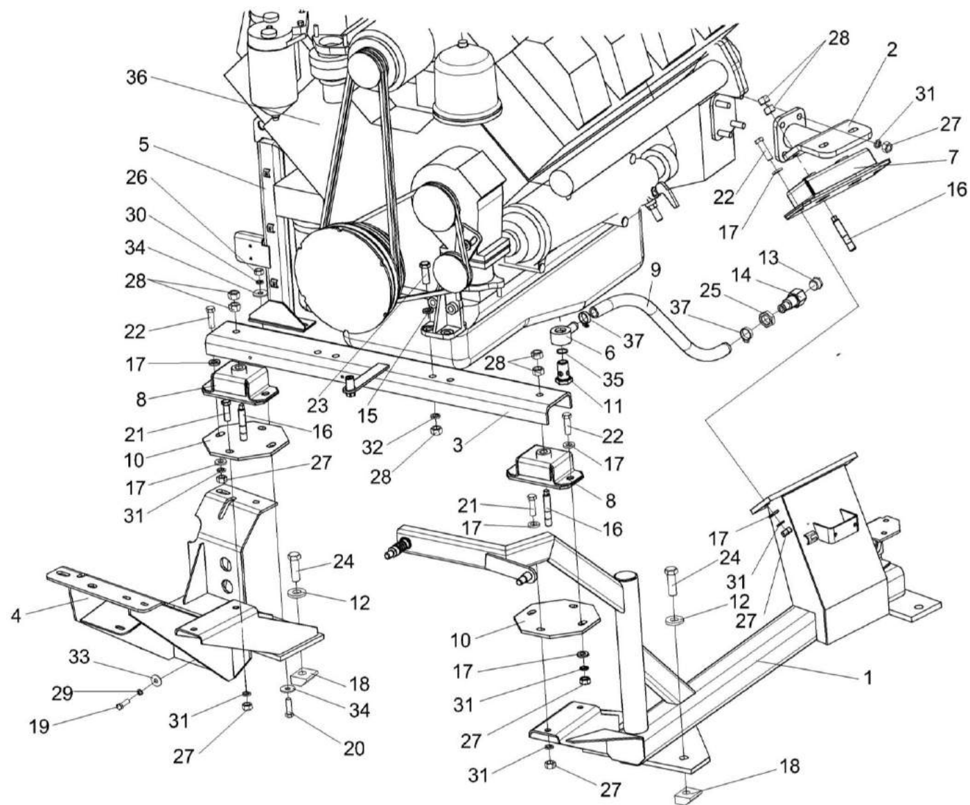
Рисунок 65 – Установка дизеля Д-280.1S2 КВС-5-0150000А (установка дизеля) (лист 1)
