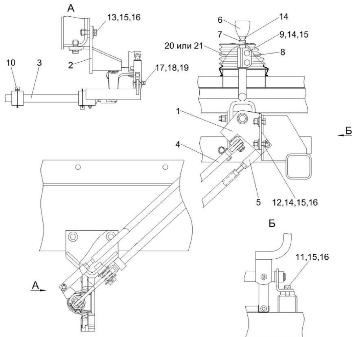
Рисунок 138 – Установка механизма управления коробкой диапазонов КВС-2-0129040
