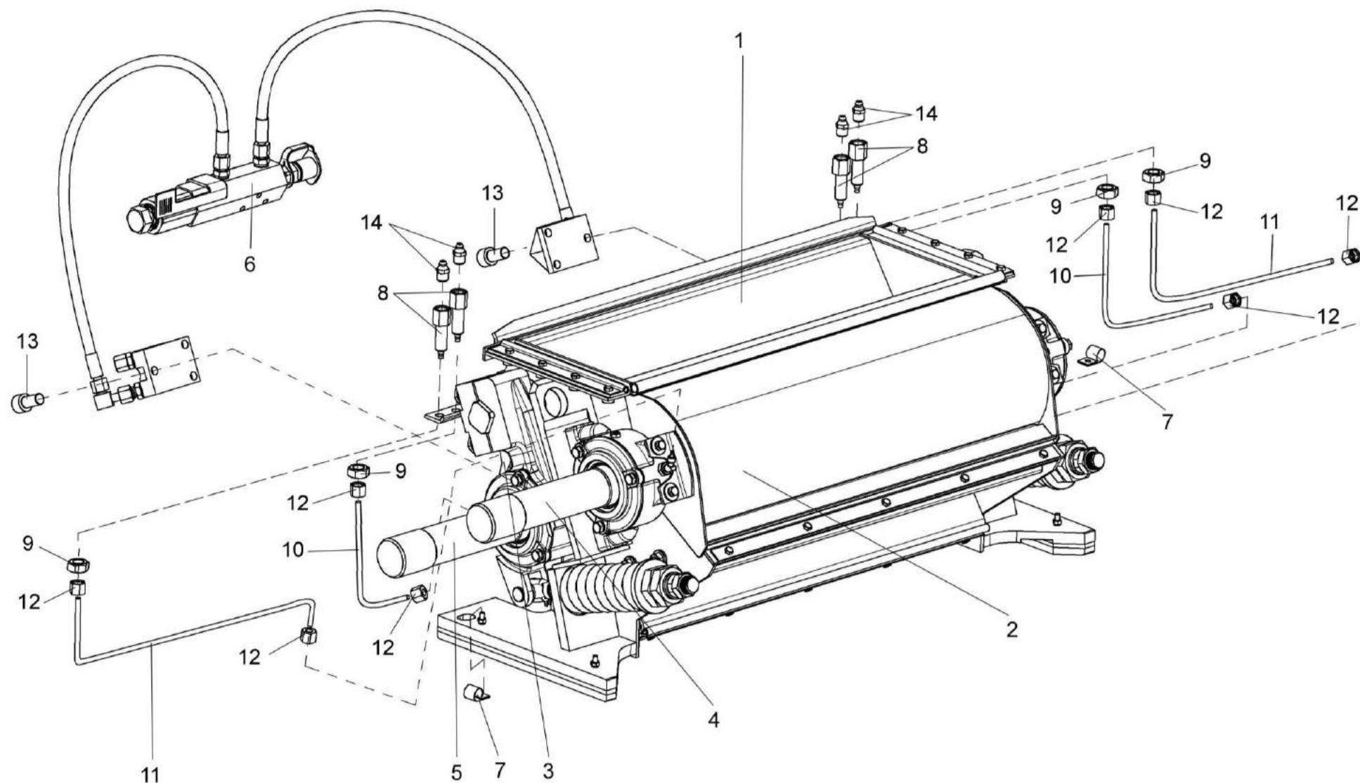
Рисунок 40 – Устройство доизмельчающее КВС-1-0148310
