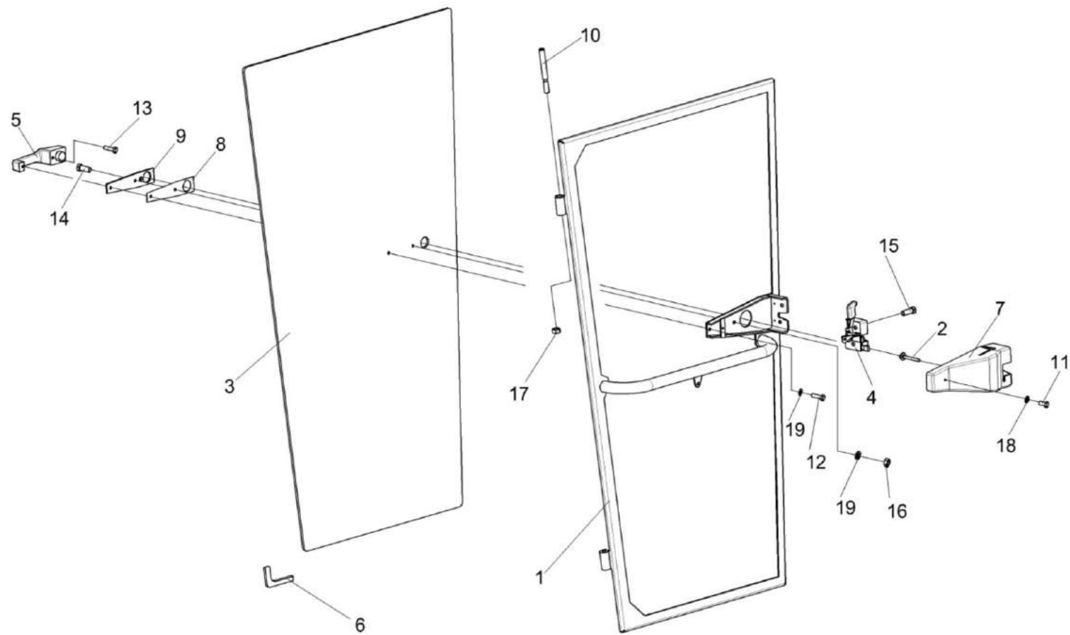
Рисунок 150 – Дверь КЗК-10-0200140
