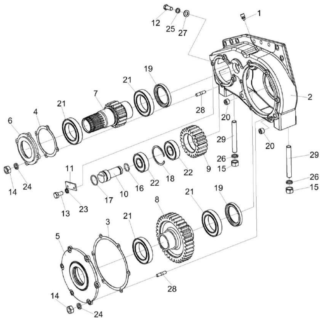
Рисунок 16 – Редуктор нижних вальцев КВС-2-0113000
