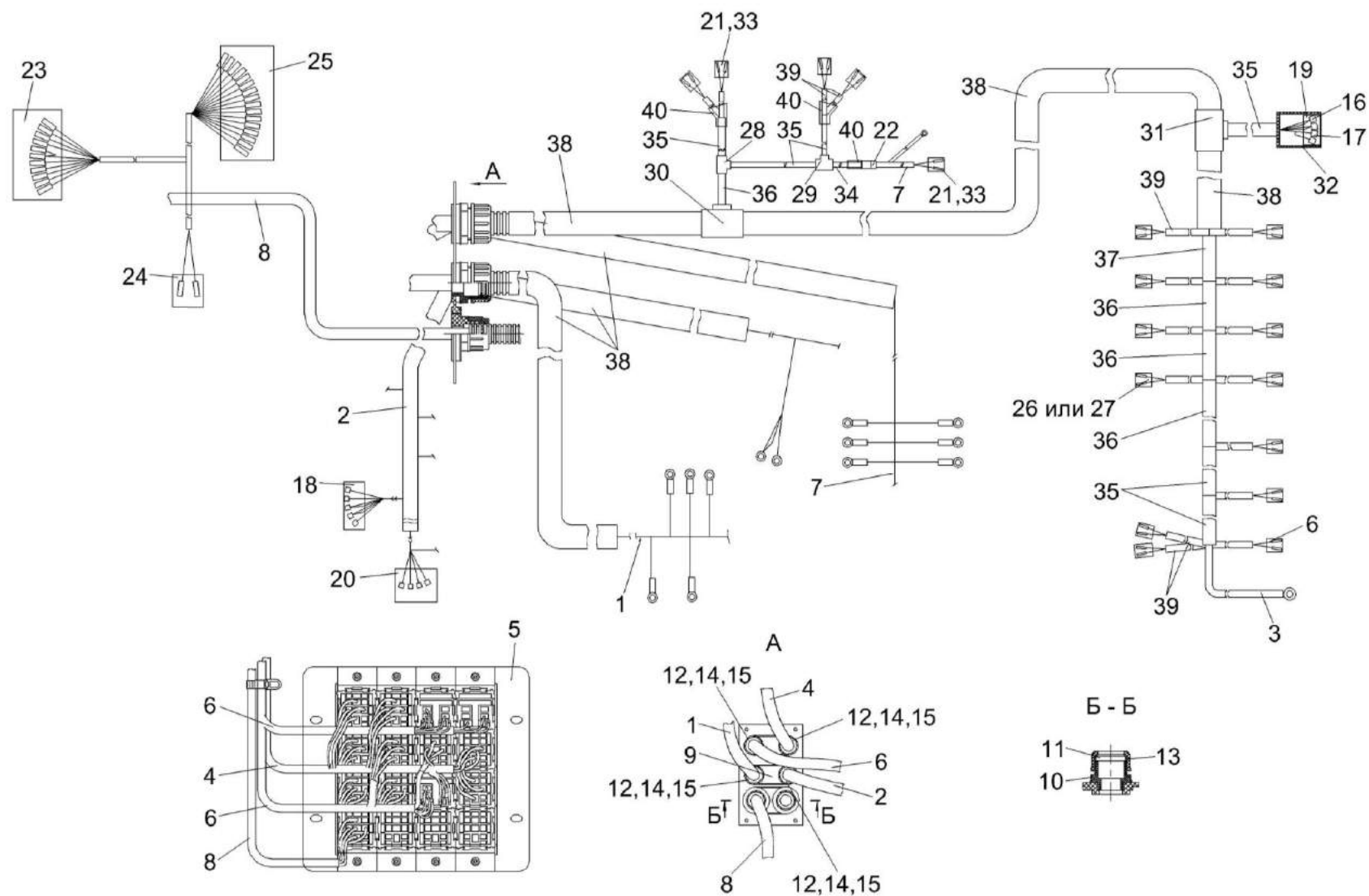
Рисунок 123 – Панель ввода жгутов КВС-5-0700470-01
