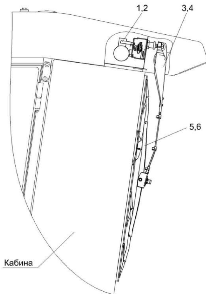
Рисунок 151 – Установка стеклоочистителя КЗК-12-0120810 или КЗК-12-0120810-01
