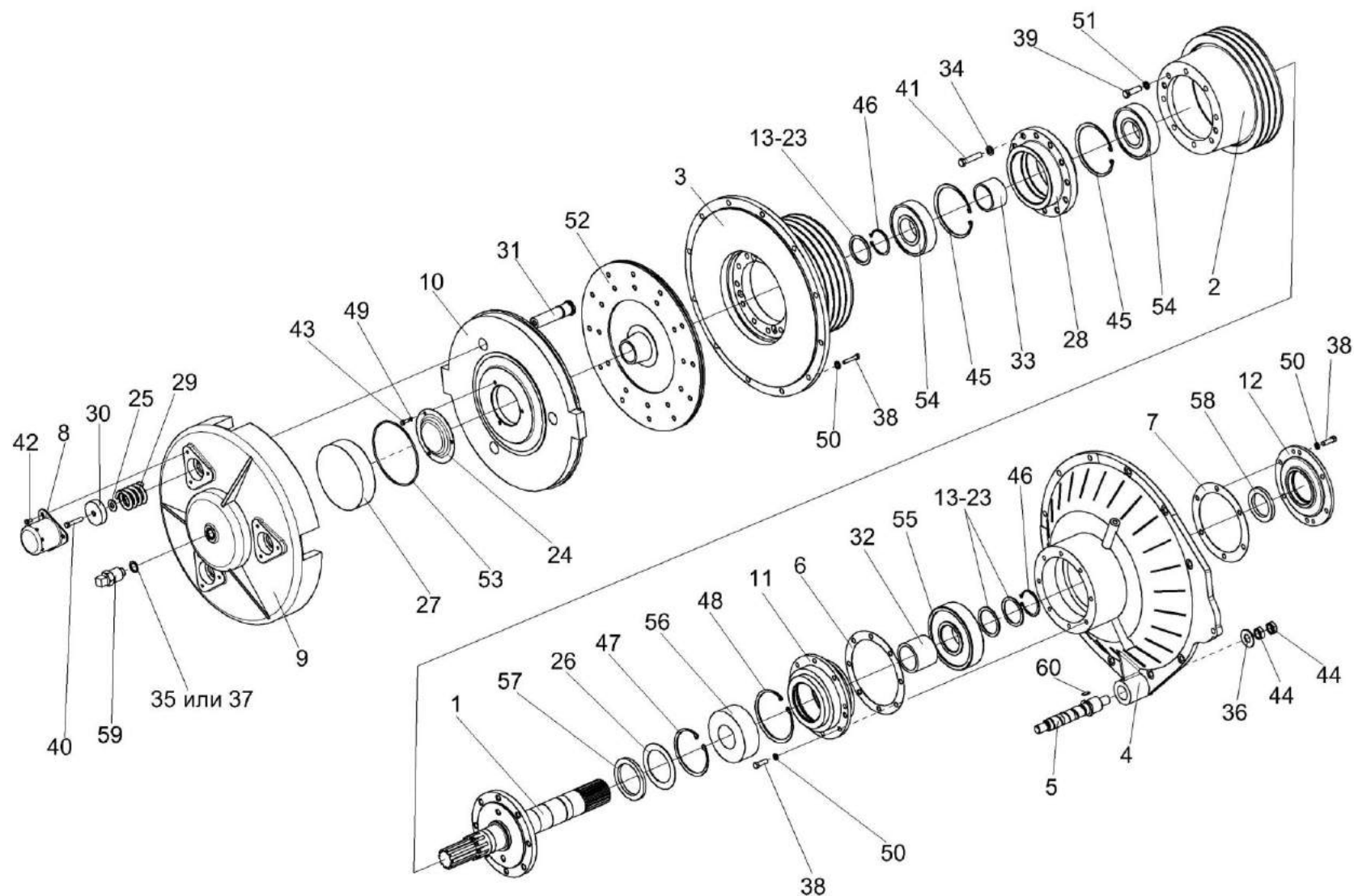
Рисунок 68 – Главный привод КВС-5-0151000В
