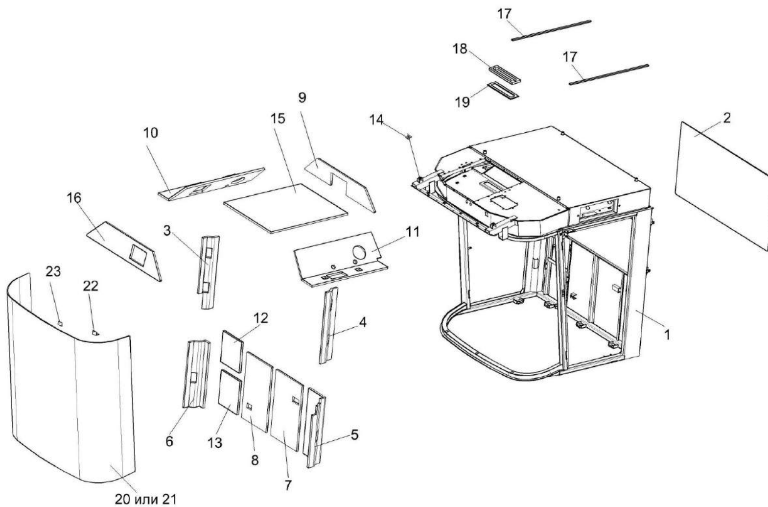
Рисунок 148 – Каркас КВС-2-0122010
