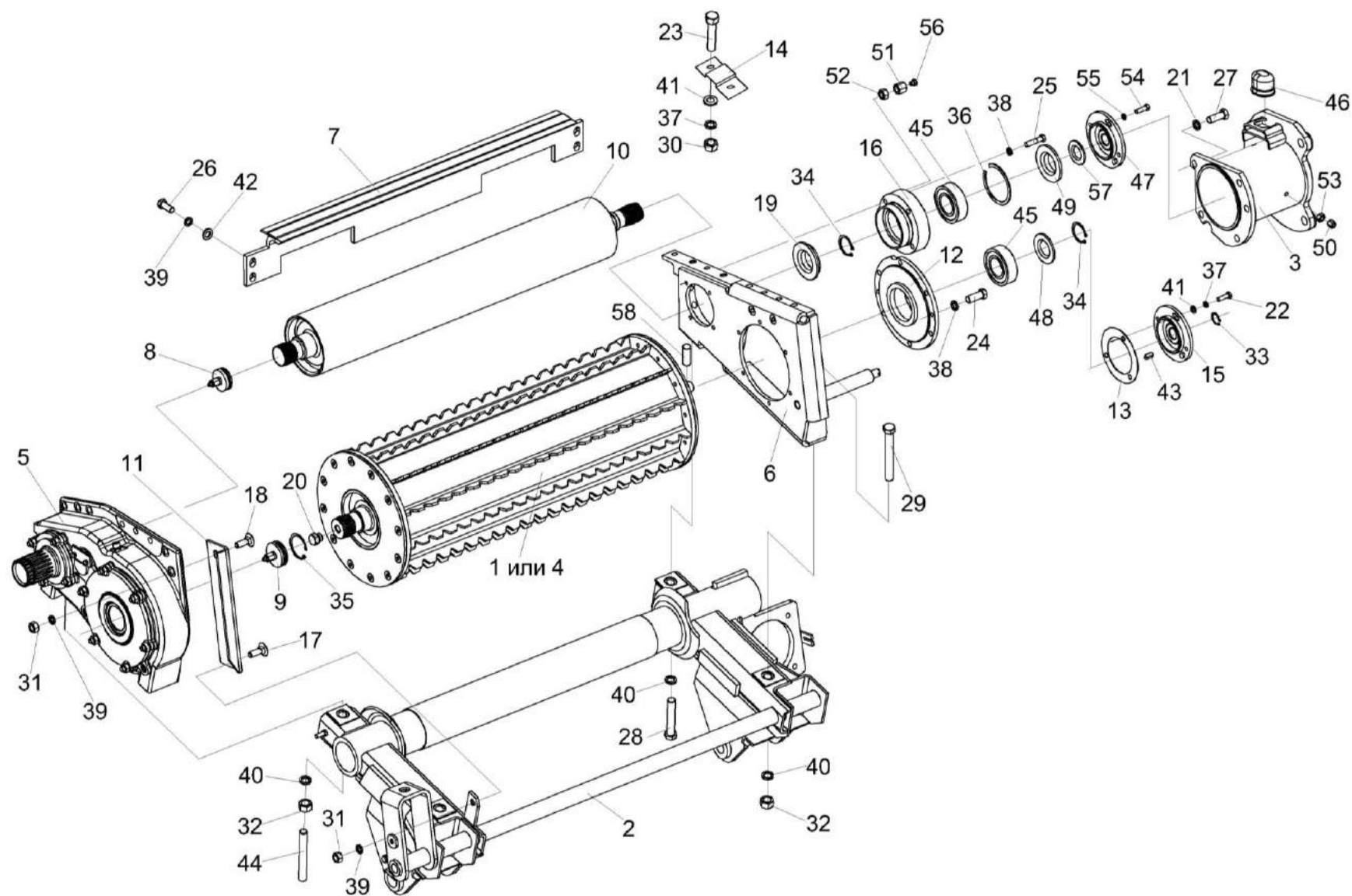
Рисунок 13 – Вальцы нижние КВС-2-0111200Г-02
