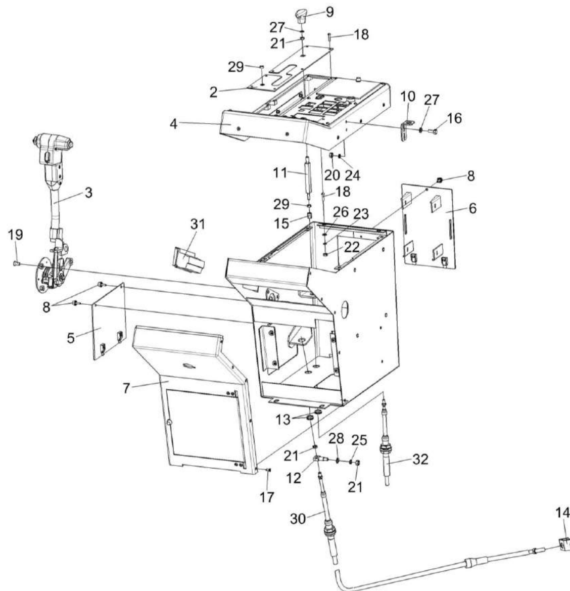
Рисунок 117 – Пульт управления КВС-5-0129050А-02
