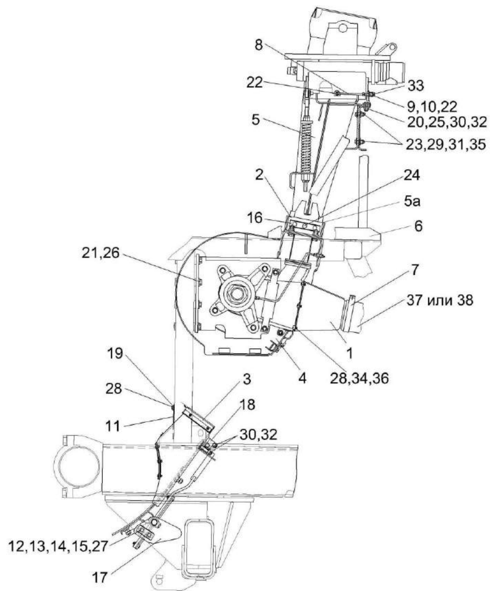
Рисунок 51 – Установка ускорителя выброса, камеры приемной и основания силосопровода КВС-1-0140000
