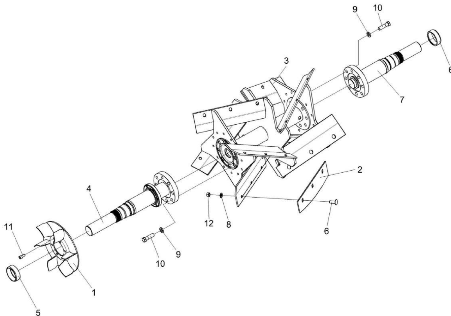
Рисунок 56 – Вал ускорителя выброса КВС-1-0142910
