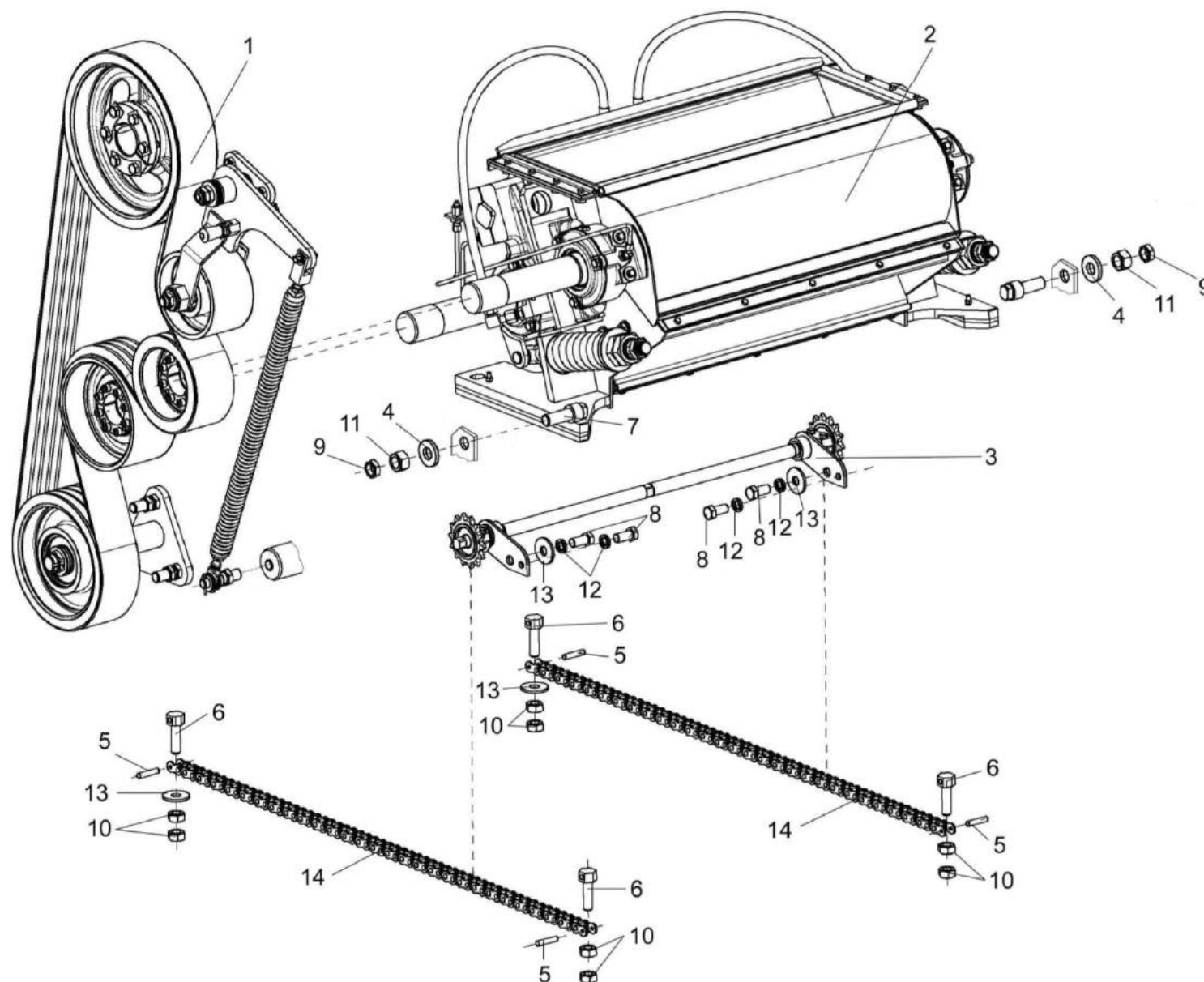
Рисунок 36 – Устройство доизмельчающее КВС-1-0148000
