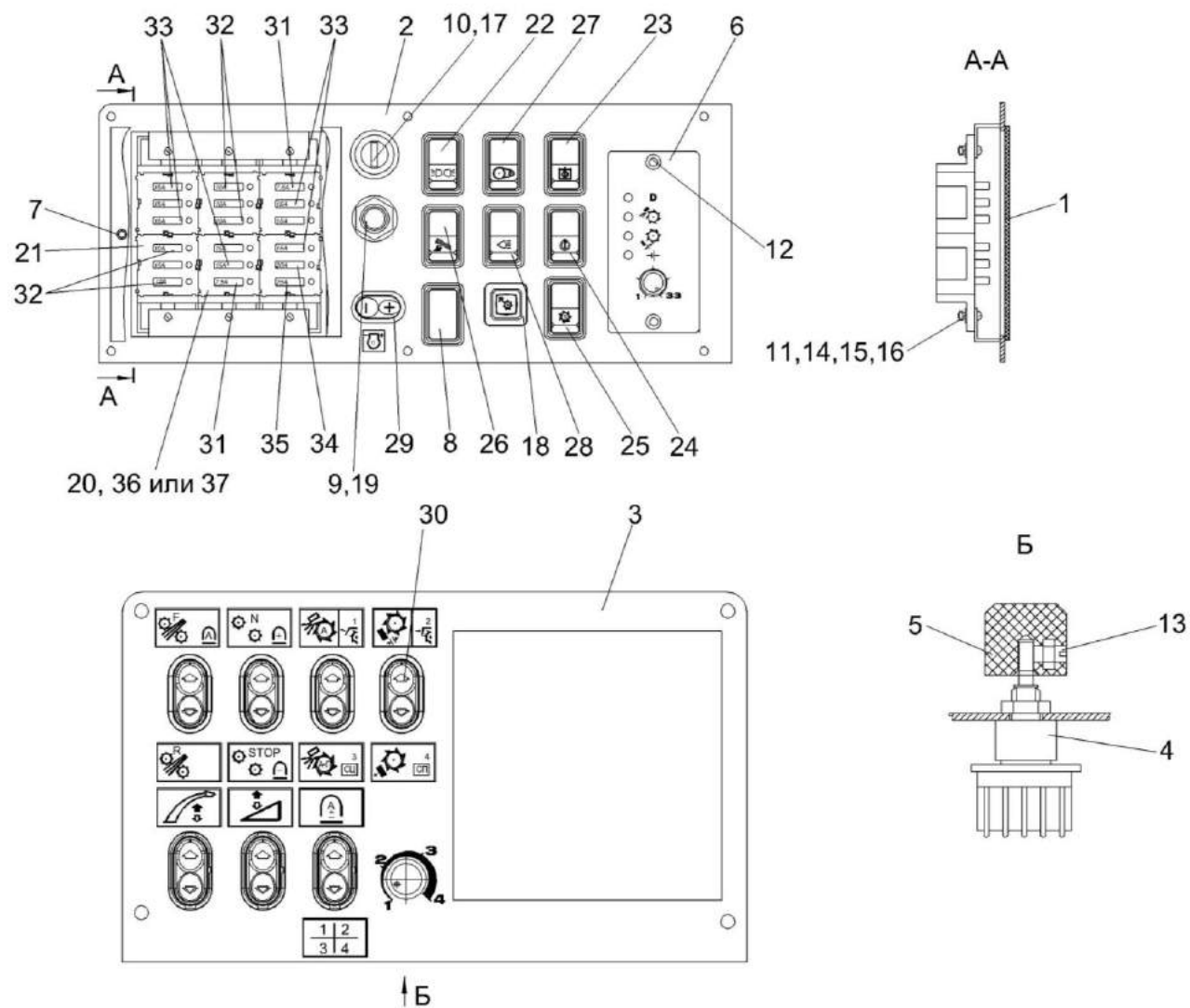
Рисунок 122 – Панели пульта управления КВС-5-0700450 и КВС-2-0700460Б
