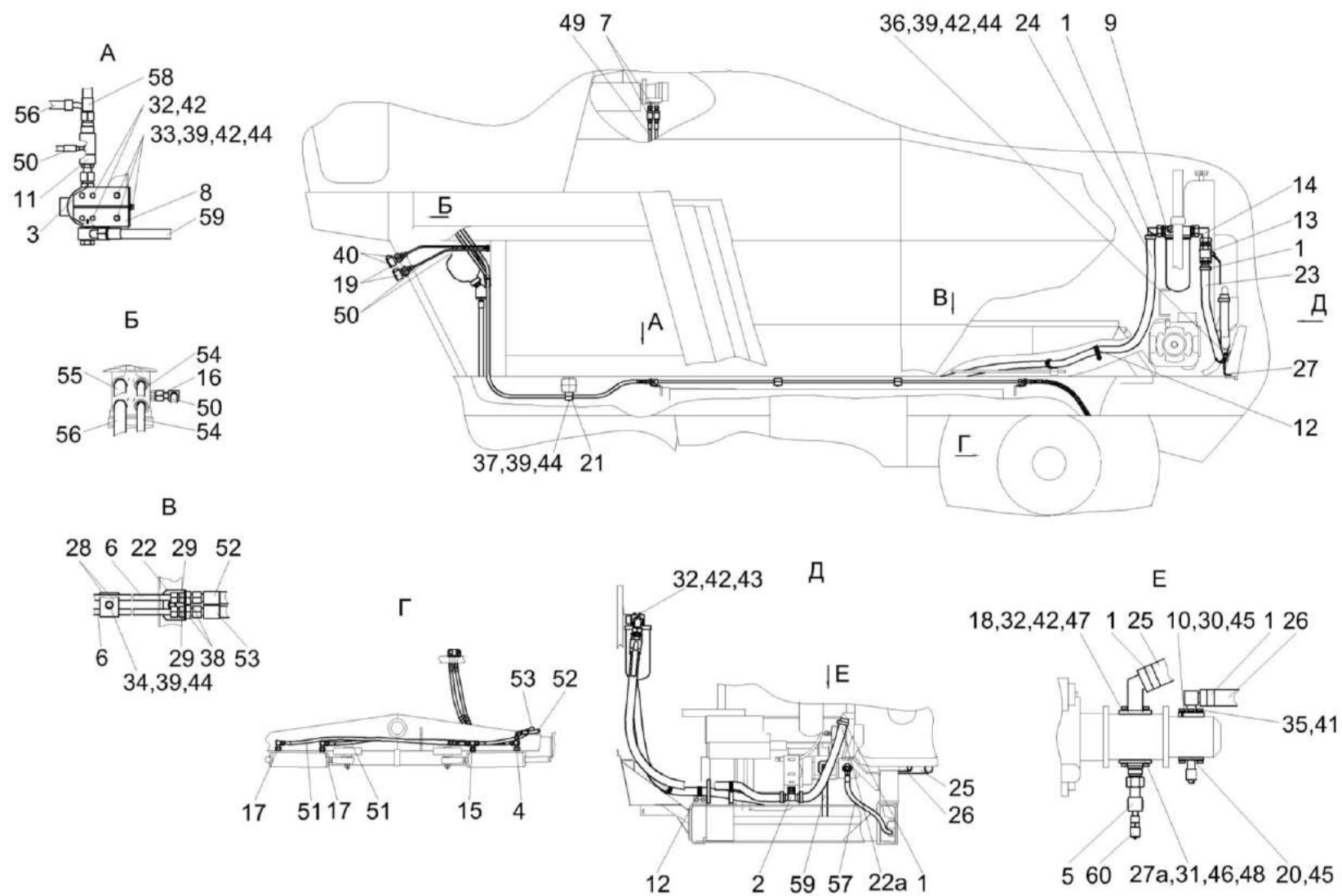
Рисунок 189 – Гидросистема рабочих органов и рулевого управления КВС-5-0602000 (лист 2)
