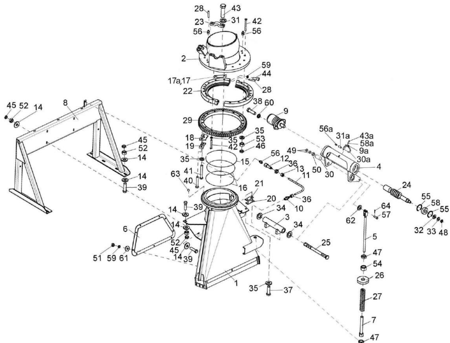
Рисунок 58 – Основание силосопровода и механизм поворота КВС-1-0143000
