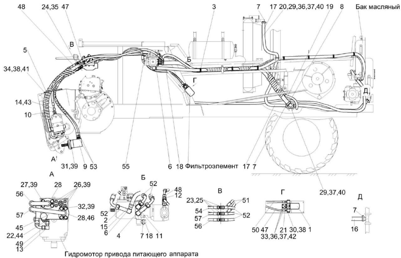
Рисунок 168 – Гидросистема привода питающего аппарата и адаптеров комбайна КВК-800-36 КВС-5-0604000 (лист 1)
