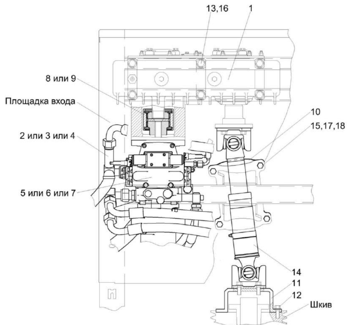
Рисунок 165 – Установка гидросистемы привода питающего аппарата и адаптеров КВС-2-0131500 , КВС-2-0131500-01 и КВС-2-0131500-02
