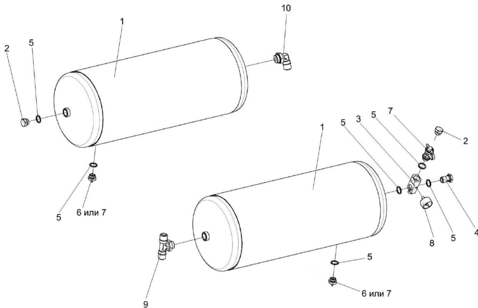
Рисунок 205 – Ресиверы КВС-5-0800030 и КВС-5-0800050
