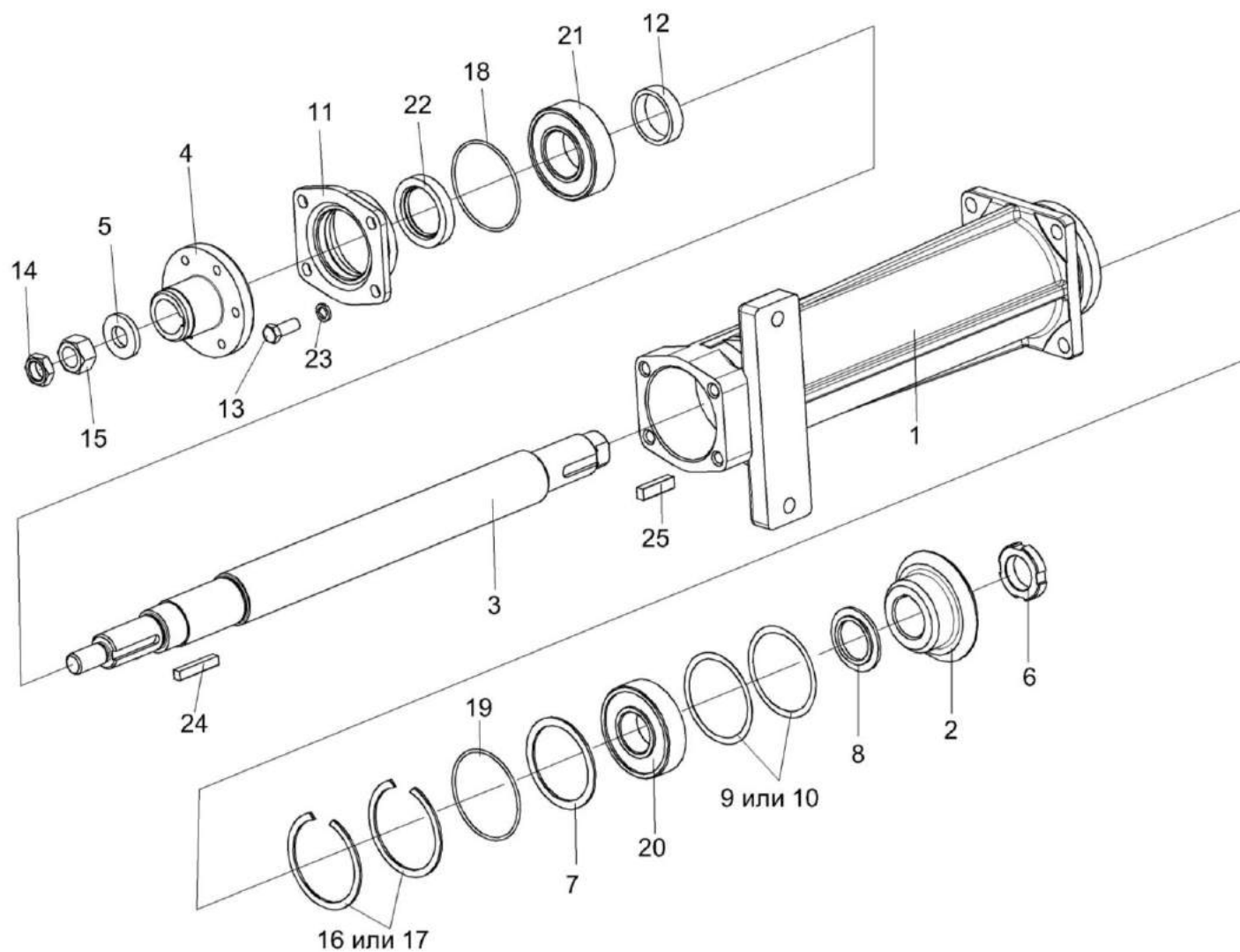
Рисунок 74 – Стакан КВС-1-0135020А
