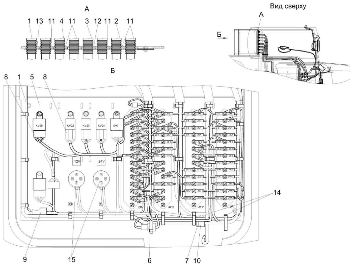
Рисунок 210 – Электрооборудование электрощафа KBC-2-0702010A-01
