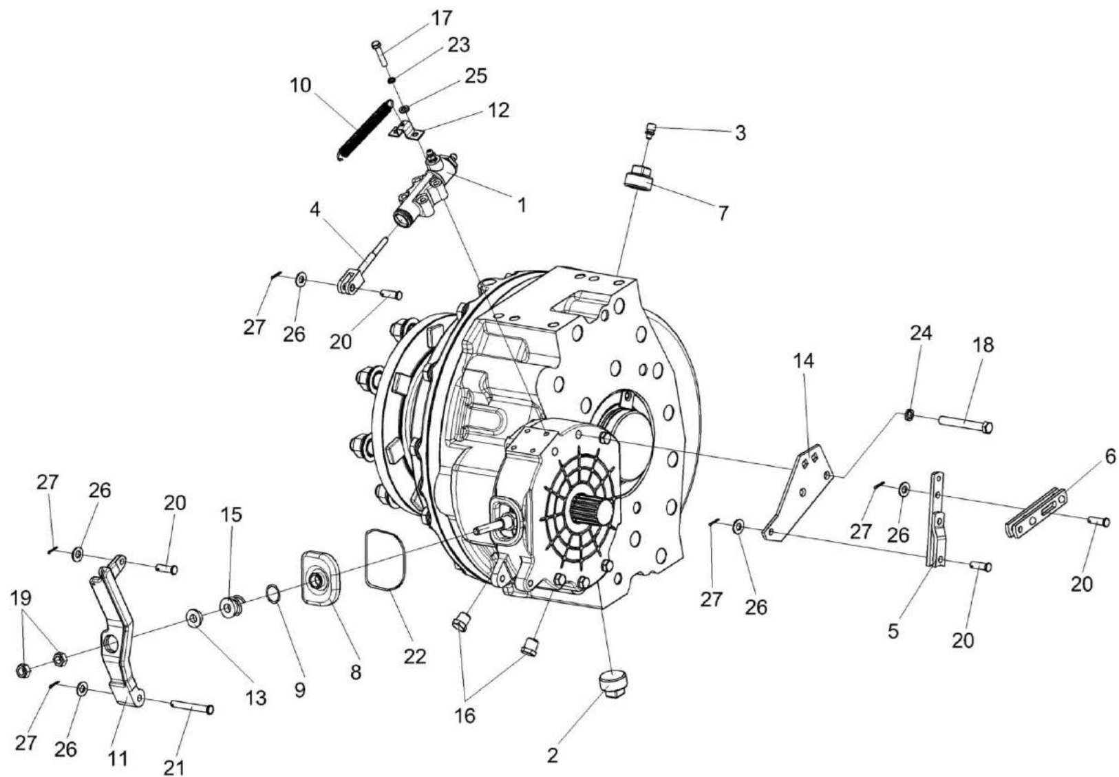
Рисунок 94 – Редуктор бортовой КЗК-10-0107200-02
