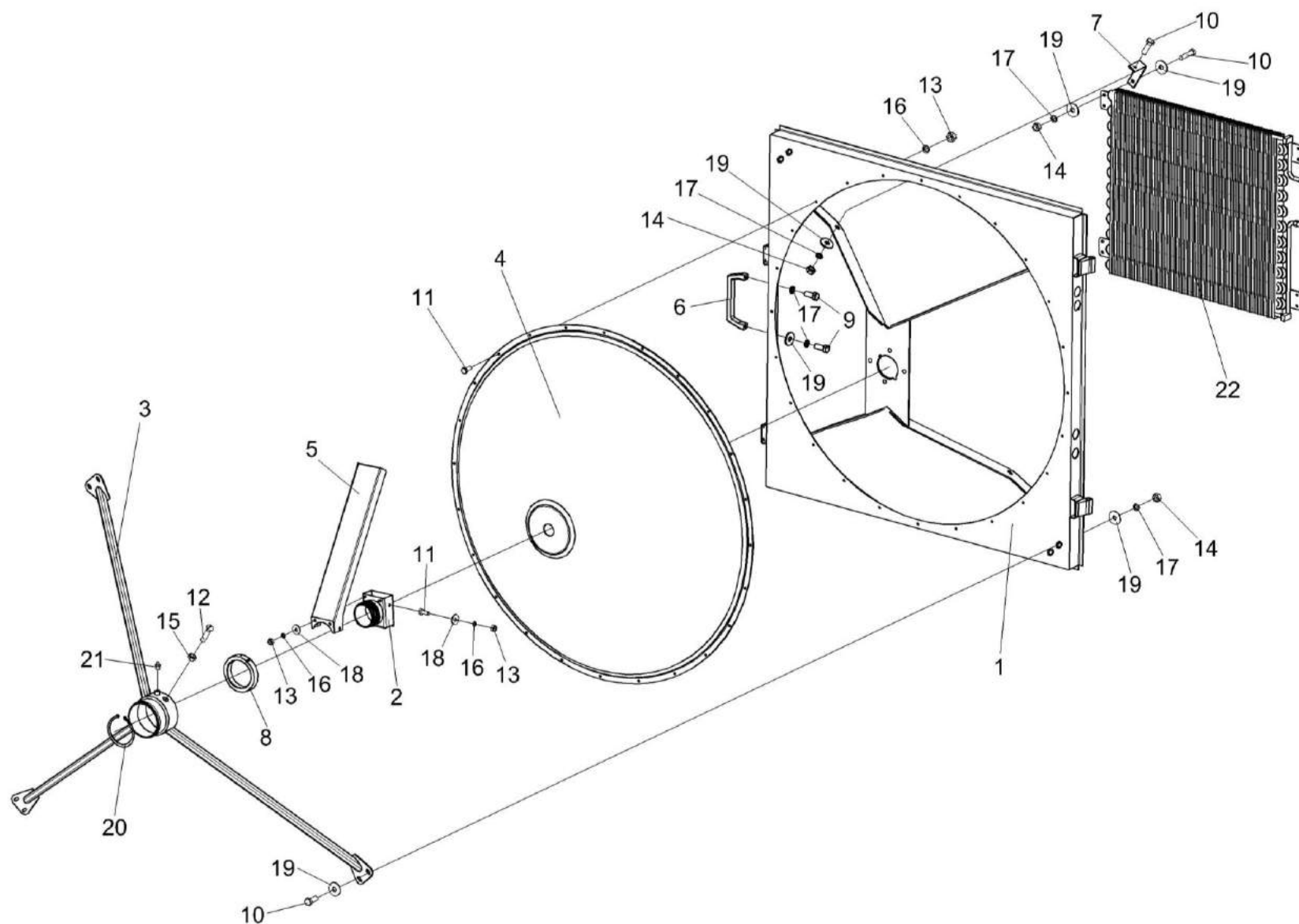
Рисунок 70 – Воздухозаборник КВС-5-0155000 (лист 1)
