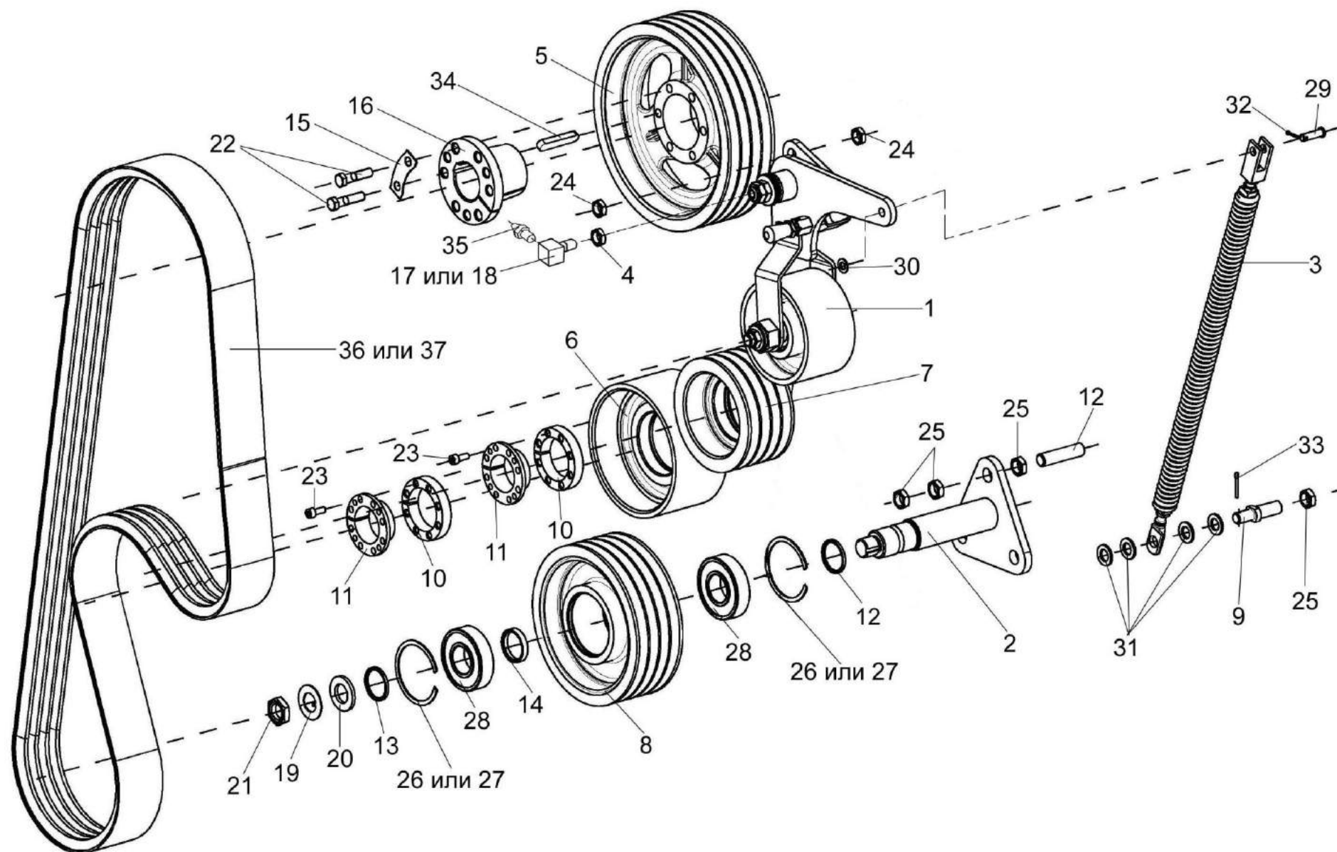
Рисунок 37 – Привод доизмельчающего устройства KBC-1-0132100
