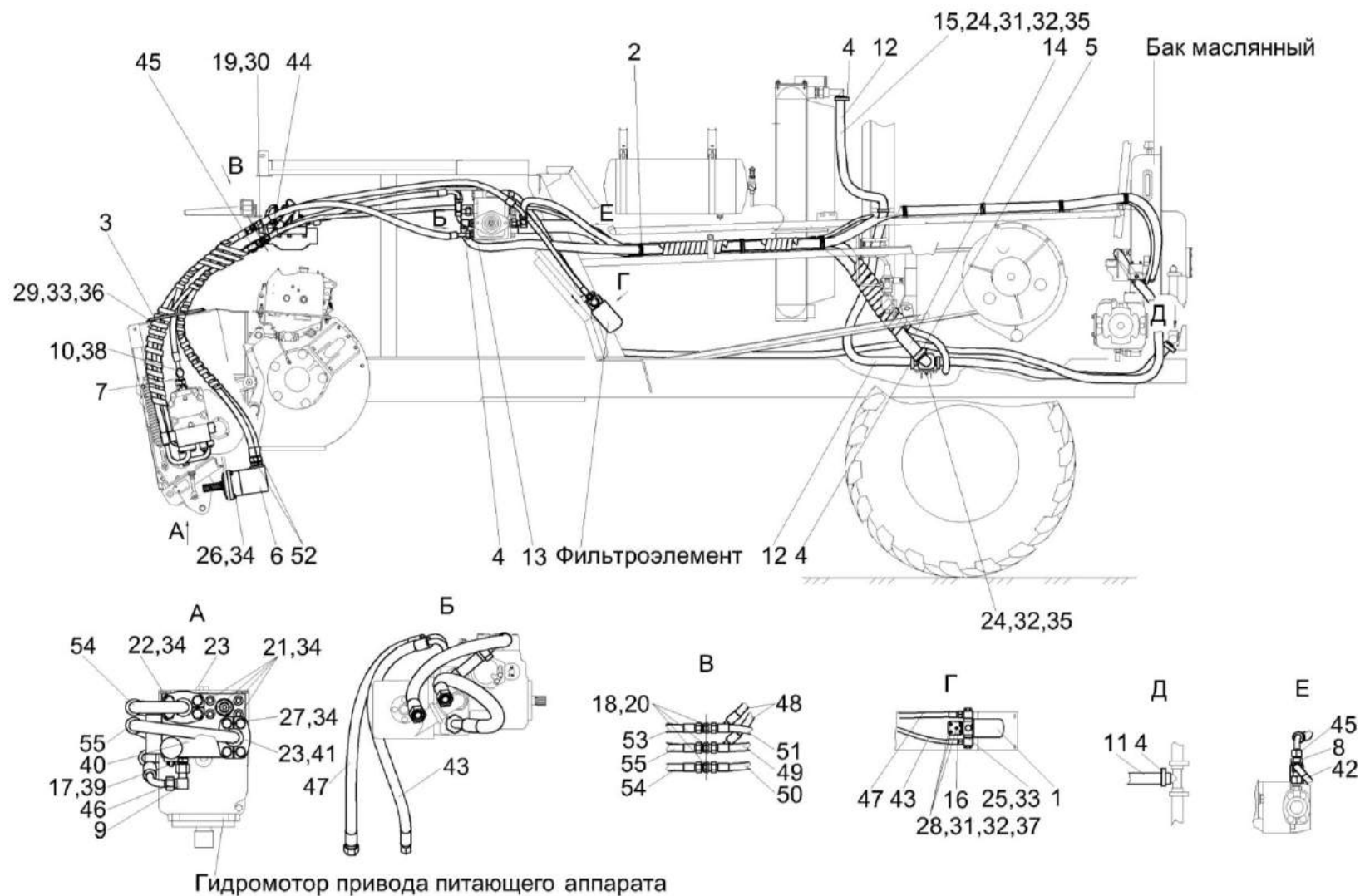
Рисунок 170 – Гидросистема привода питающего аппарата и адаптеров комбайна КВК-800-36 КВС-5-0614000 (лист 1)
