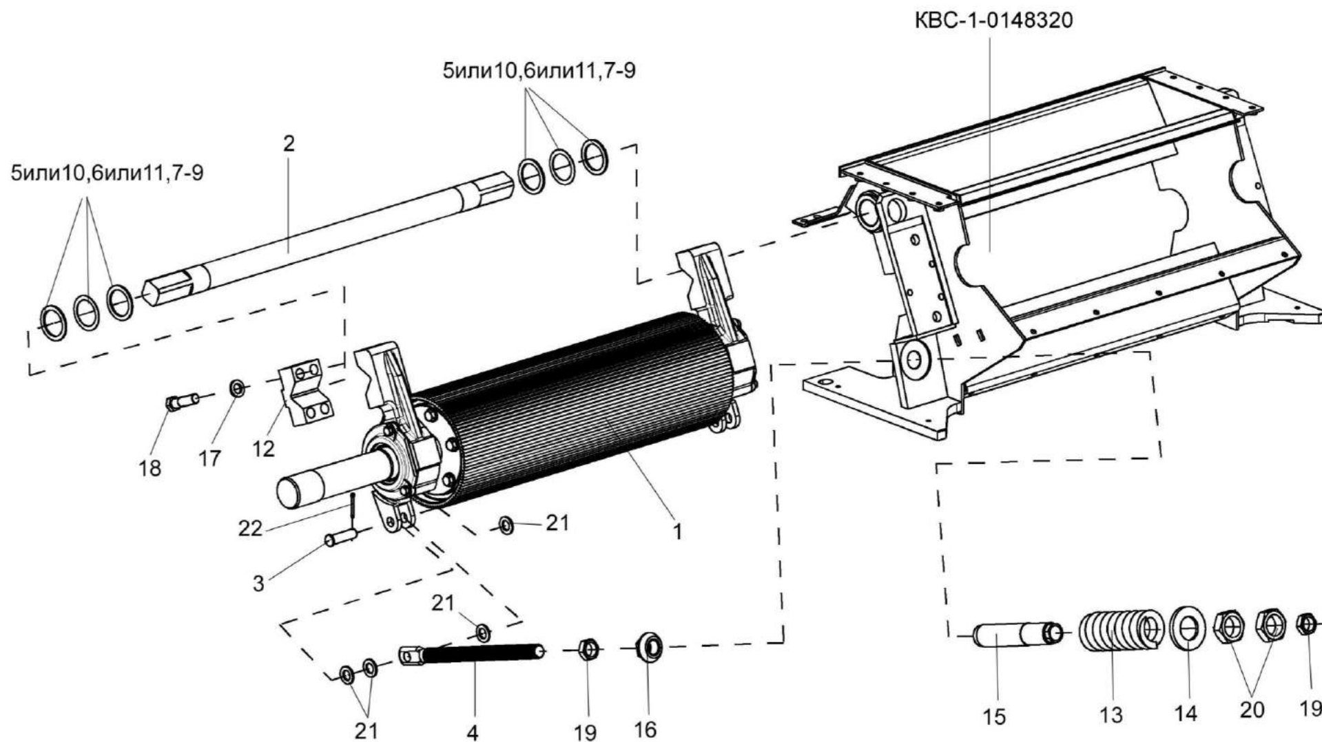
Рисунок 43 – Устройство доизмельчающее КВС-1-0148310 (установка нижнего вальца)
