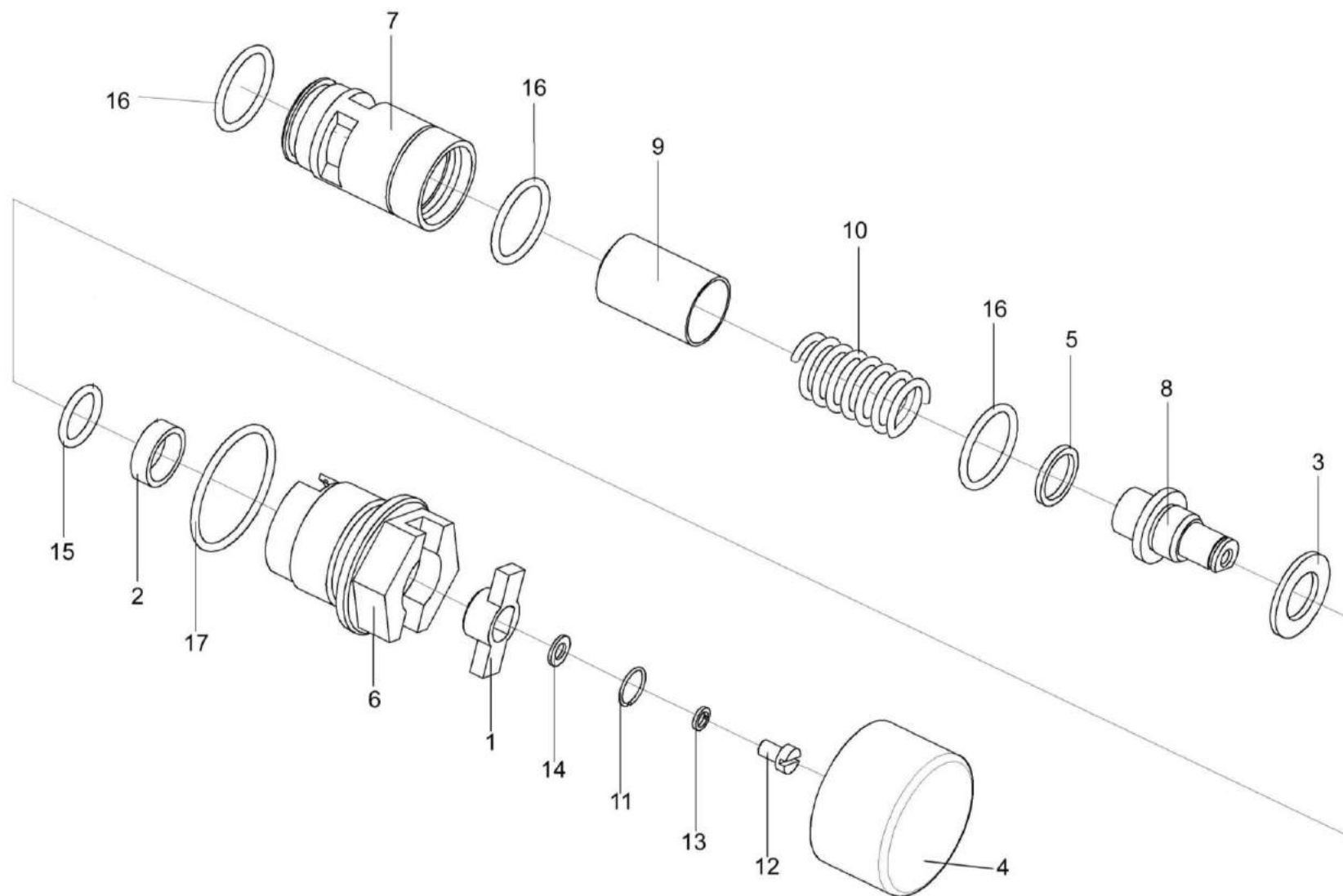
Рисунок 192 – Клапан-сигнализатор УЭС 0603660-01
