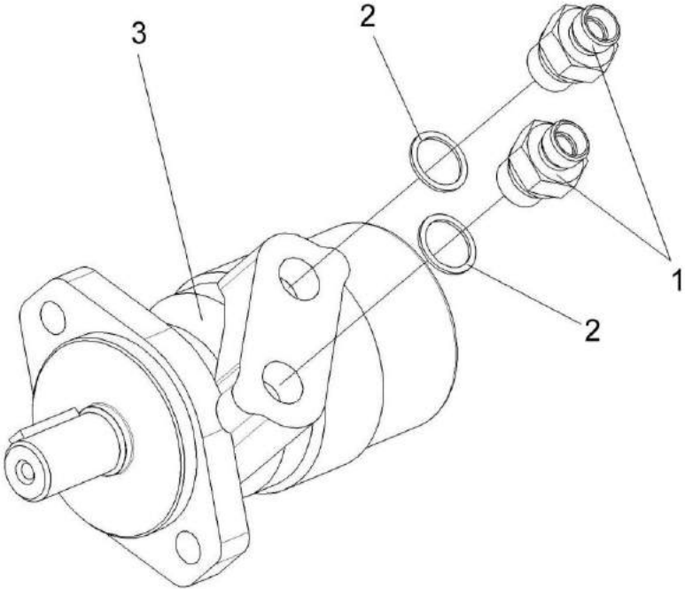
Рисунок 72 – Гидромотор воздухозаборника КВС-5-0602100
