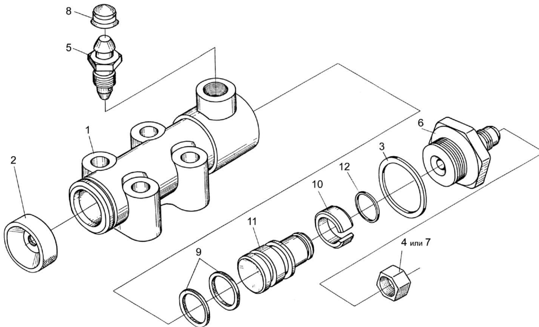
Рисунок 112 – Гидроцилиндр тормоза МК-23М.03.220А
