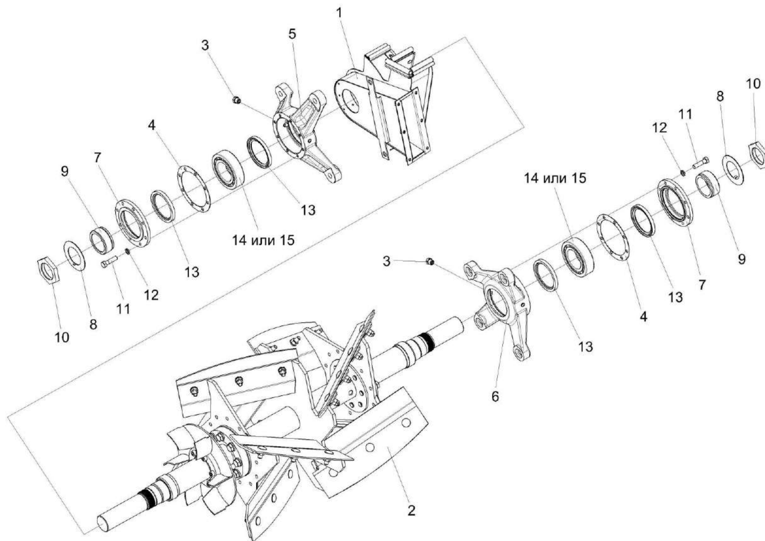
Рисунок 57 – Вал ускорителя выброса КВС-2-0142100
