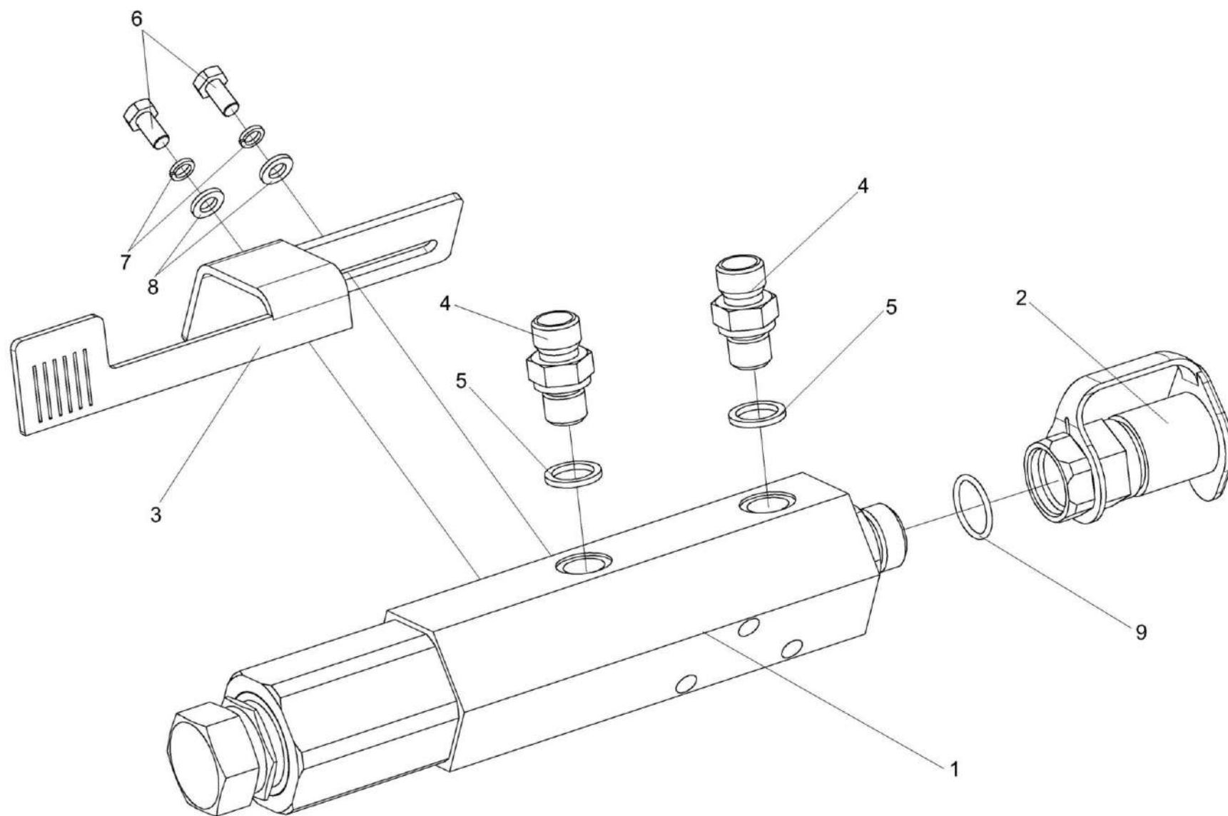
Рисунок 50 – Цилиндр КВС-1-0603110
