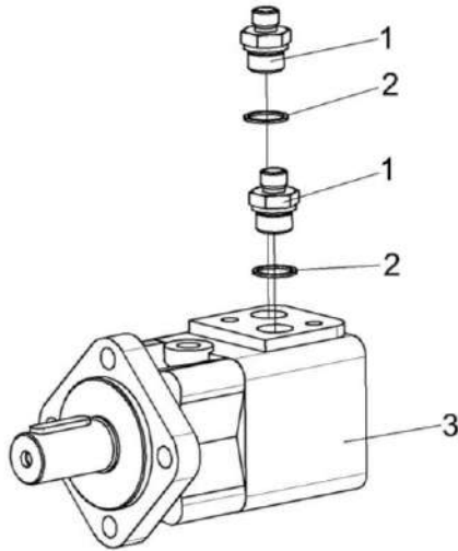
Рисунок 31 – Гидромотор заточного устройства КВС-1-0602650
