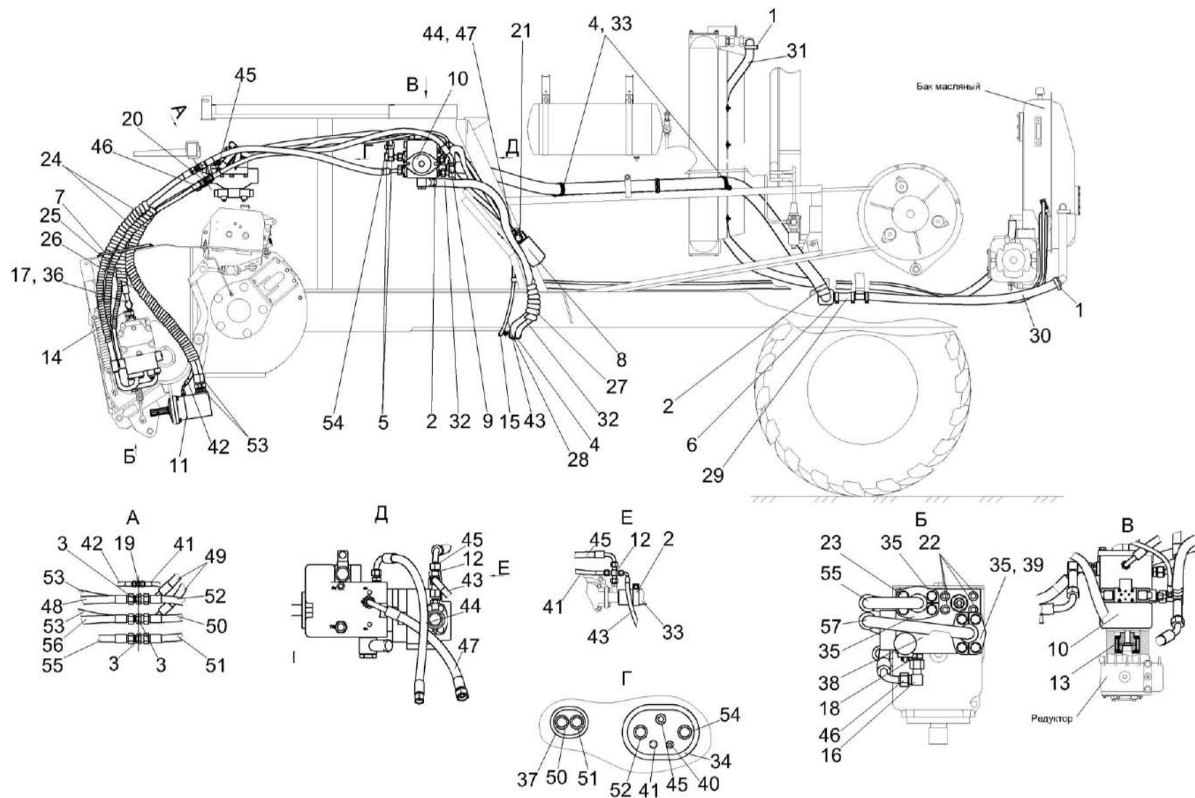
Рисунок 209 – Гидросистема привода питающего аппарата и адаптеров КВС-8-0624000 (вид слева)
