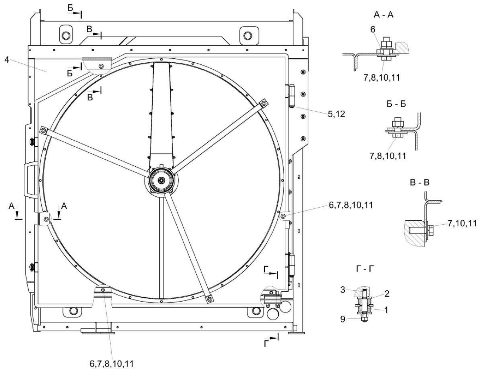
Рисунок 73 – Установка блока радиаторов КВС-8-0152000 (лист 2)
