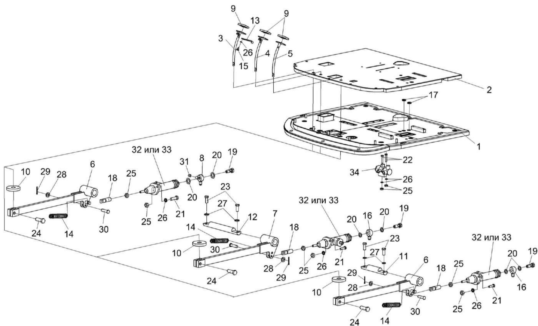
Рисунок 128 – Площадка управления КВС-8-0129000 (лист 2)
