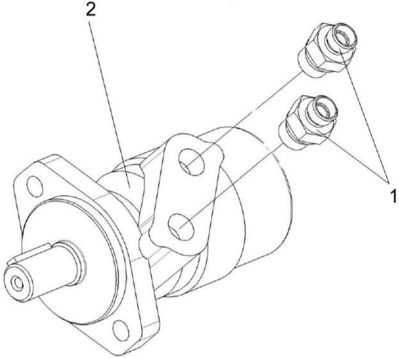
Рисунок 79 – Гидромотор воздухозаборника КВС-5-0602100
