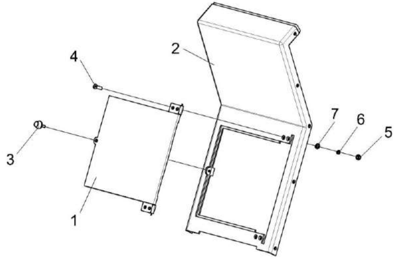
Рисунок 132 – Панель КВС-1-0129740
