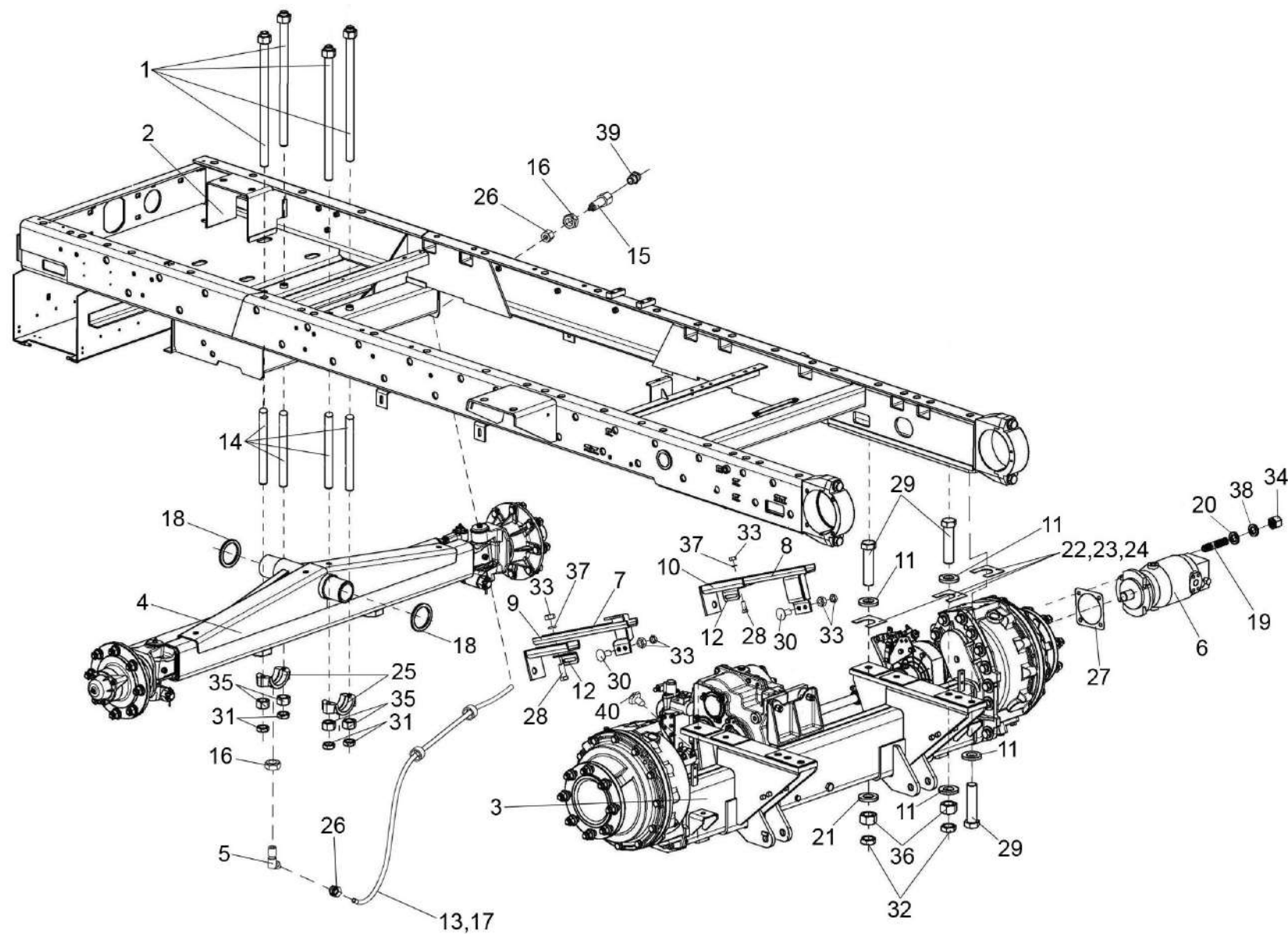
Рисунок 101 – Шасси КВС-8-0101000-01 (лист 2)
