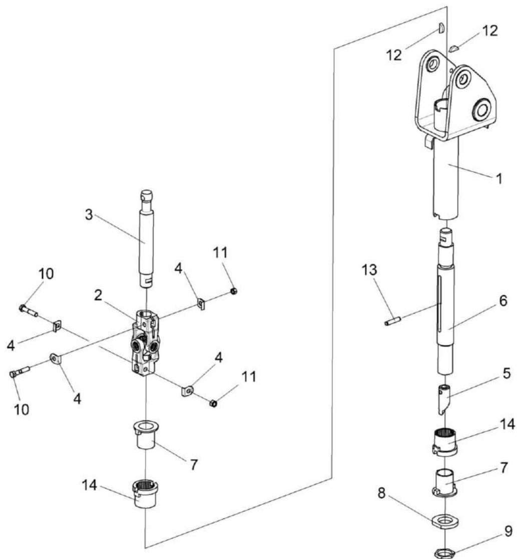
Рисунок 141 – Привод управления КЗС 0119600
