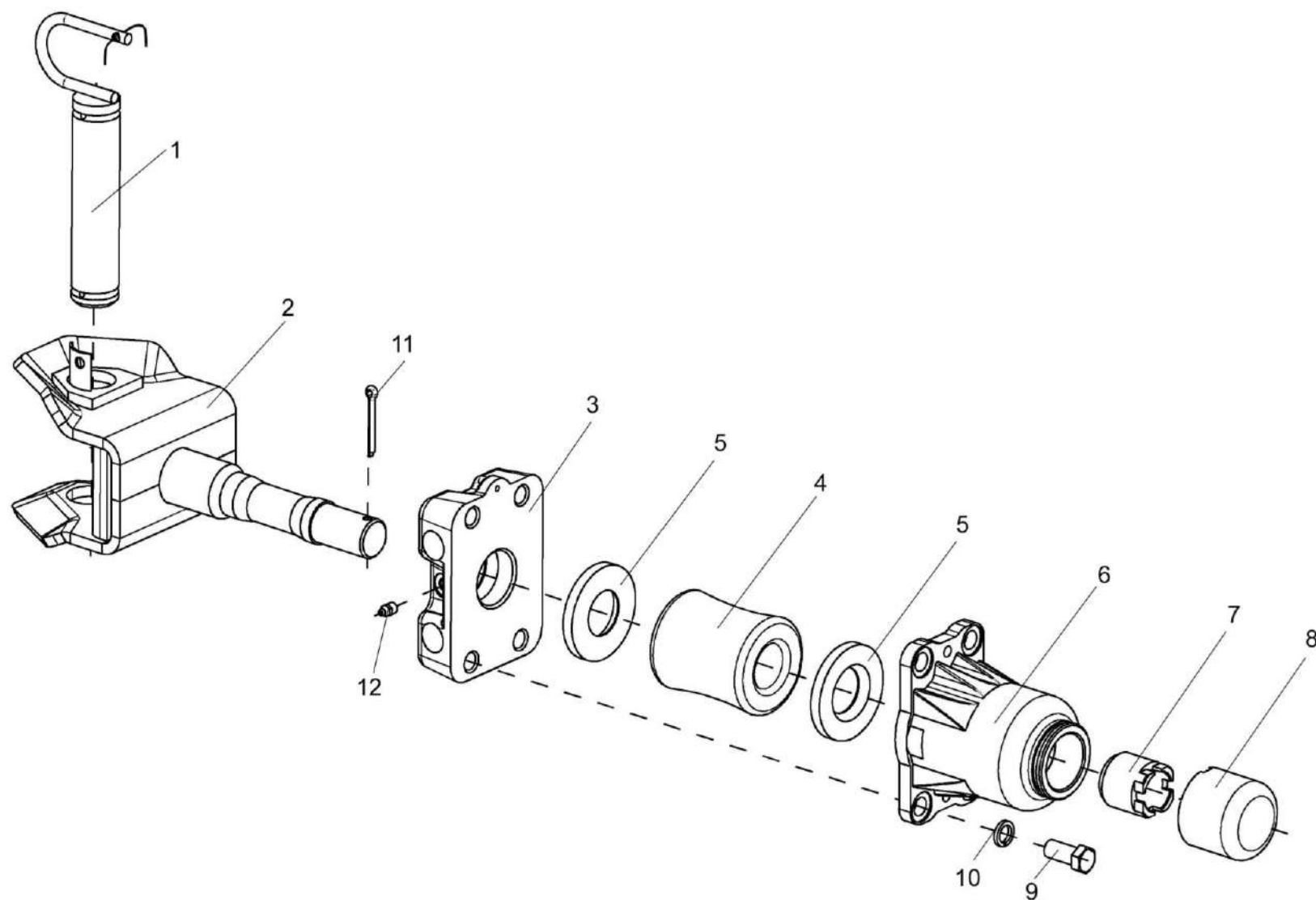
Рисунок 122 – Устройство тягово-сцепное УЭС 0003150
