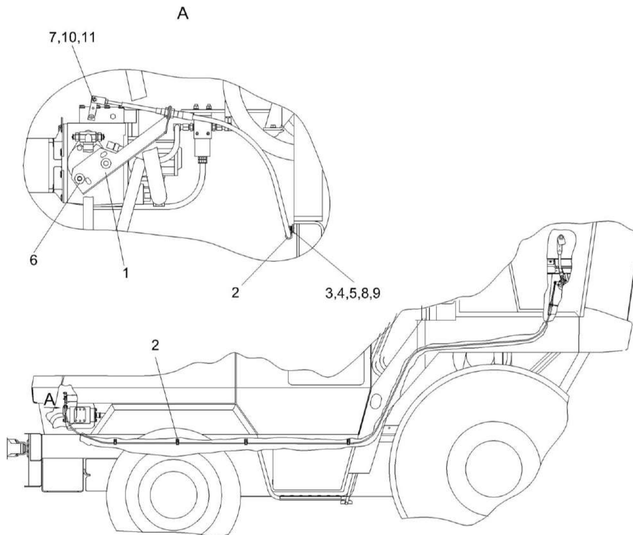
Рисунок 152 – Привод управления КВС-1-0129530А
