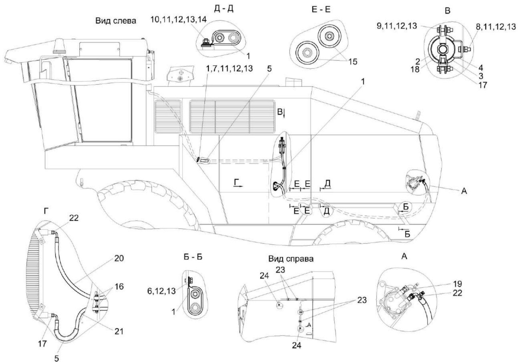
Рисунок 164 – Установка климатическая КВС-2-0121000Б-03
