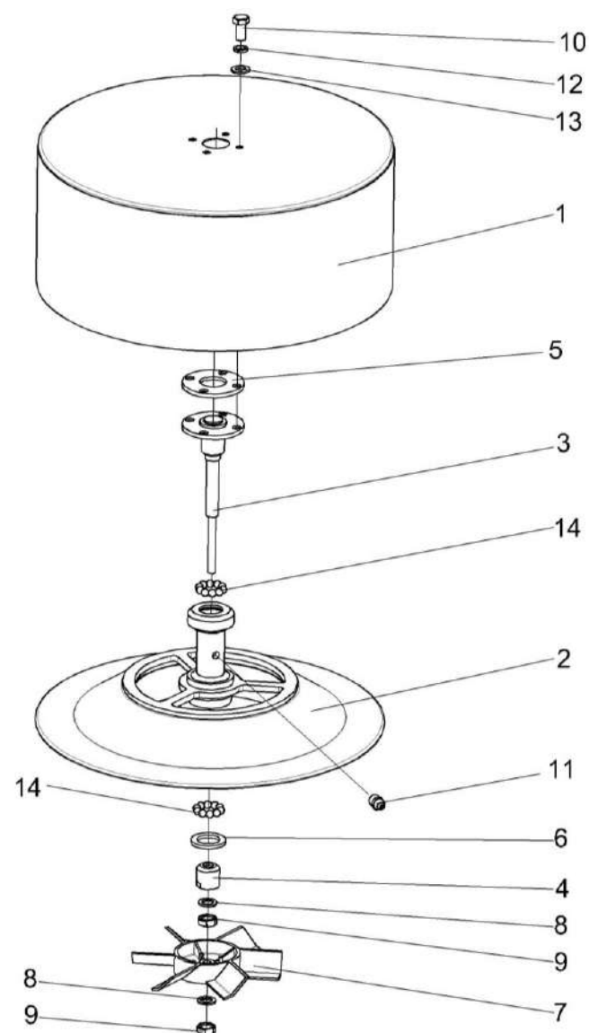
Рисунок 173 – Воздухозаборник вращающийся КВС-1-0153000А
