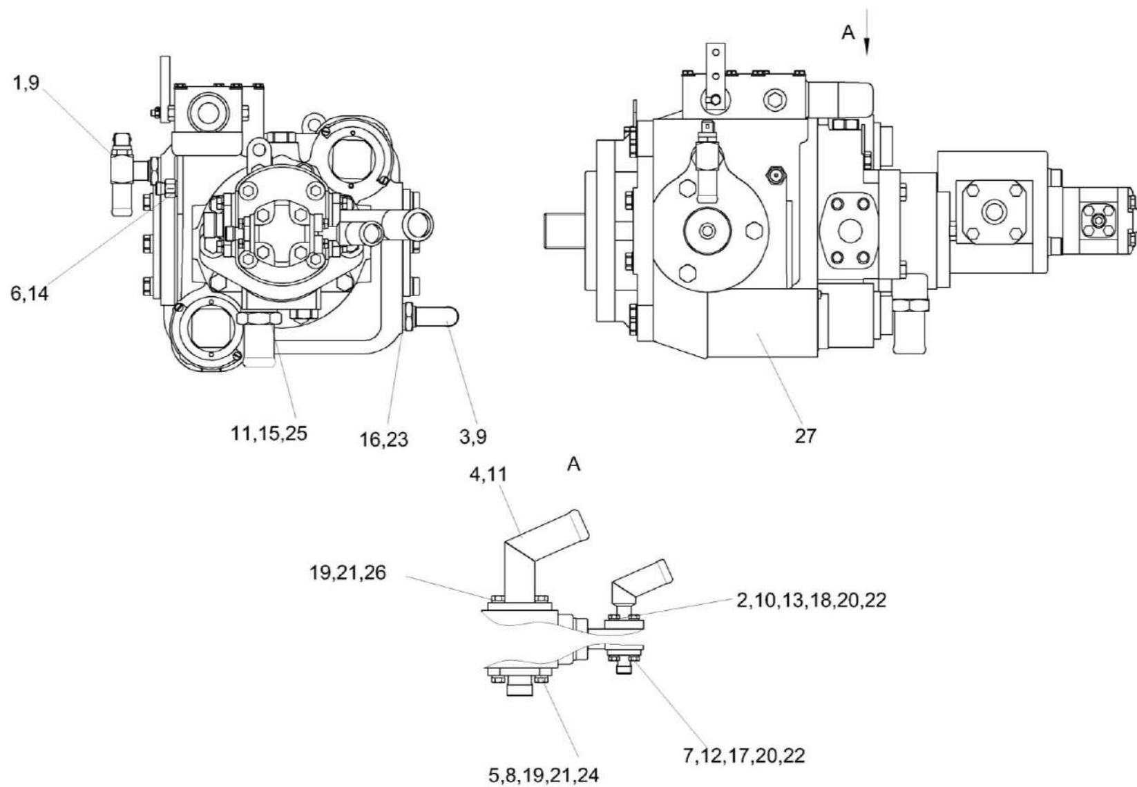
Рисунок 179 – Насос трехсекционный КВС-8-0600100
