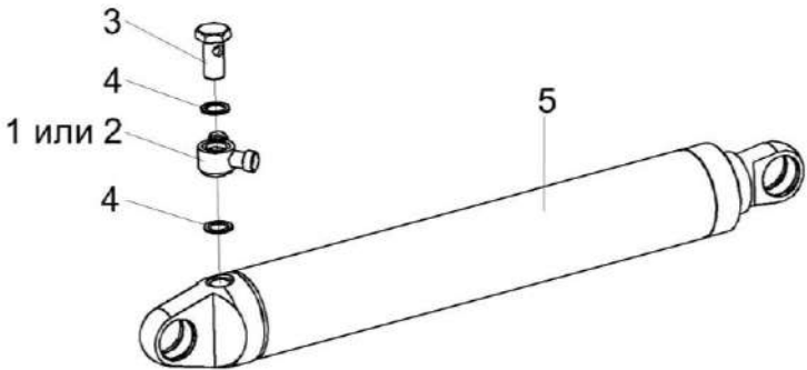
Рисунок 191 – Гидроцилиндр КВС-1-0602440 и КВС-1-0602440-01
