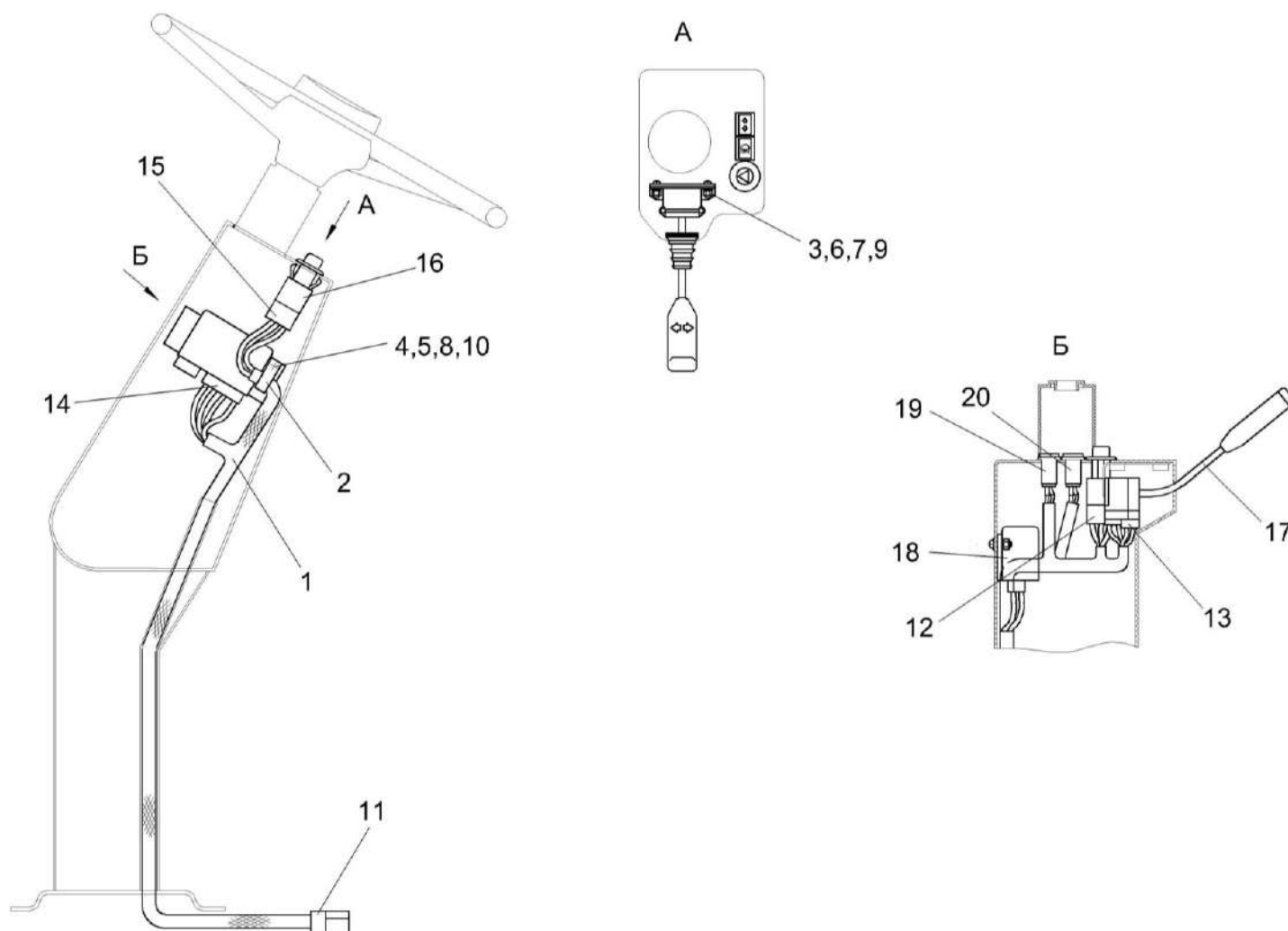
Рисунок 144 – Электрооборудование рулевой колонки КВС-1-0129230-03
