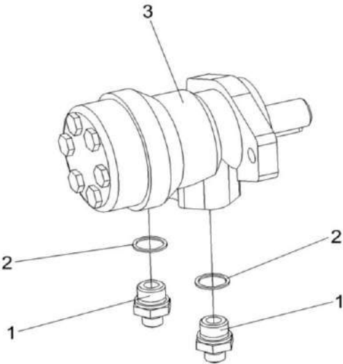
Рисунок 61 – Гидромотор силосопровода КВС-1-0602970
