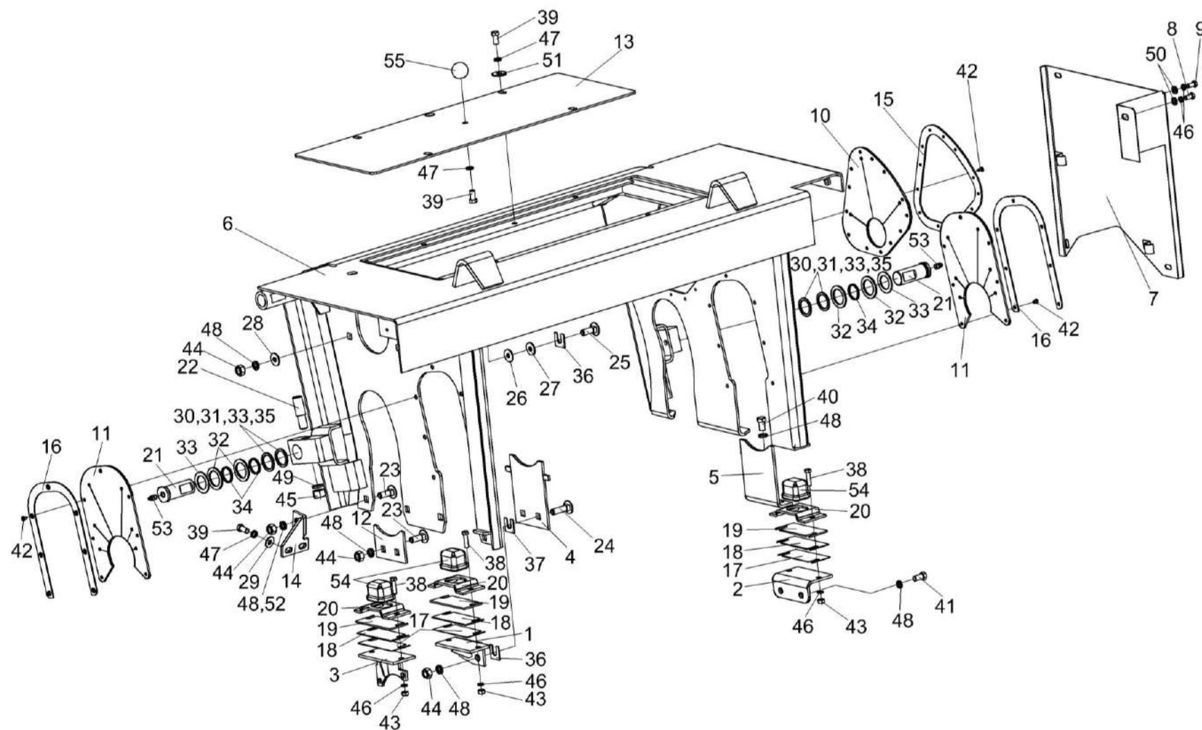
Рисунок 5 – Установка рамы верхней КВС-2-0111300В
