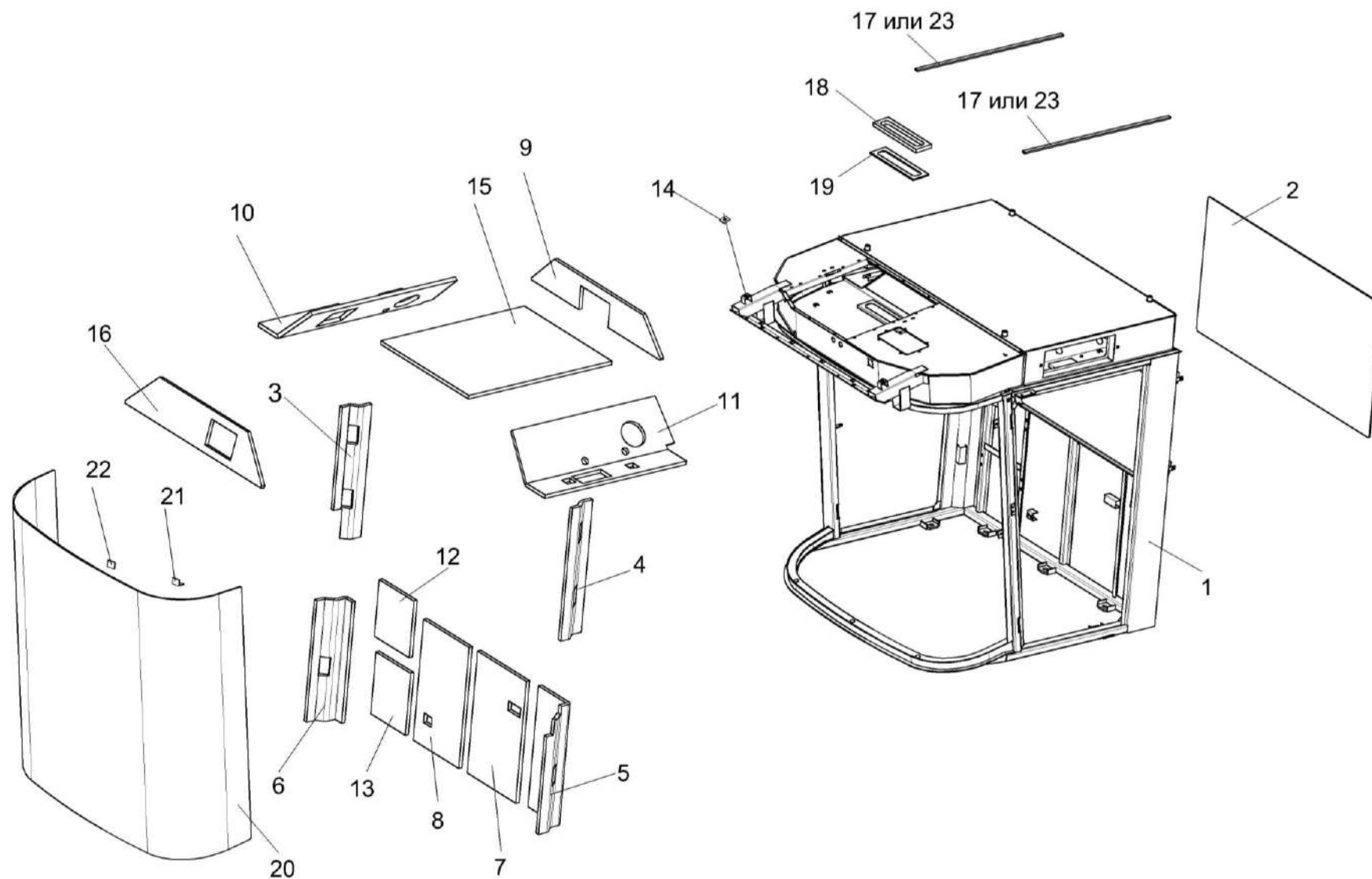
Рисунок 158 – Каркас КВС-8-0120020
