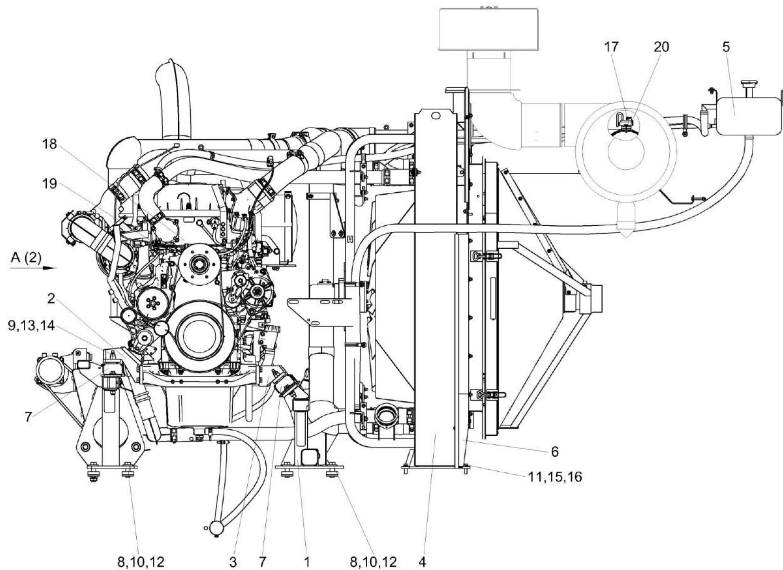
Рисунок 65 – Установка двигателя КВС-8-0150000 (лист 1)
