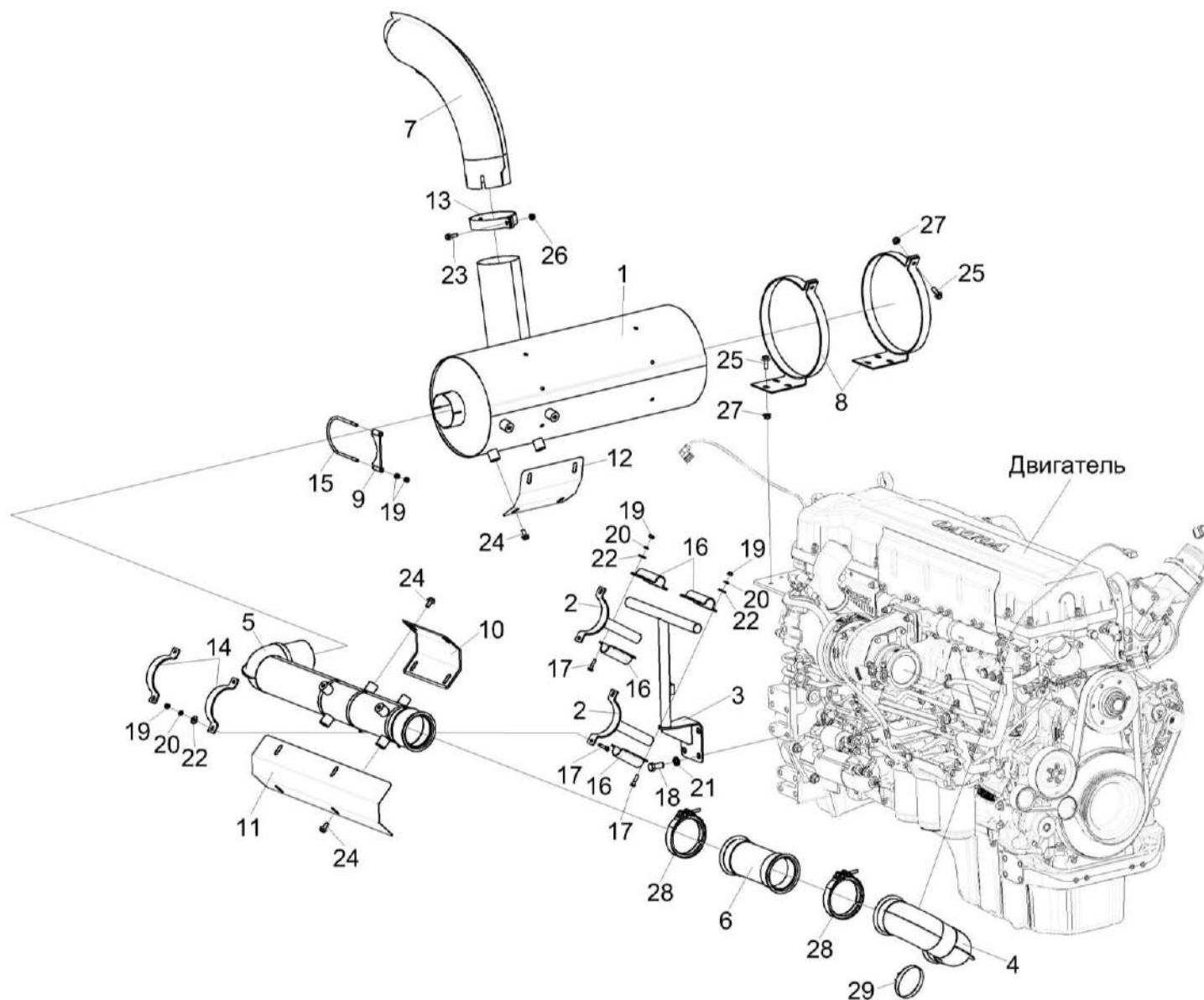
Рисунок 82 – Установка глушителя КВС-8-0157000
