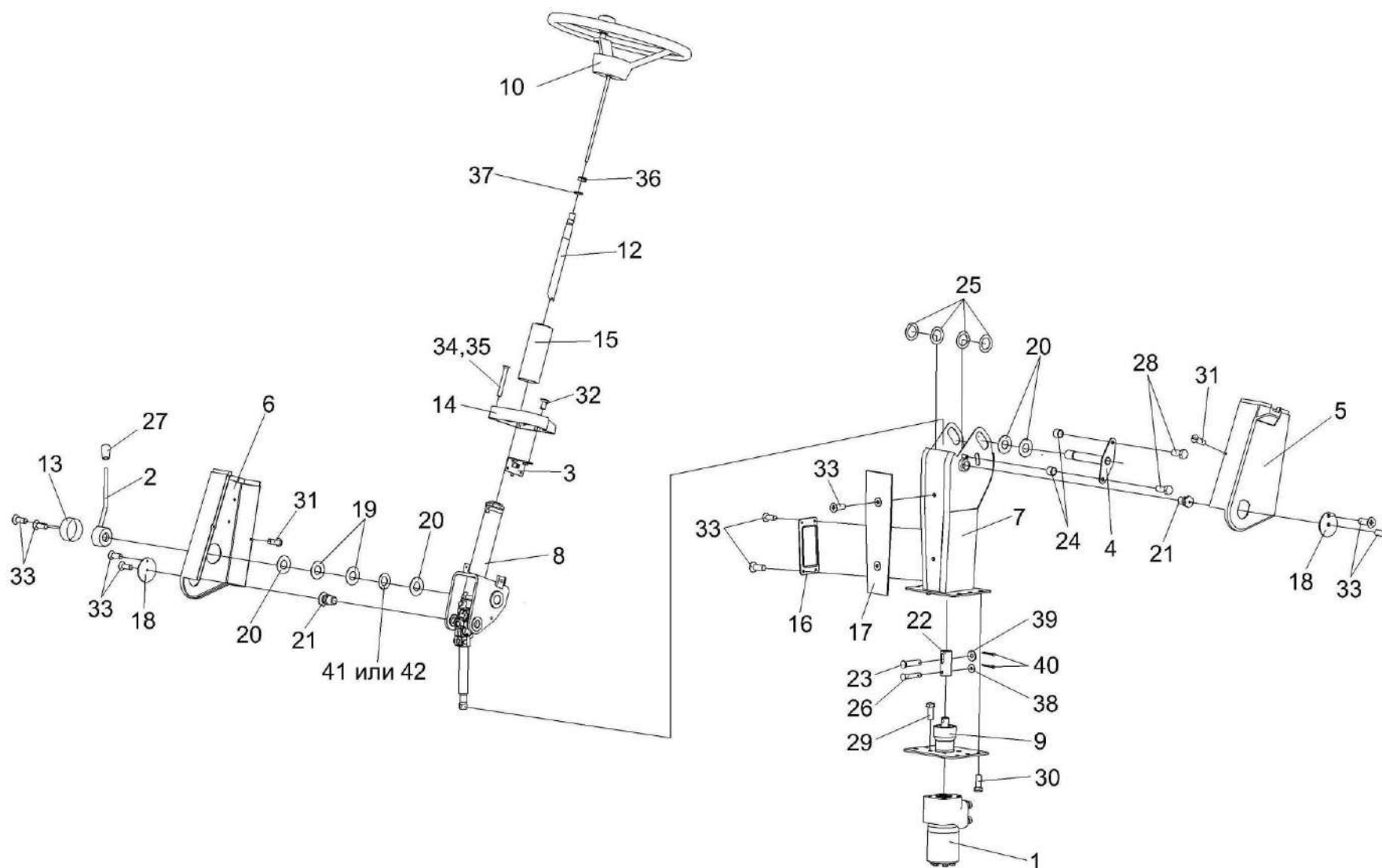
Рисунок 139 – Рулевая колонка КВС-1-0129230-03
