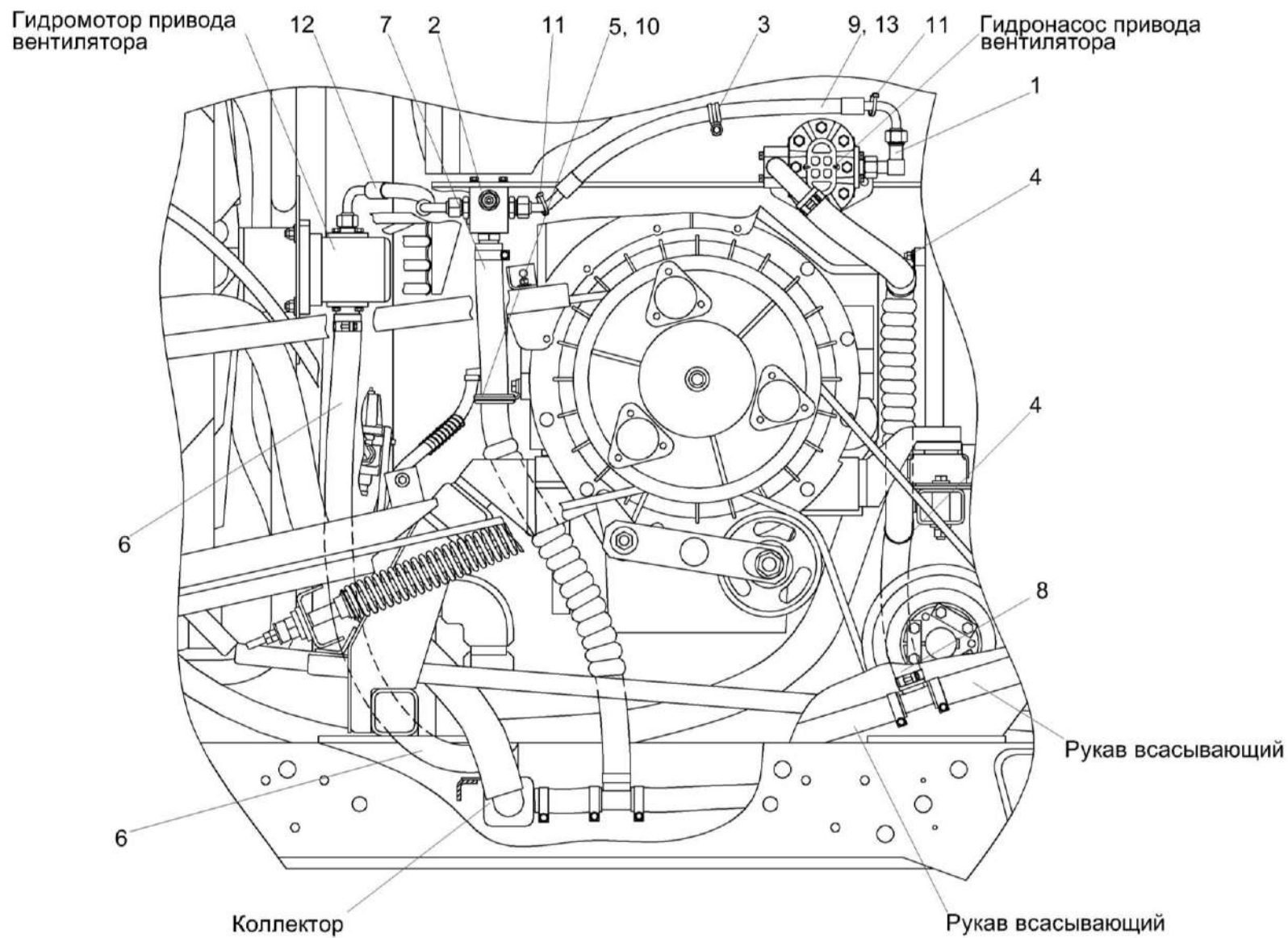
Рисунок 215 – Гидросистема привода рабочих органов КВС-8-0608000 (лист 1)
