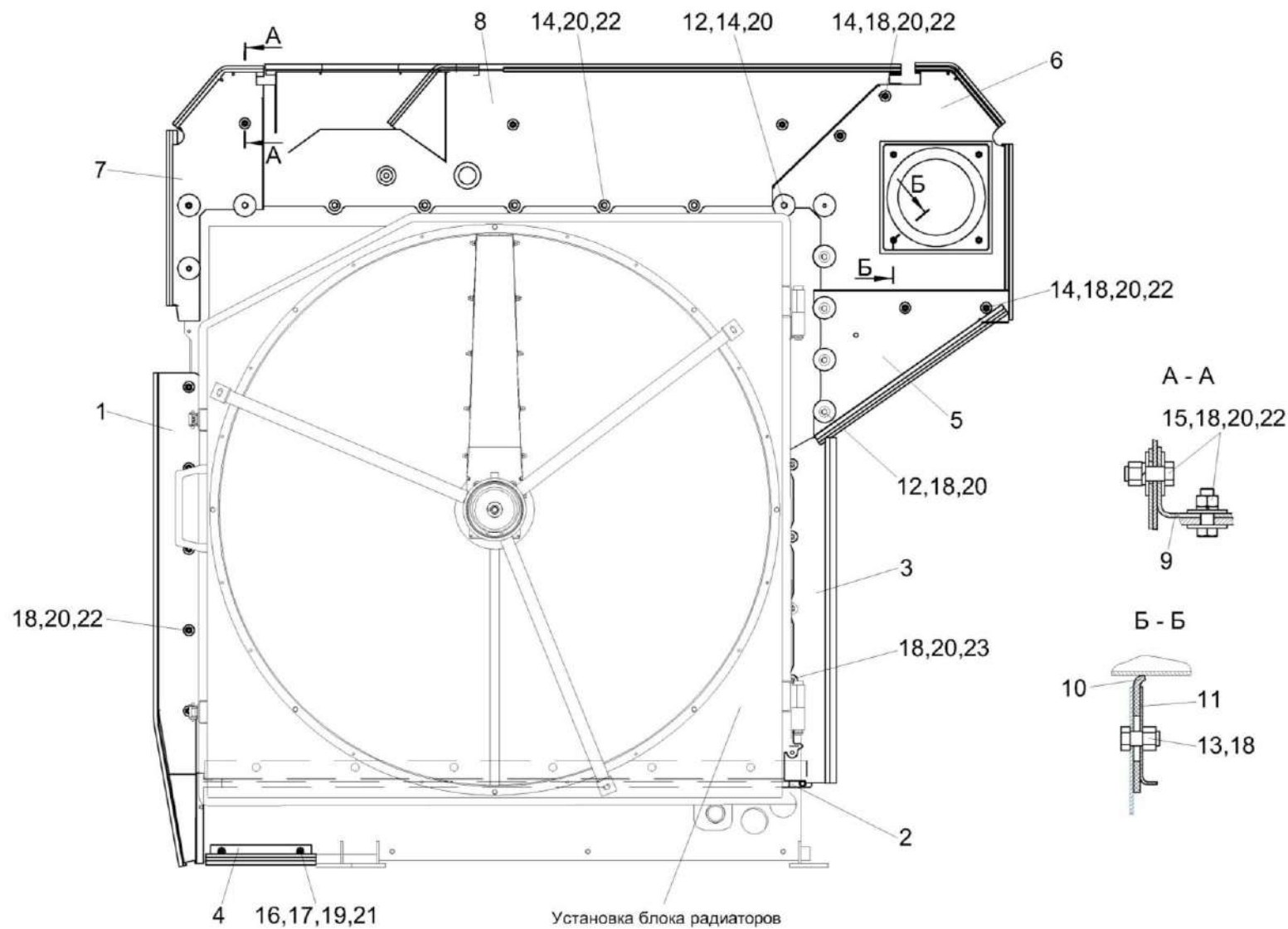
Рисунок 81 – Установка щитов КВС-8-0156000
