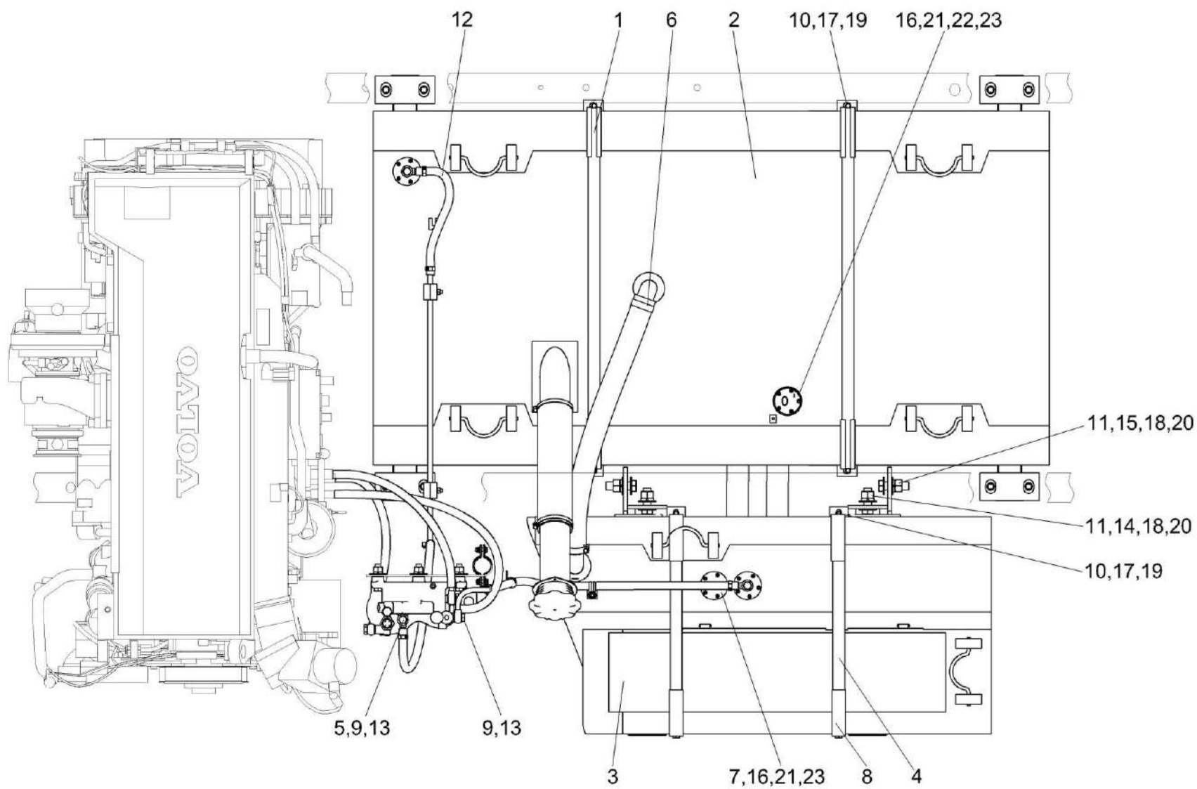
Рисунок 98 – Установка топливного оборудования КВС-8-0103000 (лист 2)
