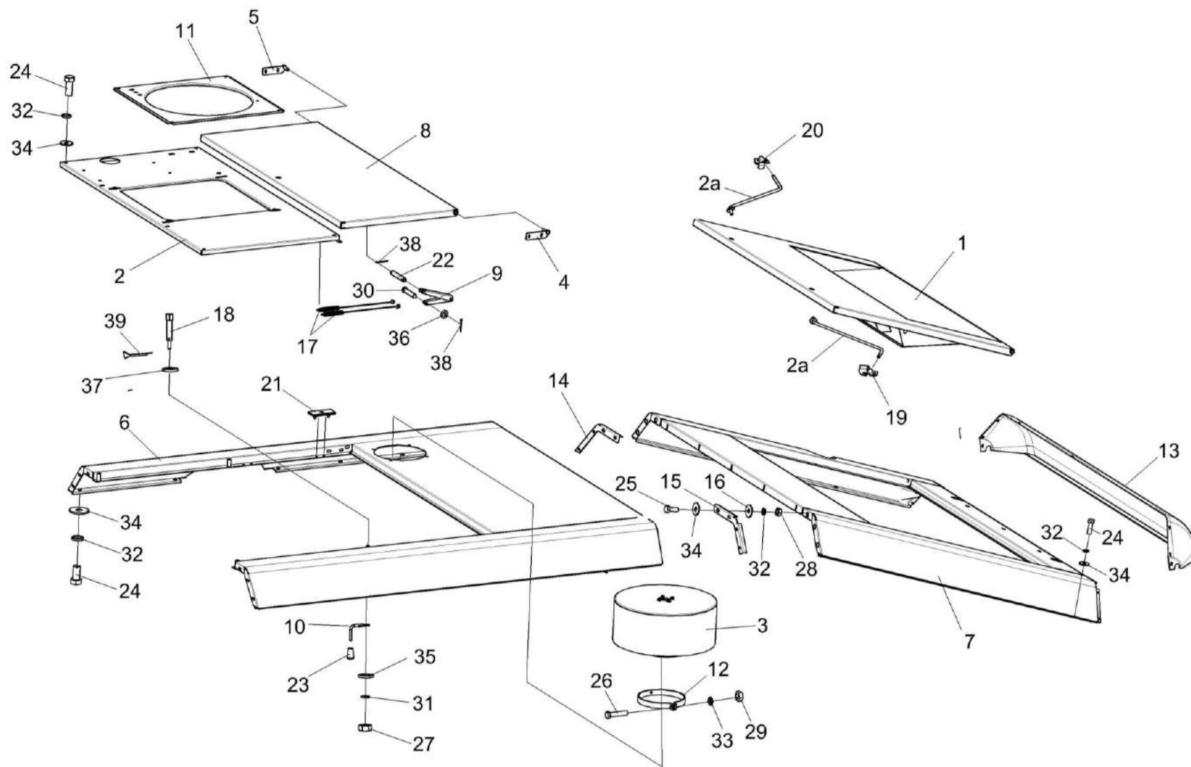
Рисунок 169 – Капот верхний КВС-8-0162000 (лист 1)
