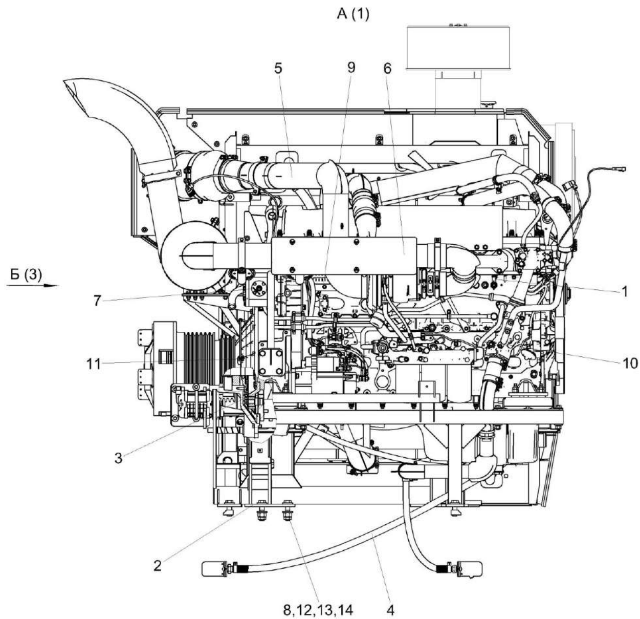
Рисунок 66 – Установка двигателя КВС-8-0150000 (лист 2)
