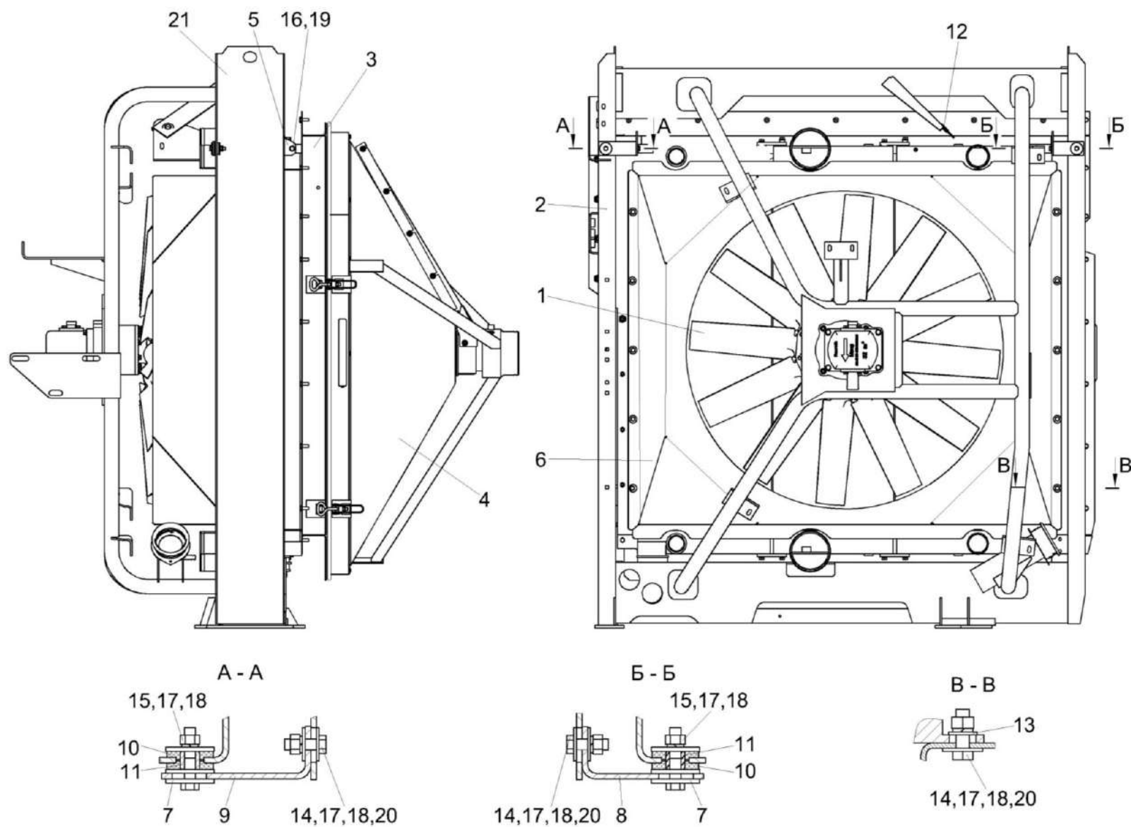
Рисунок 72 – Установка блока радиаторов КВС-8-0152000 (лист 1)
