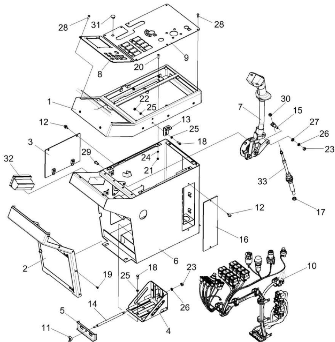
Рисунок 130 – Пульт управления КВС-8-0129050
