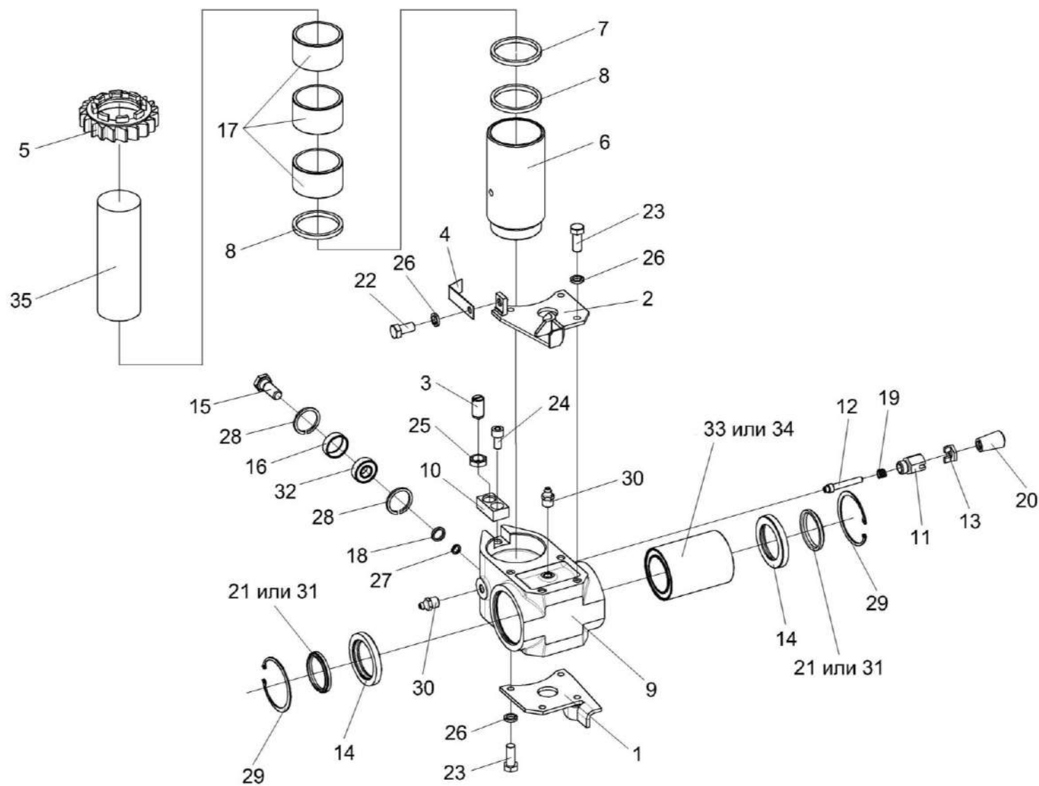
Рисунок 28 – Установка каретки КВС-2-0116510
