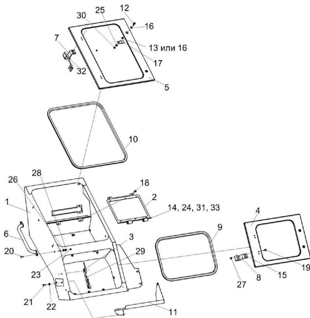
Рисунок 226 – Электрошкаф КВС-8-0702010
