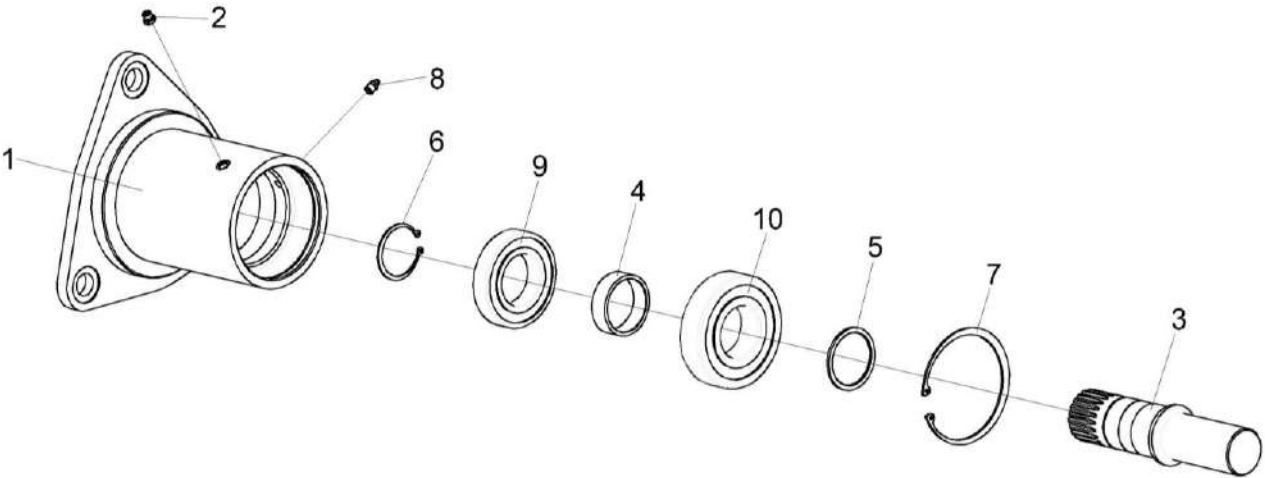
Рисунок 94 – Опора КВС-8-0133420
