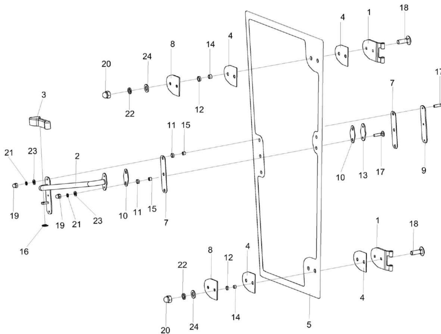
Рисунок 160 – Дверь КЗК-12-0120900-01
