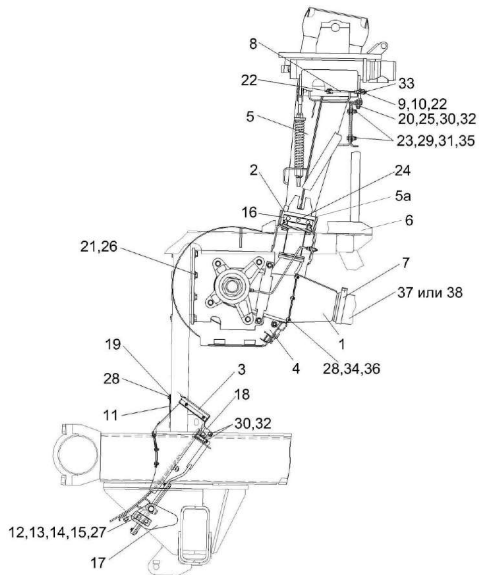
Рисунок 53 – Установка ускорителя выброса, камеры приемной и основания силосопровода КВС-1-0140000
