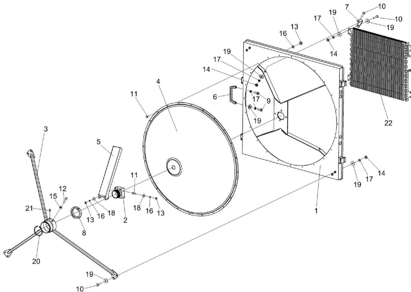
Рисунок 77 – Воздухозаборник КВС-5-0155000 (лист 1)
