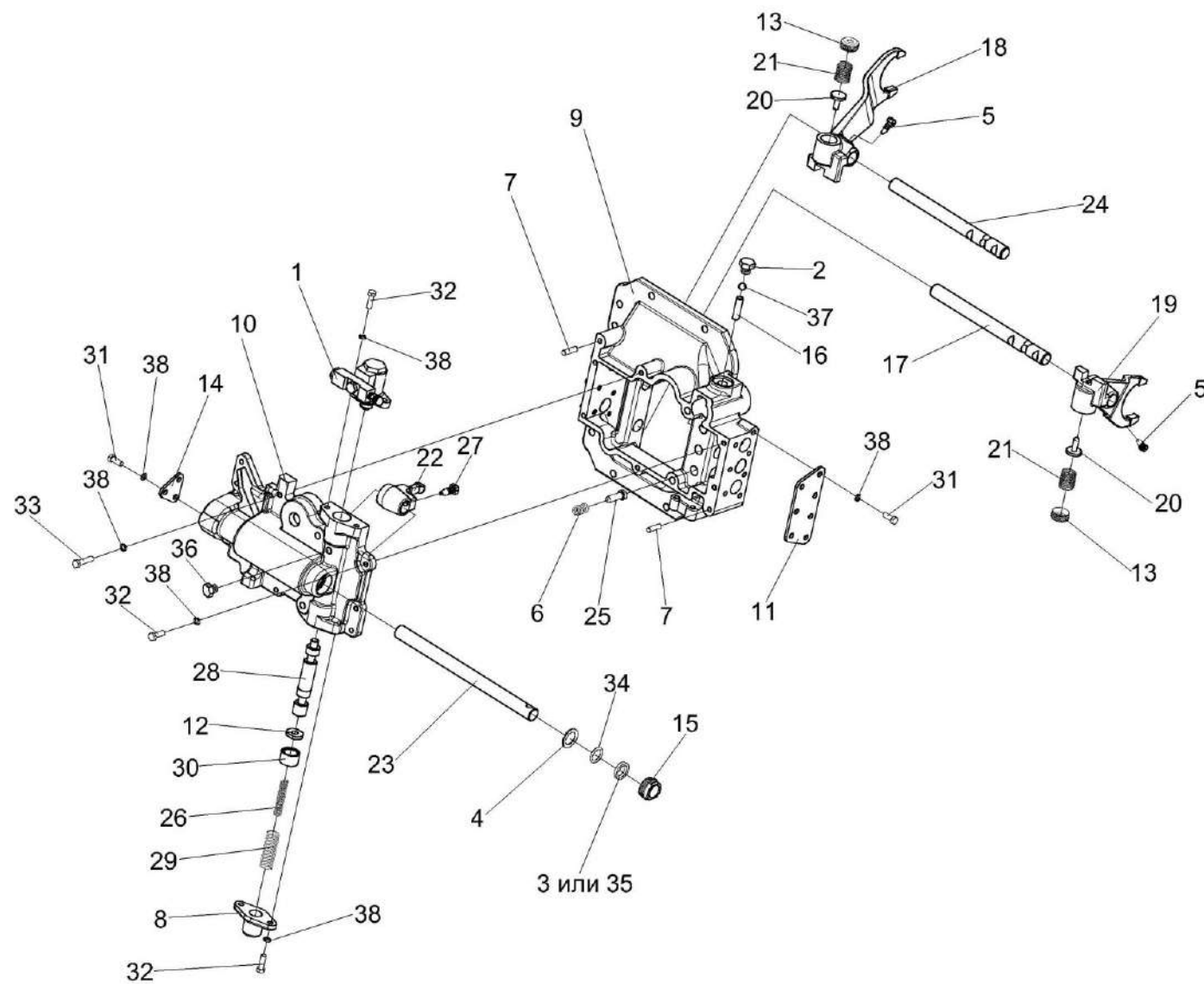
Рисунок 116 – Механизм переключения диапазонов 3518020-46160
