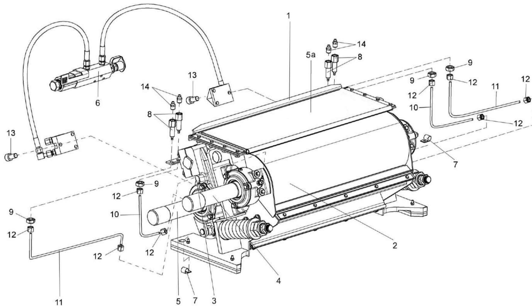
Рисунок 42 – Устройство доизмельчающее КВС-2-0148010
