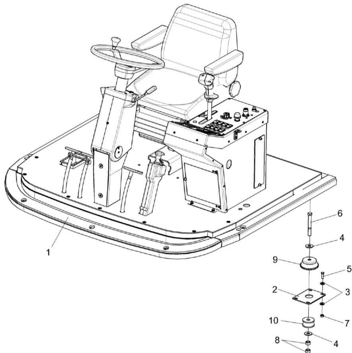
Рисунок 126 – Установка площадки управления КВС-8-0129200
