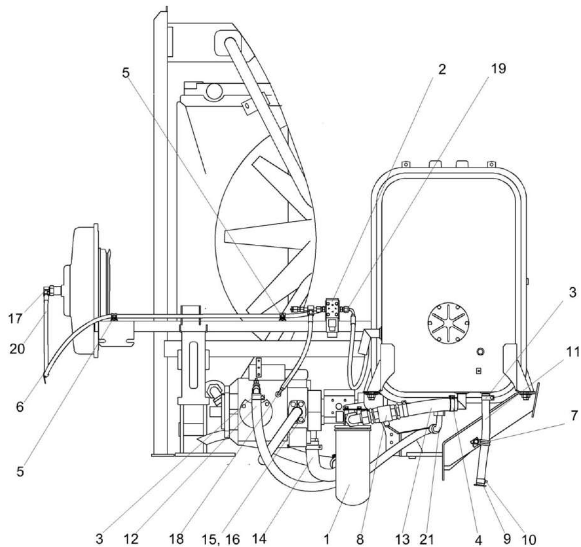
Рисунок 182 – Гидросистема привода ходовой части КВС-8-0601000(вид сзади)
