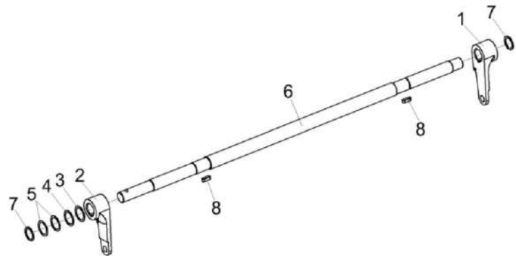
Рисунок 33 – Привод КВС-1-0115140Б
