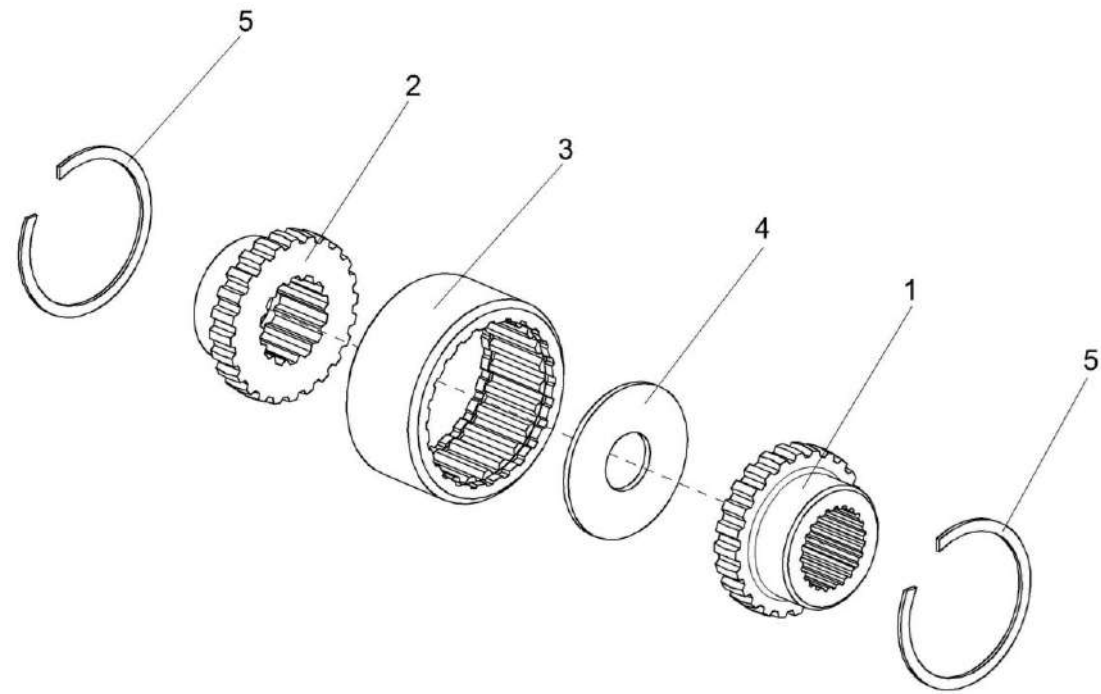
Рисунок 18 – Муфта КГС 0100120
