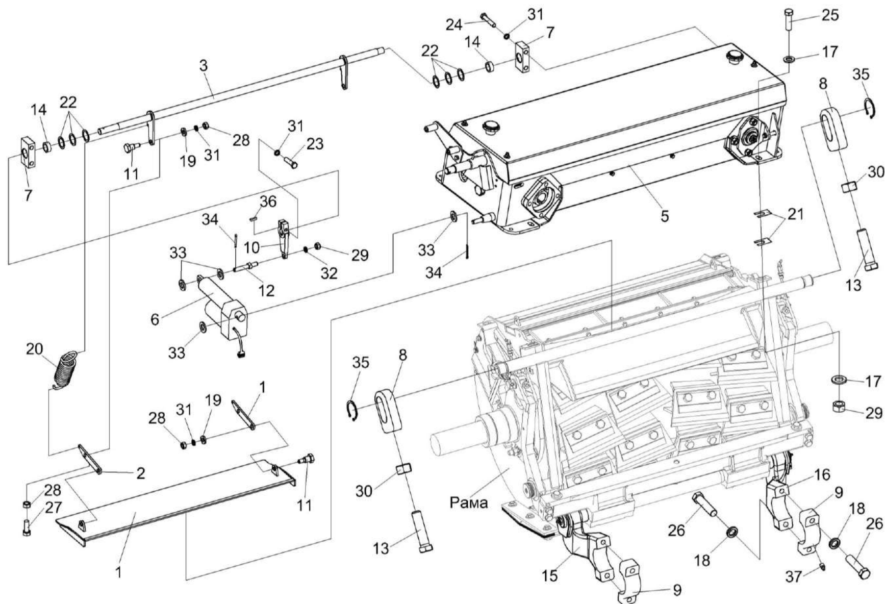
Рисунок 23 – Аппарат измельчающий КВС-8-0115000
