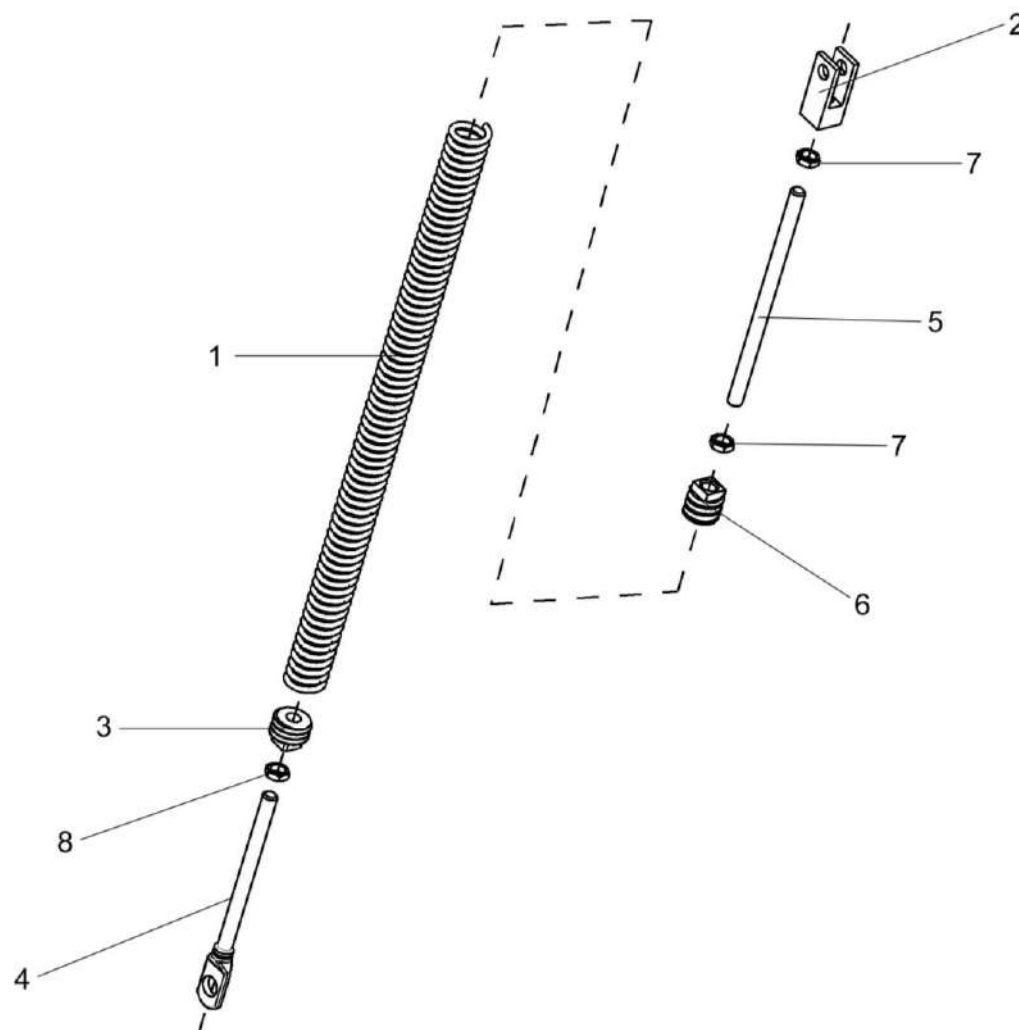
Рисунок 41 – Пружина КВС-1-0132090
