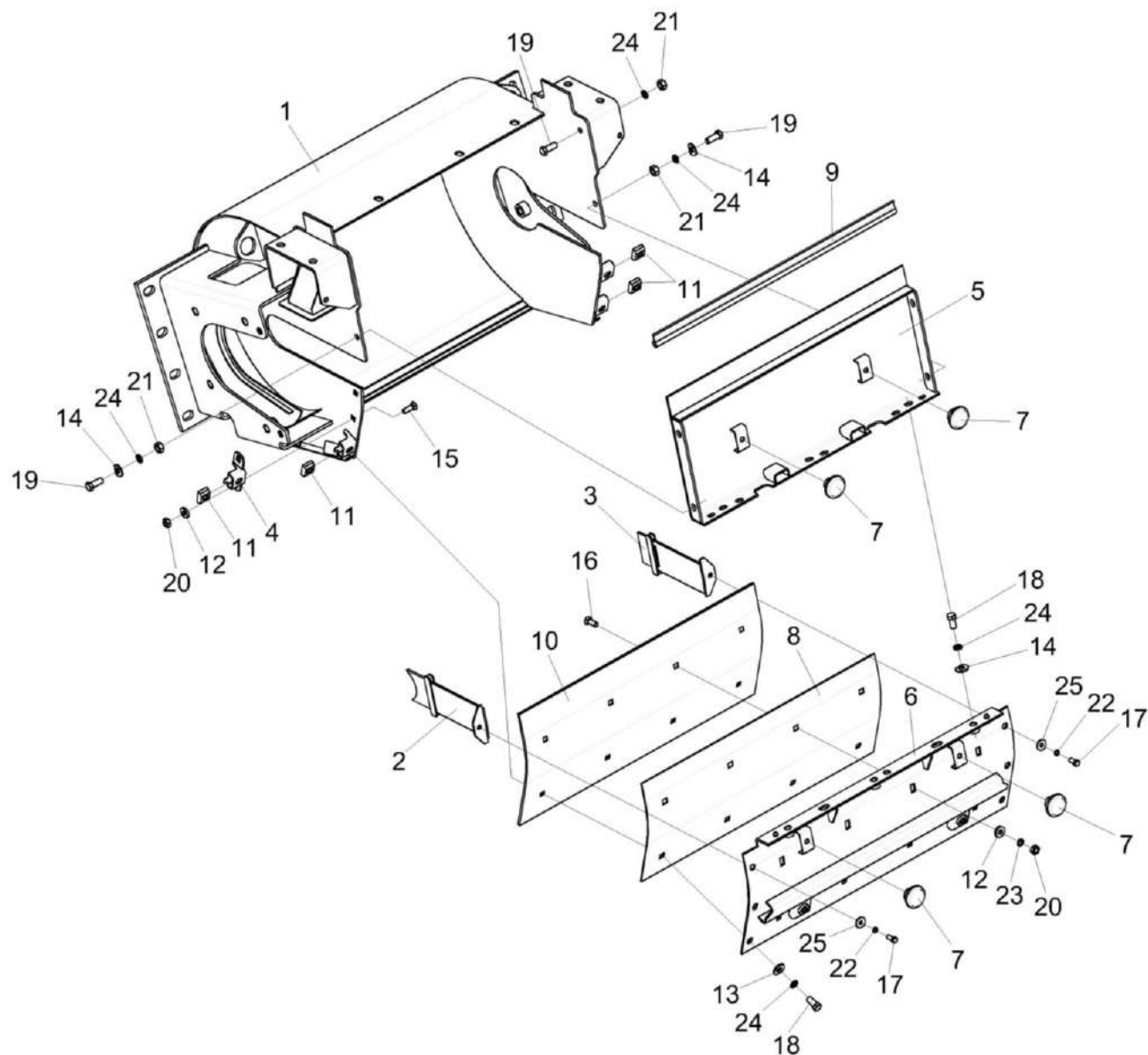
Рисунок 55 – Ускоритель выброса КВС-2-0142000 (лист 1)
