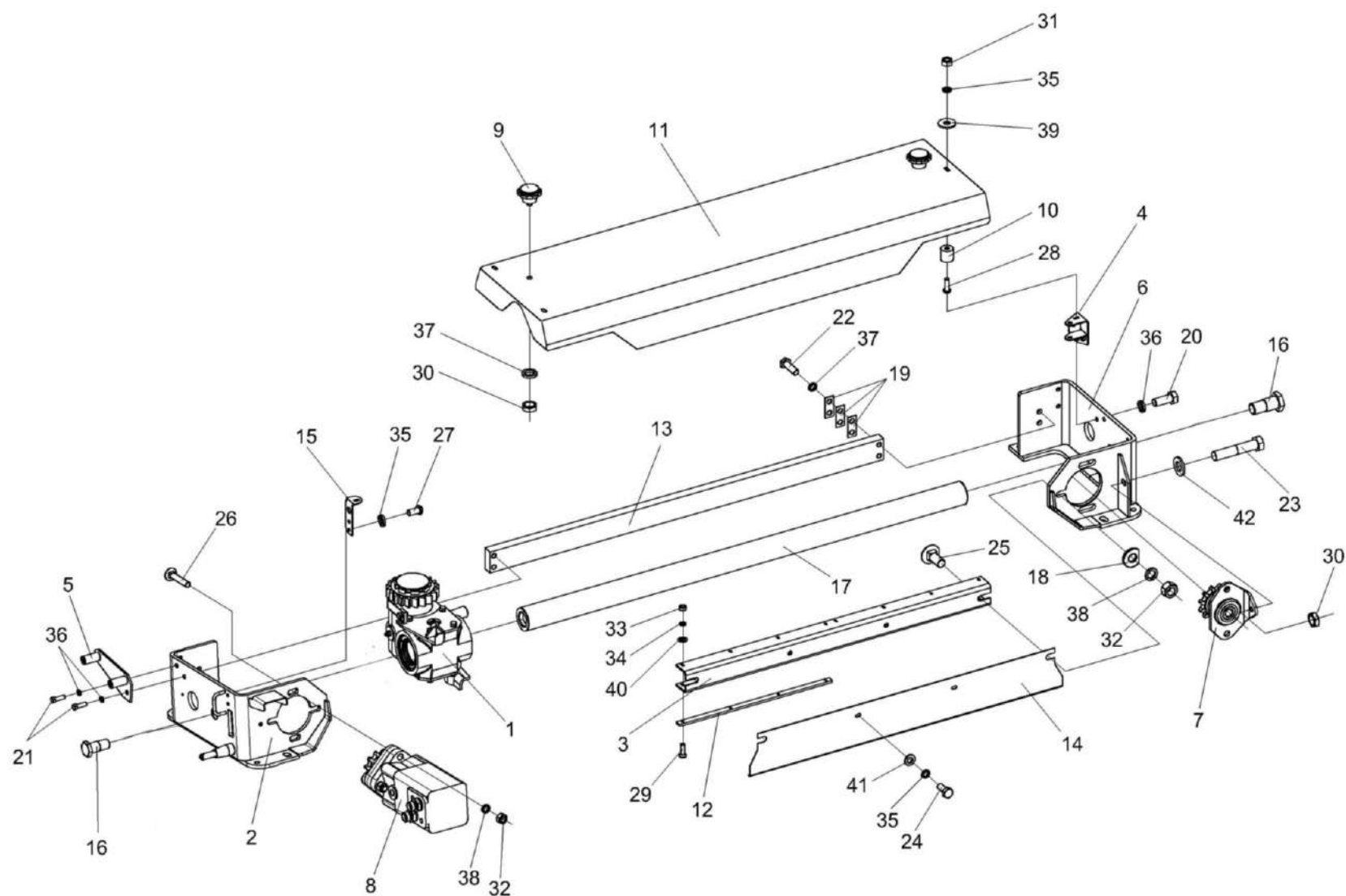
Рисунок 27 – Устройство заточное КВС-2-0116500
