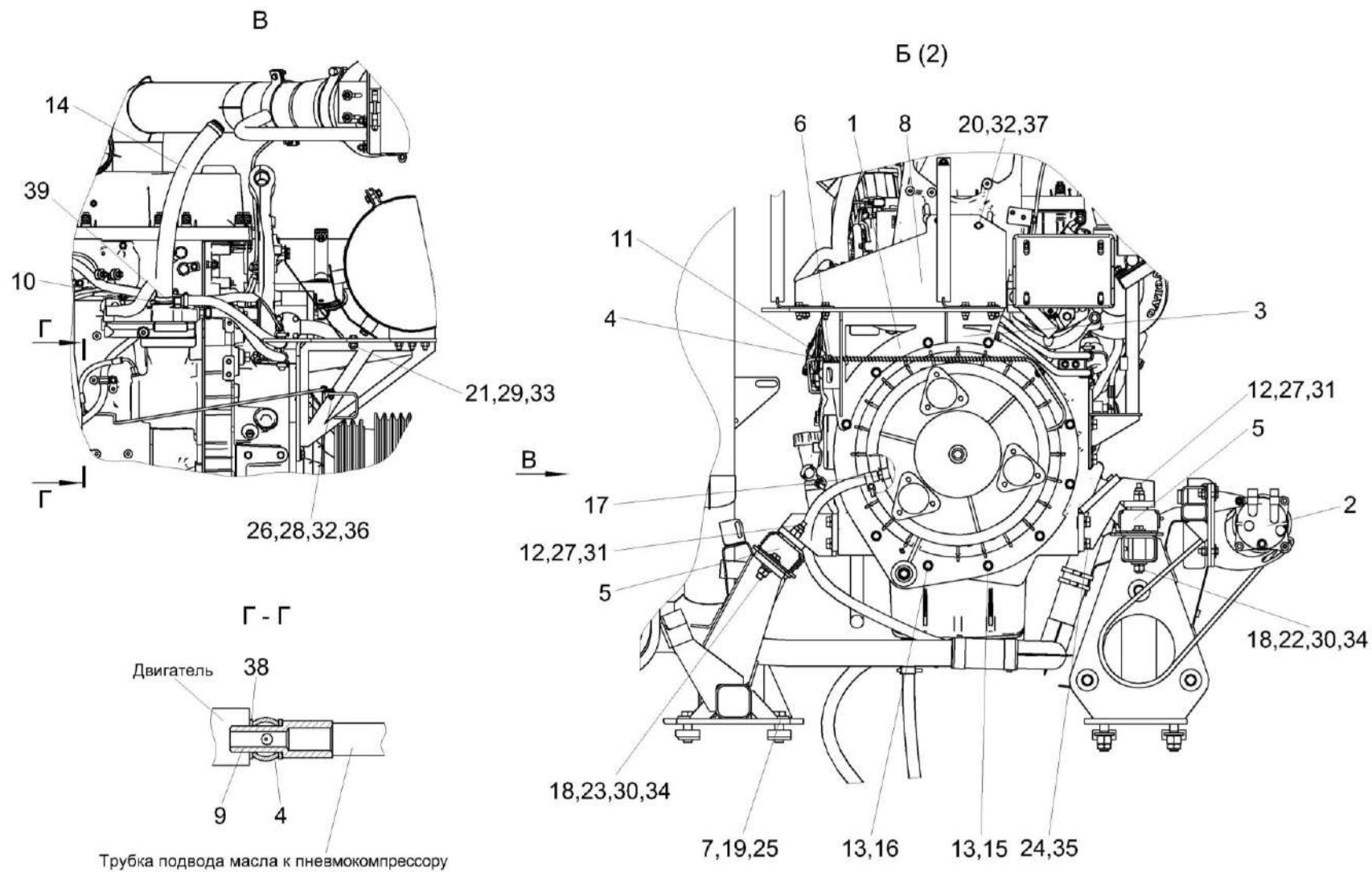
Рисунок 67 – Установка двигателя КВС-8-0150000 (лист 3)
