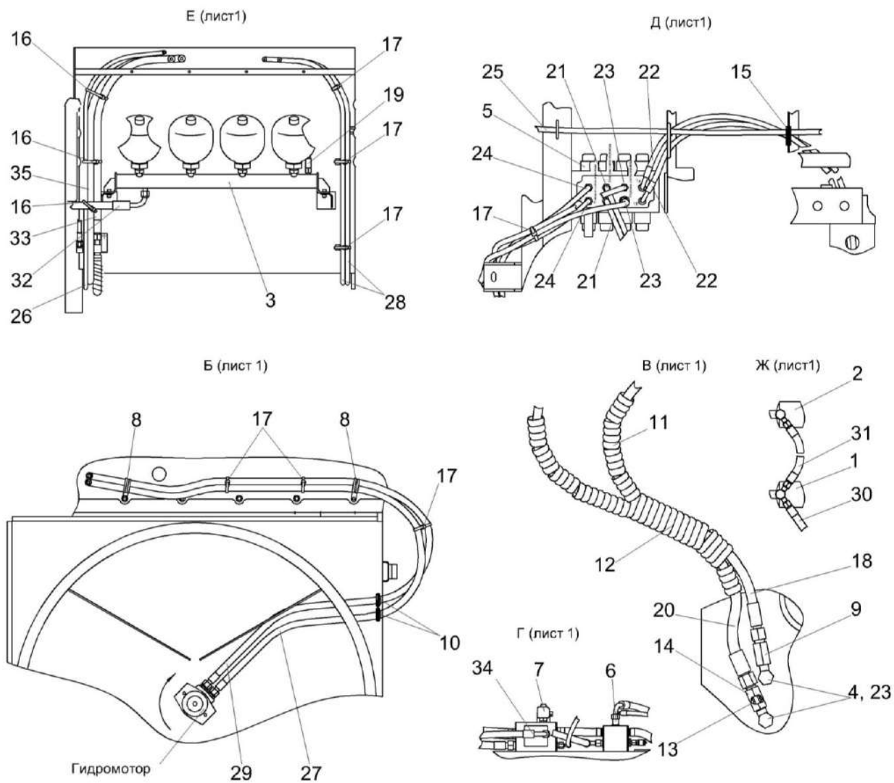
Рисунок 186 – Гидросистема рабочих органов и рулевого управления КВС-8-0602000(лист 2)
