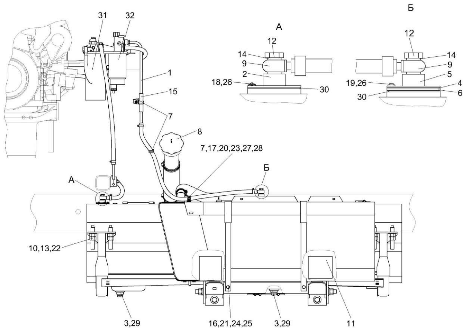
Рисунок 97 – Установка топливного оборудования КВС-8-0103000 (лист 1)
