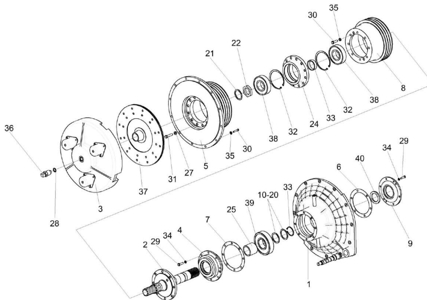
Рисунок 87 – Главный привод КВС-2-0151000Г
