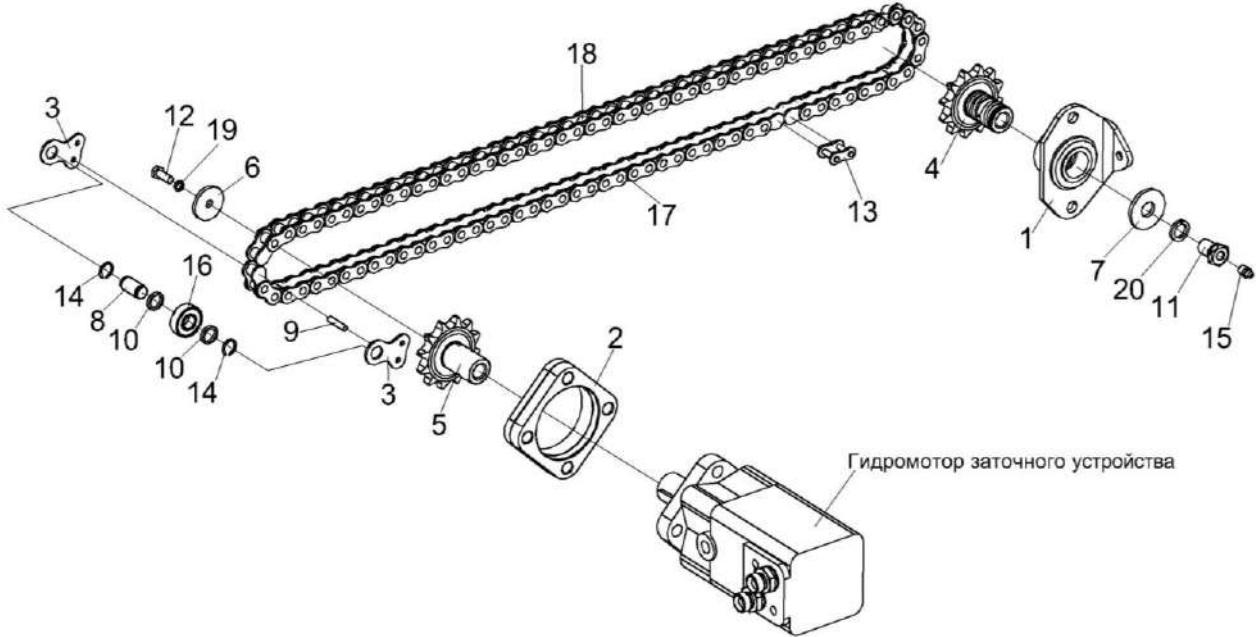
Рисунок 29 – Привод каретки КВС-2-0116510
