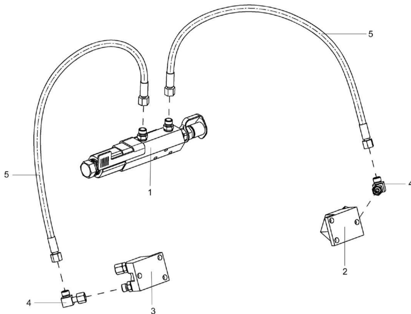
Рисунок 49 – Гидросистема регулировки зазора КВС-1-0603000
