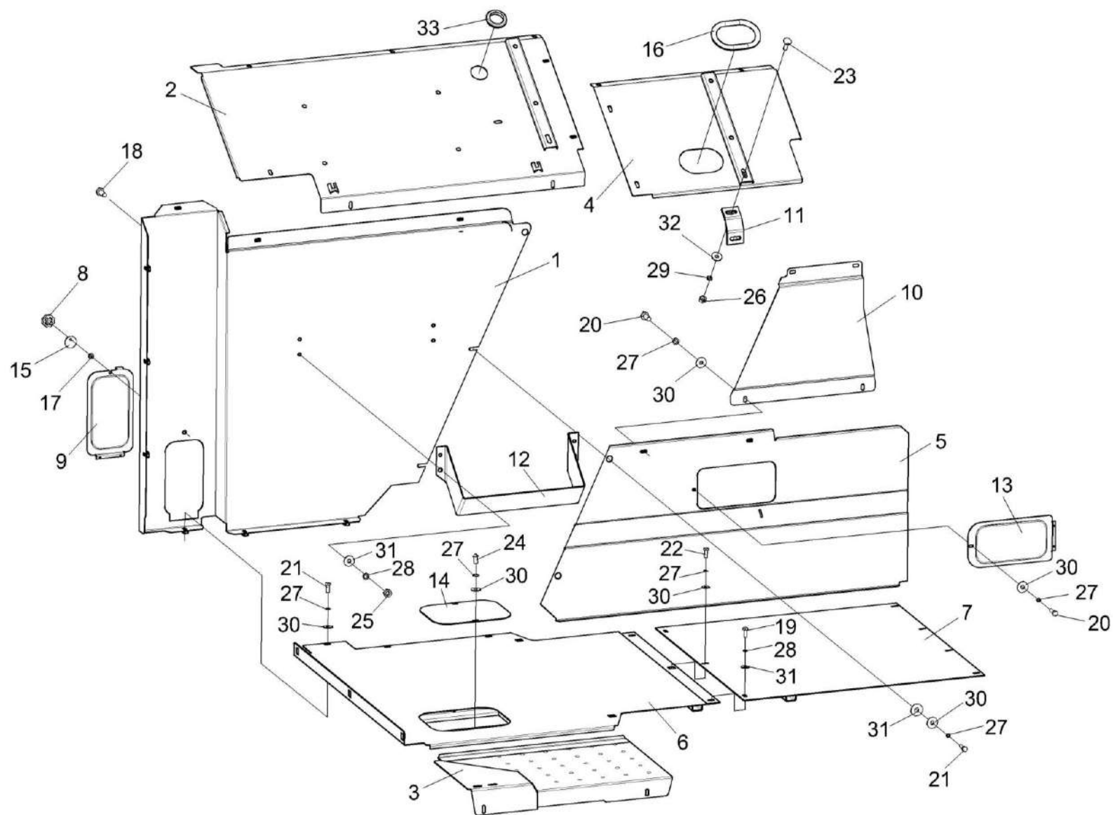
Рисунок 174 – Установка настилов и ограждений КВС-8-0169000
