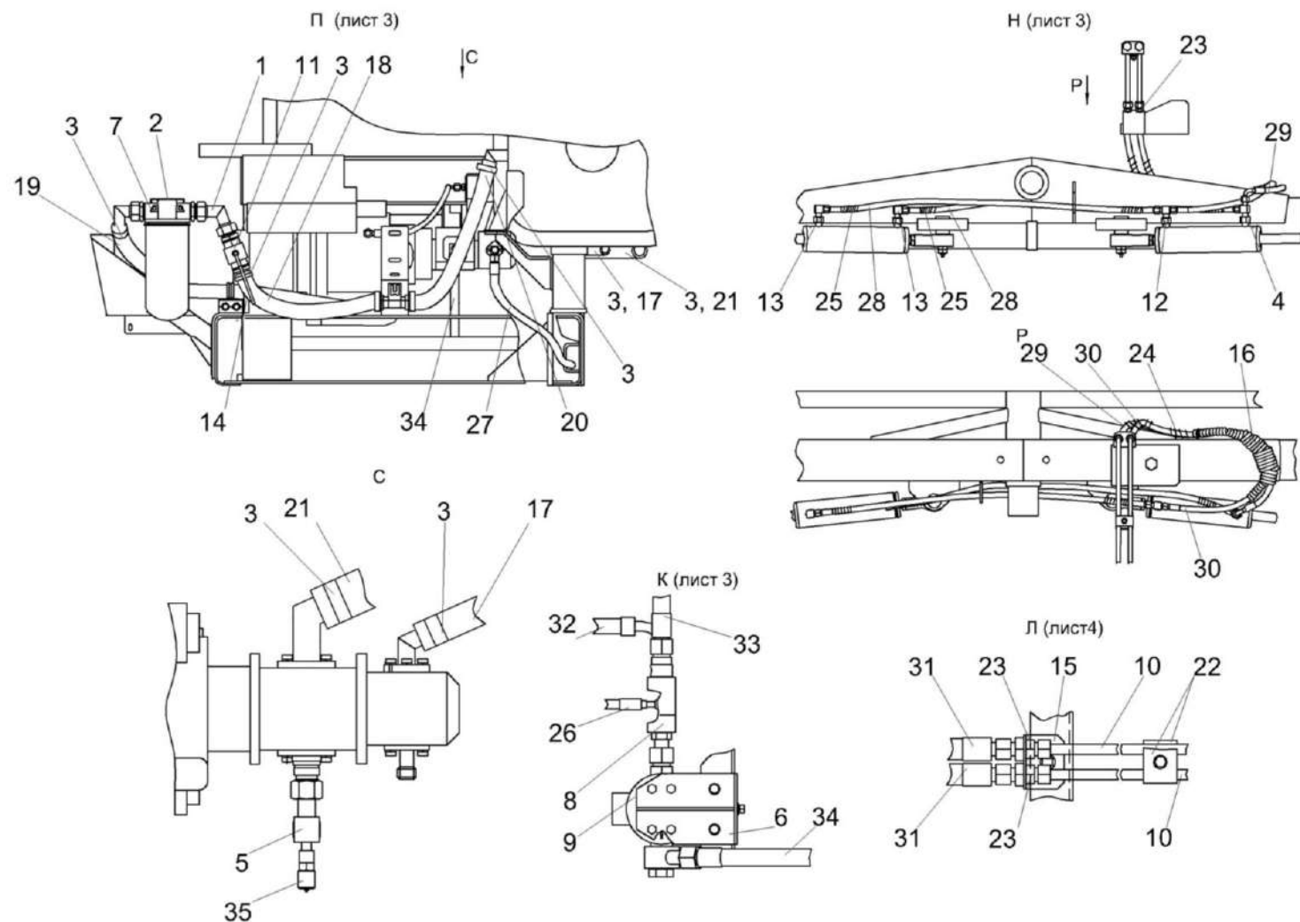
Рисунок 188 – Гидросистема рабочих органов и рулевого управления КВС-8-0602000(лист 4)
