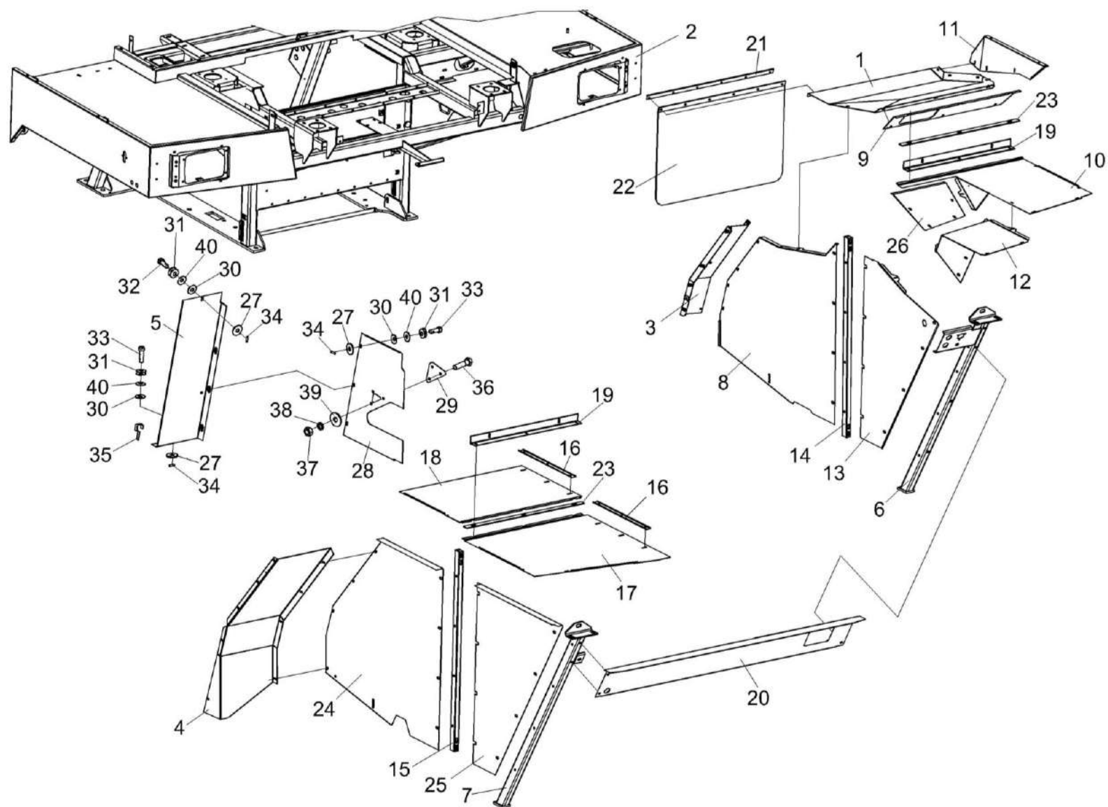
Рисунок 154 – Установка площадки входа КВС-8-0124000 (лист 2)
