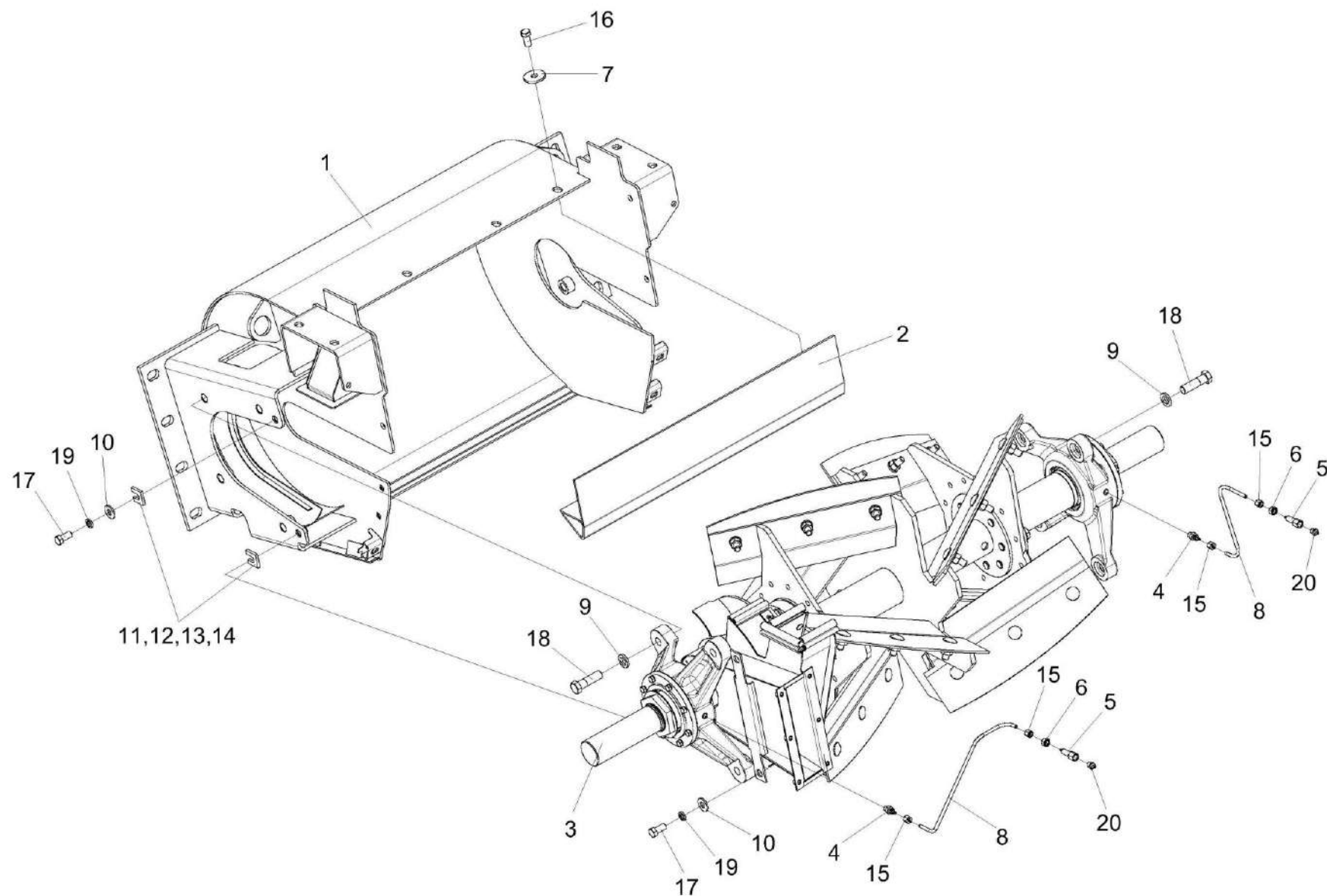
Рисунок 56 – Ускоритель выброса КВС-2-0142000 (лист 2)
