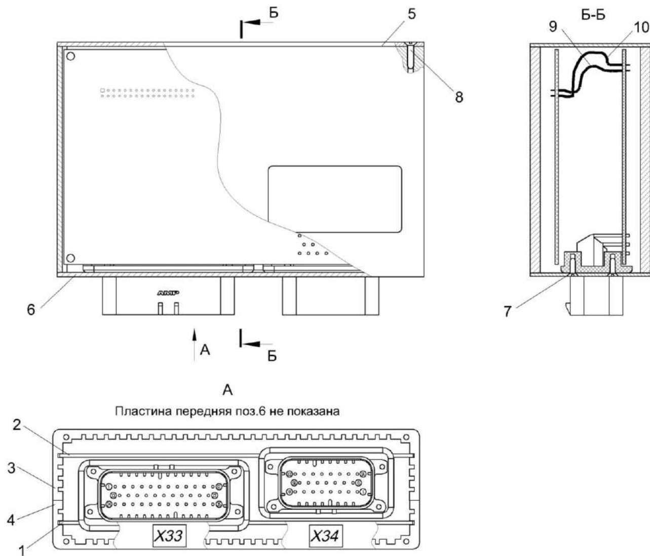
Рисунок 138 – Модуль управления питающим аппаратом КВС-8-0701400
