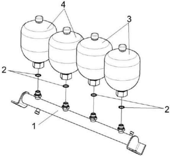
Рисунок 192 – Блок пневмогидроаккумуляторов КВС-1-0602540
