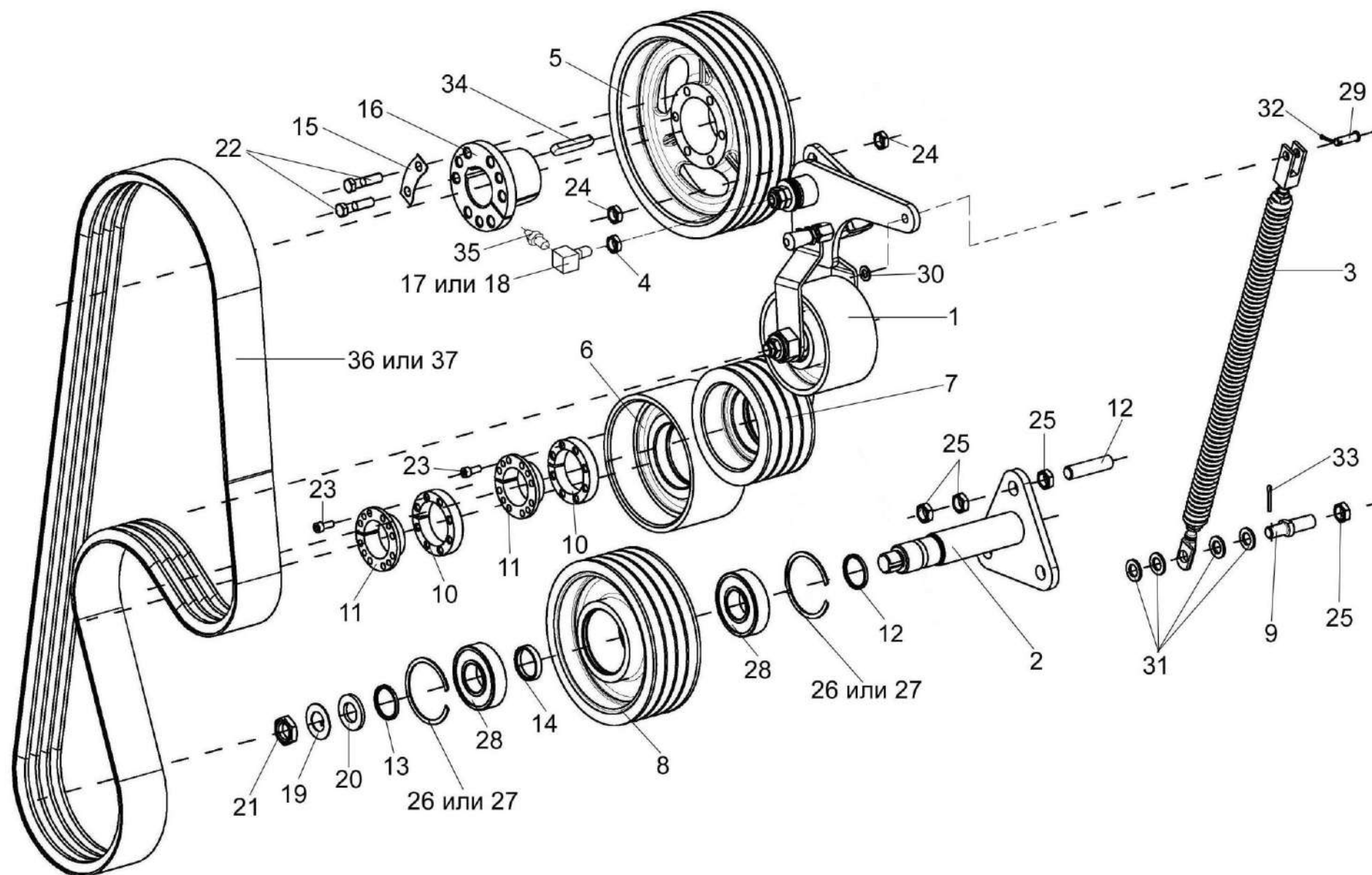
Рисунок 39 – Привод доизмельчающего устройства KBC-1-0132100
