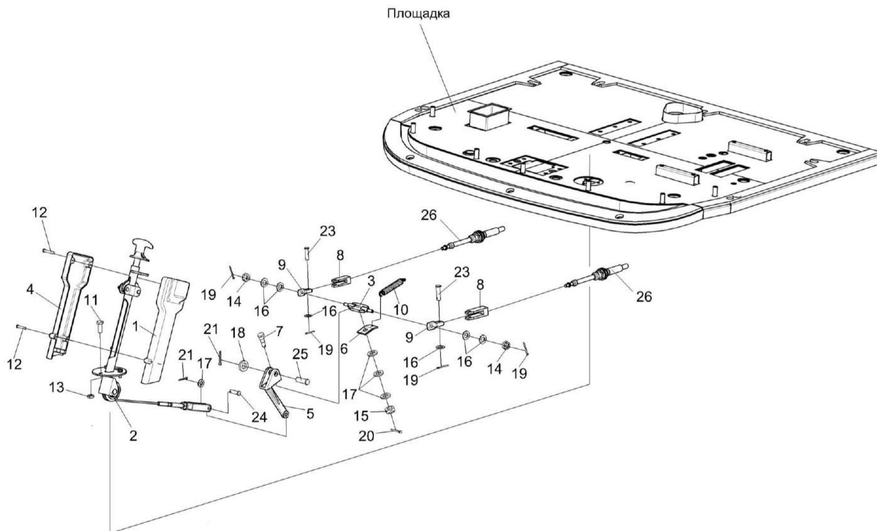
Рисунок 145 – Установка колонки привода УЭС 0300710
