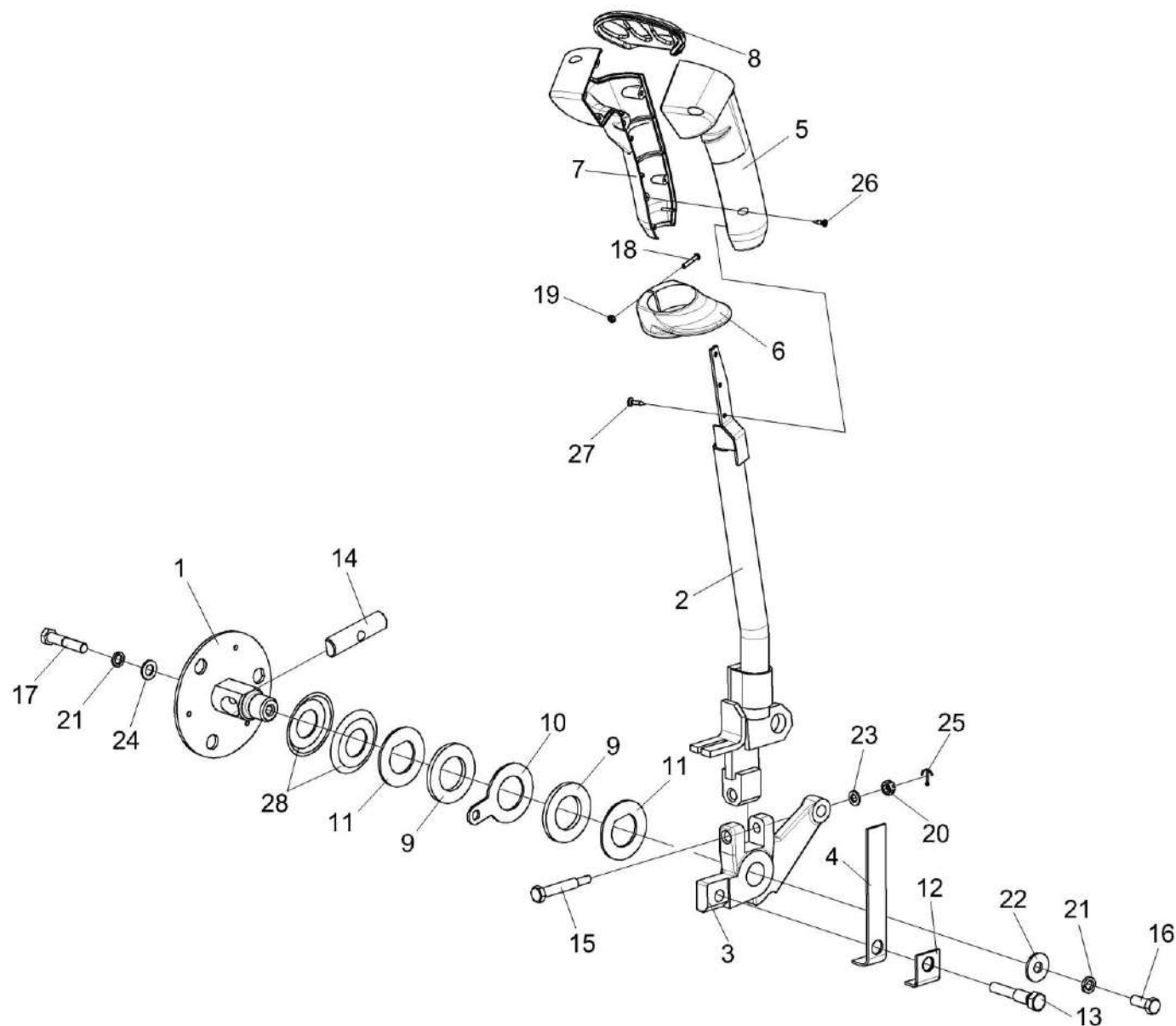
Рисунок 134 – Привод КВС-8-0129550
