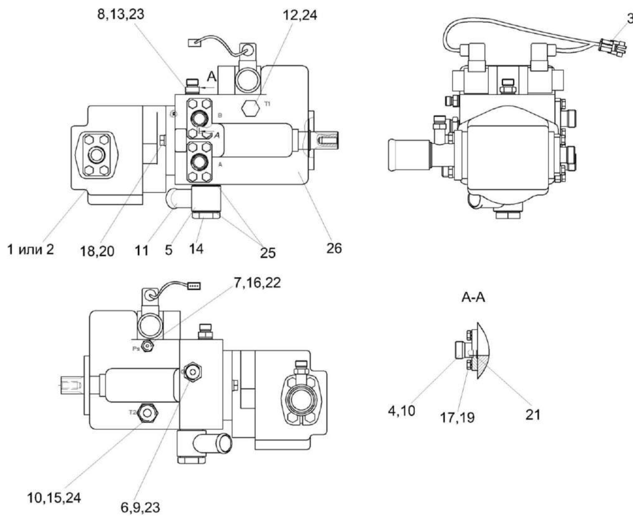
Рисунок 210 – Гидронасос двухсекционный КВС-5-0624340
