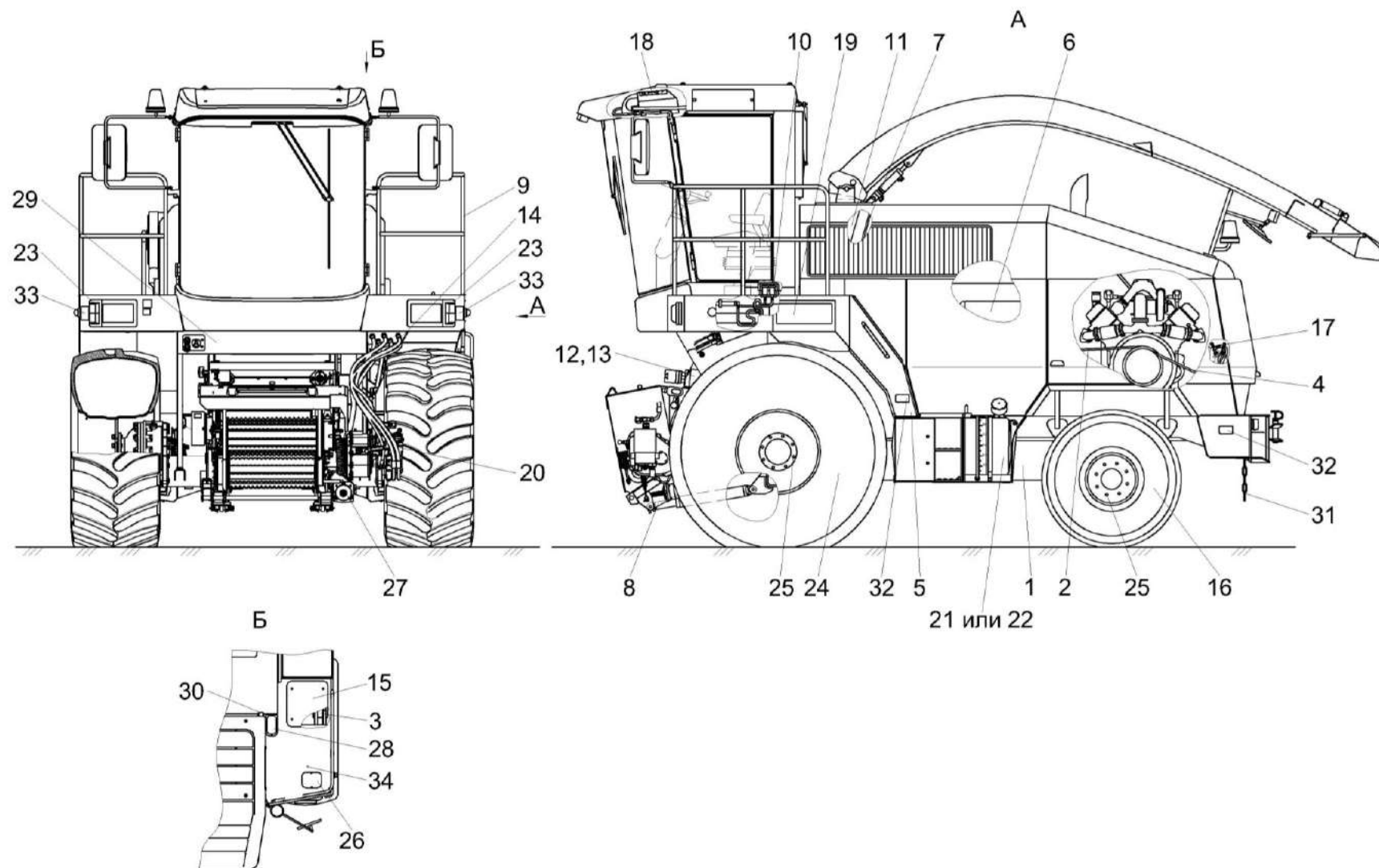
Рисунок 2 – Измельчитель самоходный КВС-8-0100000 (лист 2)
