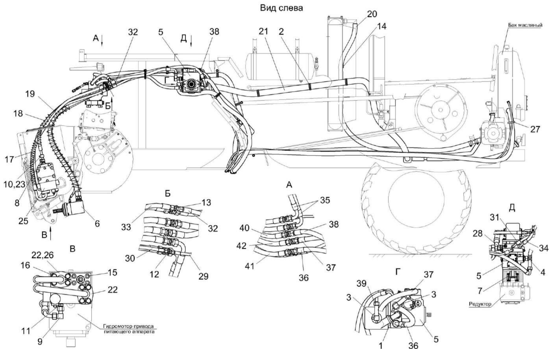
Рисунок 205 – Гидросистема привода питающего аппарата и адаптеров КВС-8-0614000 (лист 1)
