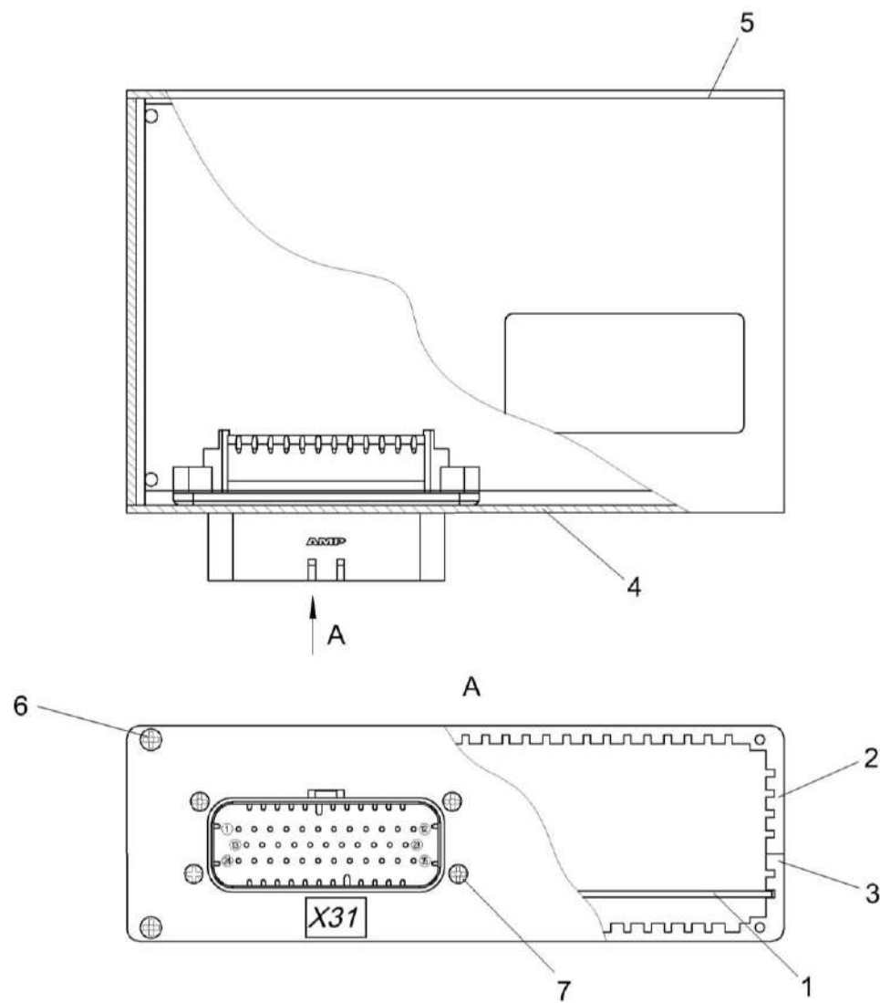
Рисунок 137 – Модуль бортиформатора КВС-8-0701100
