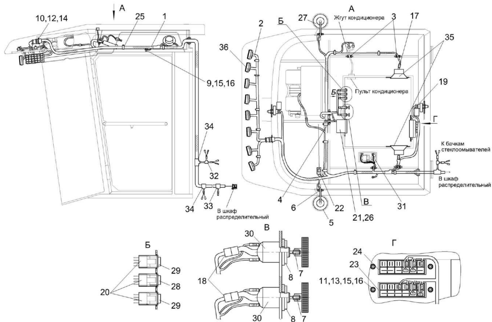
Рисунок 162 – Установка электрооборудования кабины КВС-8-0722000
