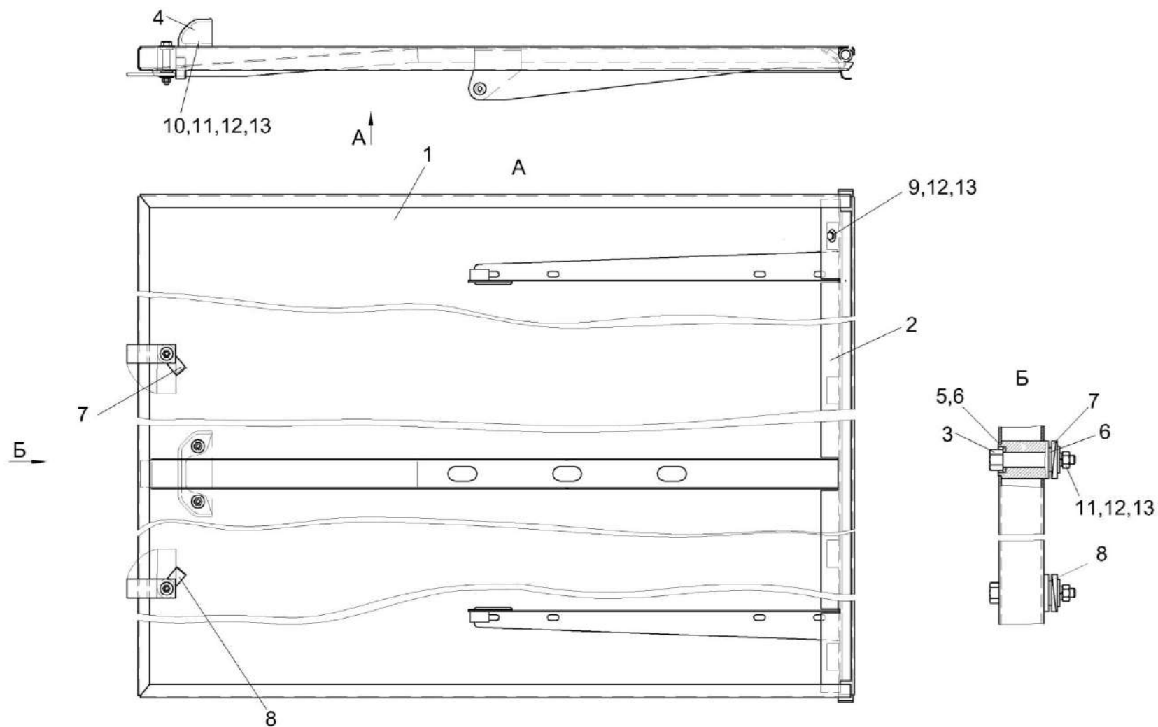
Рисунок 172 – Крышка КВС-8-0162050
