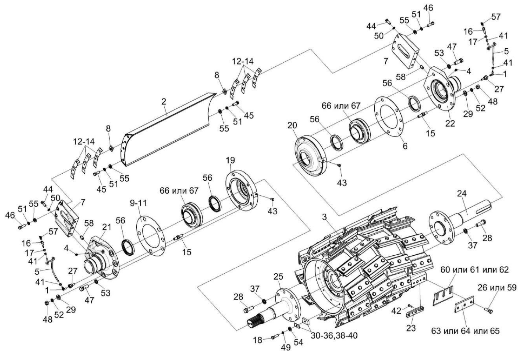
Рисунок 25 – Установка барабана КВС-2-0115430
