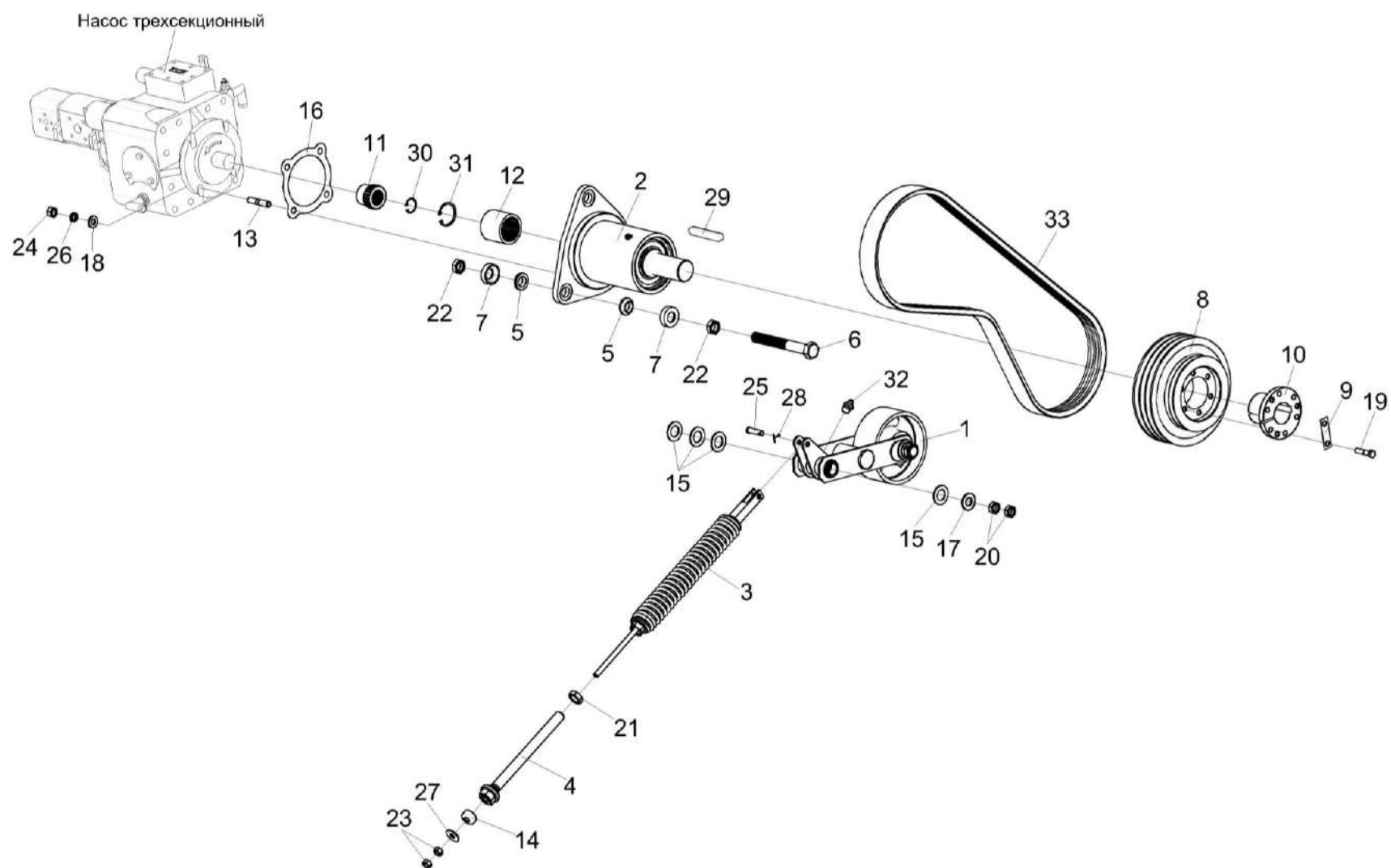
Рисунок 92 – Привод гидростата КВС-8-0133000
