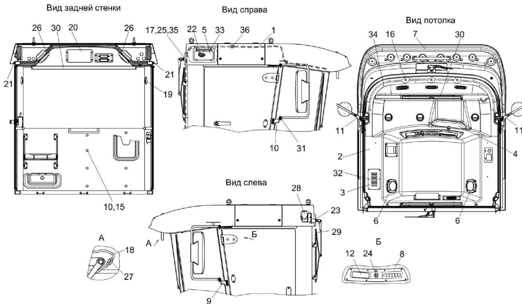
Рисунок 157 – Кабина КВС-8-0120010 (лист 2)
