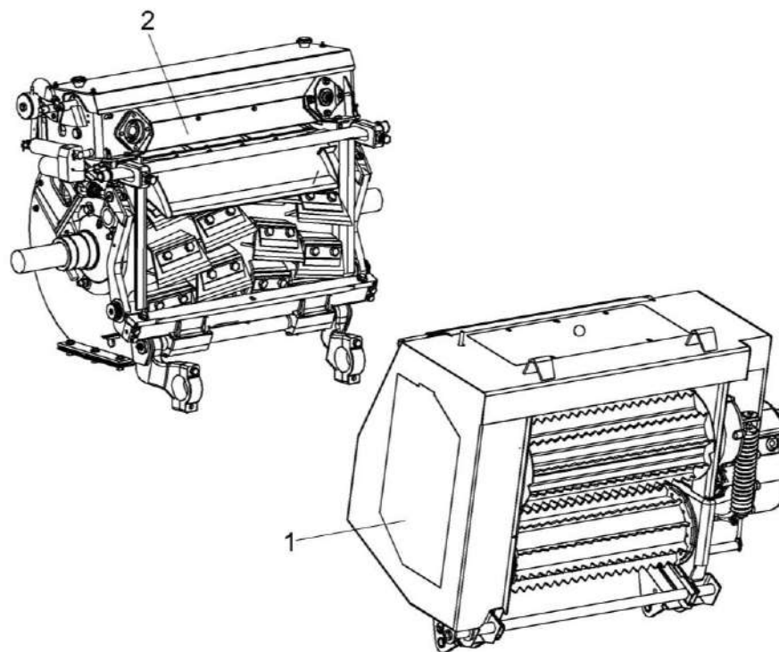
Рисунок 3 – Аппарат питающе-измельчающий КВС-8-0110000
