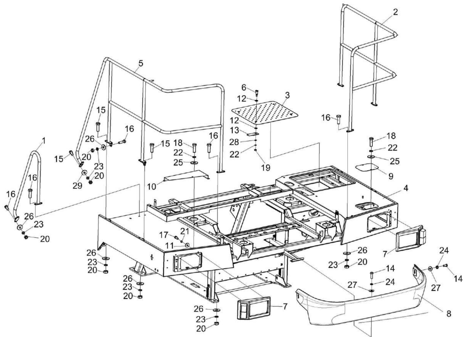
Рисунок 153 – Установка площадки входа КВС-8-0124000 (лист 1)
