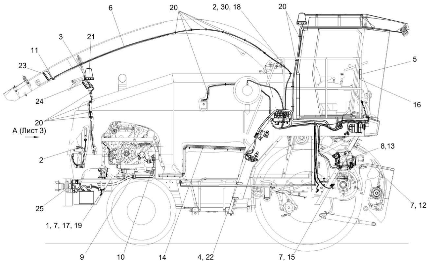
Рисунок 221 – Установка электрооборудования измельчителя КВС-8-0721000 (лист 1)
