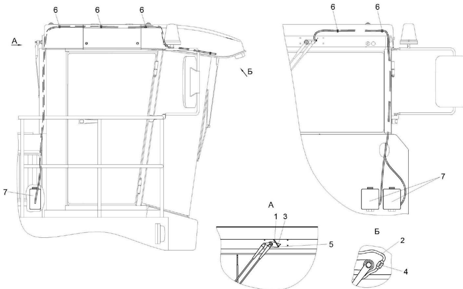
Рисунок 163 – Установка стеклоомывателей КВС-2-0122030
