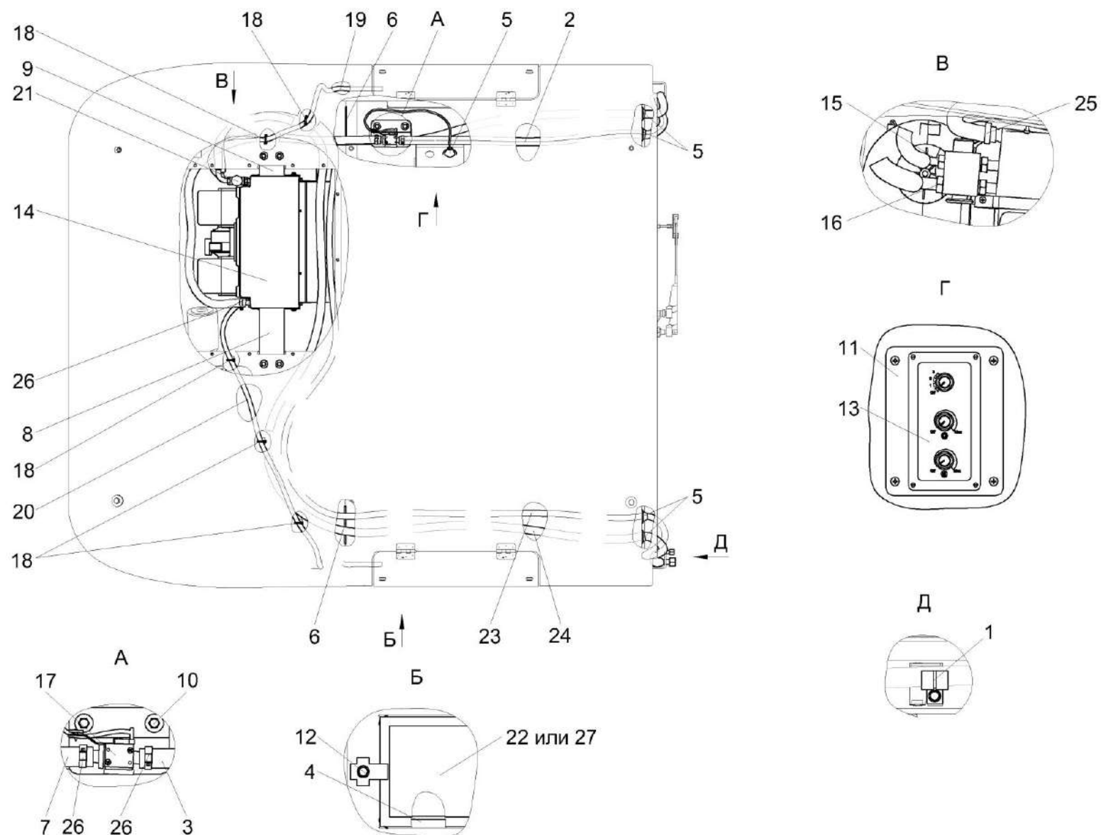
Рисунок 165 – Установка испарителя КВС-2-0121050-01
