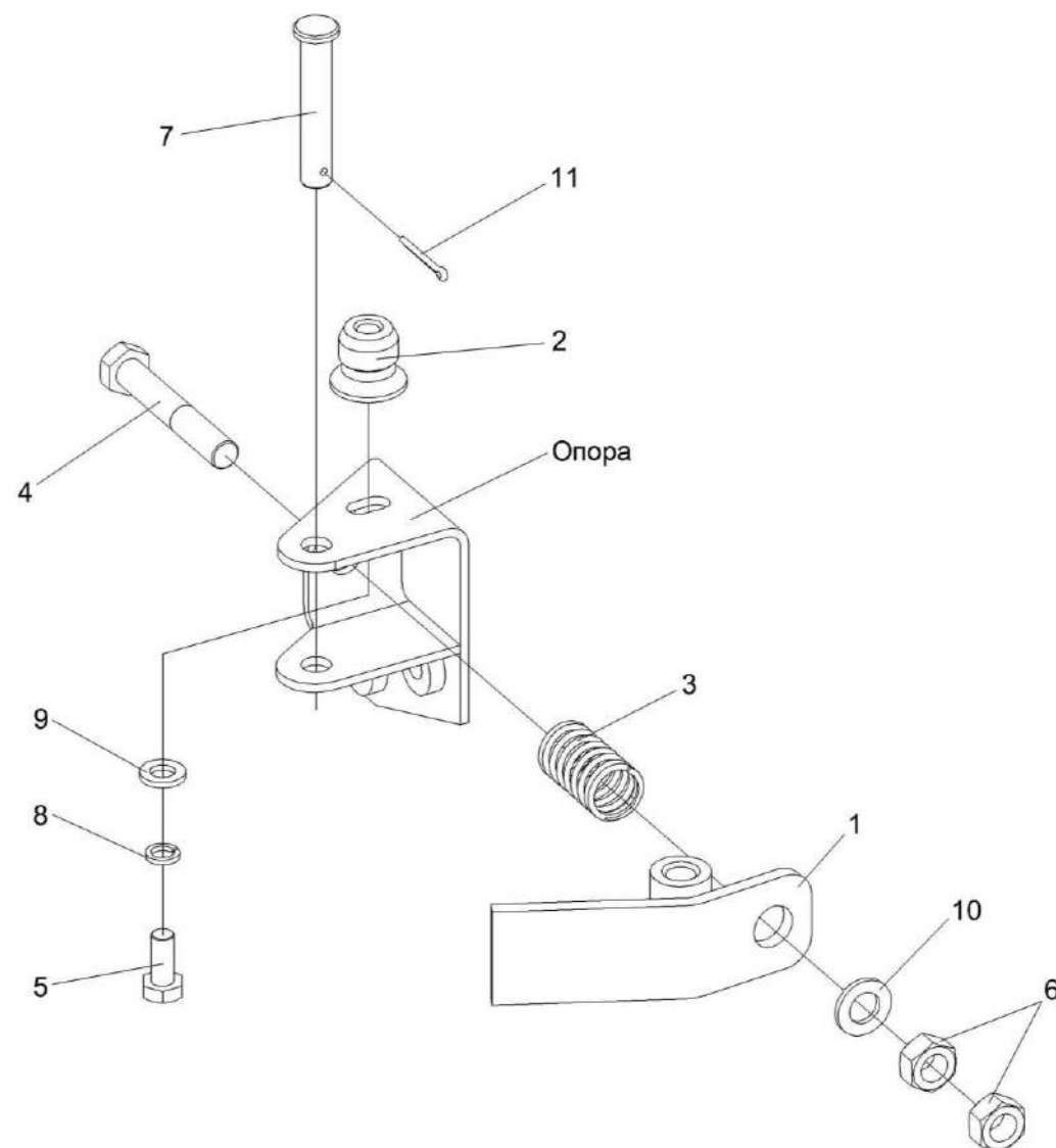
Рисунок 30 – Установка опоры КВС-2-0116550
