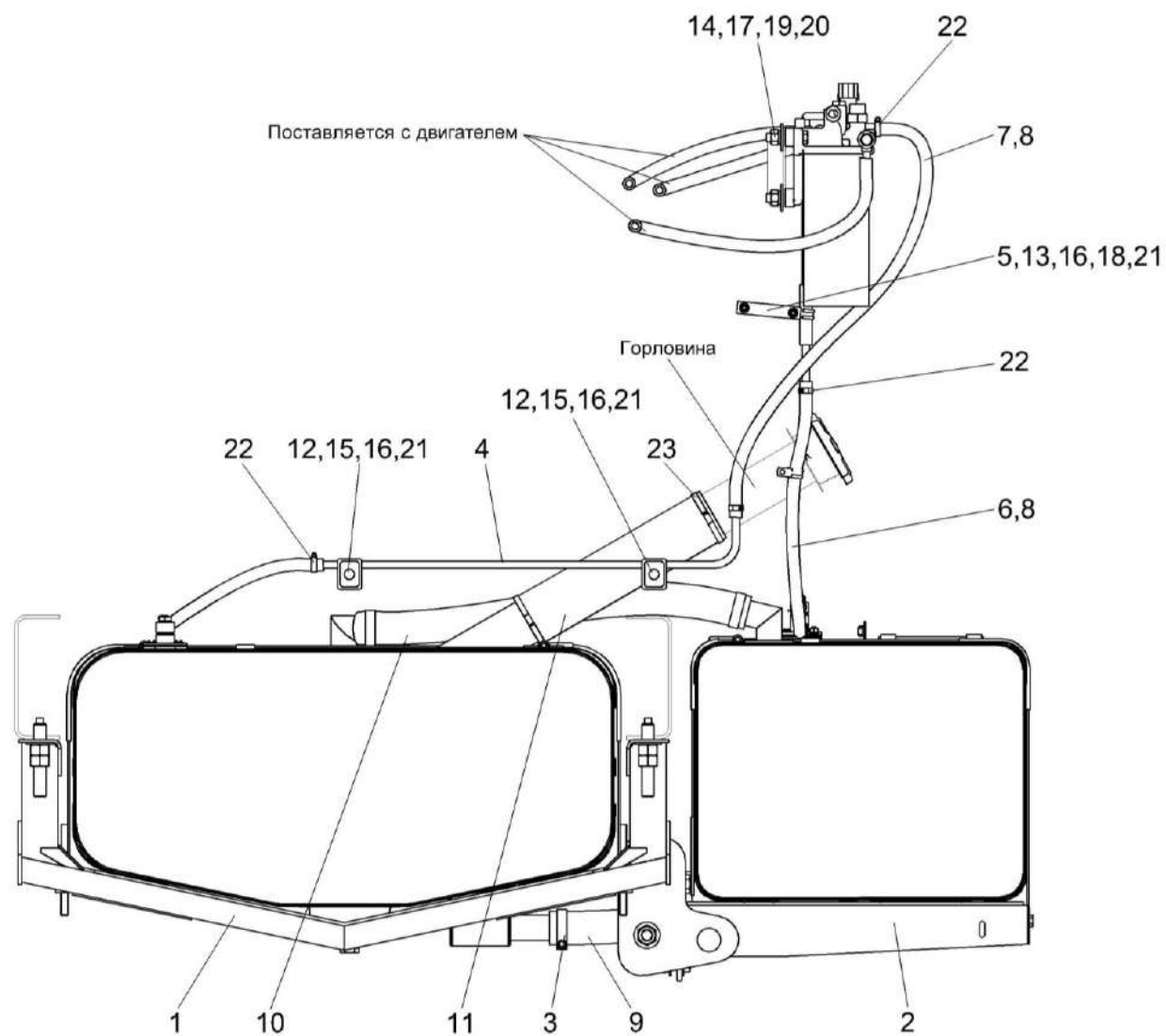
Рисунок 99 – Установка топливного оборудования КВС-8-0103000 (лист 3)
