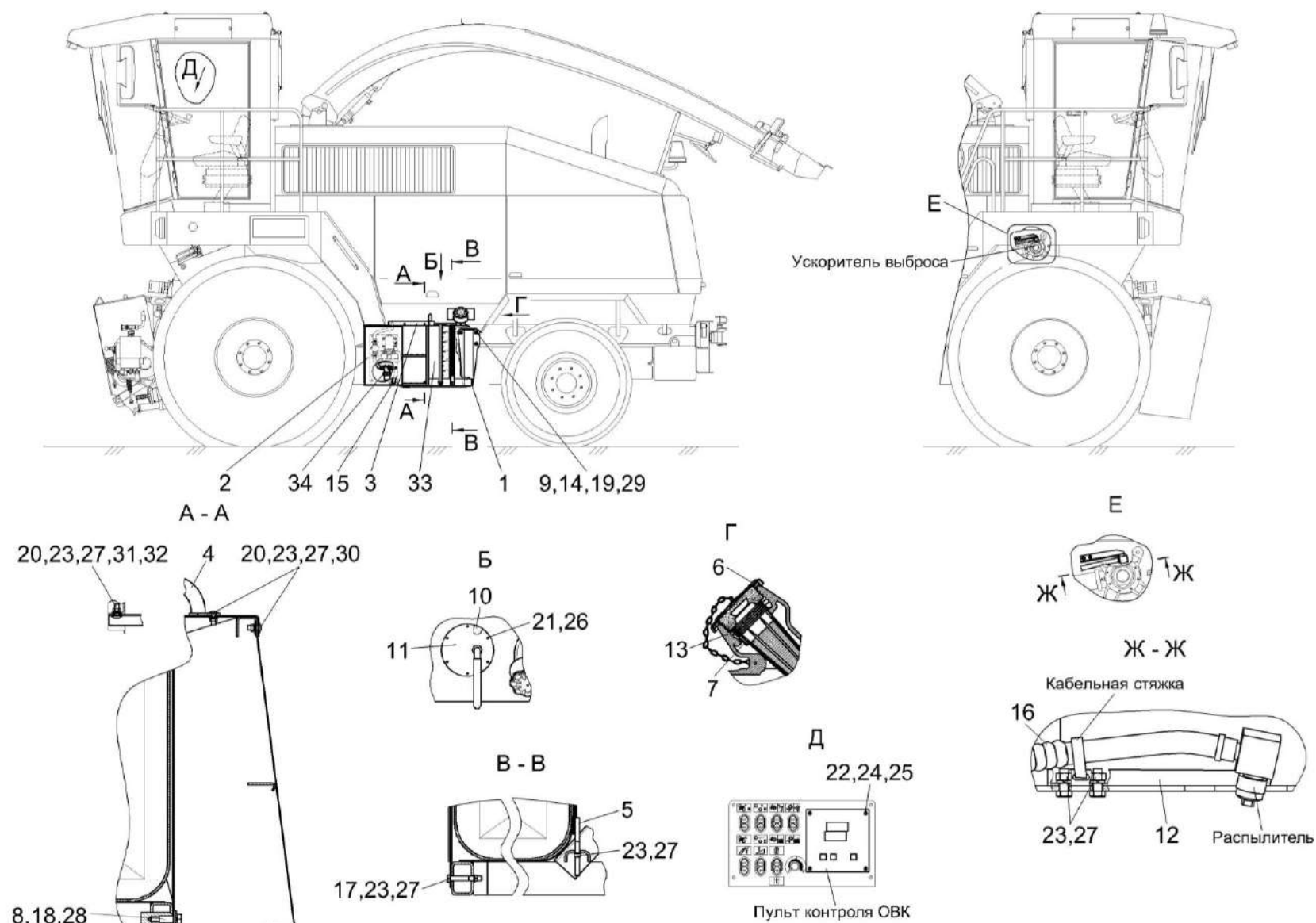
Рисунок 227 – Установка ОВК КВС-2-0900000А
