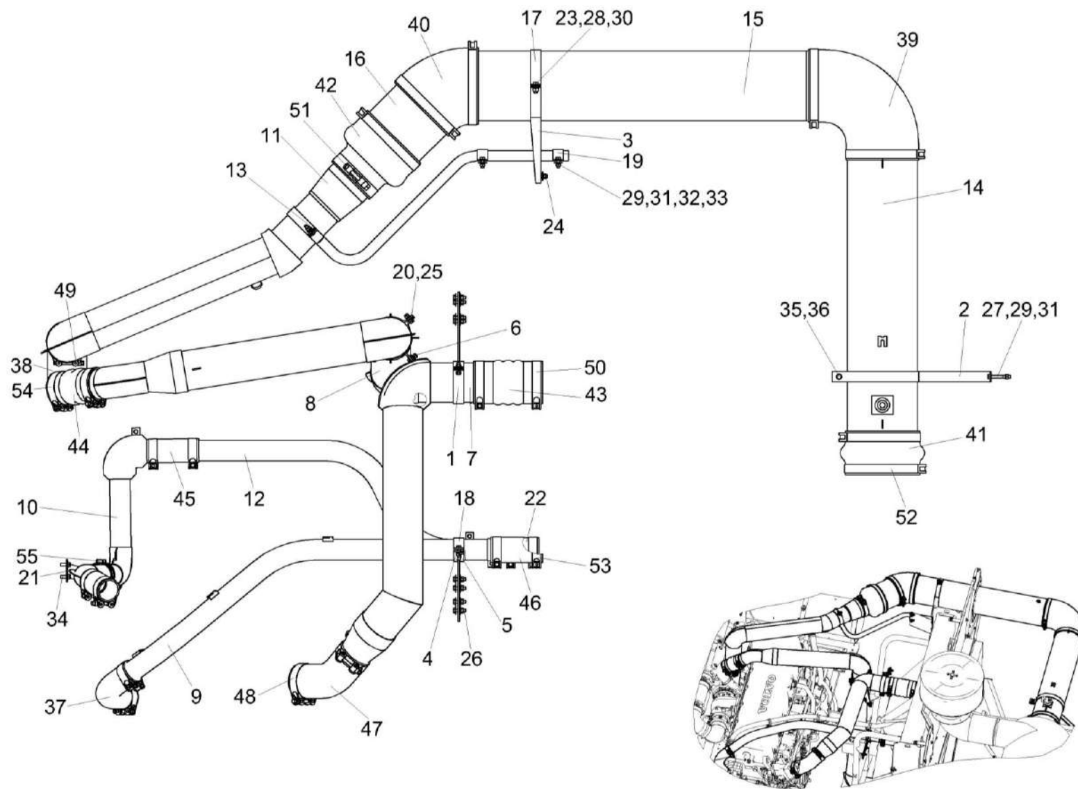
Рисунок 70 – Установка труб КВС-8-0150300
