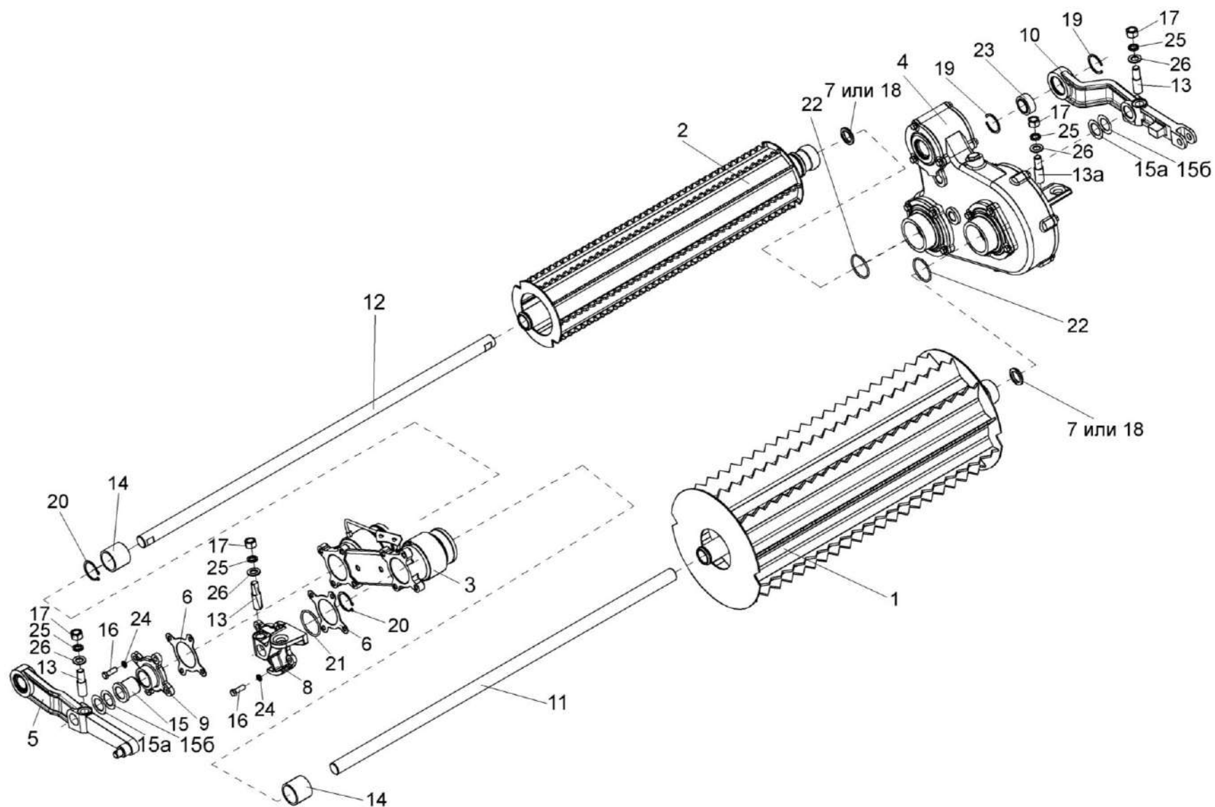
Рисунок 20 – Вальцы верхние КВС-2-0111100
