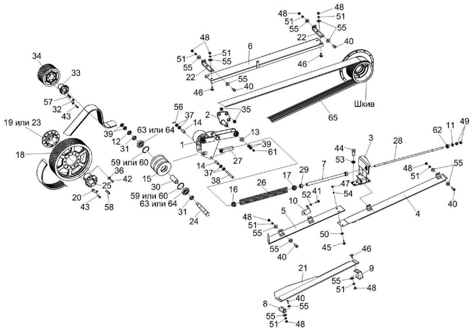
Рисунок 36 – Привод измельчающего барабана КВС-8-0130000
