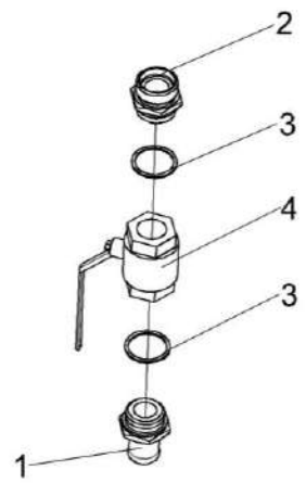
Рисунок 201 – Кран КЗК-10-0602380
