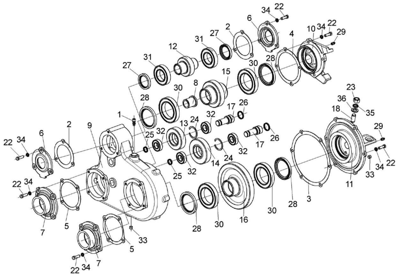
Рисунок 22 – Редуктор верхних вальцев КВС-2-0112000
