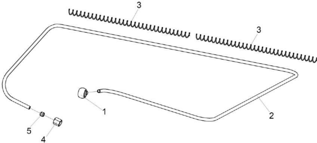
Рисунок 71 – Маслопровод КВС-8-0150500
