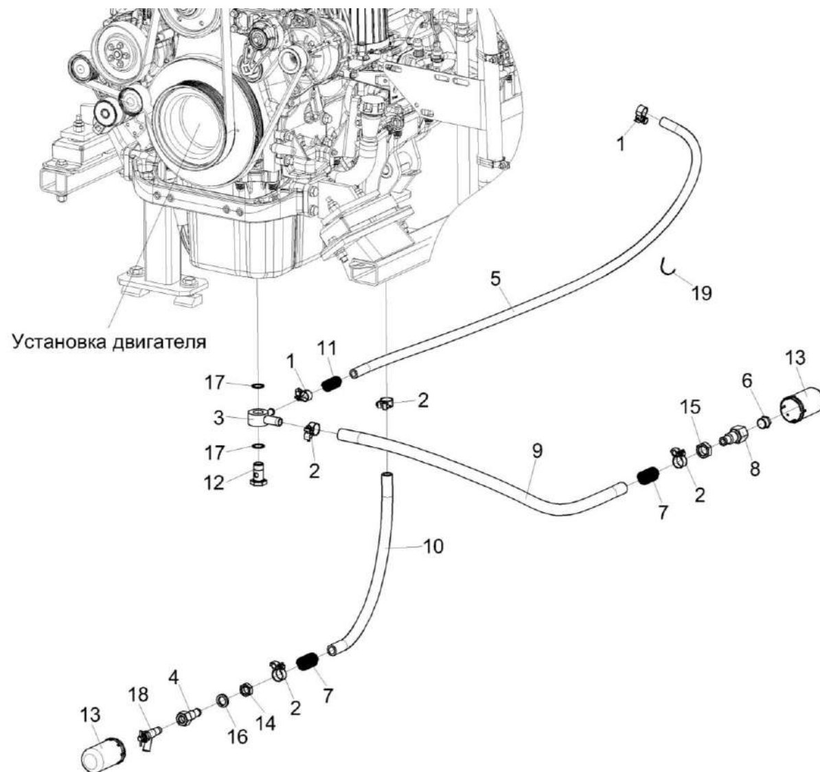
Рисунок 69 – Установка сливных рукавов КВС-8-0150260
