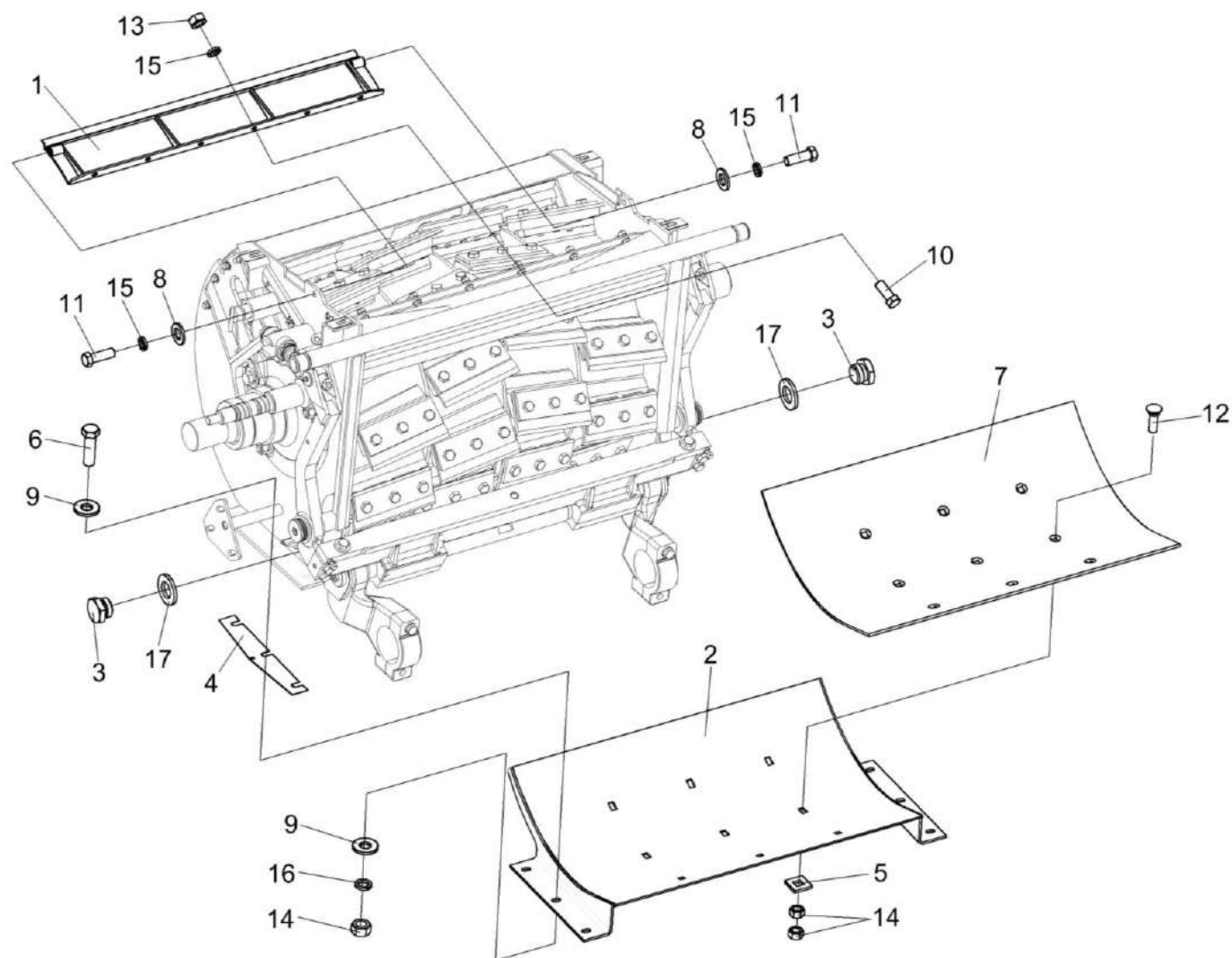
Рисунок 24 – Установка поддона КВС-2-0115050
