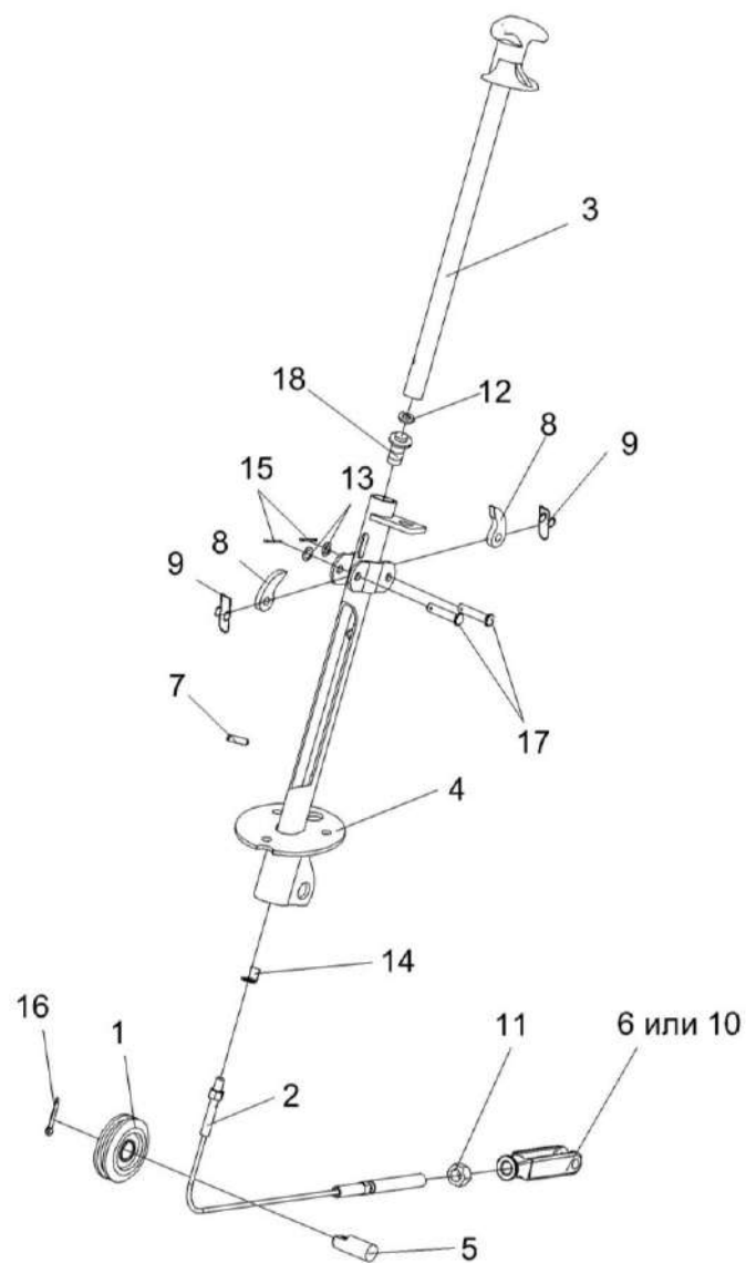
Рисунок 146 – Колонка привода УЭС 0300710
