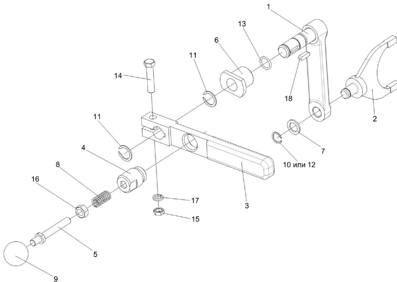
Рисунок 17 – Установка рычага КВС-2-0114020А
