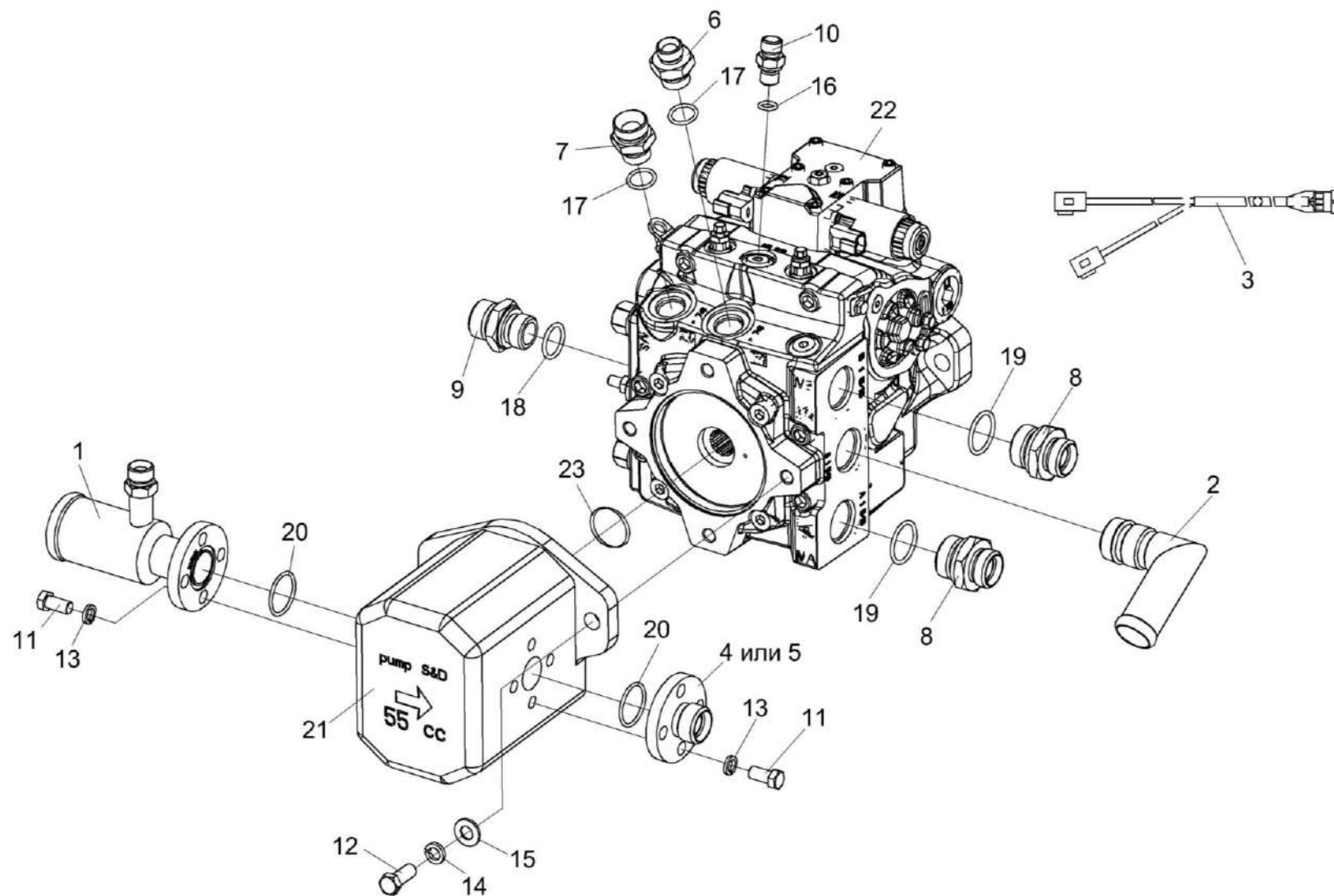
Рисунок 207 – Гидронасос двухсекционный КВС-5-0614340
