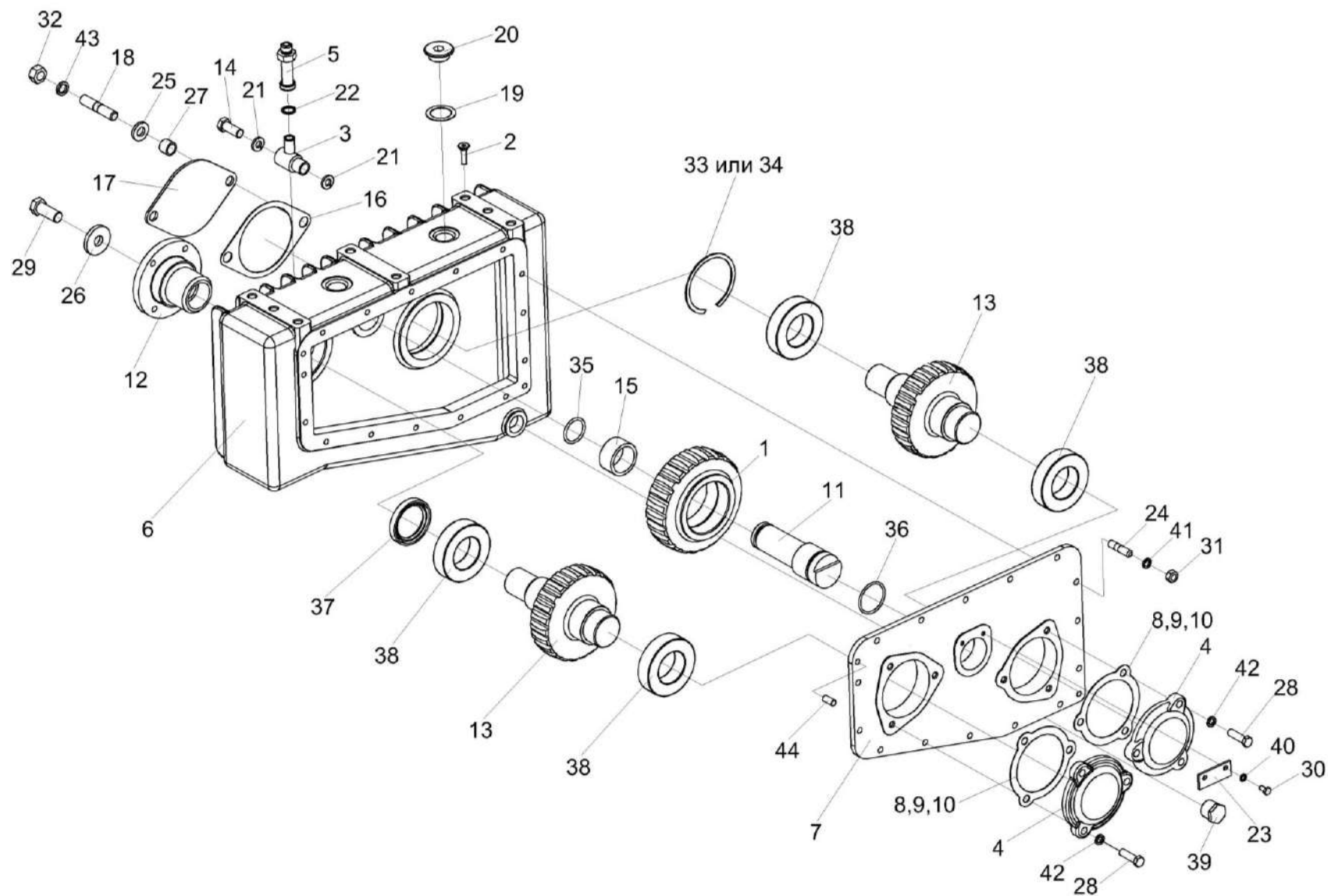
Рисунок 176 – Редуктор КВС-2-0104100
