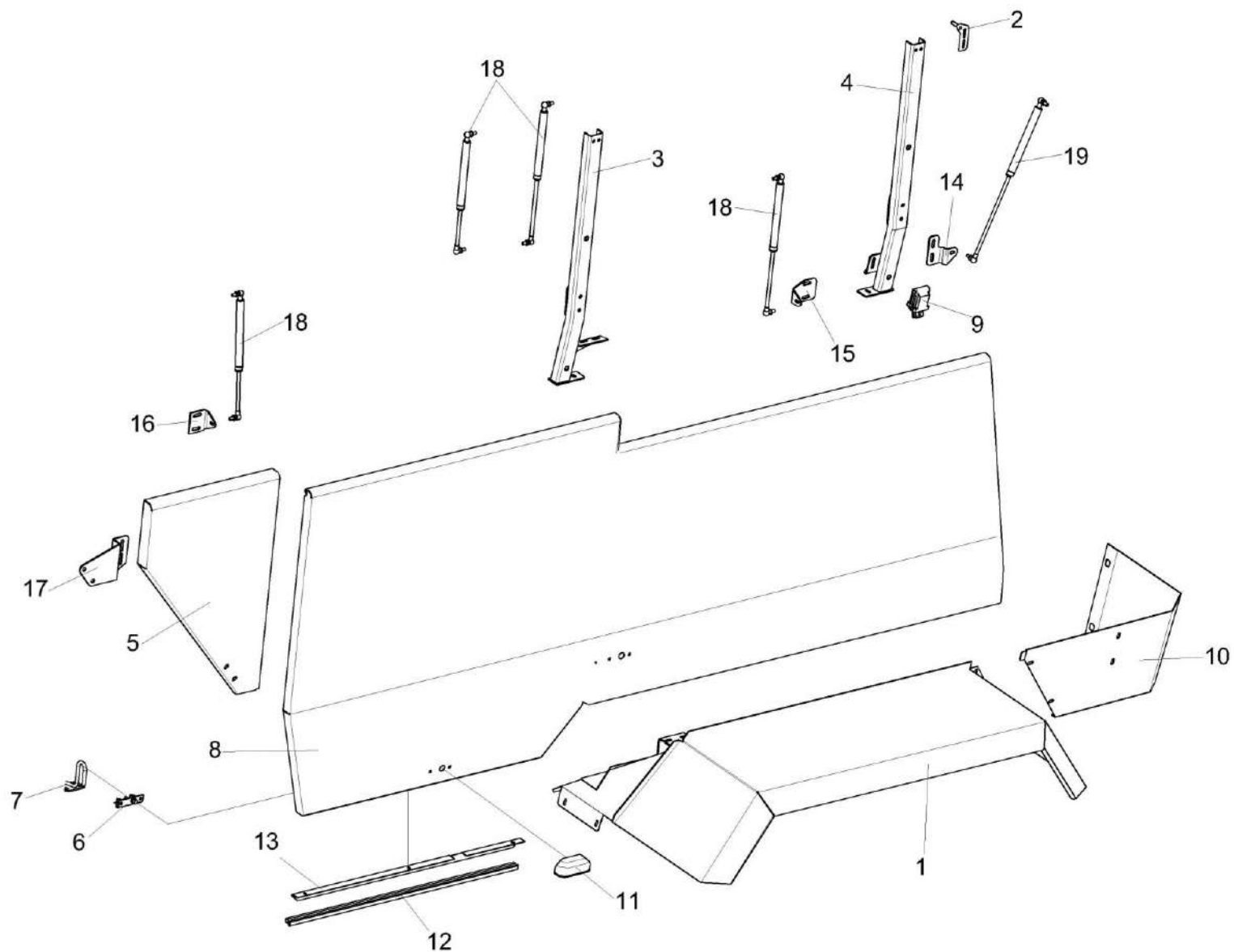
Рисунок 166 – Установка капотов КВС-8-0160000 (лист 1)
