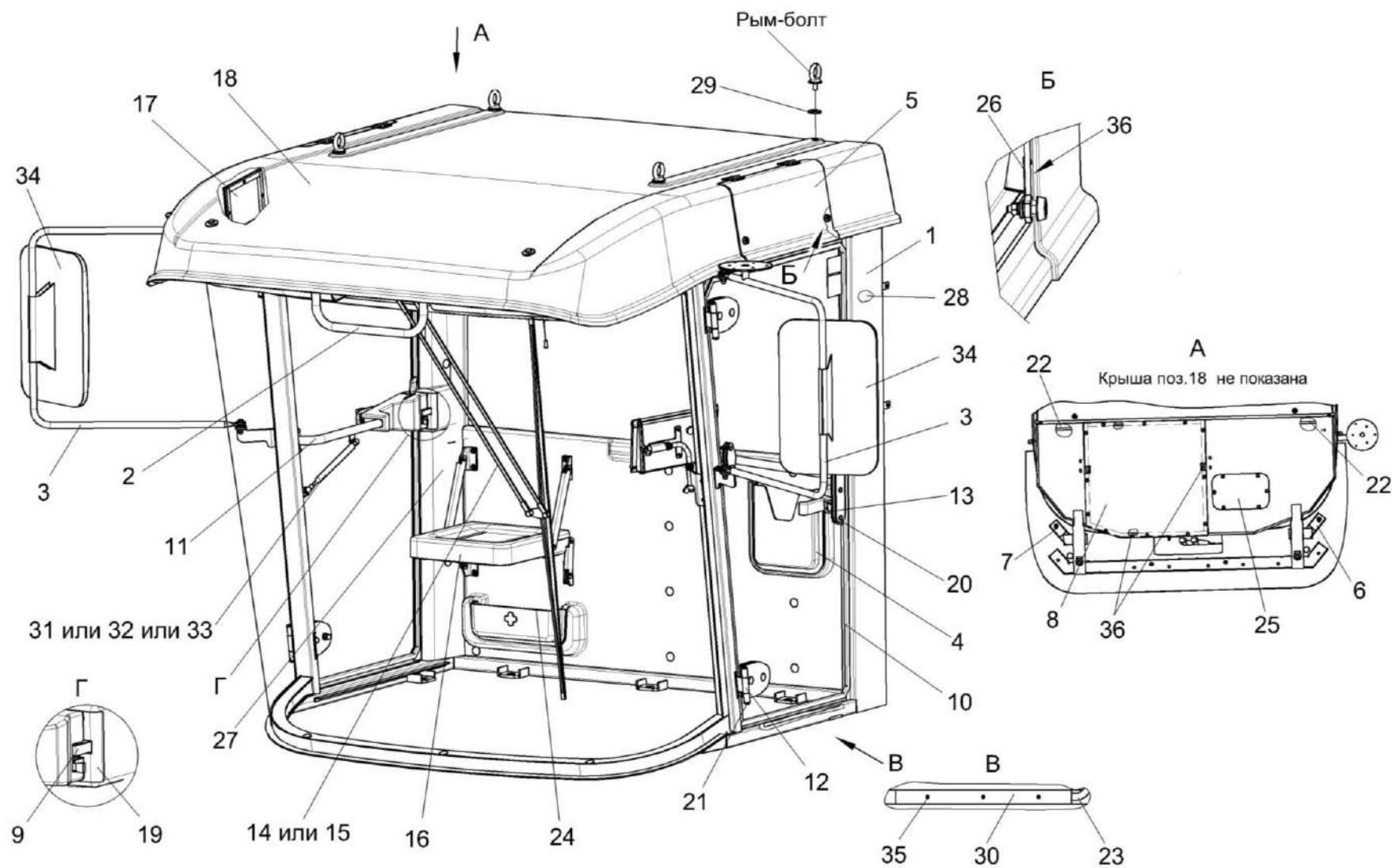
Рисунок 156 – Кабина КВС-8-0120010 (лист 1)
