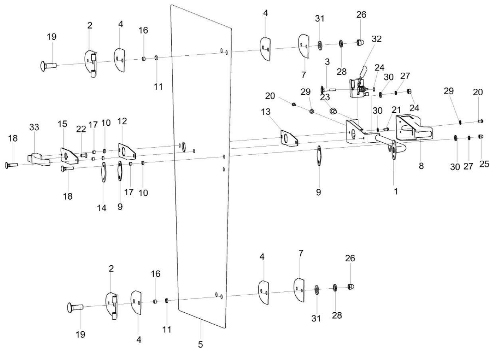
Рисунок 159 – Дверь КЗК-12-0120870-01
