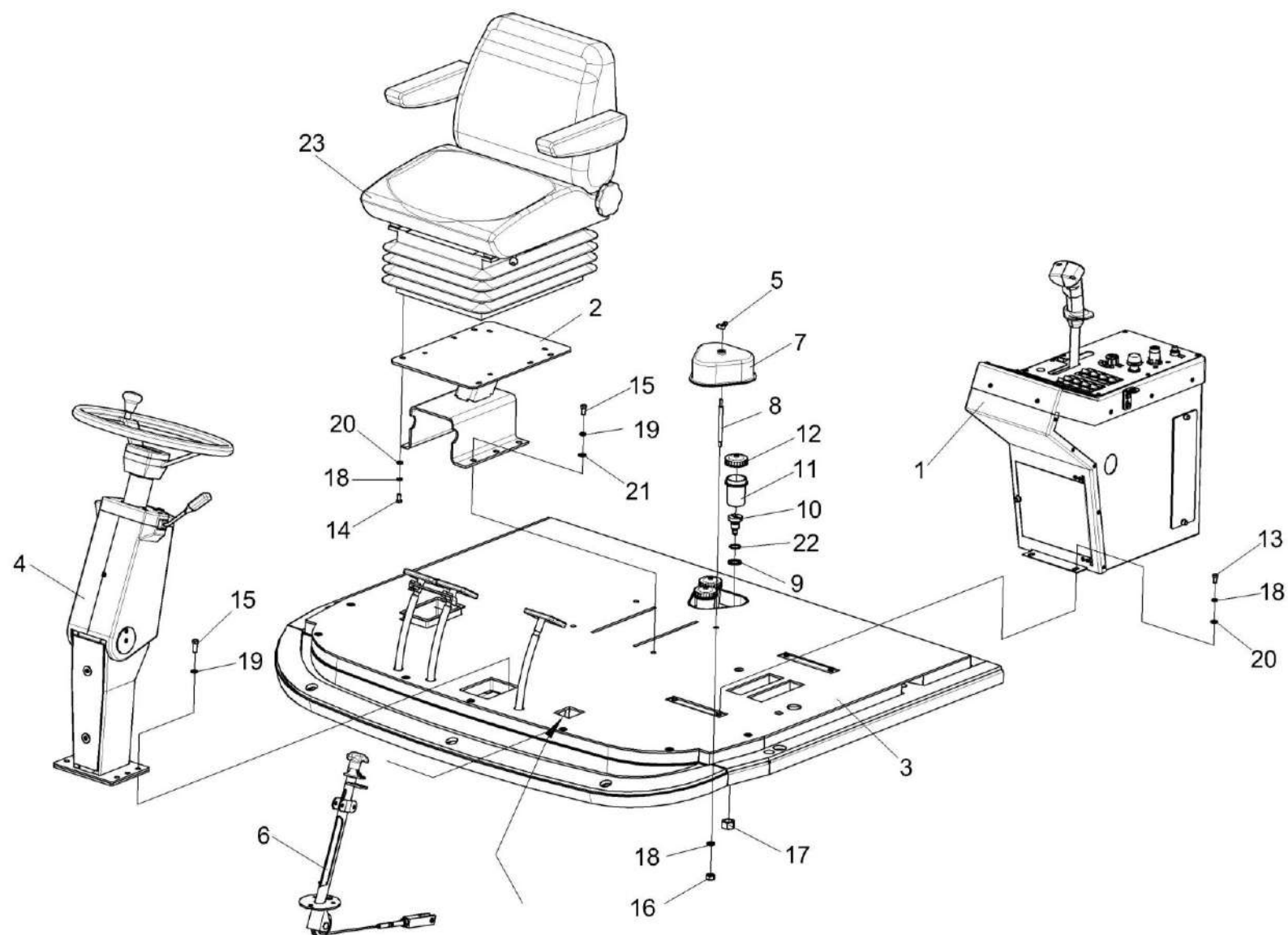
Рисунок 127 – Площадка управления КВС-8-0129000 (лист 1)
