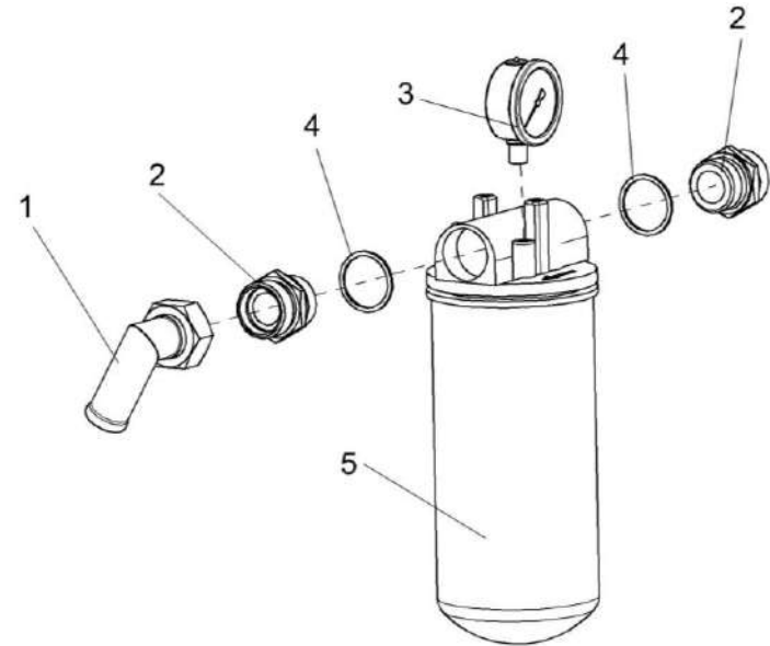
Рисунок 194 – Фильтр сливной КВС-2-0602020-01
