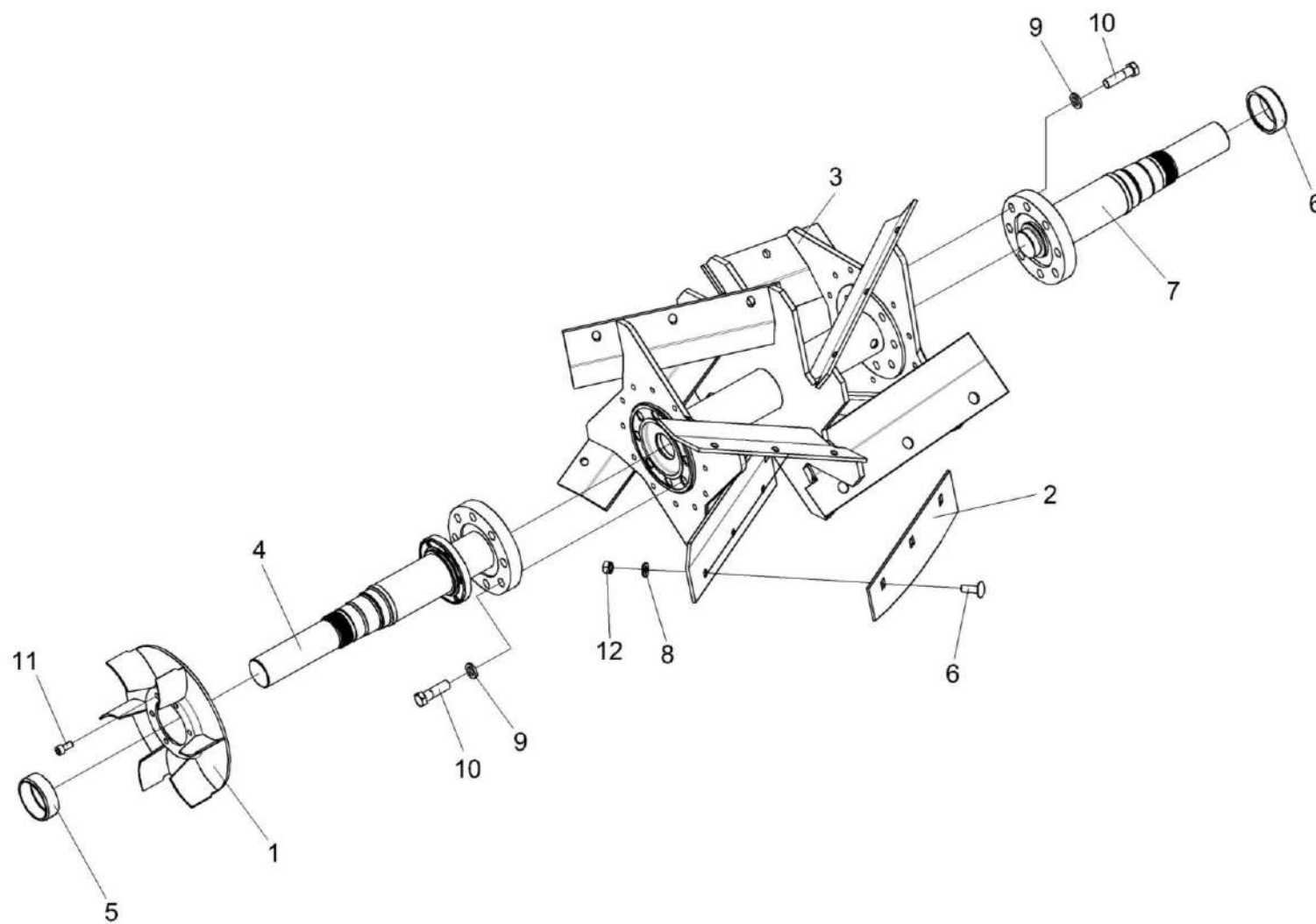
Рисунок 58 – Вал ускорителя выброса КВС-1-0142910А
