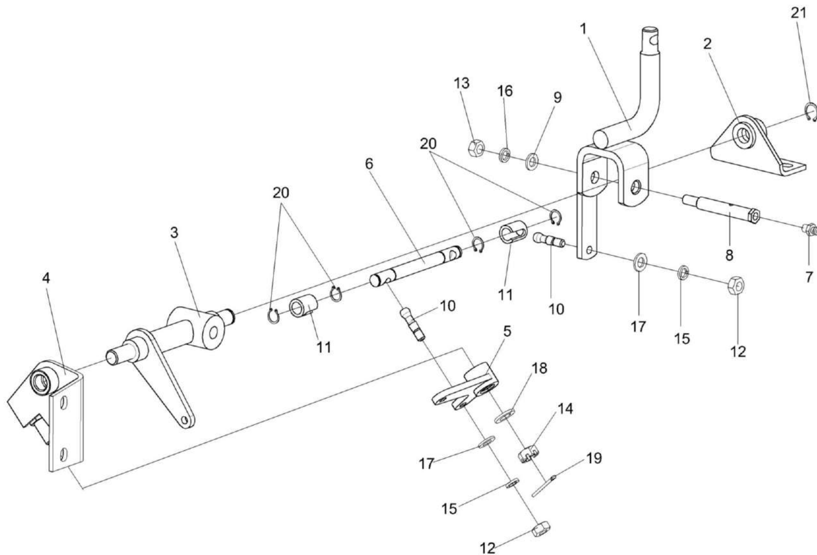
Рисунок 148 – Блок переключения КВС-2-0129070
