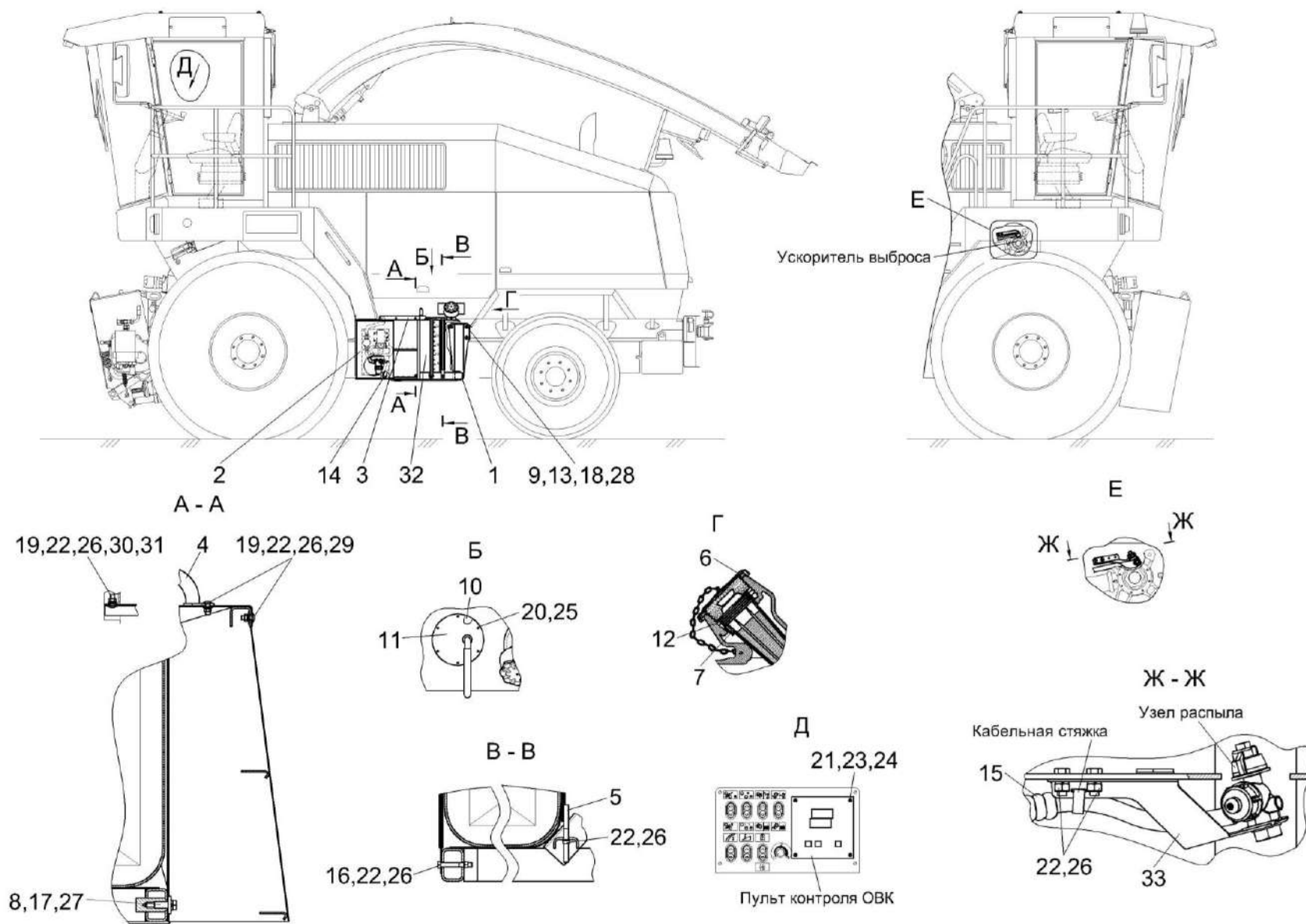
Рисунок 228 – Установка ОVK КВС-2-0900000А-01
