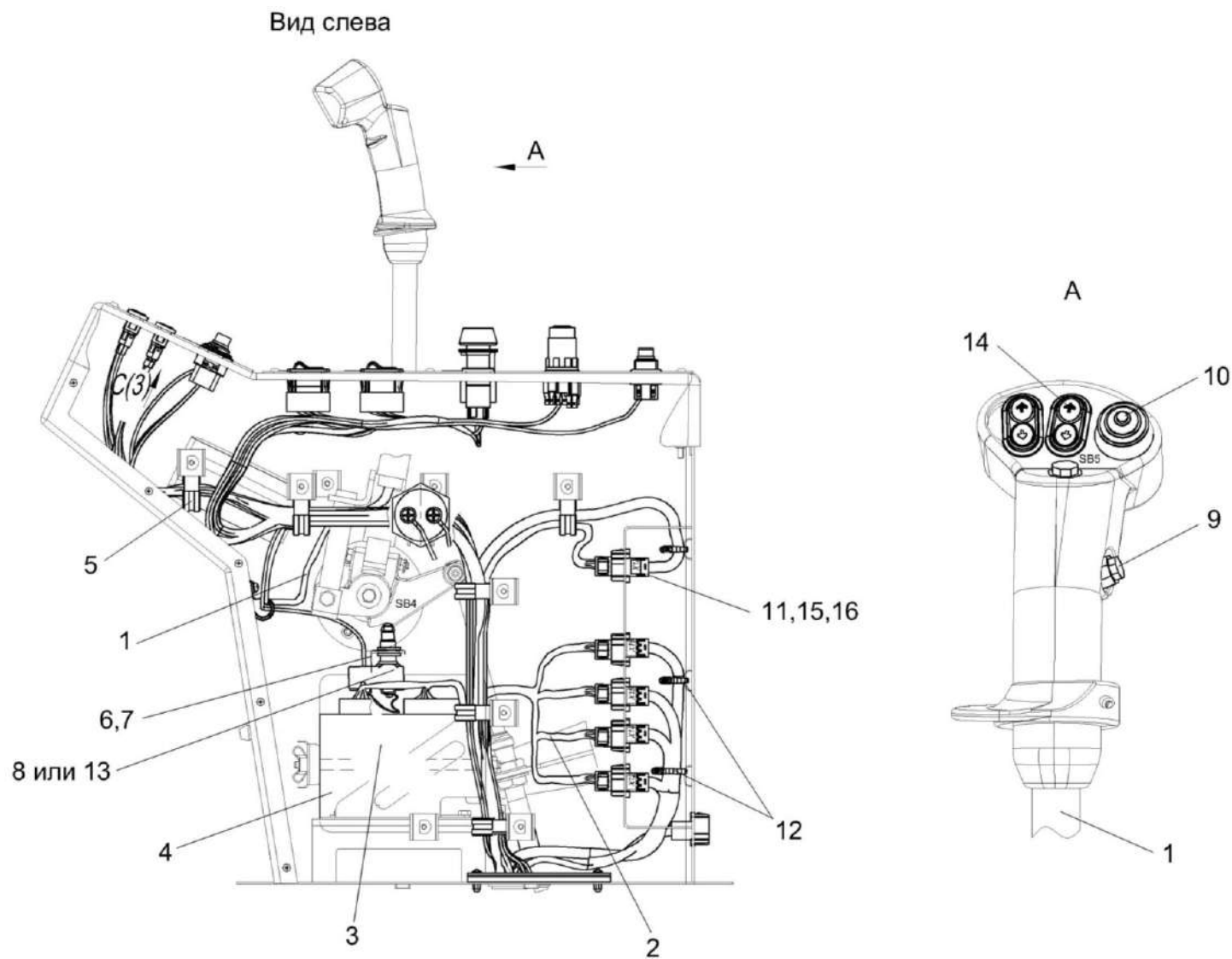
Рисунок 136 – Установка электрооборудования пульта управления КВС-8-0725000 (лист 2)
