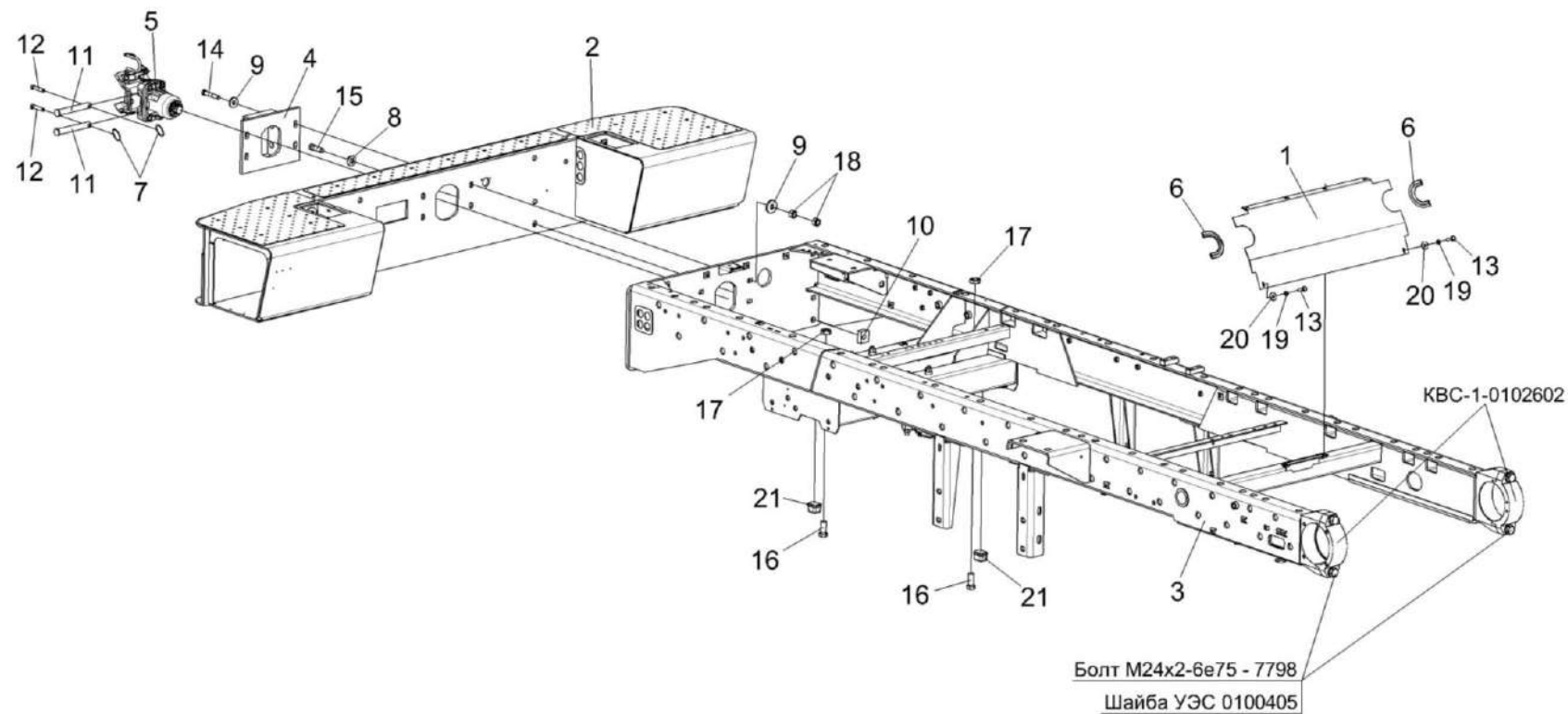
Рисунок 100 – Шасси КВС-8-0101000-01 (лист 1)
