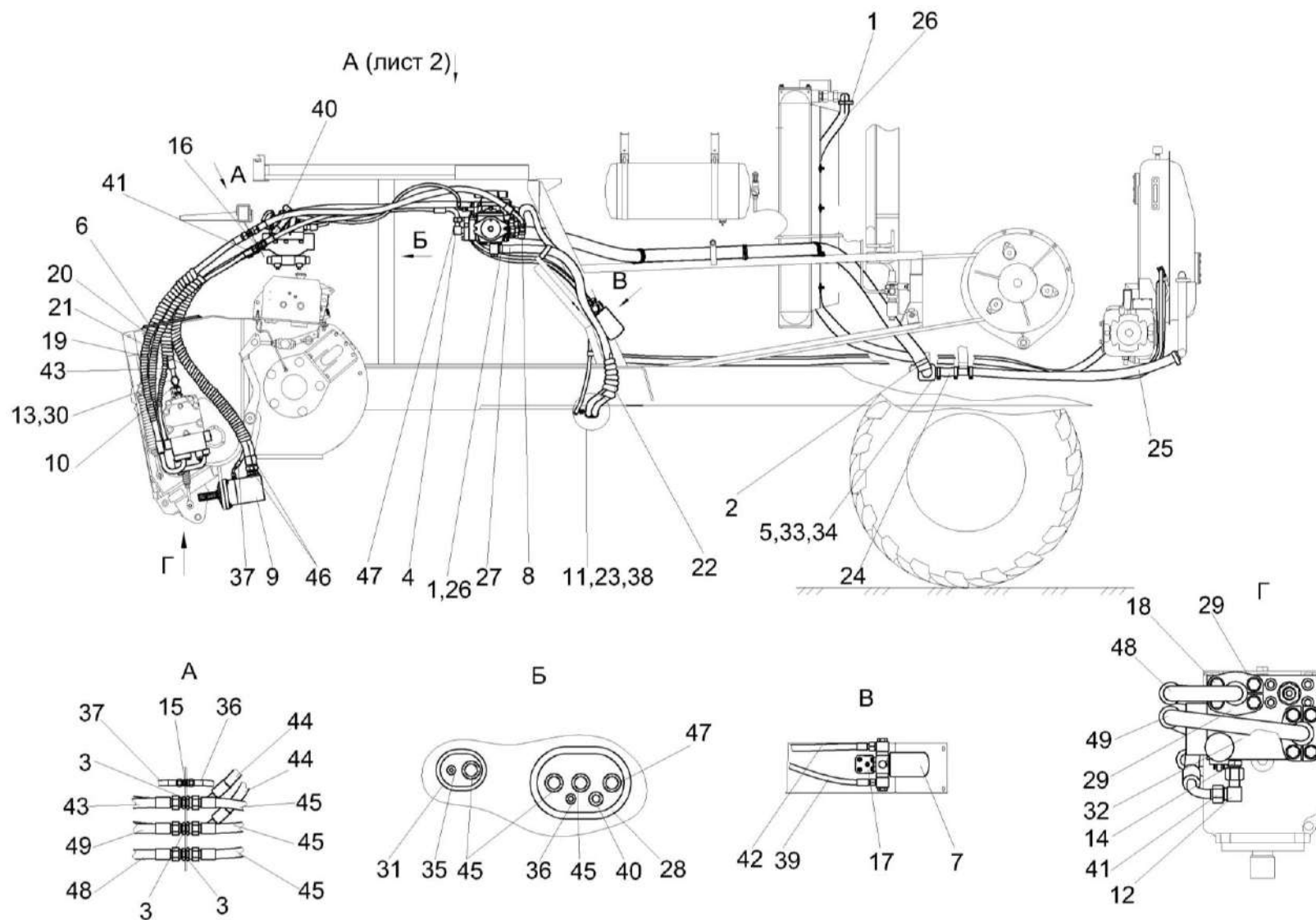
Рисунок 202 – Гидросистема привода питающего аппарата и адаптеров КВС-8-0604000 (лист 1)
